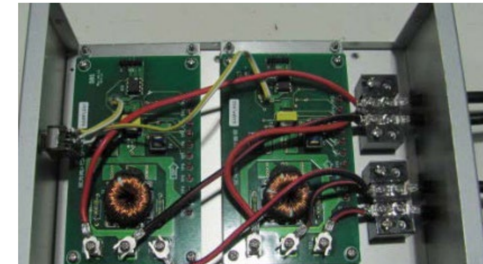
図 配分回路の外観
