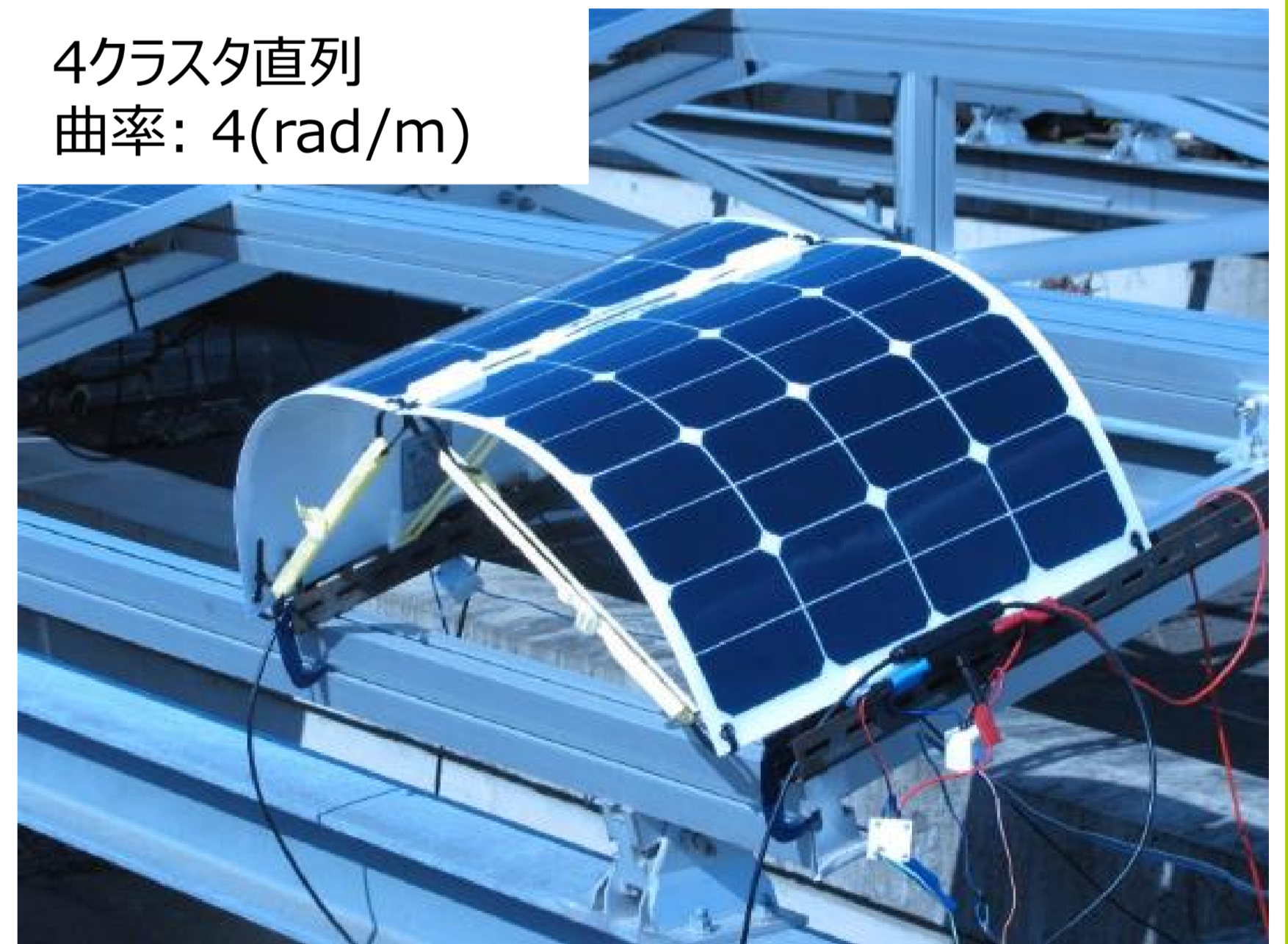
ALLPOWERS ソーラー パネル P max :50 W×2枚
