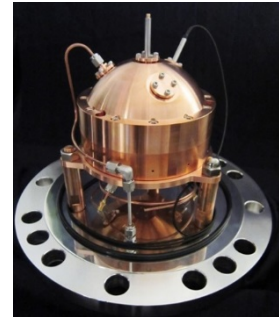
音響気体温度計の擬球形共鳴器
