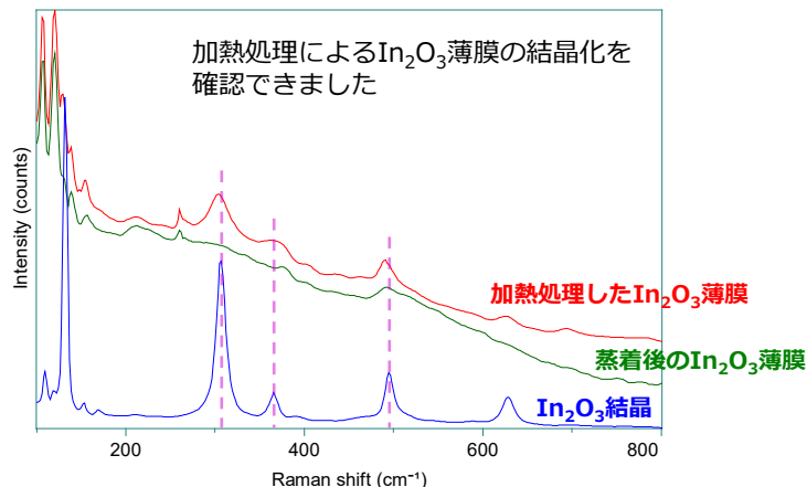
金属基板上に形成したIn 2 O 3 薄膜の結晶化評価
