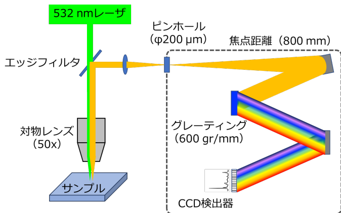
薄膜評価に用いた顕微ラマン分光装置の概要
