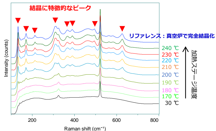
加熱によるSi基板上に形成した薄膜 ( \text{In}_2\text{O}_3 ) の結晶化の追跡評価
