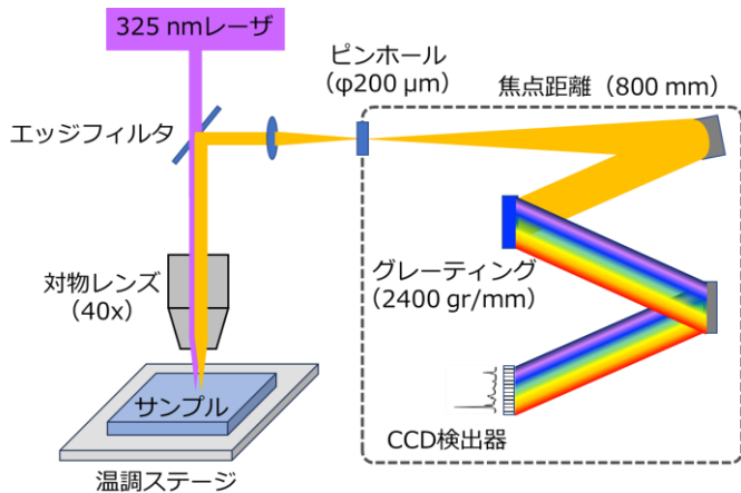
薄膜評価に用いた顕微ラマン分光装置の概要
