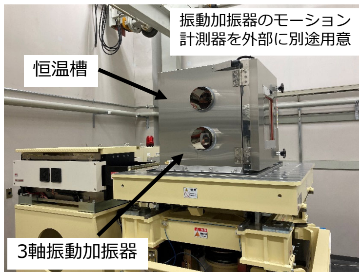
温湿度に対する加速度センサの周波数応答評価装置
