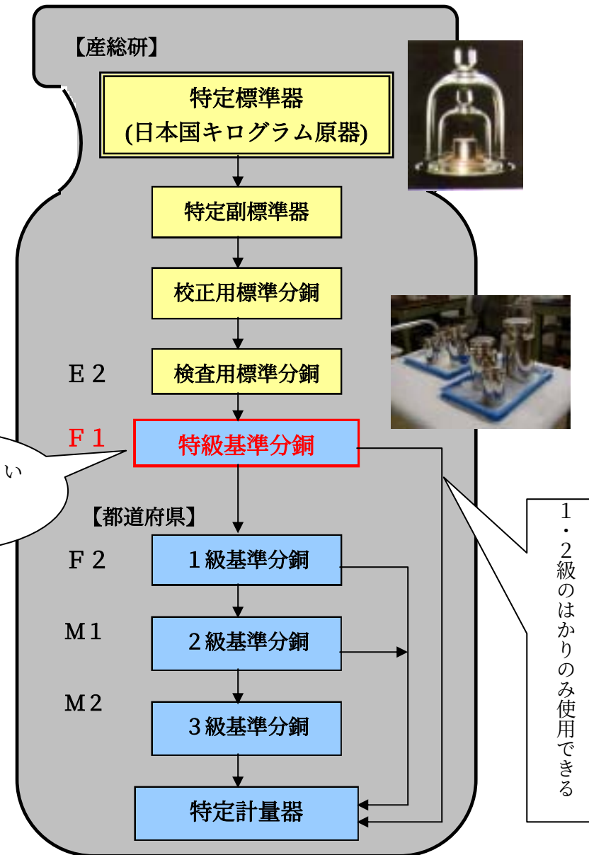
分銅体系図
