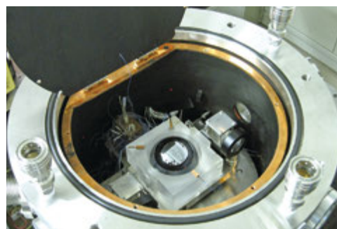
2018年に実施されたキログラムの定義改定に貢献した、NMIJが開発したシリコン単結晶球体直径測定用レーザー干渉計
