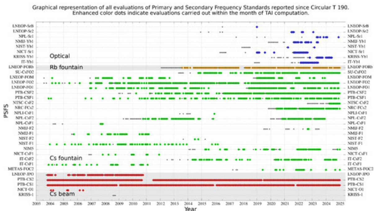
各国の一次及び二次周波数標準の TAI 校正への寄与。光時計による寄与が増大しつつある。
