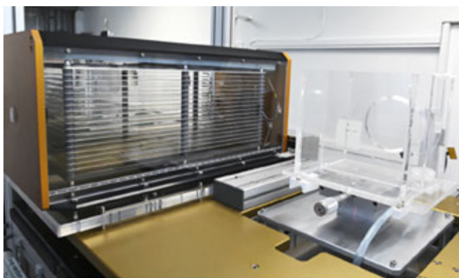
更新した一次標準自由空気電離箱と水ファントム
