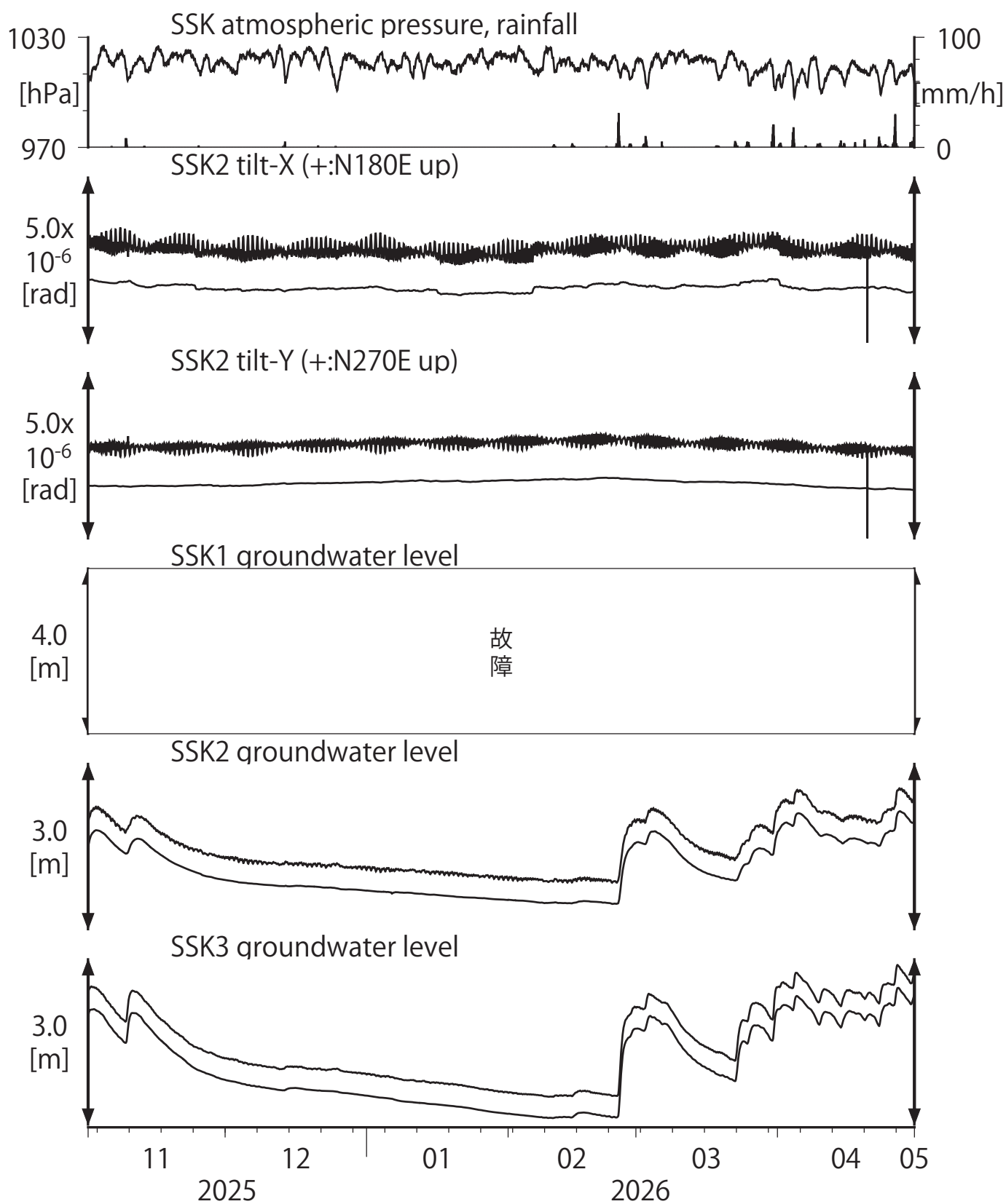
第30図 Tilt and groundwater level at SSK (時間値) (2025/11/01 00:00 - 2026/05/01 00:00 (JST))
