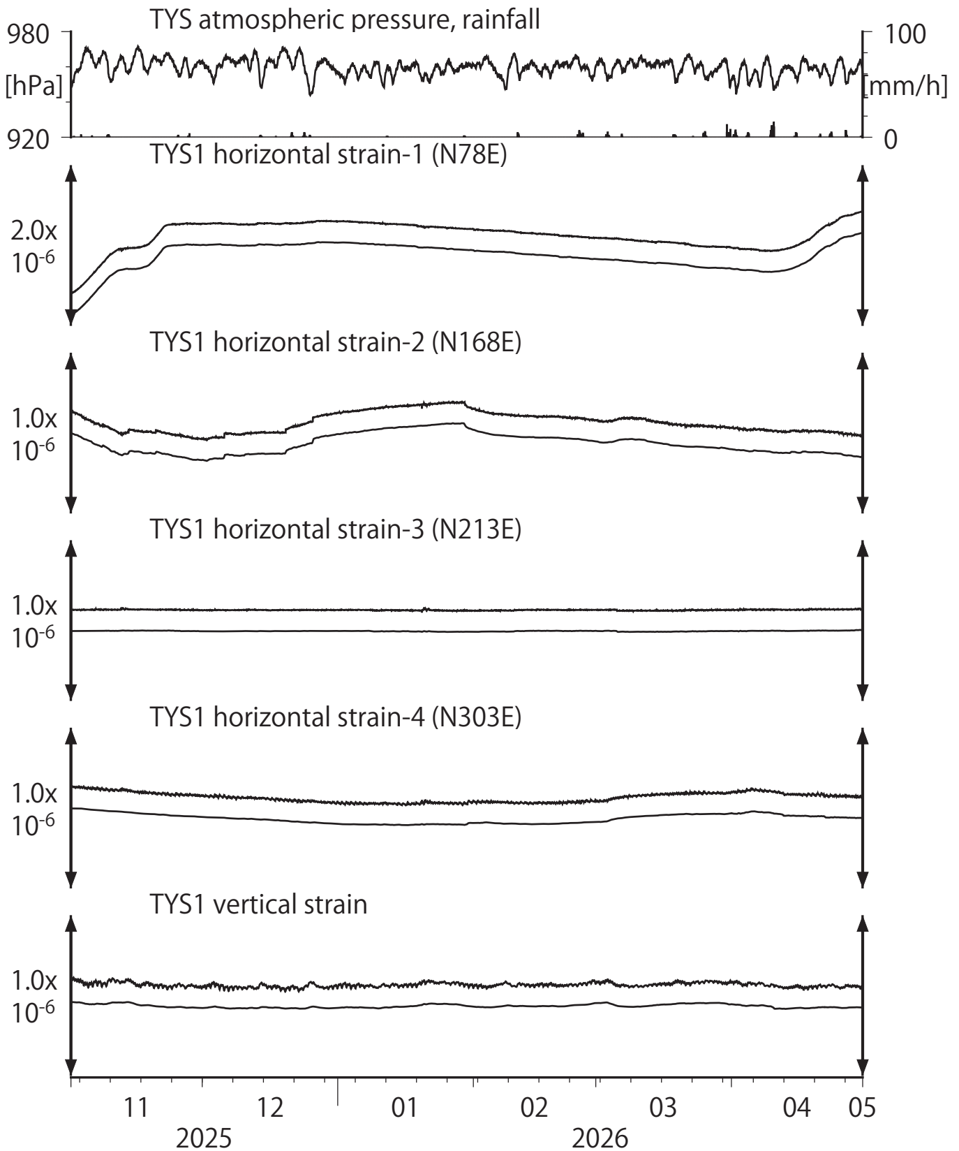
第2図 Crustal strains at TYS (時間値) (2025/11/01 00:00 - 2026/05/01 00:00 (JST))
