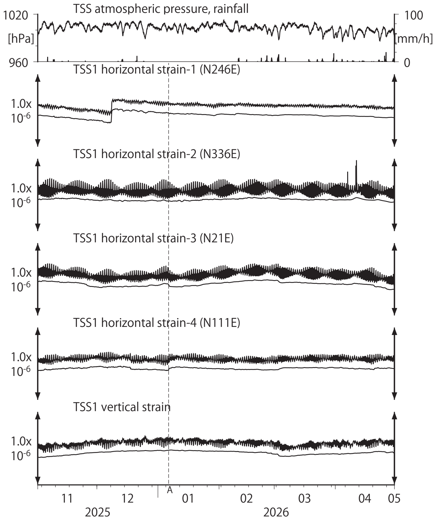
第31図 Crustal strains at TSS (時間値) (2025/11/01 00:00 - 2026/05/01 00:00 (JST))
