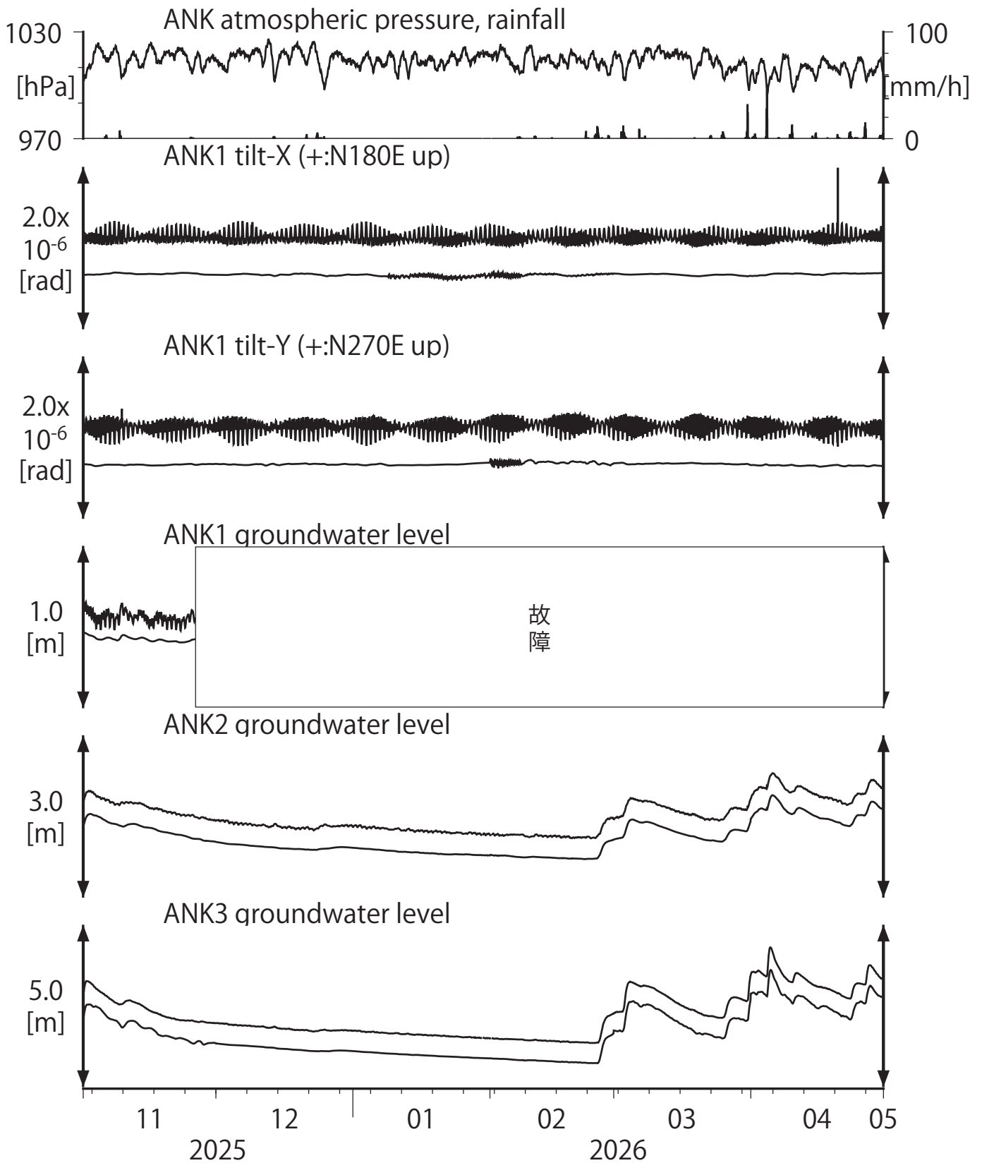
第22図 Tilt and groundwater level at ANK (時間値) (2025/11/01 00:00 - 2026/05/01 00:00 (JST))
