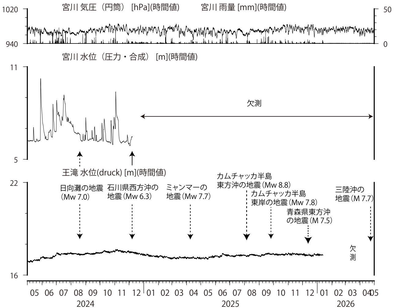
第3図 宮川と王滝における水位観測結果 (2年間) Fig.3 Results of groundwater levels at Miyagawa and Outaki (for 2 years).
