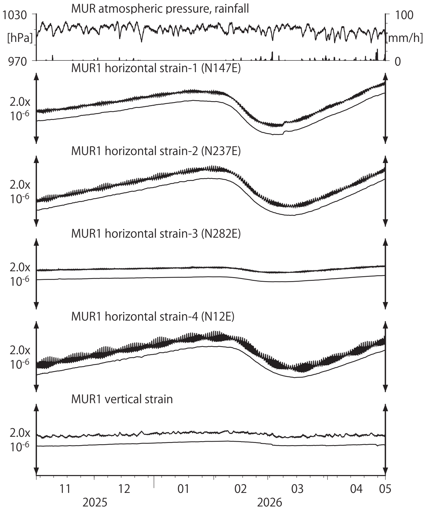
第26図 Crustal strains at MUR (時間値) (2025/11/01 00:00 - 2026/05/01 00:00 (JST))
