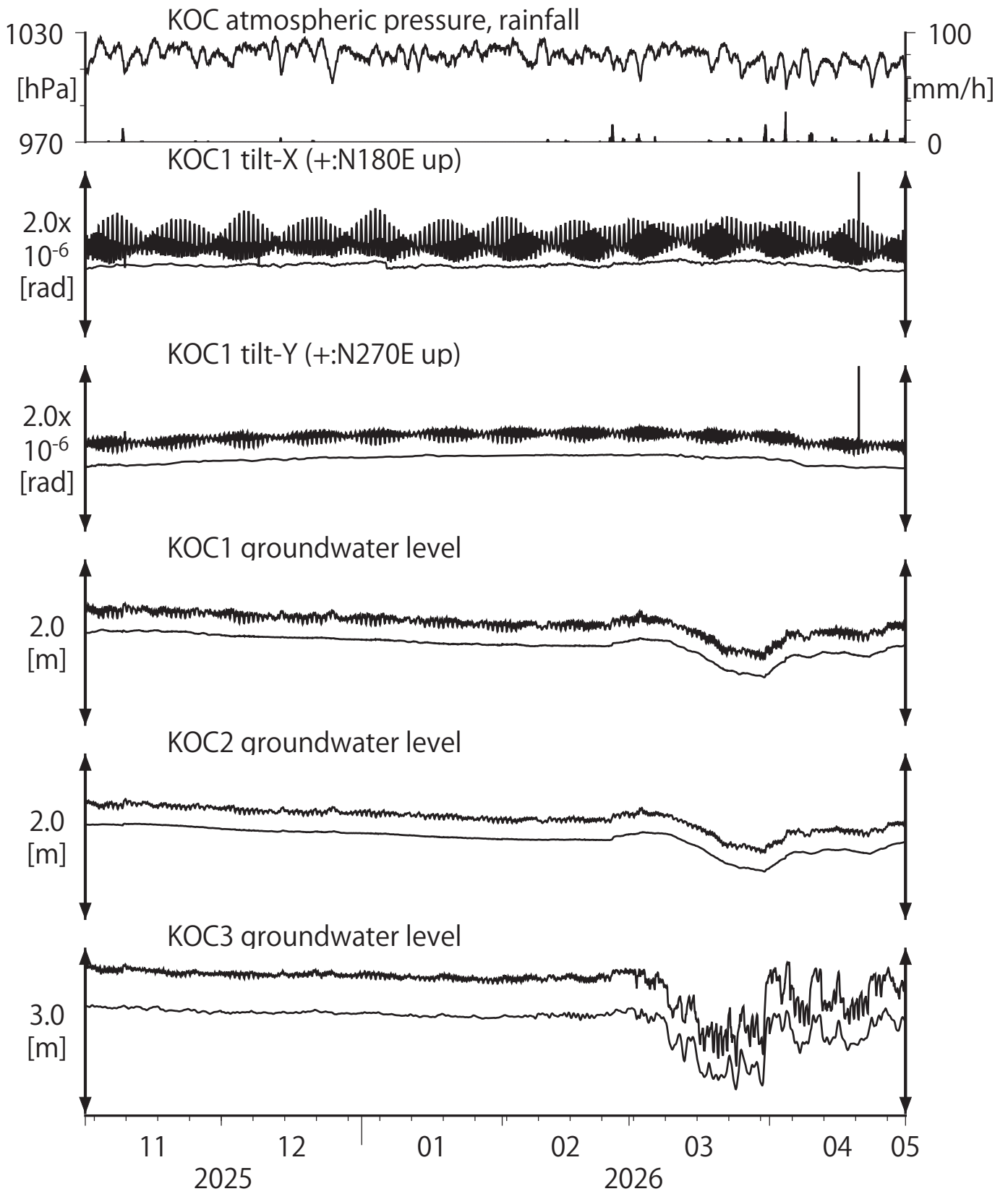
第28図 Tilt and groundwater level at KOC (時間値) (2025/11/01 00:00 - 2026/05/01 00:00 (JST))
