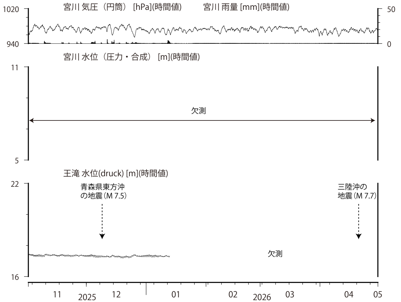
第2図 宮川と王滝における水位観測結果 (6ヶ月間) Fig.2 Results of groundwater levels at Miyagawa and Outaki (for 6 months).
