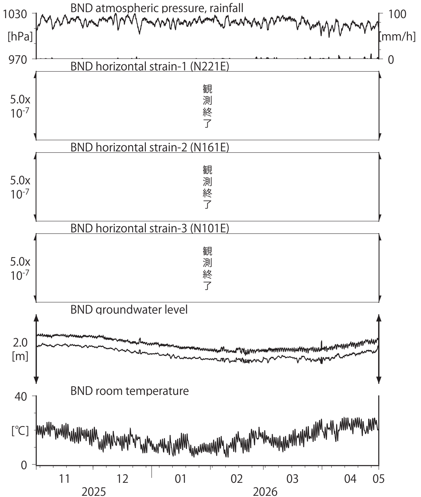
第21図 Crustal strains and groundwater level at BND (時間値) (2025/11/01 00:00 - 2026/05/01 00:00 (JST))
