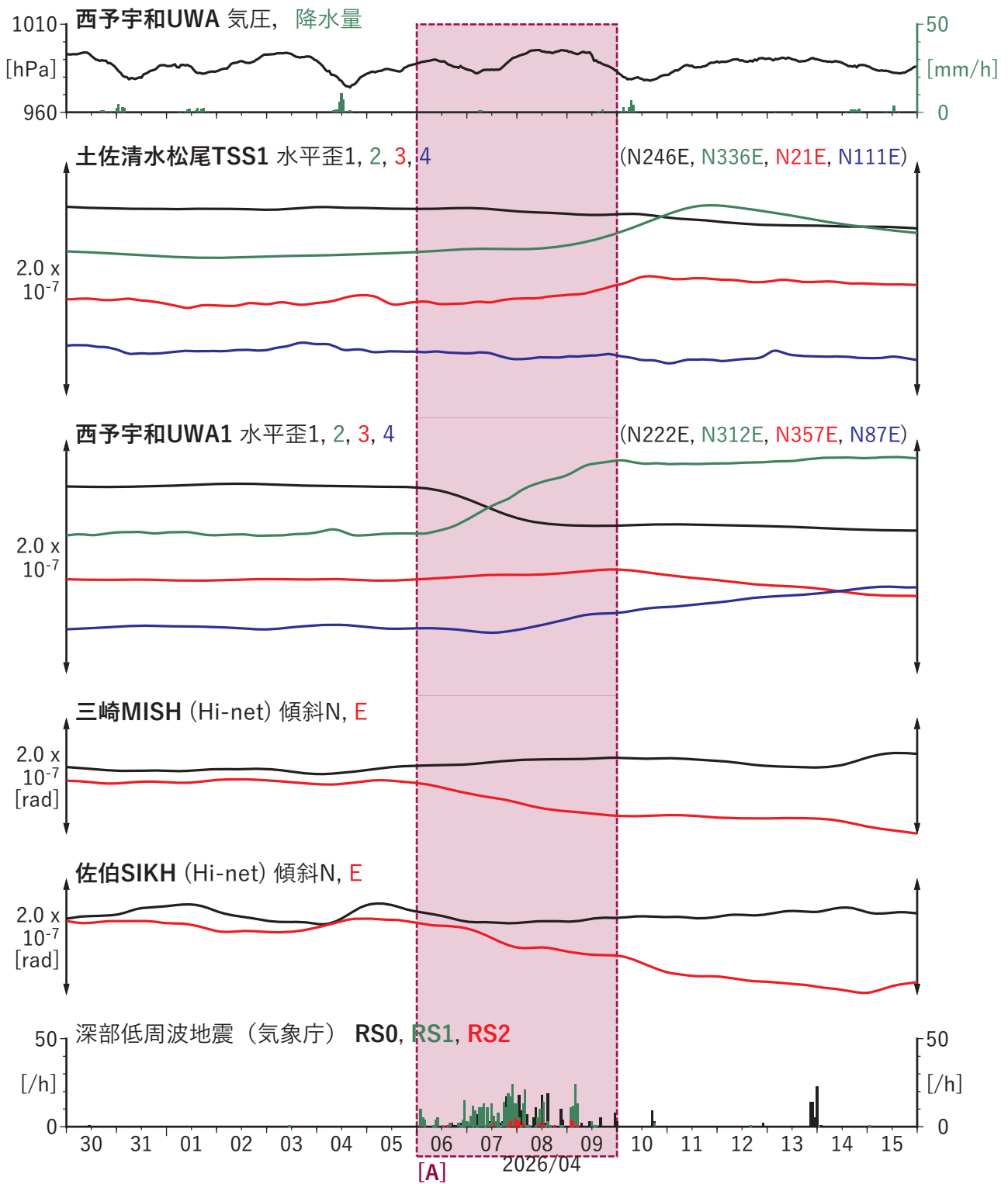
第49図 歪・傾斜の時間変化 (2026/03/30 00:00–2026/04/16 00:00 (JST))
