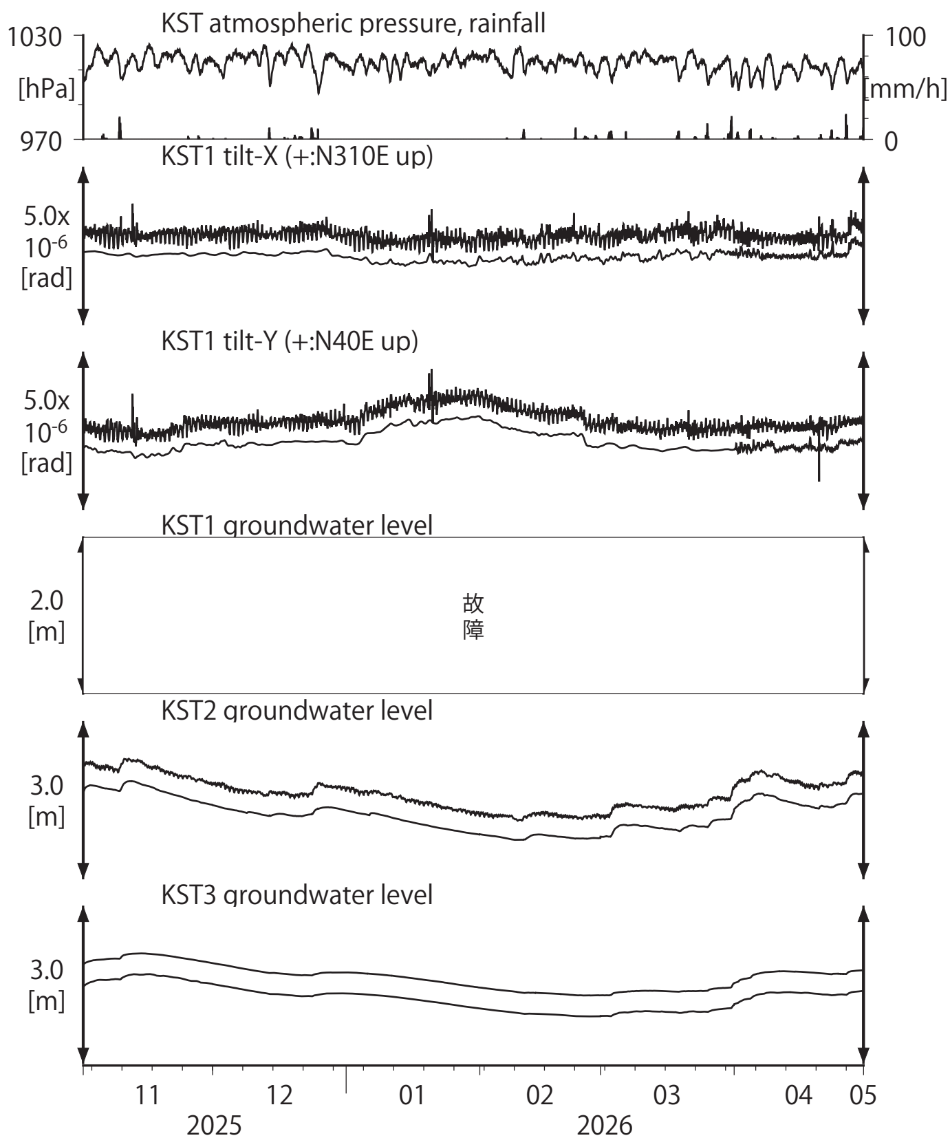
第18図 Tilt and groundwater level at KST (時間値) (2025/11/01 00:00 - 2026/05/01 00:00 (JST))
