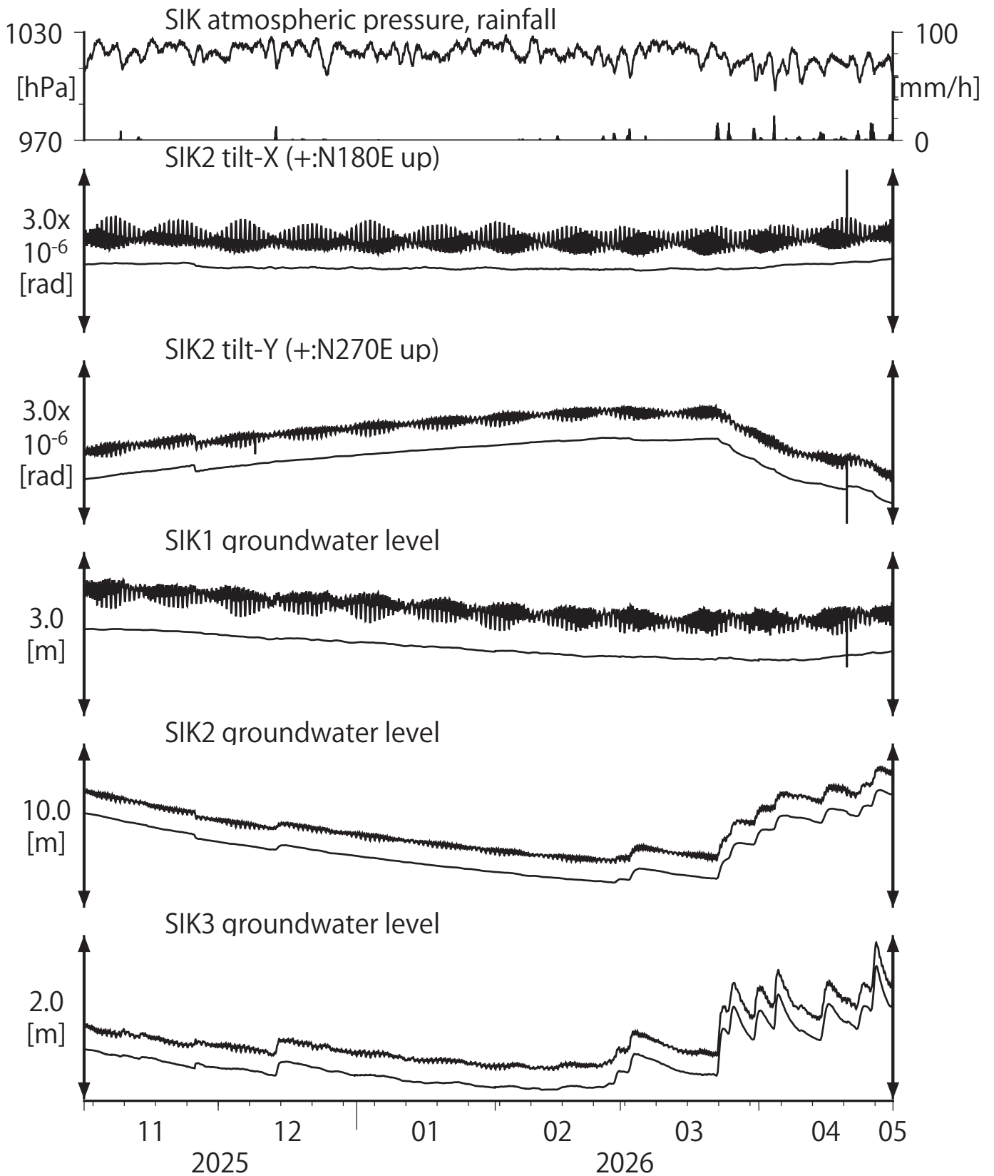
第39図 Tilt and groundwater level at SIK (時間値) (2025/11/01 00:00 - 2026/05/01 00:00 (JST))
