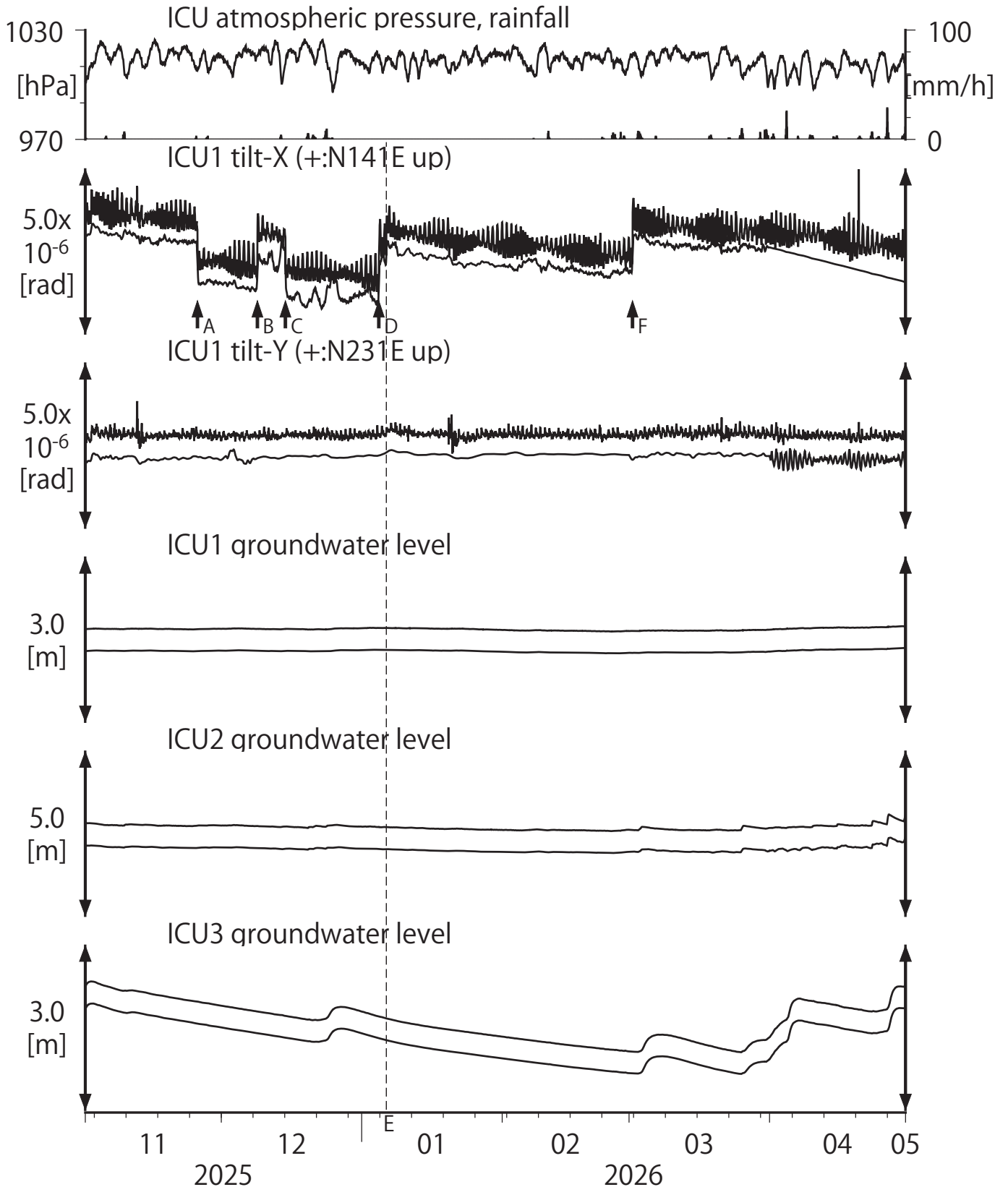
第14図 Tilt and groundwater level at ICU (時間値) (2025/11/01 00:00 - 2026/05/01 00:00 (JST))
