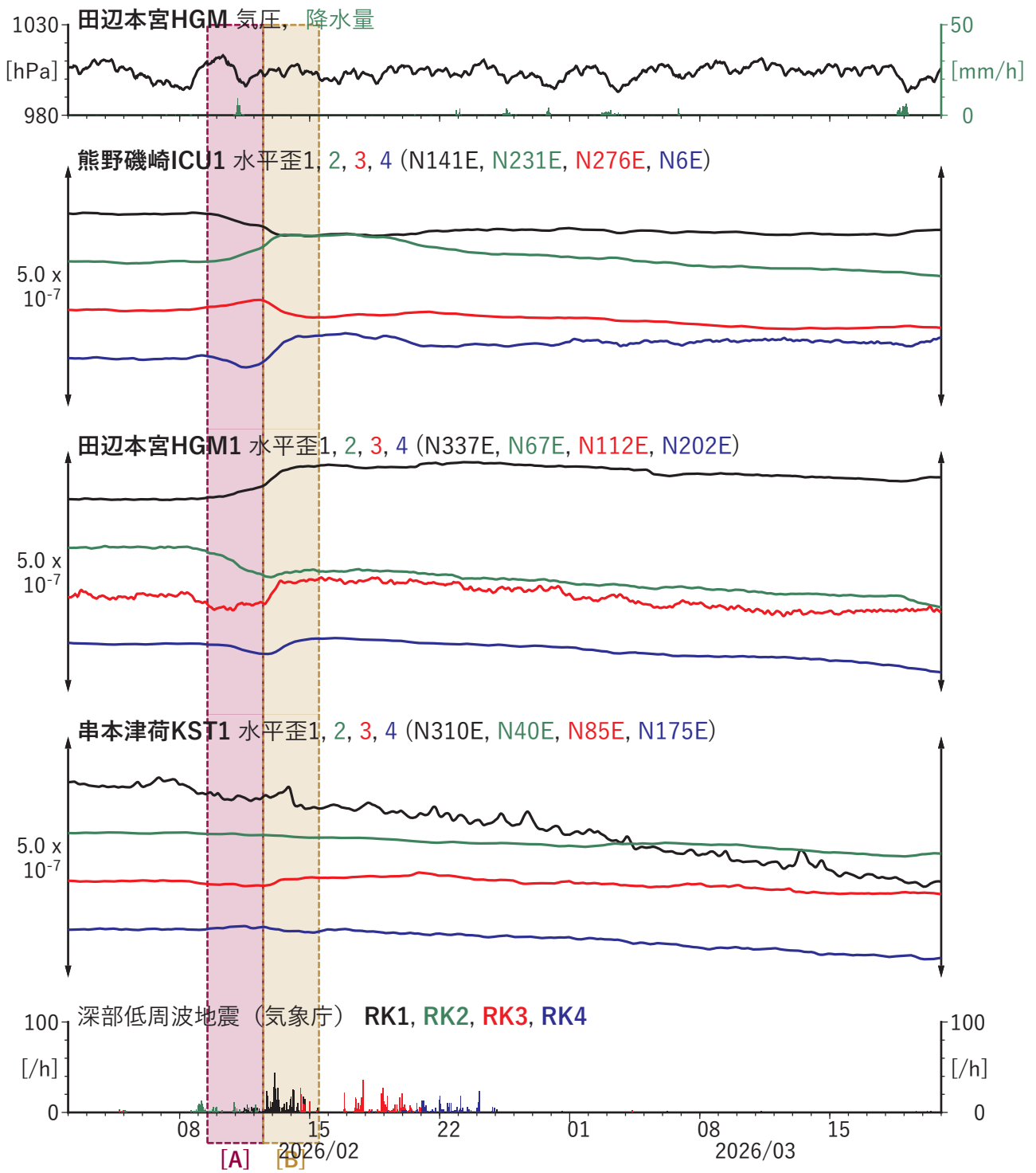
第41図 歪・傾斜の時間変化(1) (2026/02/02 00:00-2026/03/20 00:00 (JST))
