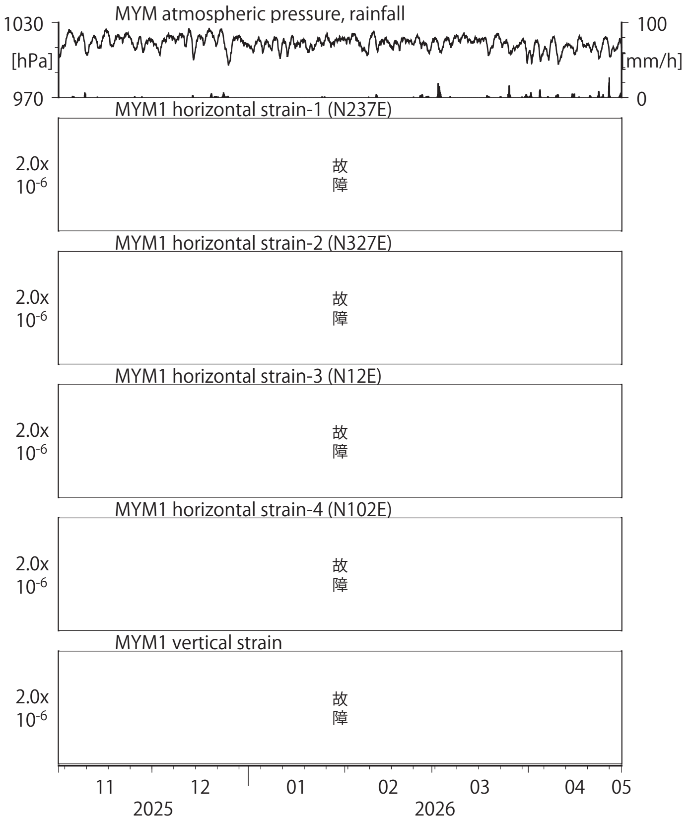
第11図 Crustal strains at MYM (時間値) (2025/11/01 00:00 - 2026/05/01 00:00 (JST))
