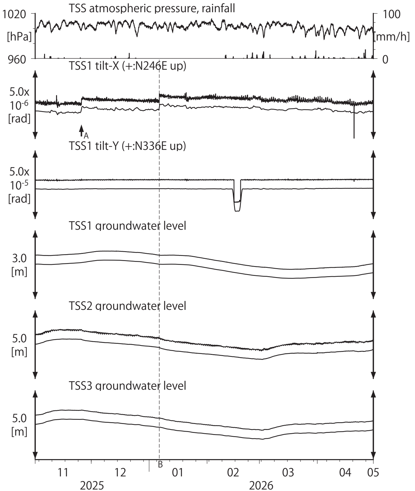
第32図 Tilt and groundwater level at TSS (時間値) (2025/11/01 00:00 - 2026/05/01 00:00 (JST))
