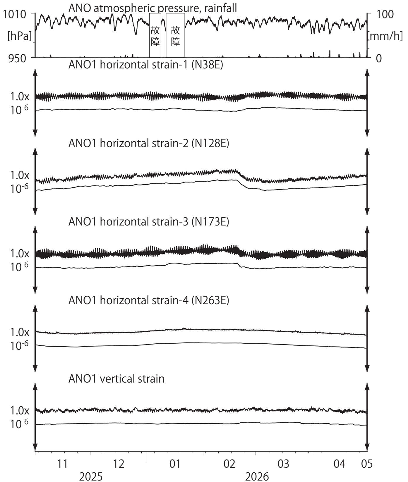
第8図 Crustal strains at ANO (時間値) (2025/11/01 00:00 - 2026/05/01 00:00 (JST))
