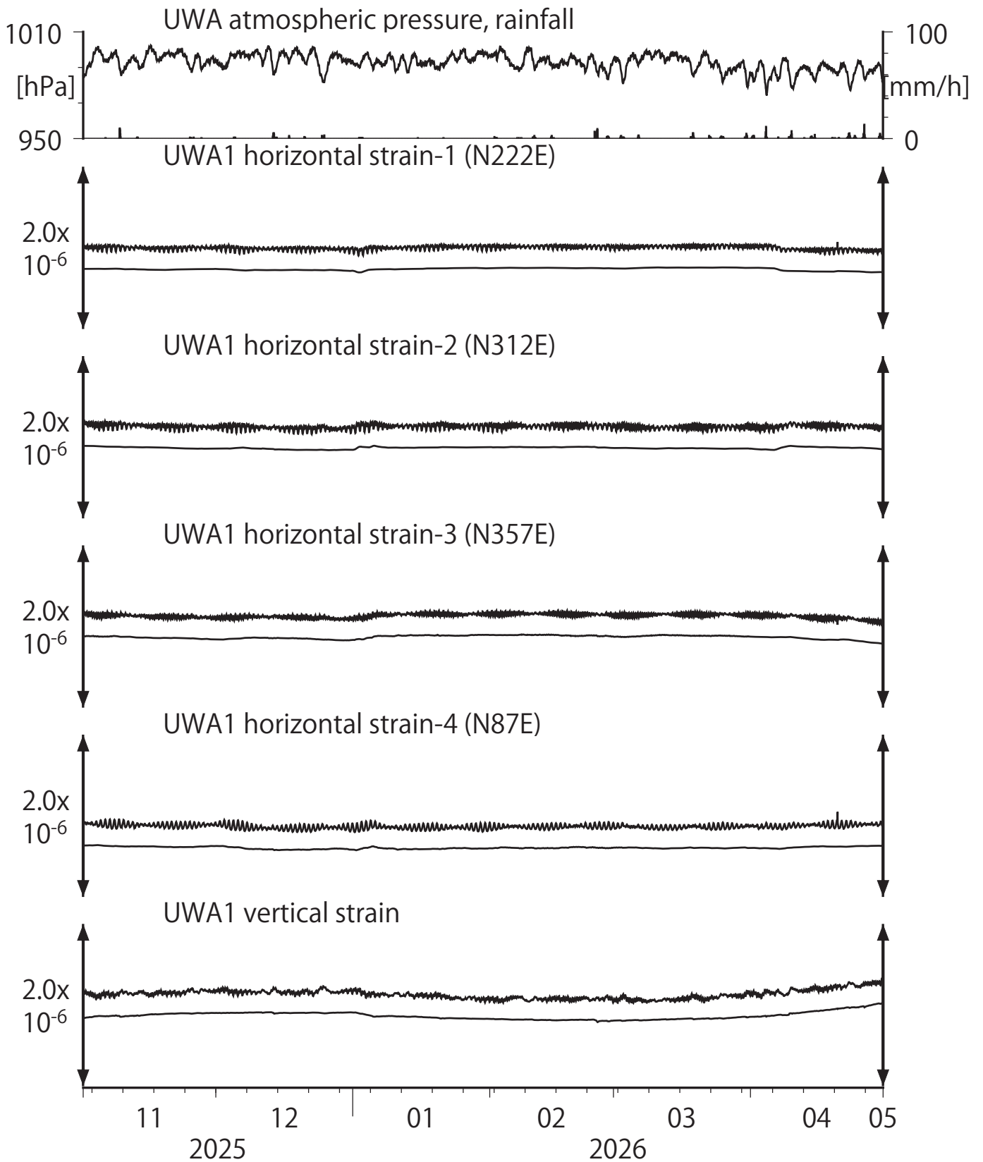
第33図 Crustal strains at UWA (時間値) (2025/11/01 00:00 - 2026/05/01 00:00 (JST))
