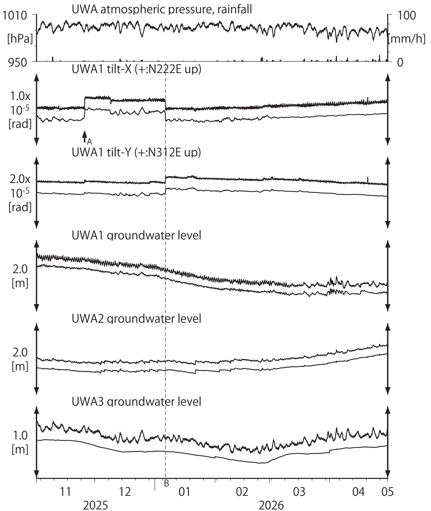
第34図 Tilt and groundwater level at UWA (時間値) (2025/11/01 00:00 - 2026/05/01 00:00 (JST))
