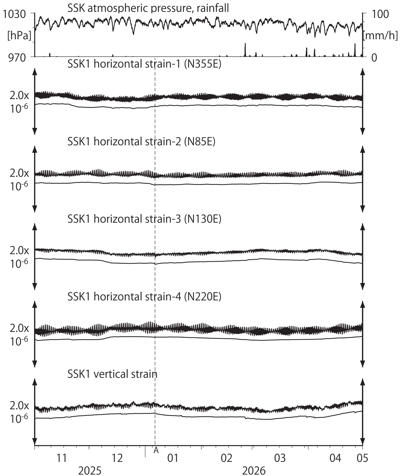
第29図 Crustal strains at SSK (時間値) (2025/11/01 00:00 - 2026/05/01 00:00 (JST))
