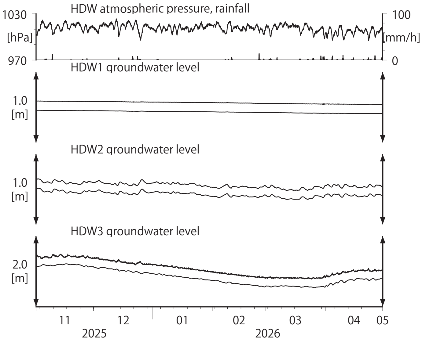
第20図 Groundwater level at HDW (時間値) (2025/11/01 00:00 - 2026/05/01 00:00 (JST))
