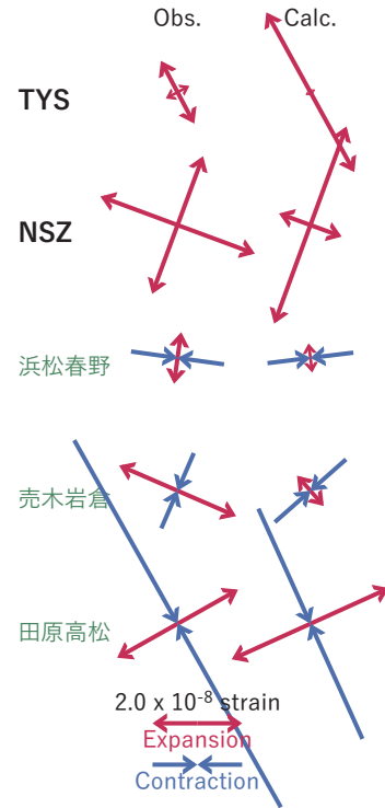
第46図 2026/03/02PM-07AMの歪・傾斜変化(第41図[E])を説明する断層モデル。
