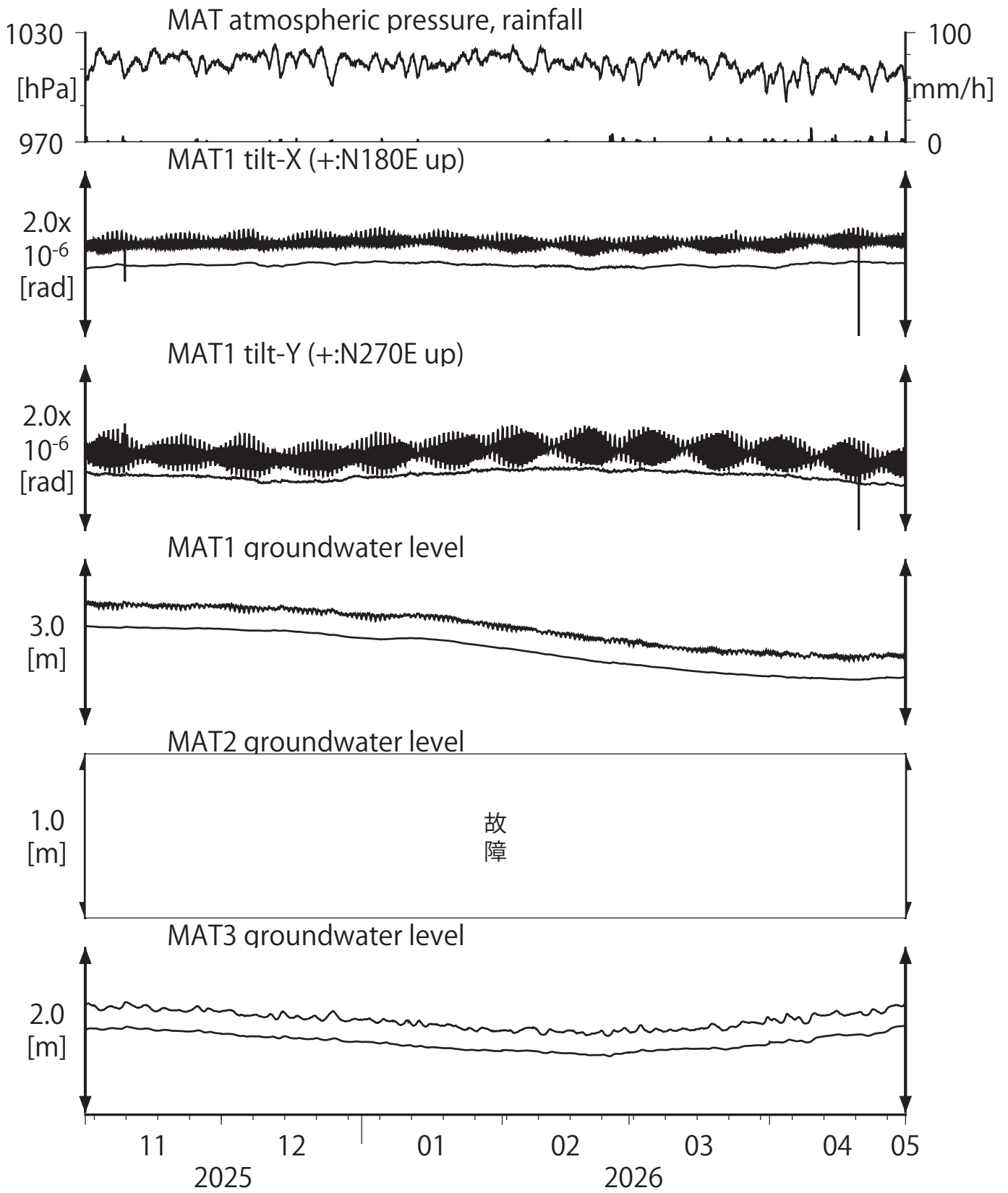
第35図 Tilt and groundwater level at MAT (時間値) (2025/11/01 00:00 - 2026/05/01 00:00 (JST))
