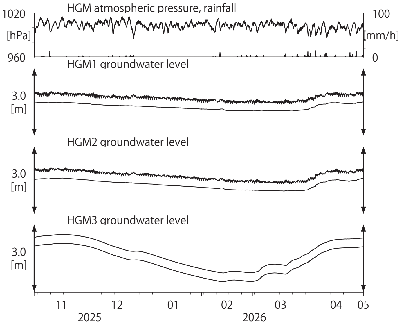
第16図 Tilt and groundwater level at HGM (時間値) (2025/11/01 00:00 - 2026/05/01 00:00 (JST))
