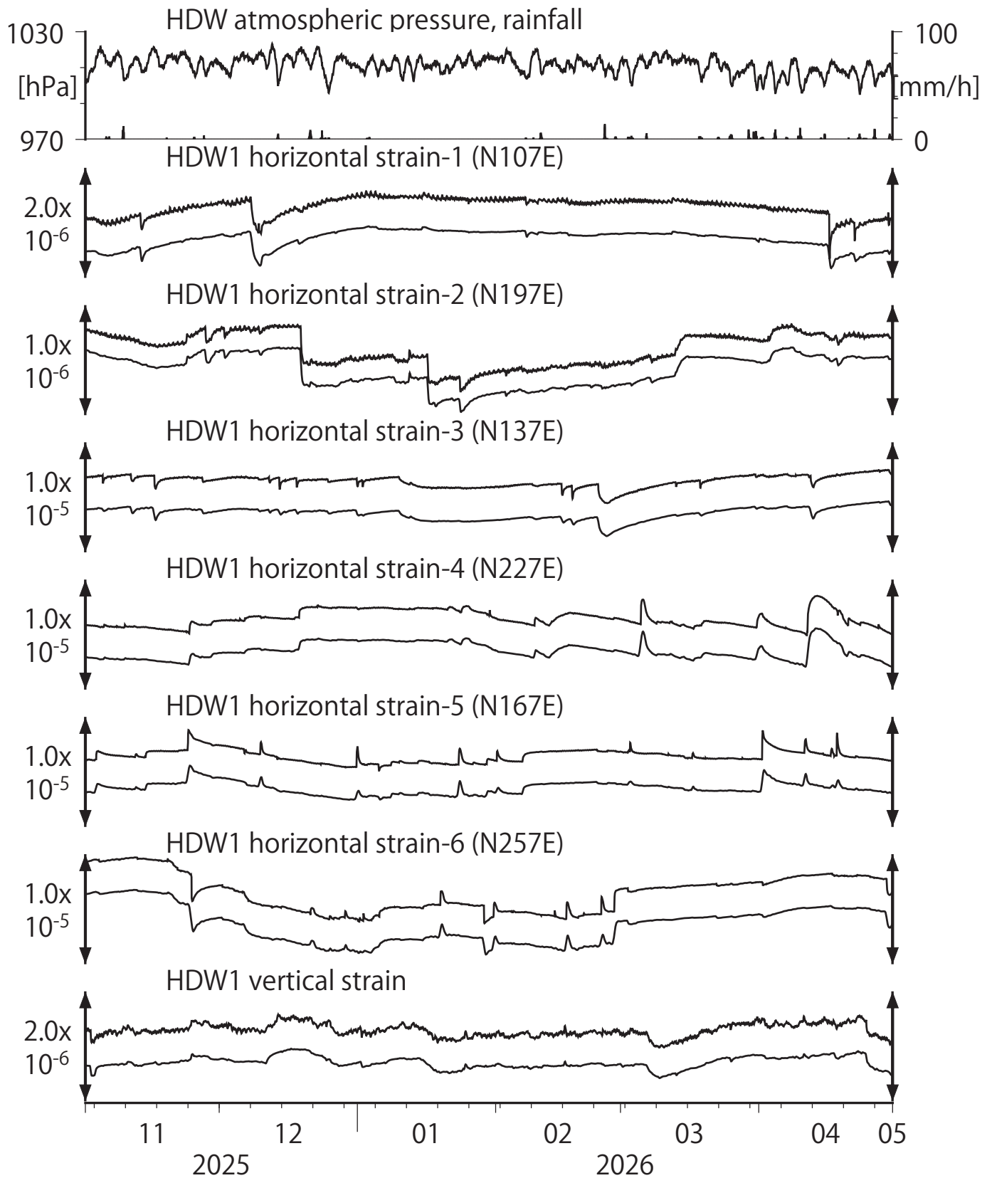
第19図 Crustal strains at HDW (時間値) (2025/11/01 00:00 - 2026/05/01 00:00 (JST))
