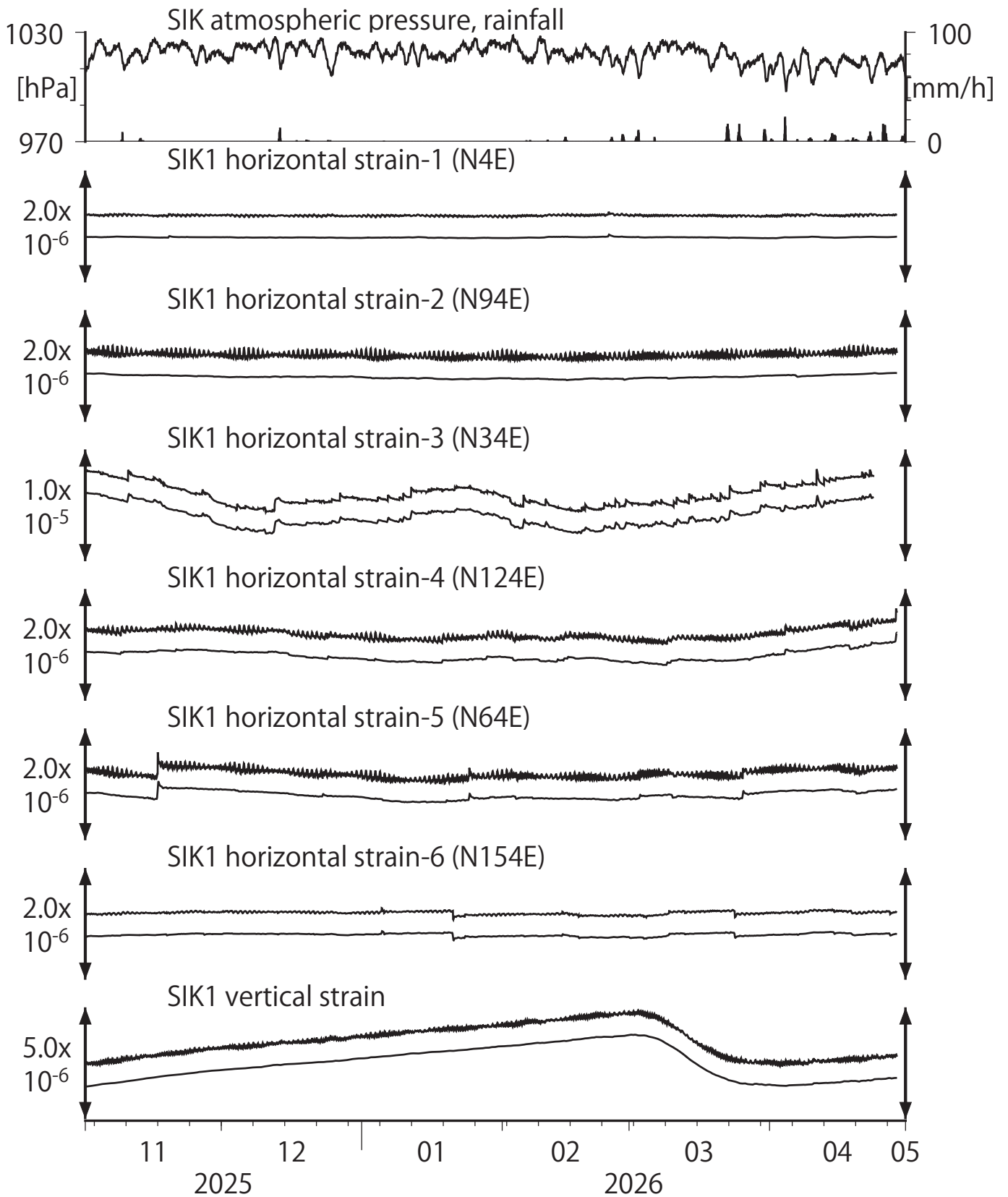
第38図 Crustal strains at SIK (時間値) (2025/11/01 00:00 - 2026/05/01 00:00 (JST))
