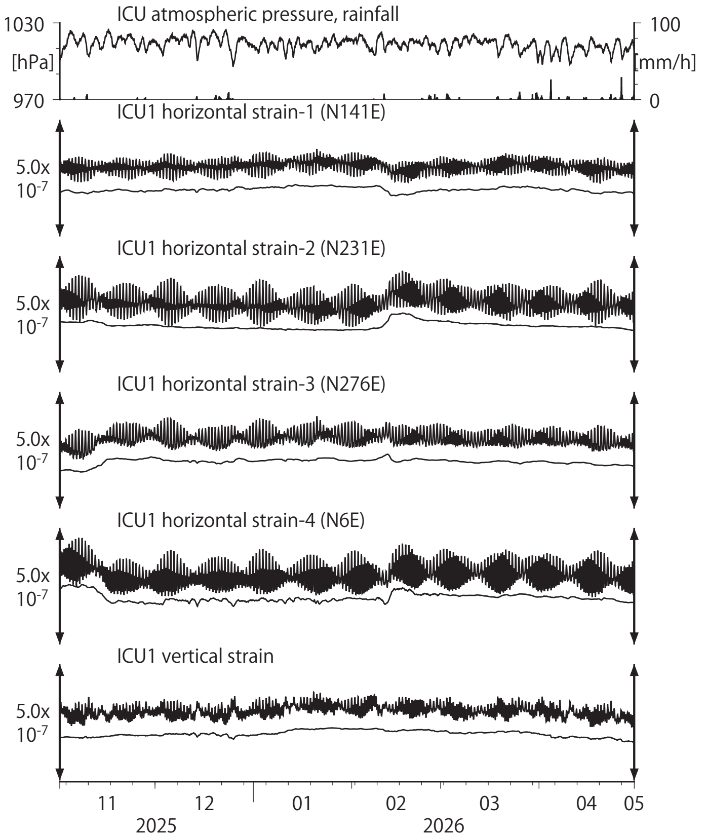
第13図 Crustal strains at ICU (時間値) (2025/11/01 00:00 - 2026/05/01 00:00 (JST))
