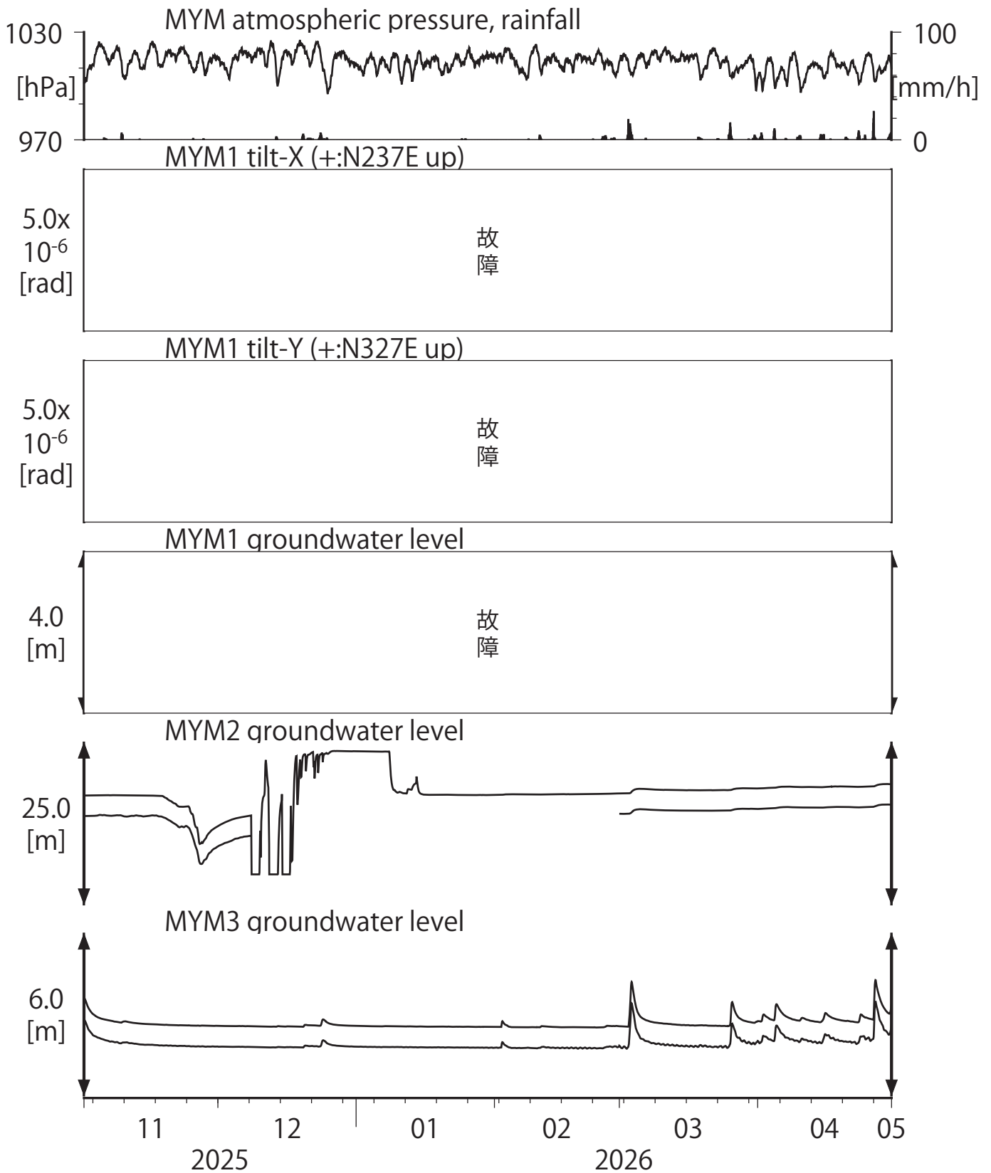
第12図 Tilt and groundwater level at MYM (時間値) (2025/11/01 00:00 - 2026/05/01 00:00 (JST))
