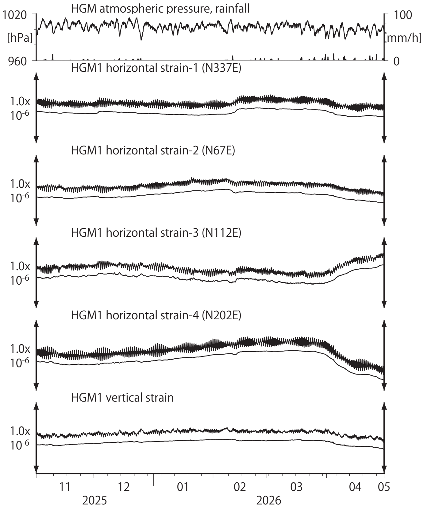
第15図 Crustal strains at HGM (時間値) (2025/11/01 00:00 - 2026/05/01 00:00 (JST))
