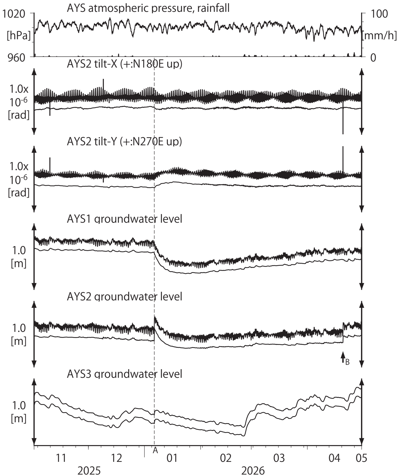
第24図 Tilt and groundwater level at AYS (時間値) (2025/11/01 00:00 - 2026/05/01 00:00 (JST))
