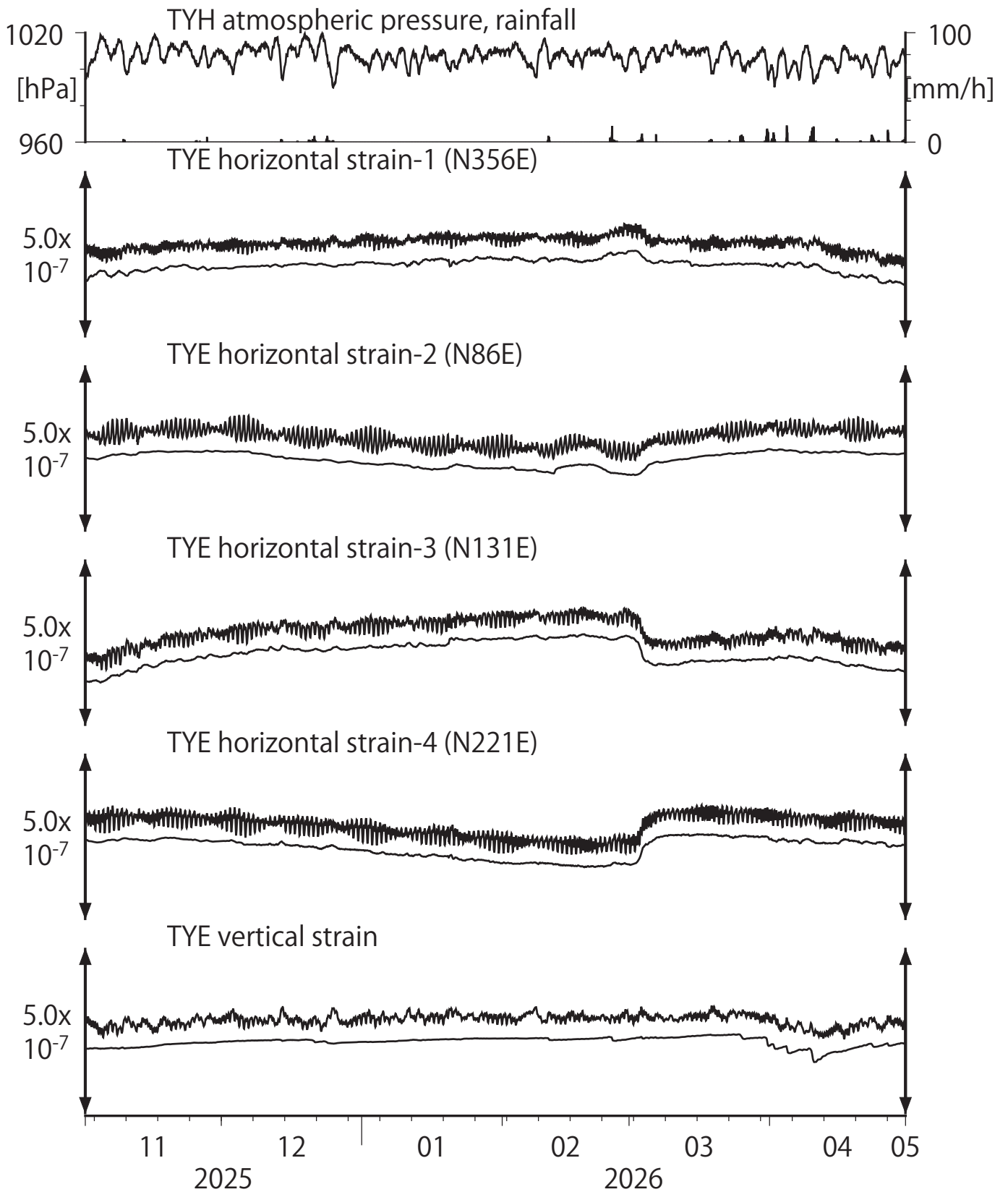
第6図 Crustal strain at TYE (時間値) (2025/11/01 00:00 - 2026/05/01 00:00 (JST))
