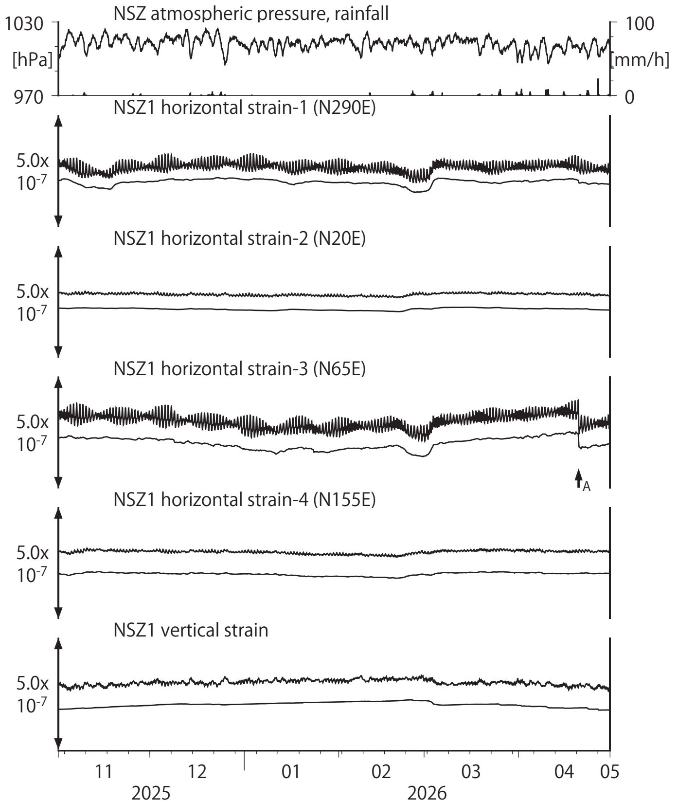
第4図 Crustal strains at NSZ (時間値) (2025/11/01 00:00 - 2026/05/01 00:00 (JST))
