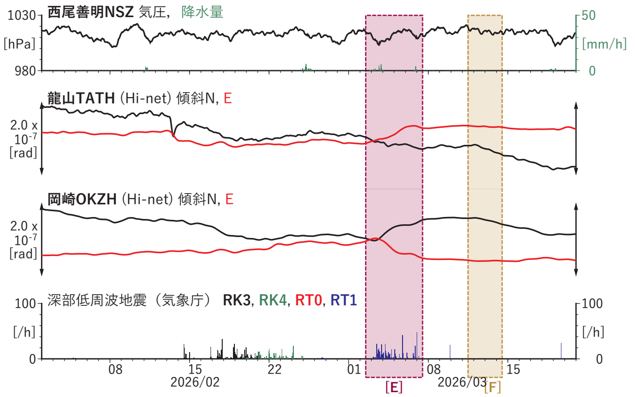
第41図 歪・傾斜の時間変化(4) (2026/02/02 00:00-2026/03/20 00:00 (JST))
