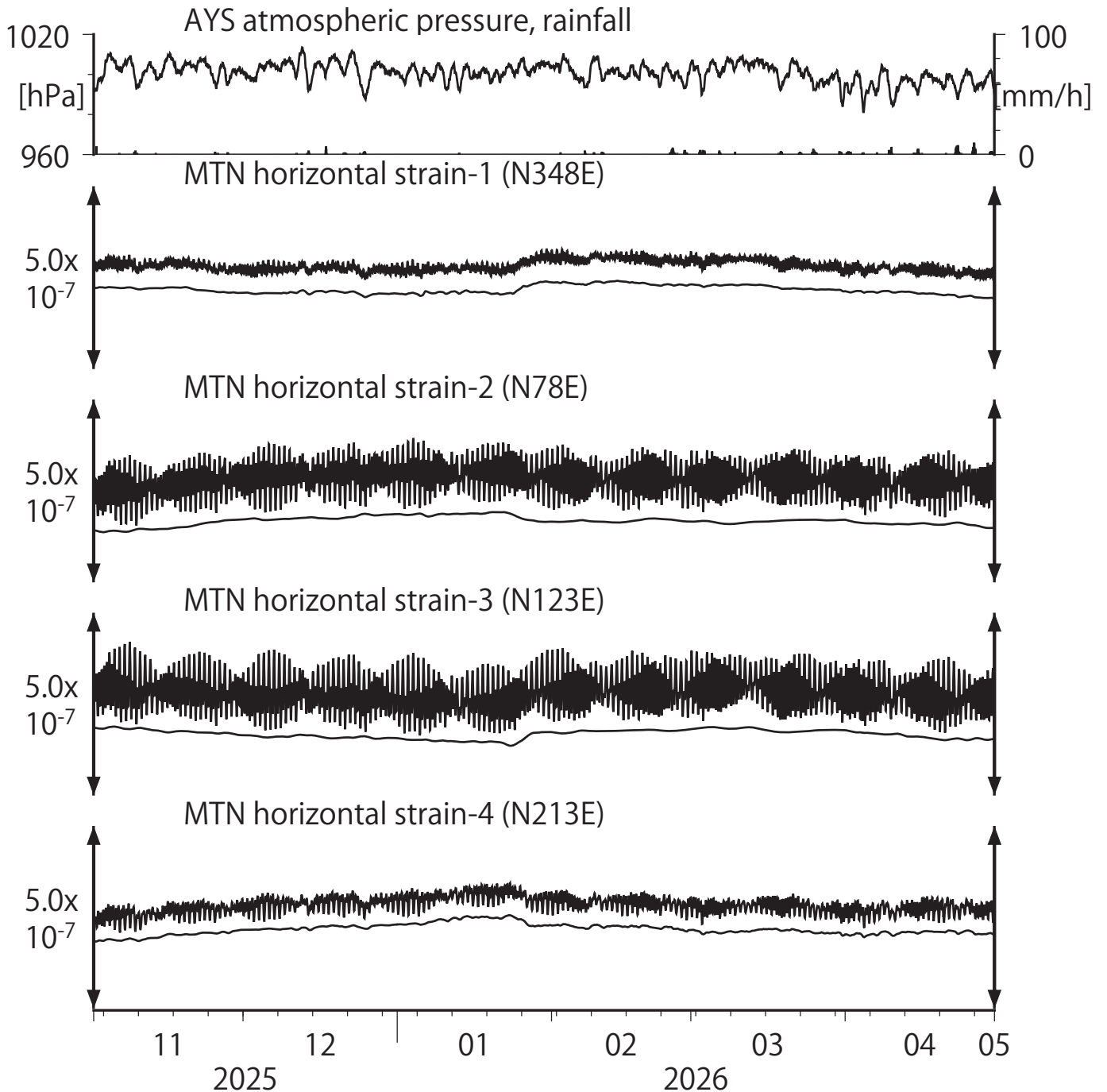
第25図 Crustal strains at MTN (時間値) (2025/11/01 00:00 - 2026/05/01 00:00 (JST))
