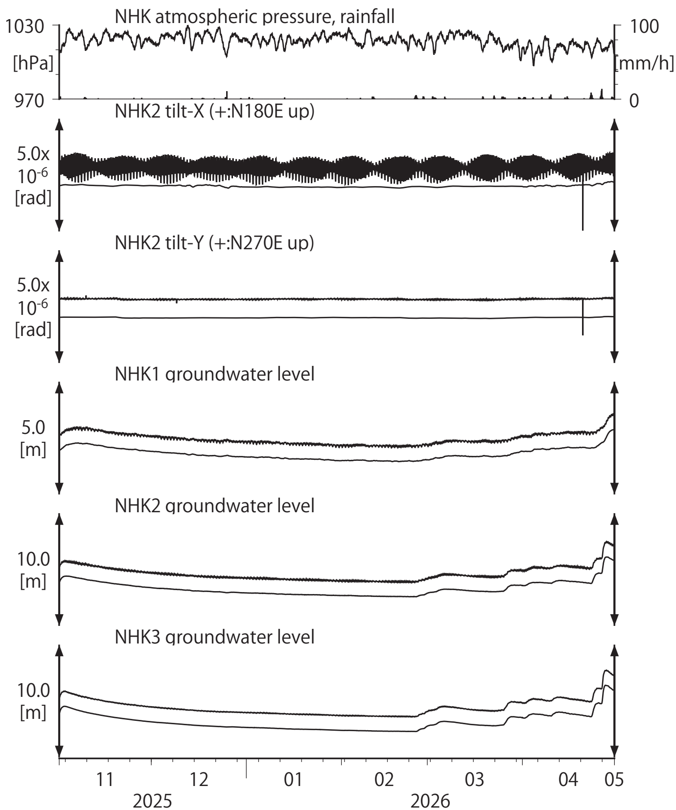
第37図 Tilt and groundwater level at NHK (時間値) (2025/11/01 00:00 - 2026/05/01 00:00 (JST))
