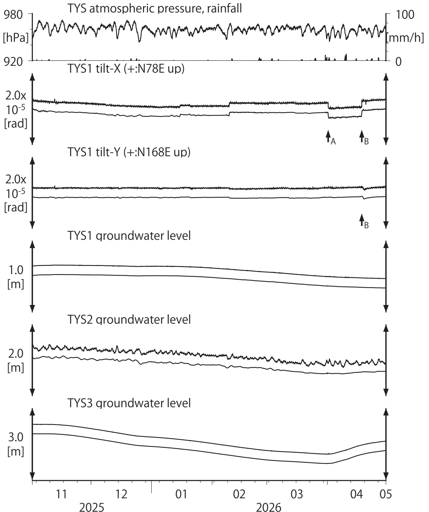
第3図 Tilt and groundwater level at TYS (時間値) (2025/11/01 00:00 - 2026/05/01 00:00 (JST))
