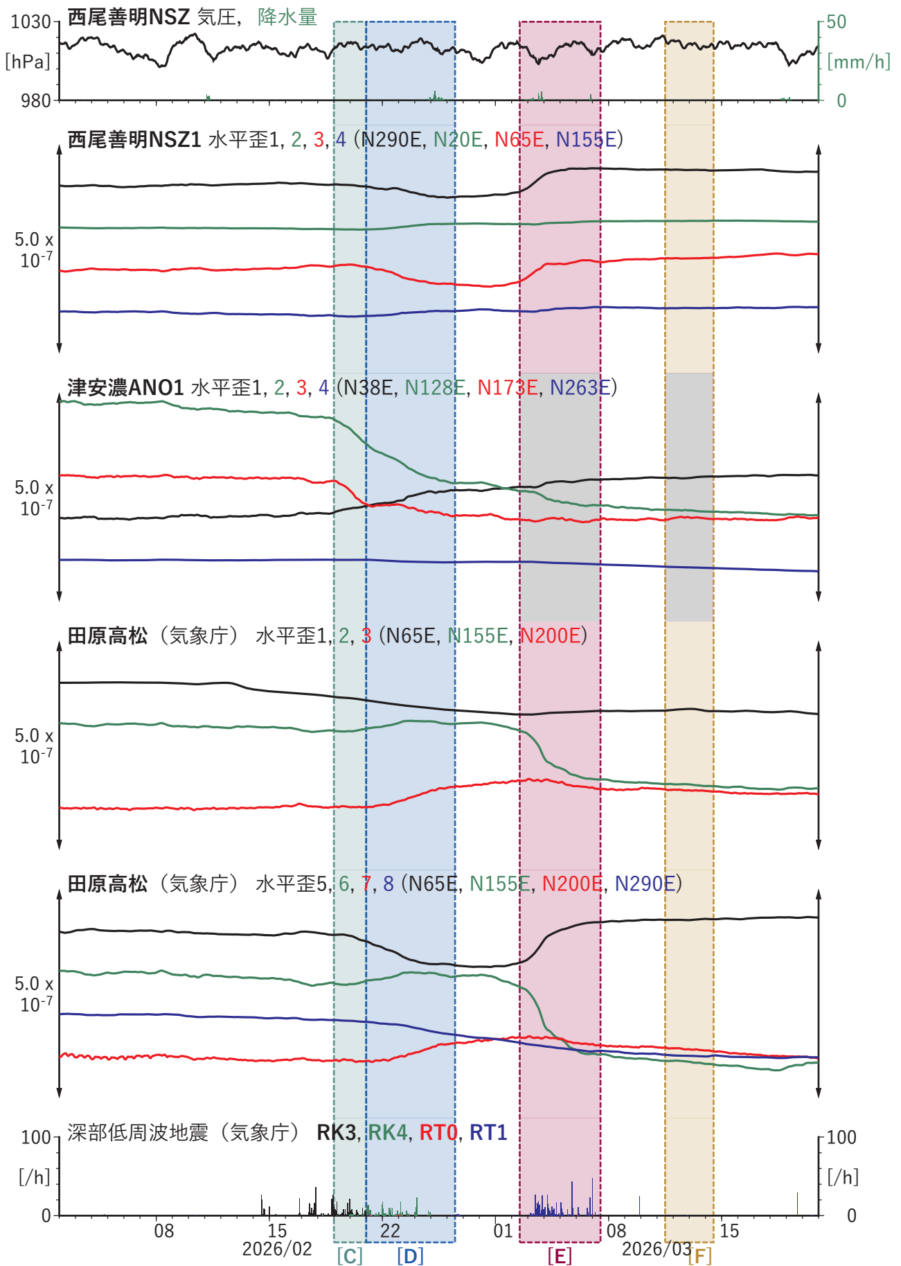
第41図 歪・傾斜の時間変化(2) (2026/02/02 00:00–2026/03/20 00:00 (JST))
