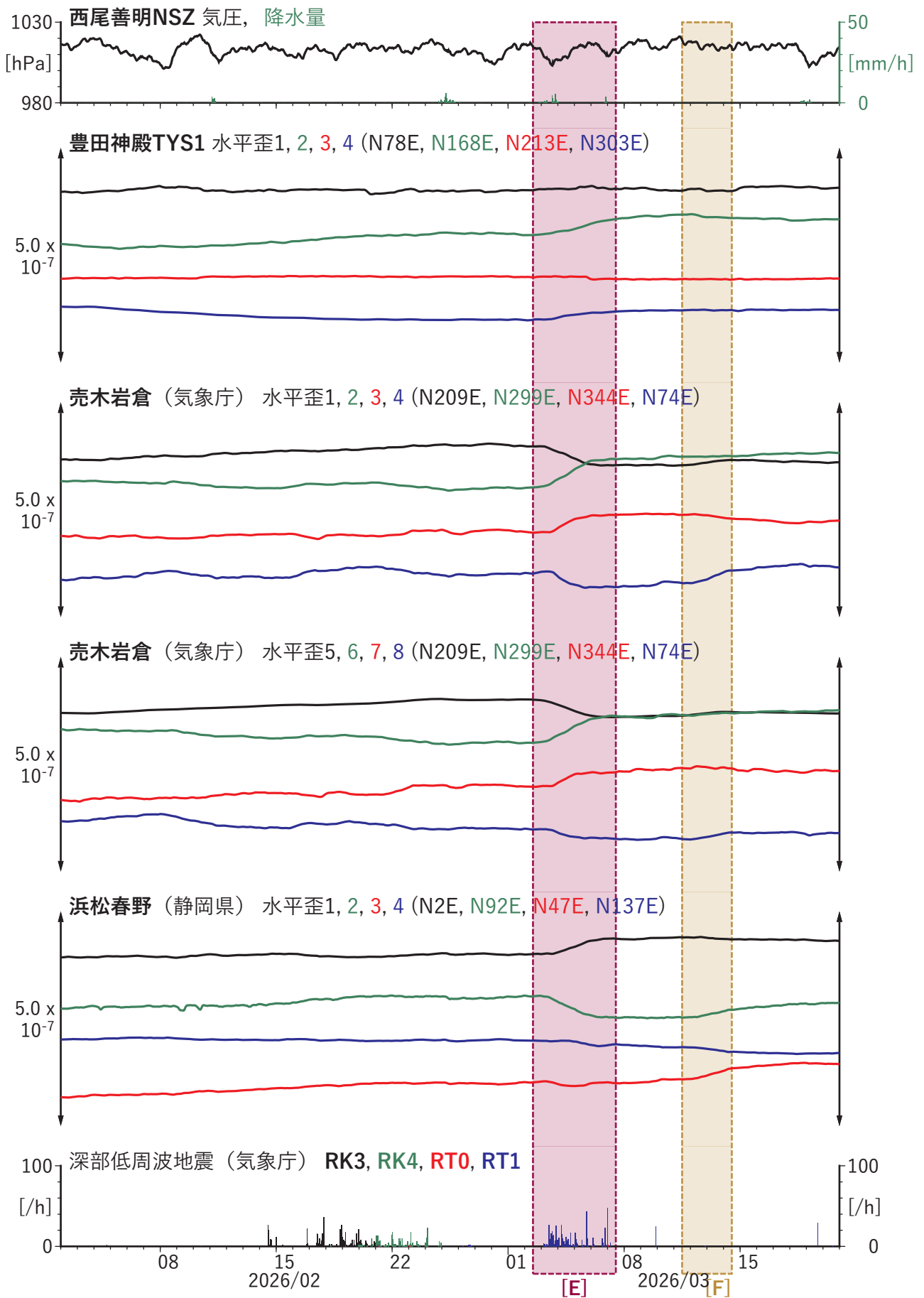
第41図 歪・傾斜の時間変化(3) (2026/02/02 00:00–2026/03/20 00:00 (JST))
