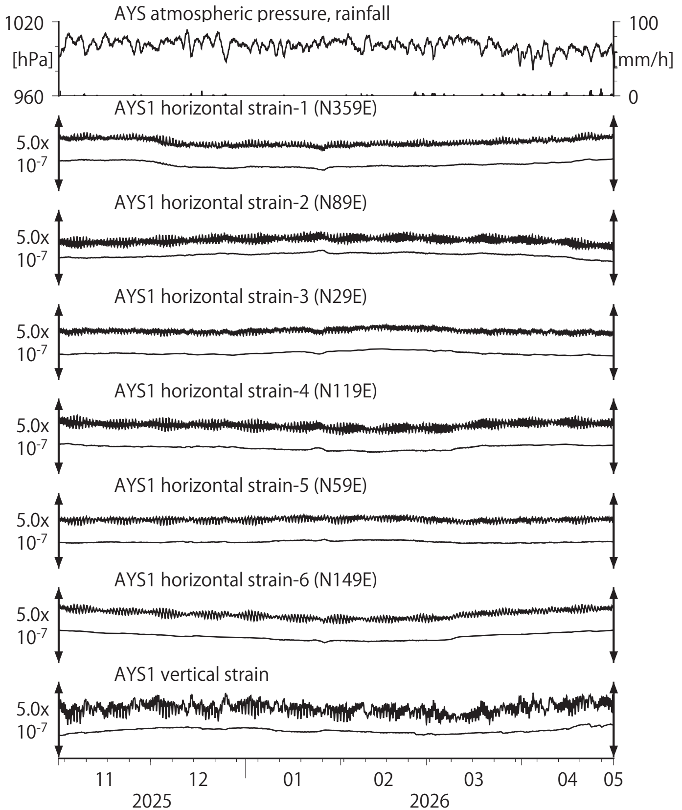
第23図 Crustal strains at AYS (時間値) (2025/11/01 00:00 - 2026/05/01 00:00 (JST))
