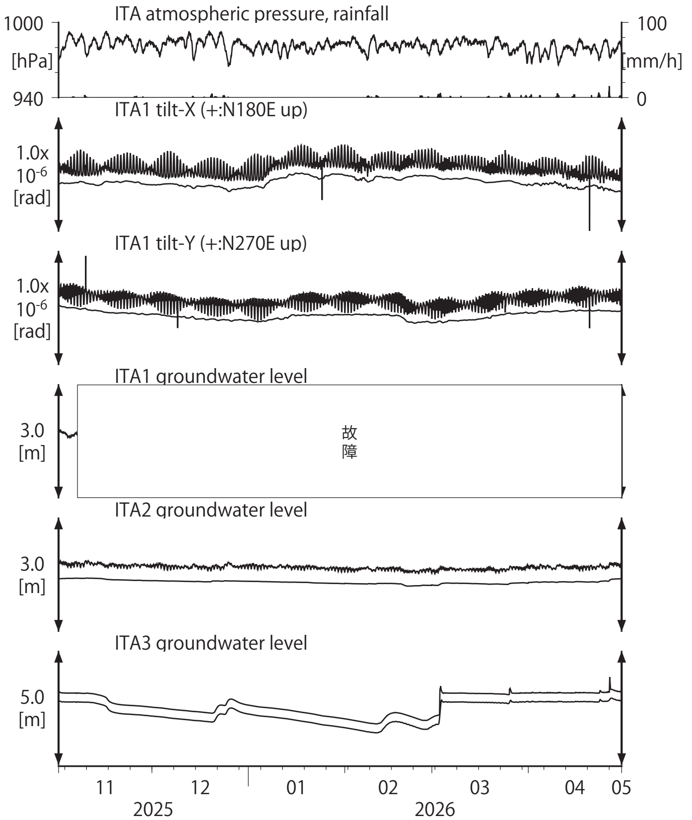
第10図 Tilt and groundwater level at ITA (時間値) (2025/11/01 00:00 - 2026/05/01 00:00 (JST))
