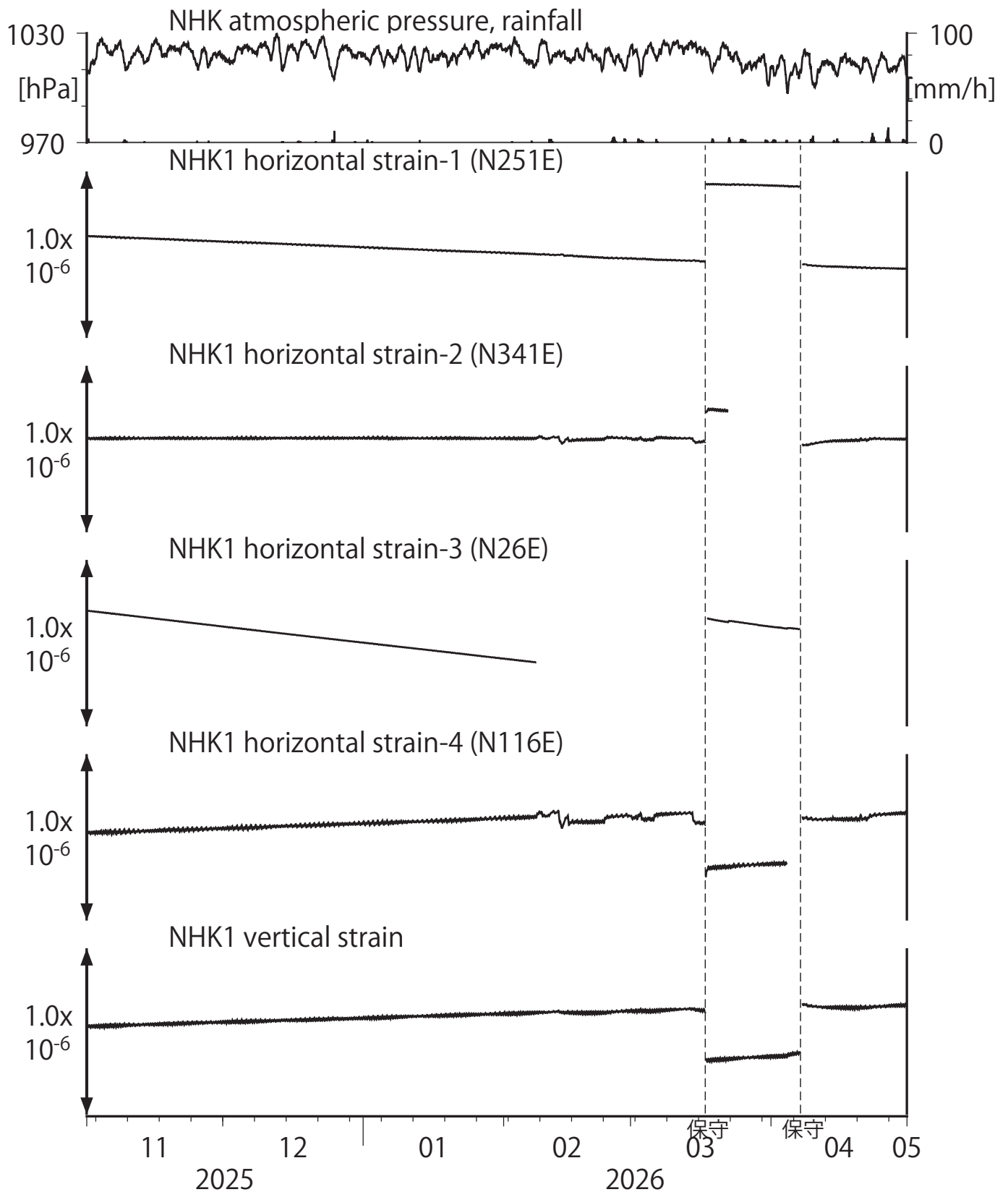
第36図 Crustal strains at NHK (時間値) (2025/11/01 00:00 - 2026/05/01 00:00 (JST))
