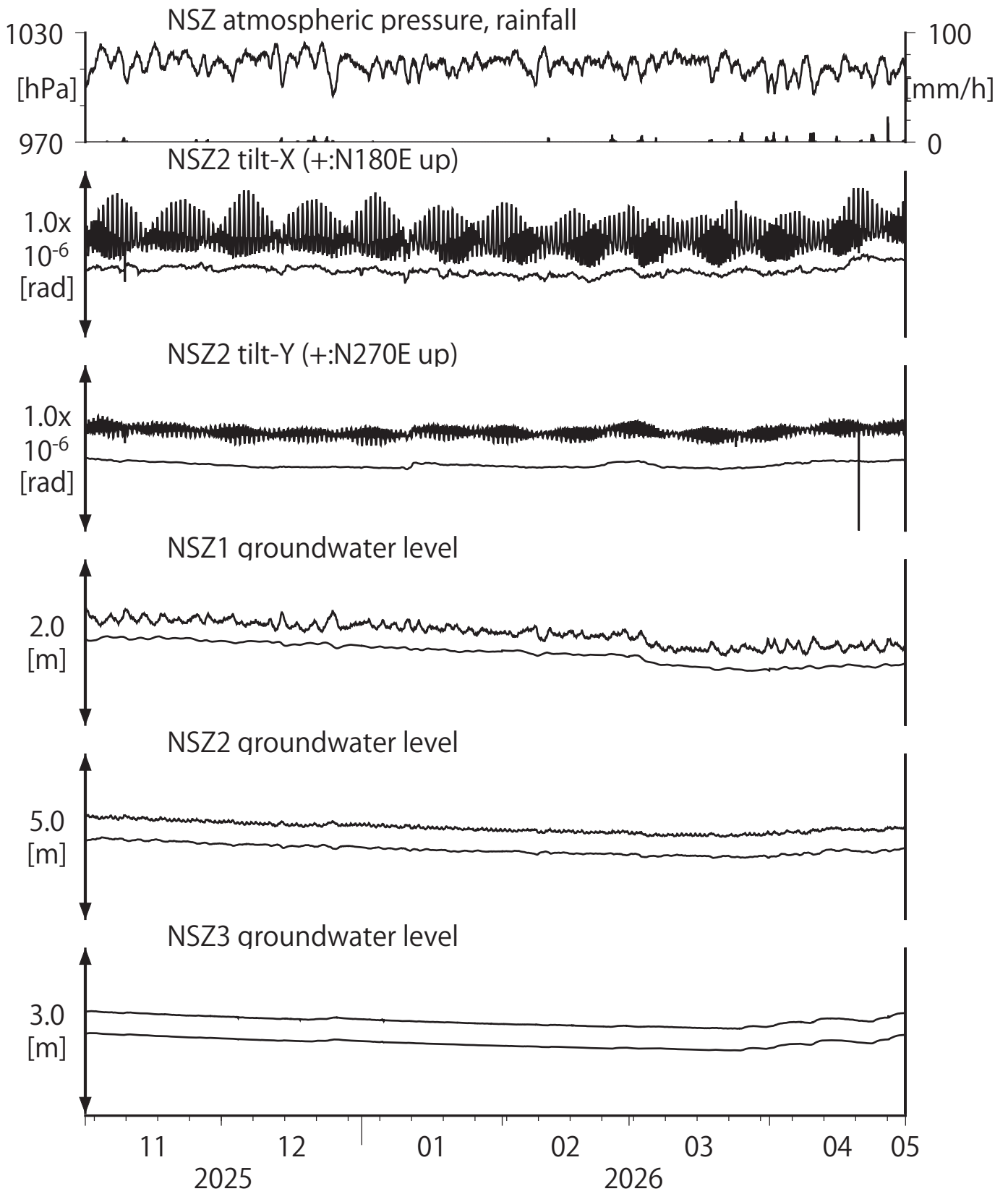
第5図 Tilt and groundwater level at NSZ (時間値) (2025/11/01 00:00 - 2026/05/01 00:00 (JST))
