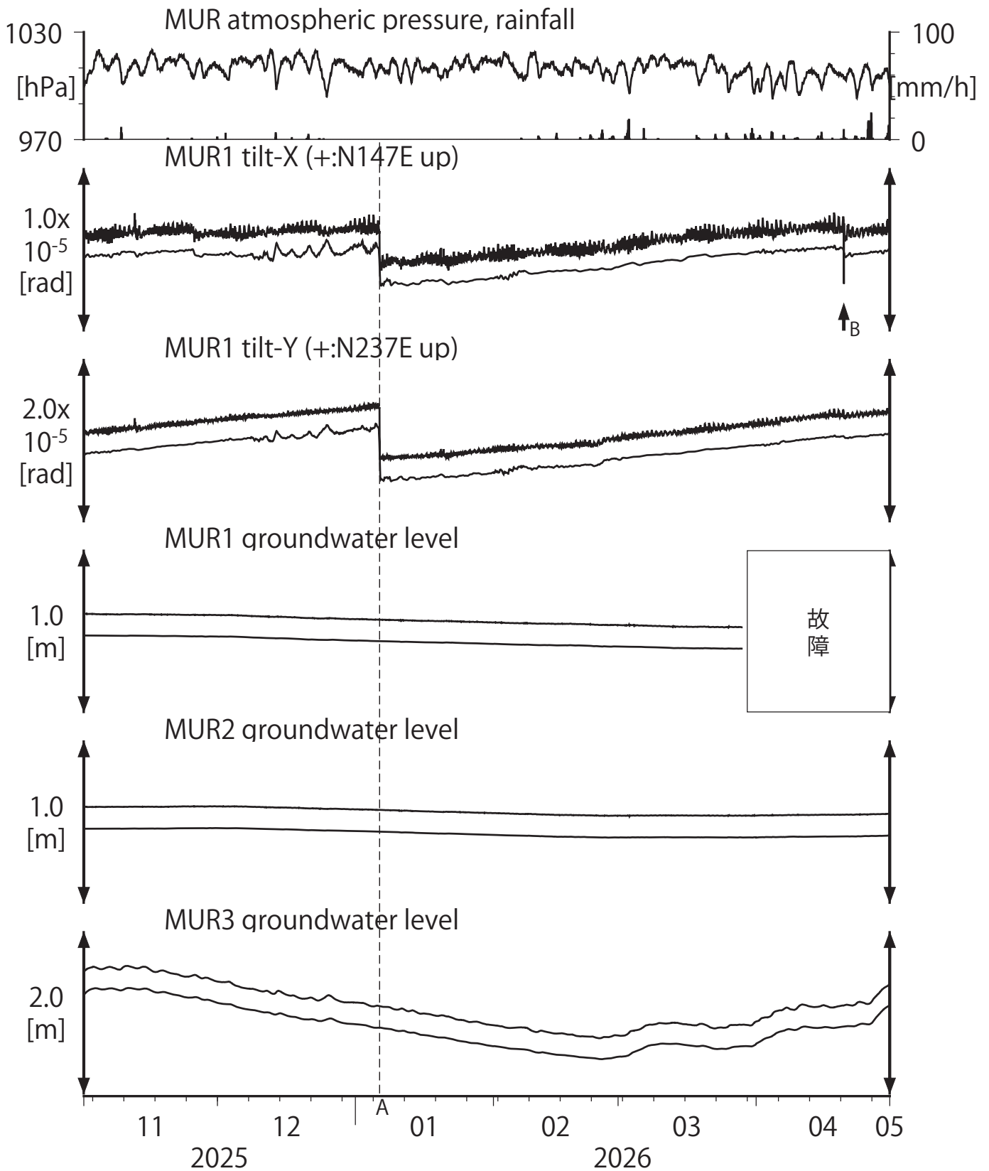
第27図 Tilt and groundwater level at MUR (時間値) (2025/11/01 00:00 - 2026/05/01 00:00 (JST))
