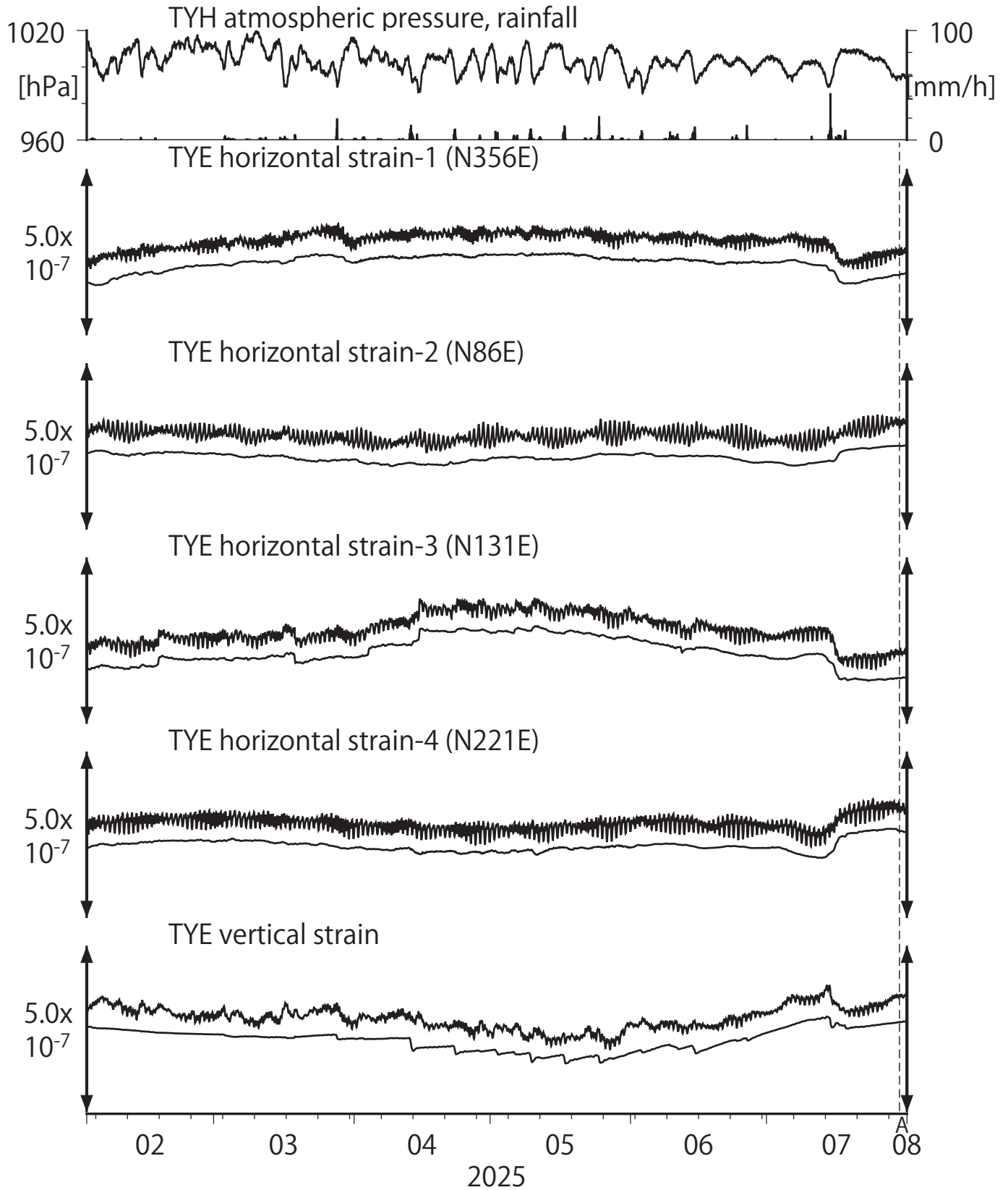
第6図 Crustal strain at TYE (時間値) (2025/02/01 00:00 - 2025/08/01 00:00 (JST))
