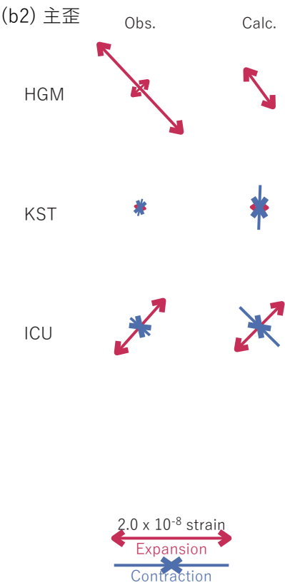
第37図 2025/04/29-30AMの歪・傾斜変化（第34図[B]）を説明する断層モデル。
