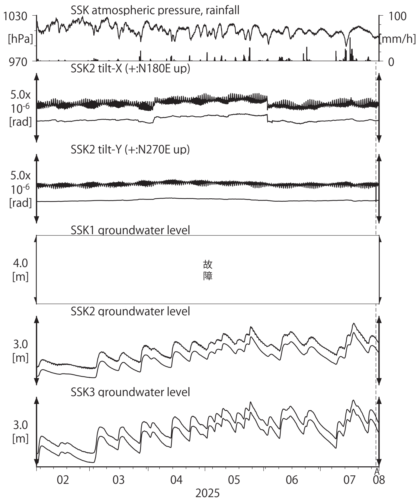
第25図 Tilt and groundwater level at SSK (時間値) (2025/02/01 00:00 - 2025/08/01 00:00 (JST))
