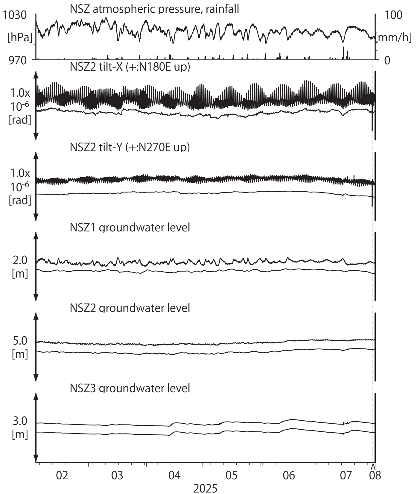
第5図 Tilt and groundwater level at NSZ (時間値) (2025/02/01 00:00 - 2025/08/01 00:00 (JST))
