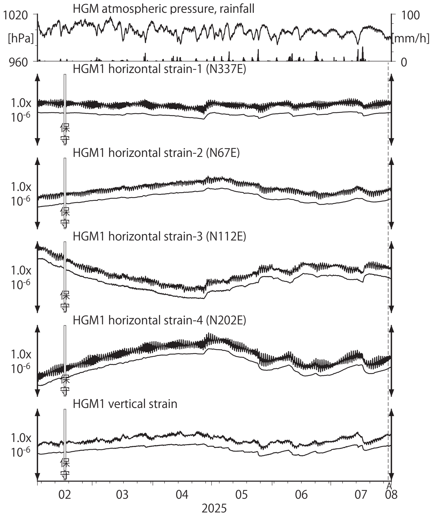
第15図 Crustal strains at HGM (時間値) (2025/02/01 00:00 - 2025/08/01 00:00 (JST))
