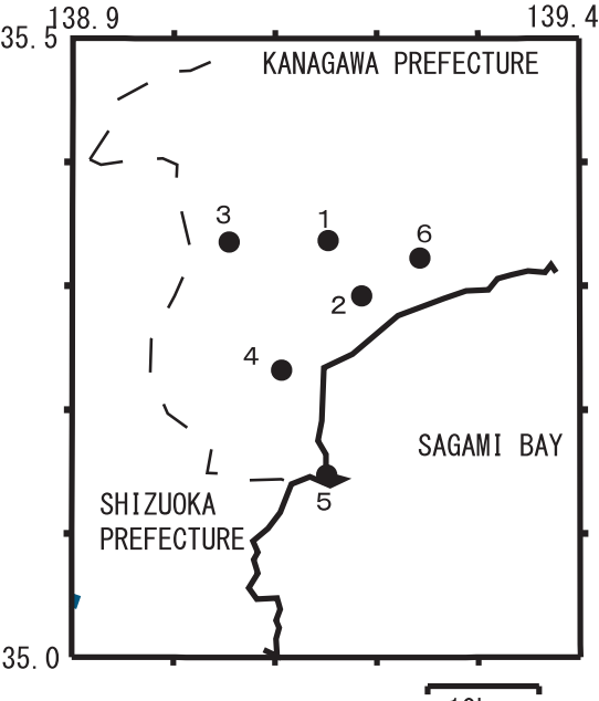
第1図 地下水位観測点の分布 (●)10km ●1: 大井, ●2: 小田原, ●3: 南足柄, ●4: 湯本, ●5: 真鶴, ●6: 二宮.
