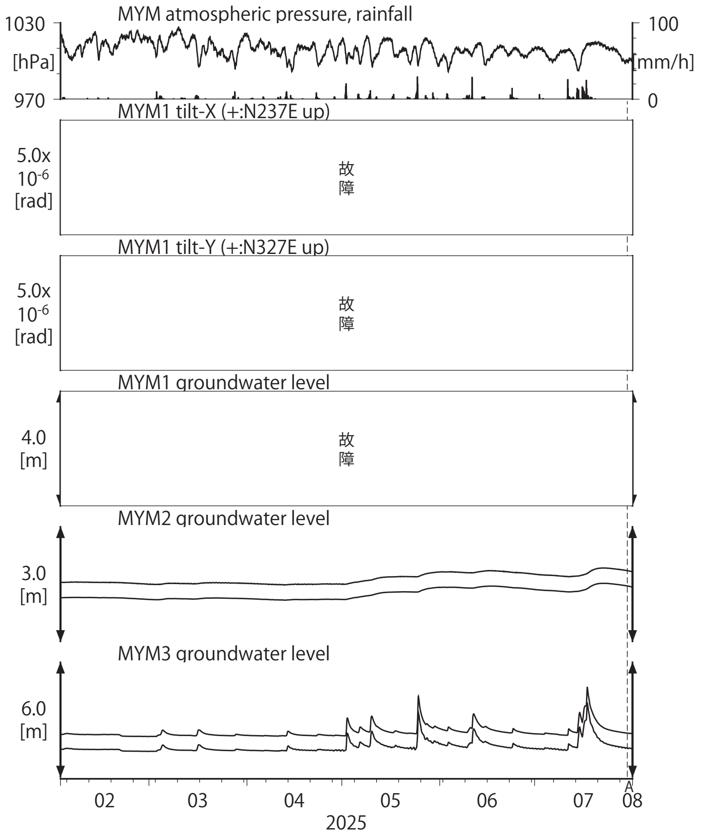
第12図 Tilt and groundwater level at MYM (時間値) (2025/02/01 00:00 - 2025/08/01 00:00 (JST))
