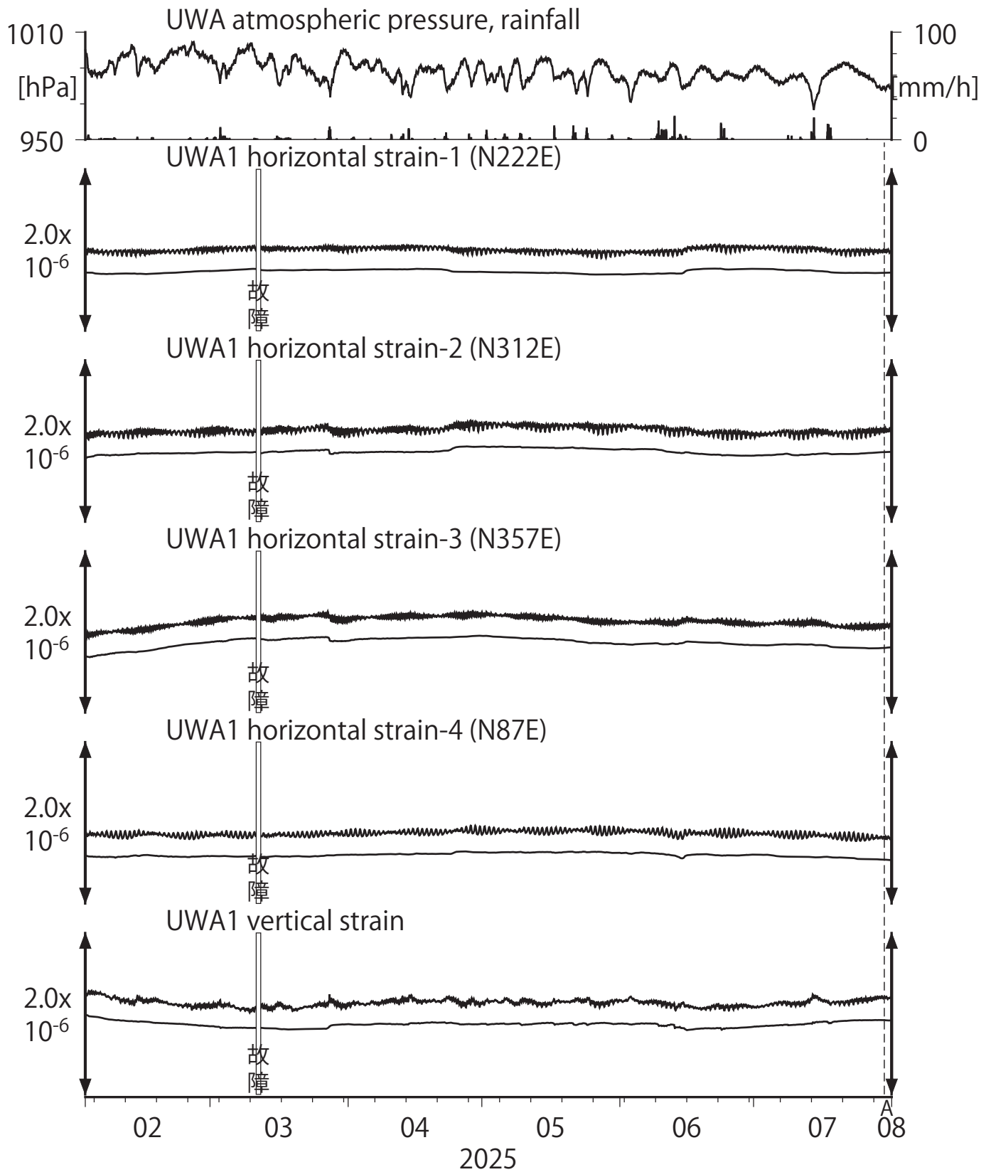
第28図 Crustal strains at UWA (時間値) (2025/02/01 00:00 - 2025/08/01 00:00 (JST))
