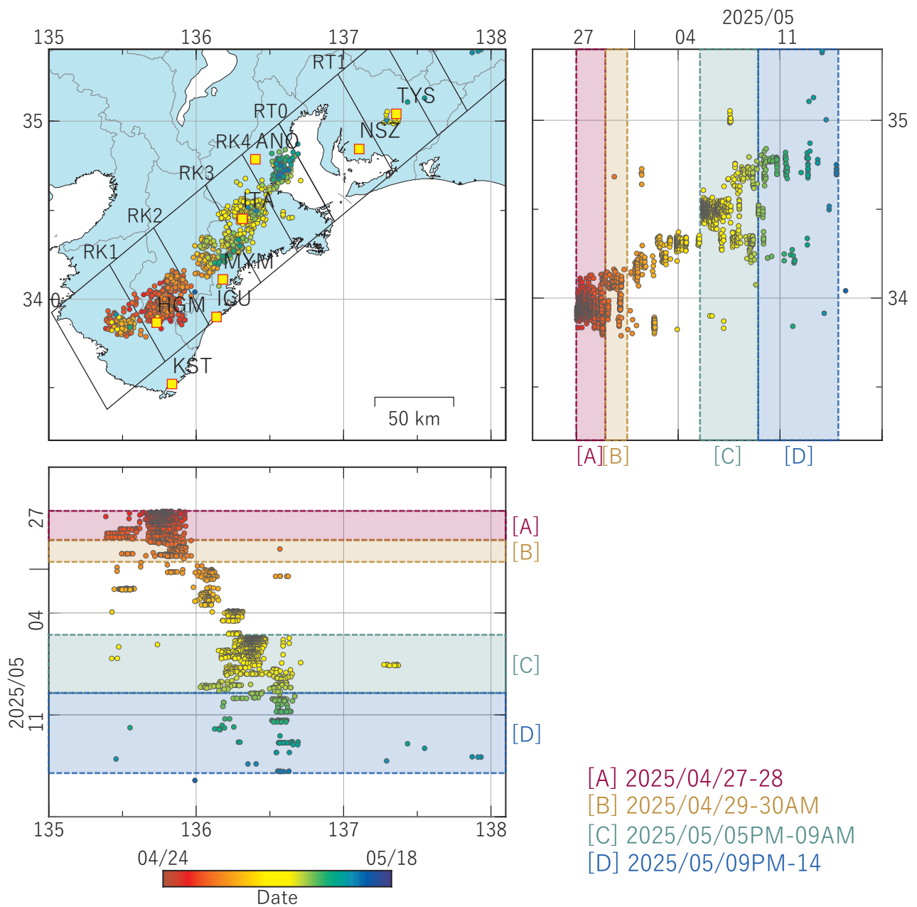
第33図 紀伊半島・東海地方における低周波地震の時空間分布図（2025/04/24 00:00 - 2025/05/18 00:00 (JST)）。気象庁カタログによる。
