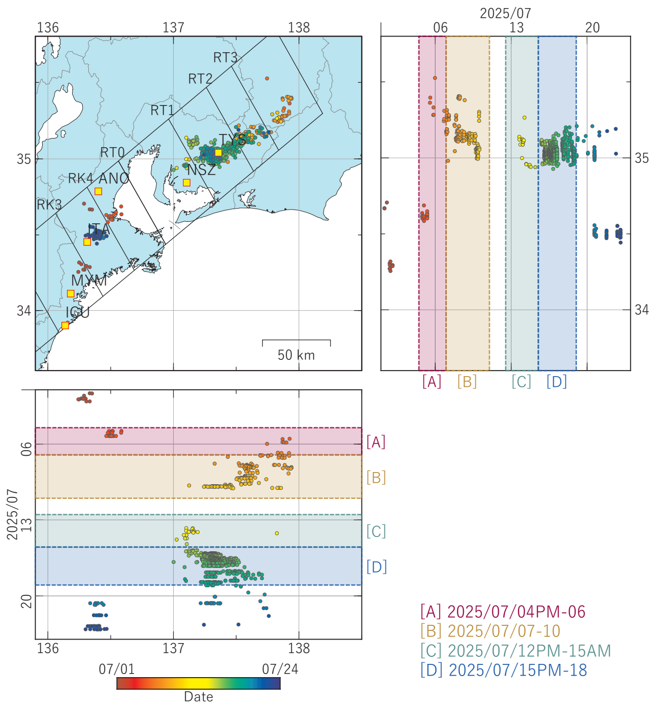
第51図 東海・紀伊半島における低周波地震の時空間分布図 (2025/07/01 00:00 - 2025/07/24 00:00 (JST))。気象庁カタログによる。 (観測点名) TYS: 豊田神殿, NSZ: 西尾善明, ANO: 津安濃, ITA: 松阪飯高, MYM: 紀北海山, ICU: 熊野磯崎
