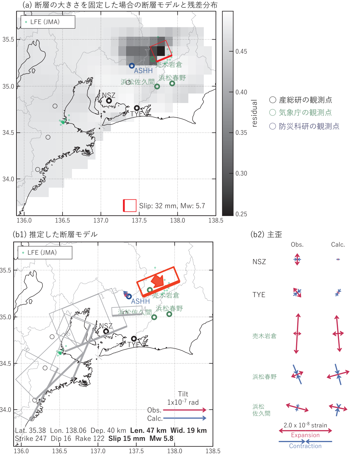
第53図 2025/07/04PM-06の歪・傾斜変化（第52図[A]）を説明する断層モデル。
