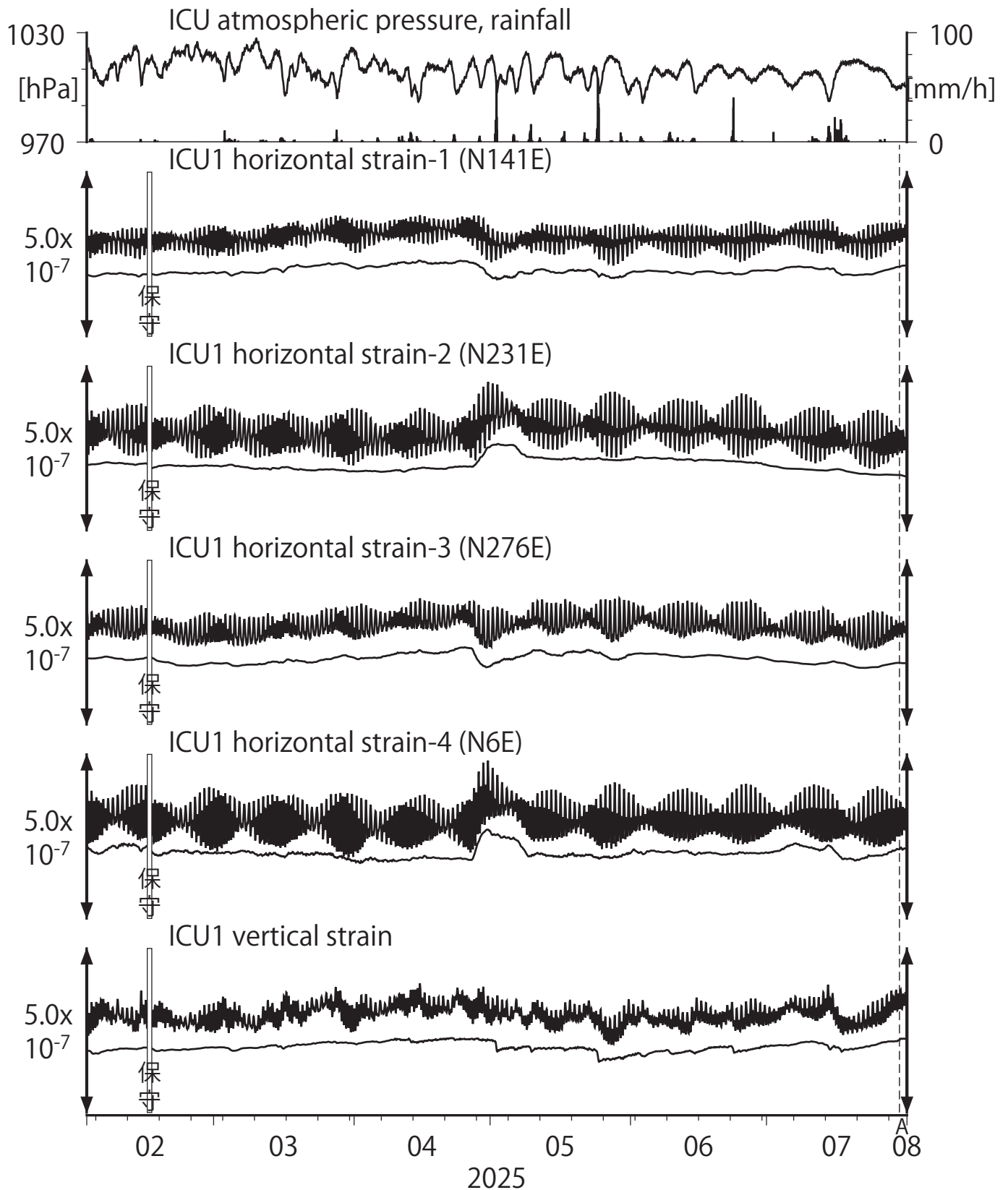
第13図 Crustal strains at ICU (時間値) (2025/02/01 00:00 - 2025/08/01 00:00 (JST))
