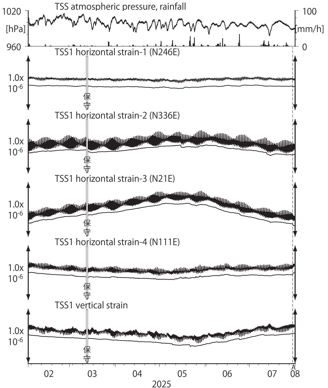
第26図 Crustal strains at TSS (時間値) (2025/02/01 00:00 - 2025/08/01 00:00 (JST))
