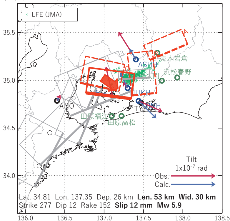
第56図 2025/07/15PM-18の歪・傾斜変化 (第52図[D]) を説明する断層モデル。
