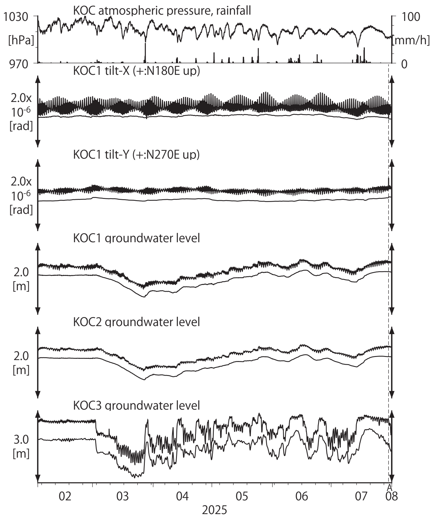
第23図 Tilt and groundwater level at KOC (時間値) (2025/02/01 00:00 - 2025/08/01 00:00 (JST))
