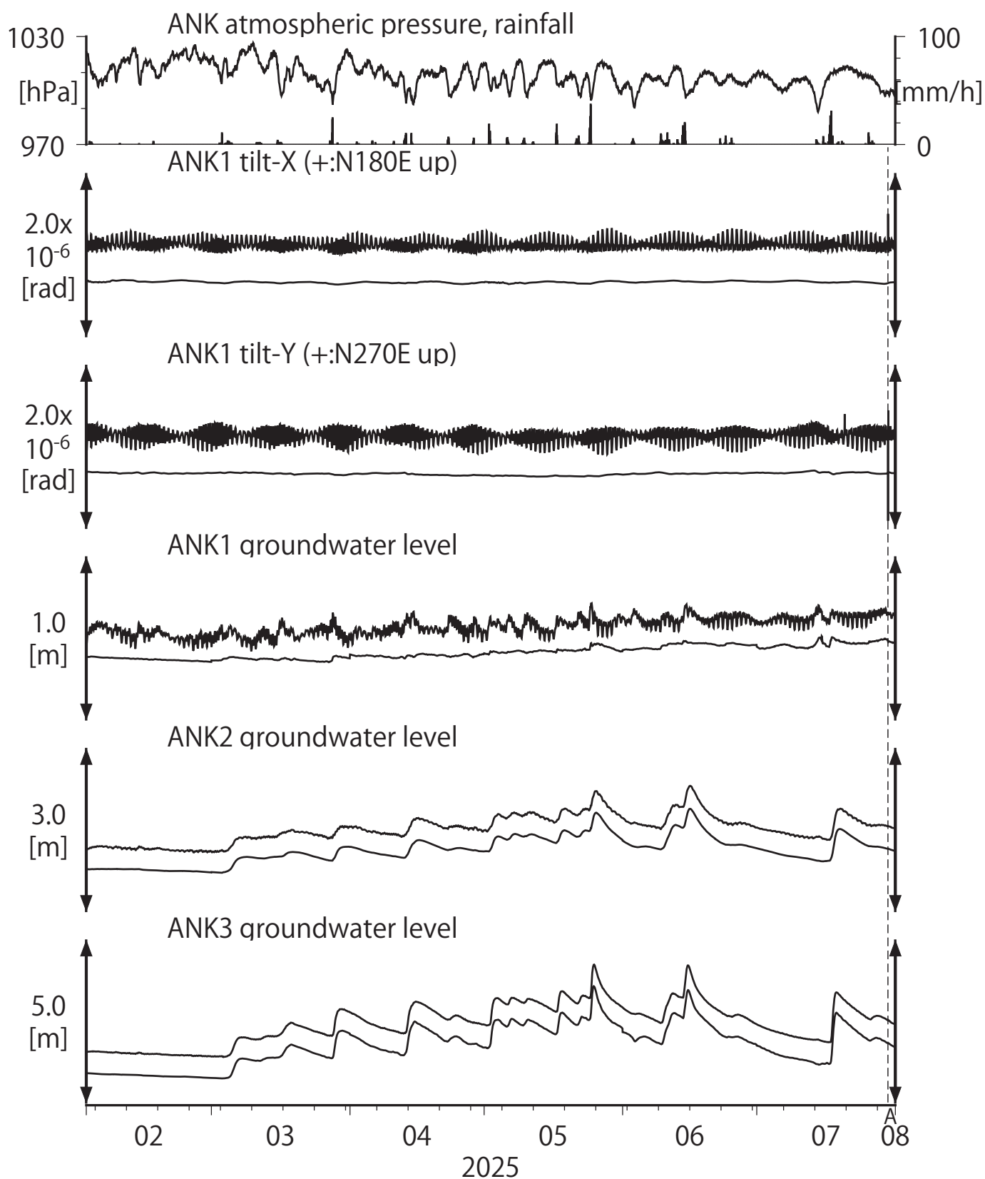
第20図 Tilt and groundwater level at ANK (時間値) (2025/02/01 00:00 - 2025/08/01 00:00 (JST))
