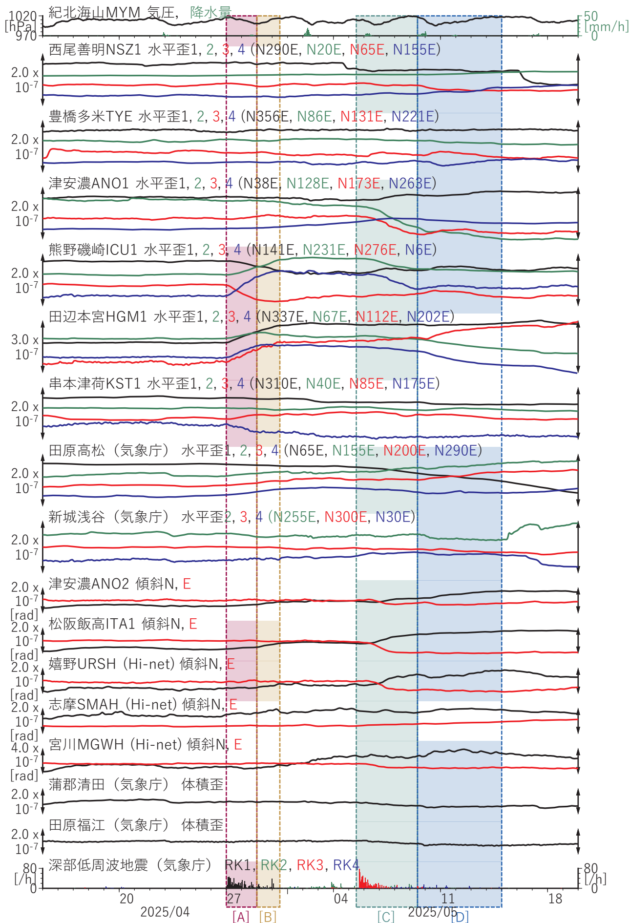
第35図 東海・紀伊半島における歪・傾斜観測結果 (2025/04/15 00:00 - 2025/05/20 00:00 (JST))
