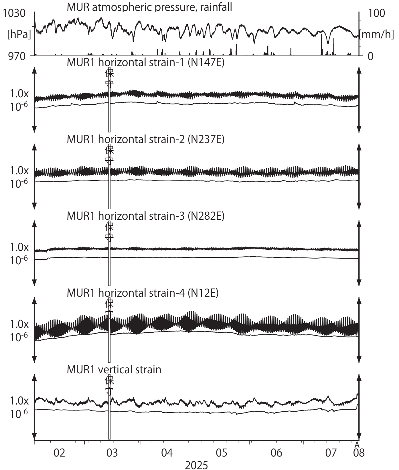
第21図 Crustal strains at MUR (時間値) (2025/02/01 00:00 - 2025/08/01 00:00 (JST))
