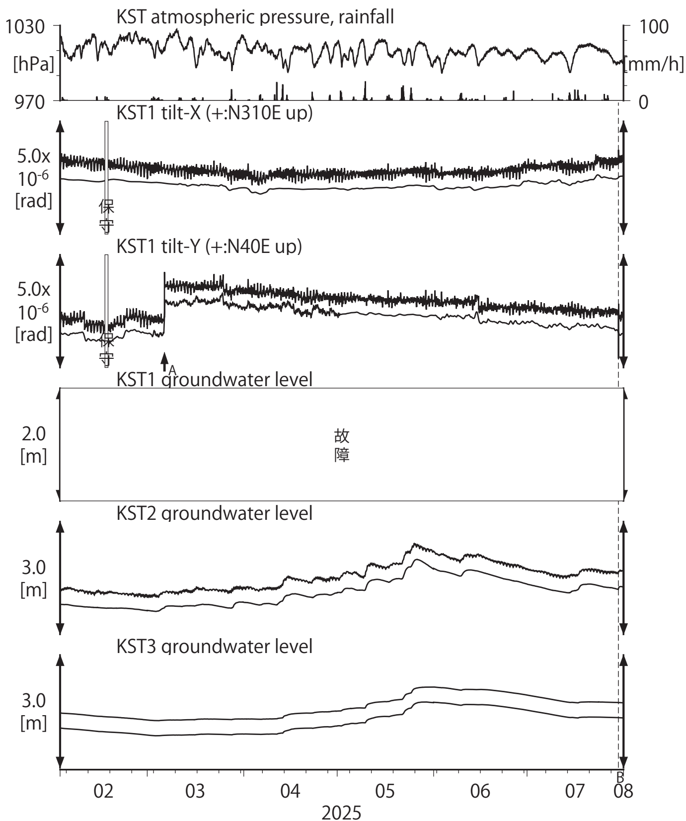
第18図 Tilt and groundwater level at KST (時間値) (2025/02/01 00:00 - 2025/08/01 00:00 (JST))
