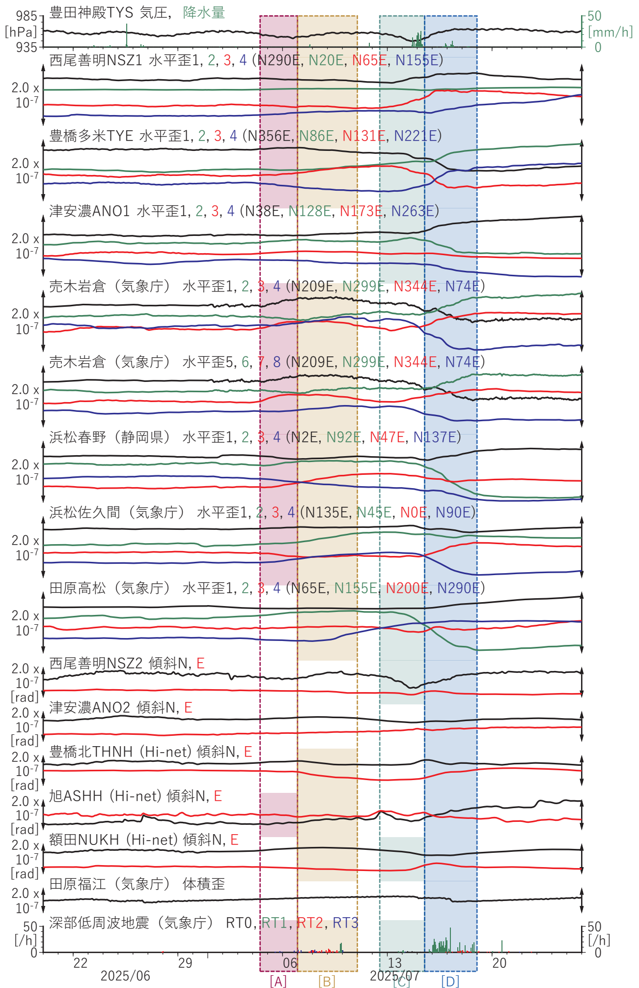
第52図 東海・紀伊半島における歪・傾斜観測結果 (2025/06/20 00:00 - 2025/07/26 00:00 (JST))
