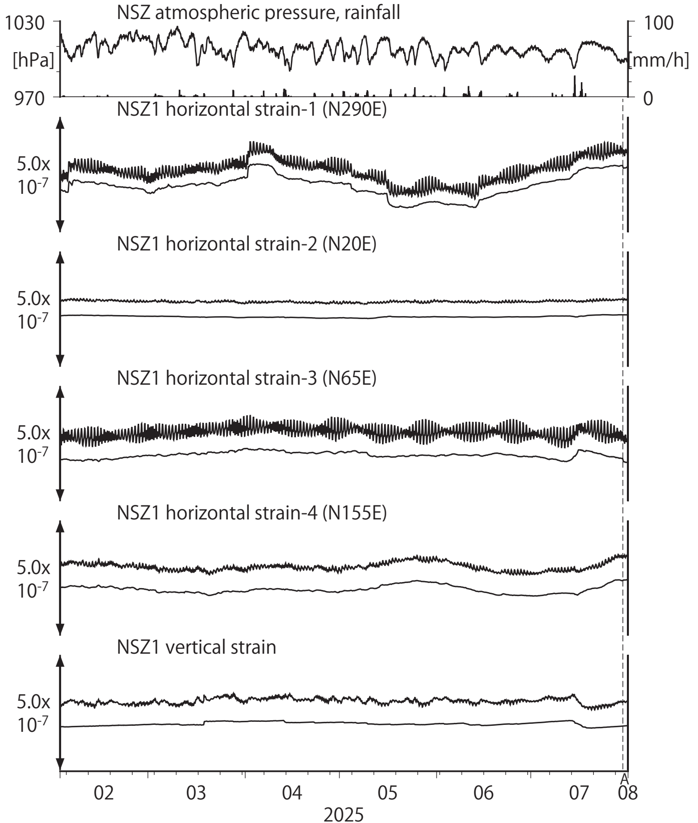
第4図 Crustal strains at NSZ (時間値) (2025/02/01 00:00 - 2025/08/01 00:00 (JST))
