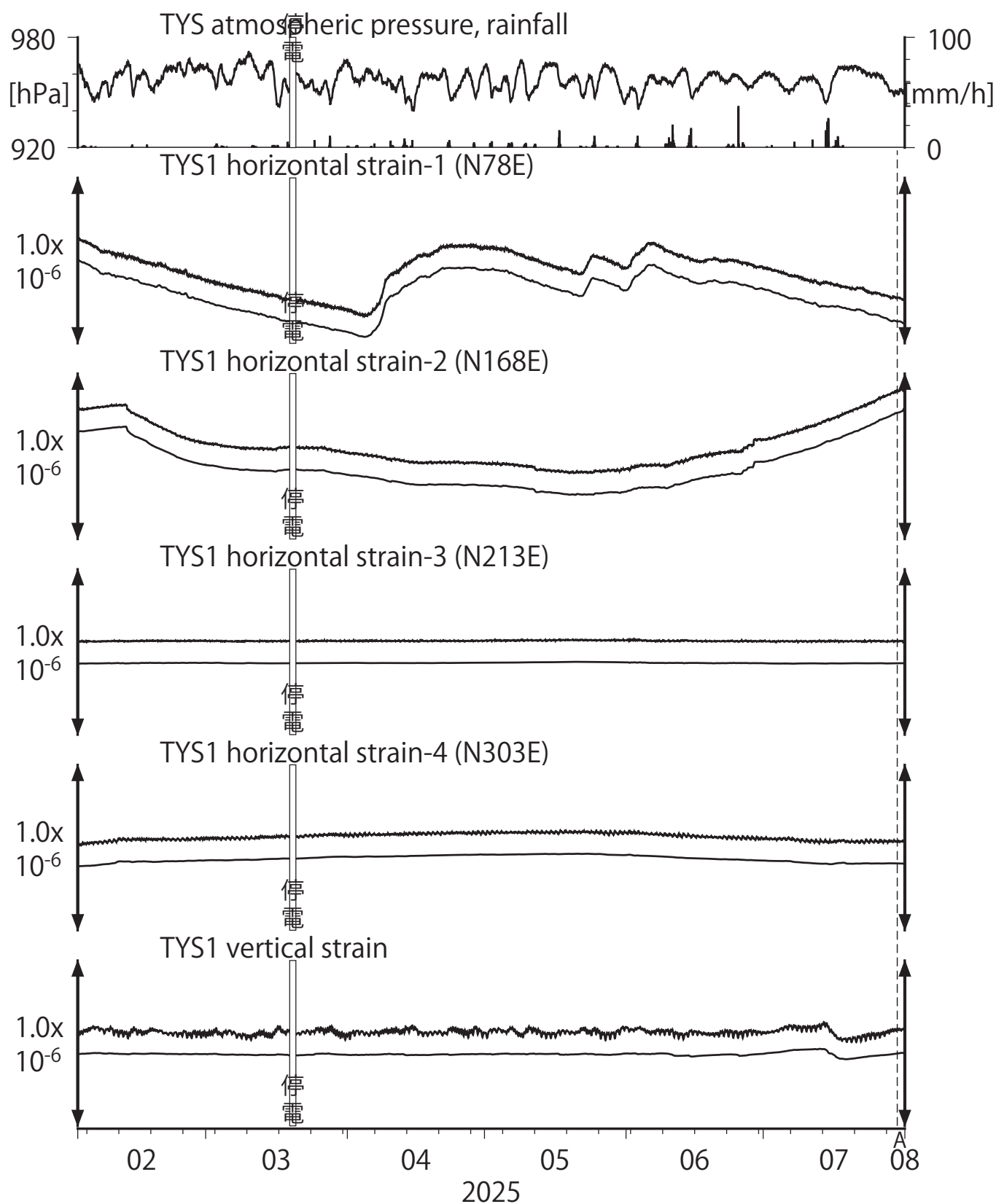
第2図 Crustal strains at TYS (時間値) (2025/02/01 00:00 - 2025/08/01 00:00 (JST))
