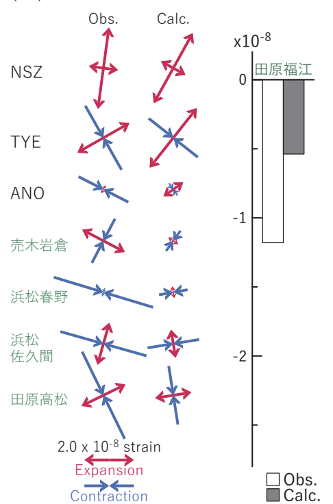
第56図 2025/07/15PM-18の歪・傾斜変化 (第52図[D]) を説明する断層モデル。
