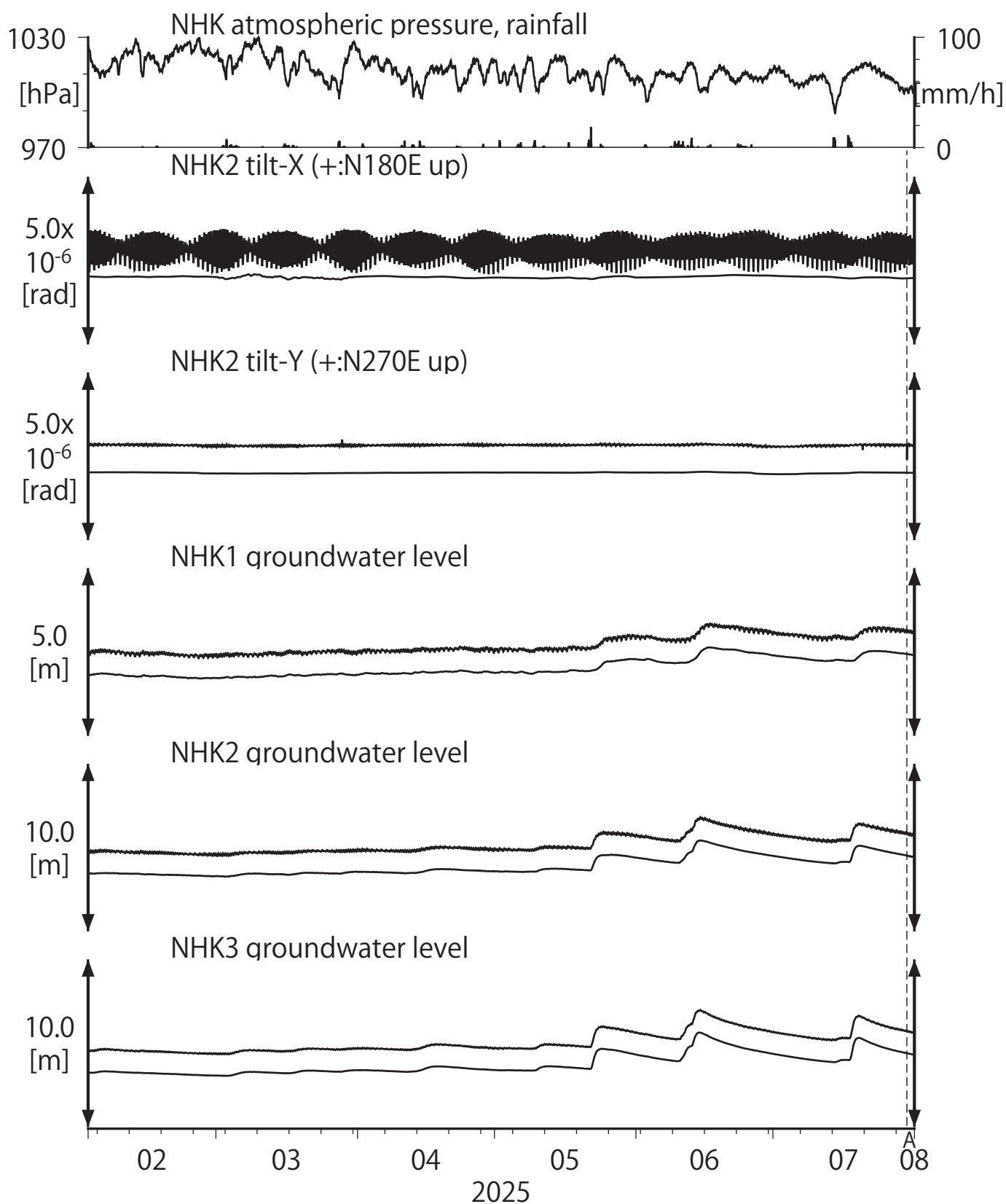
第32図 Tilt and groundwater level at NHK (時間値) (2025/02/01 00:00 - 2025/08/01 00:00 (JST))
