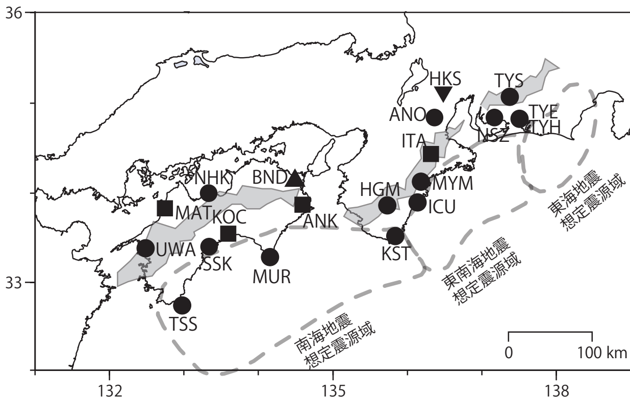
第1図: 産総研の地殻変動・地下水観測点の分布図 (●・■・▲・▼)。それぞれの観測点に設置されている機器は次のとおり。●はボアホール歪・傾斜計（デジタル）および水位計。■は傾斜計および水位計。▲はボアホール歪計（アナログ）および水位計。▼は水位計。灰色の領域は短期的SSE及び深部低周波微動が定常的に発生していると考えられる地域。
