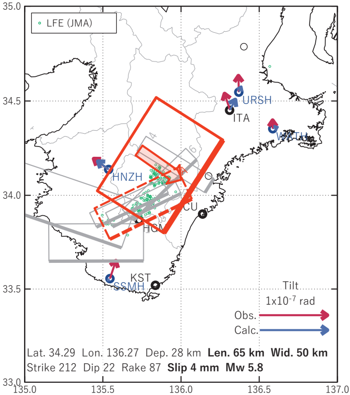
第37図 2025/04/29-30AMの歪・傾斜変化（第34図[B]）を説明する断層モデル。
