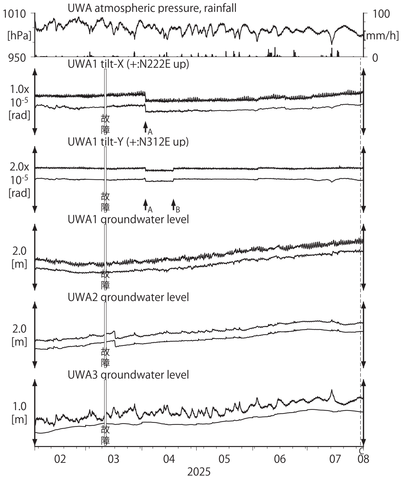
第29図 Tilt and groundwater level at UWA (時間値) (2025/02/01 00:00 - 2025/08/01 00:00 (JST))
