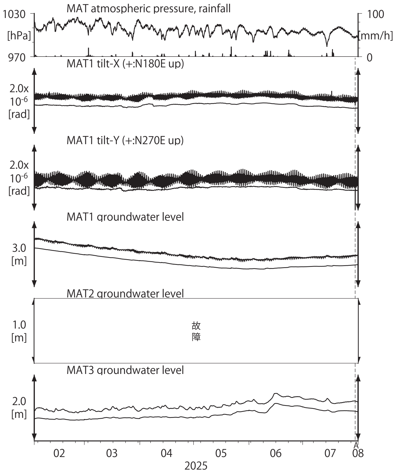
第30図 Tilt and groundwater level at MAT (時間値) (2025/02/01 00:00 - 2025/08/01 00:00 (JST))
