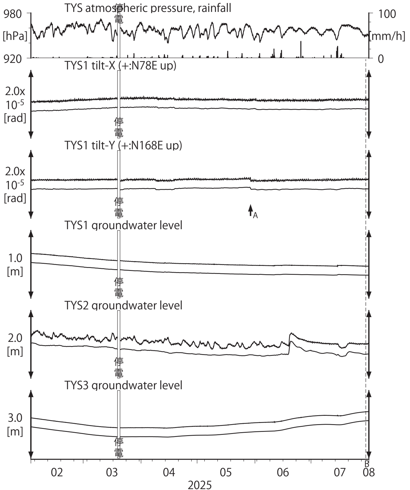
第3図 Tilt and groundwater level at TYS (時間値) (2025/02/01 00:00 - 2025/08/01 00:00 (JST))
