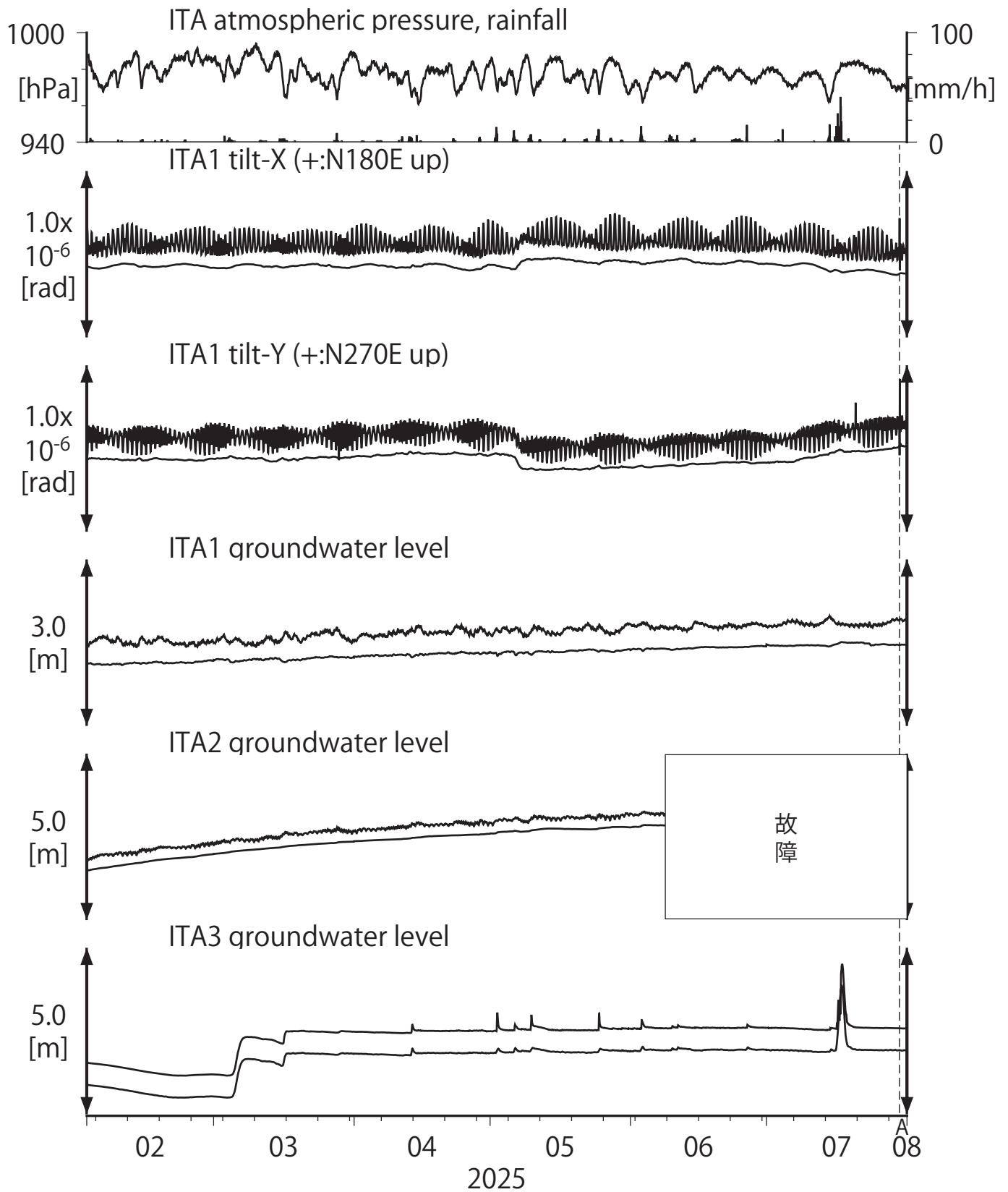
第10図 Tilt and groundwater level at ITA (時間値) (2025/02/01 00:00 - 2025/08/01 00:00 (JST))
