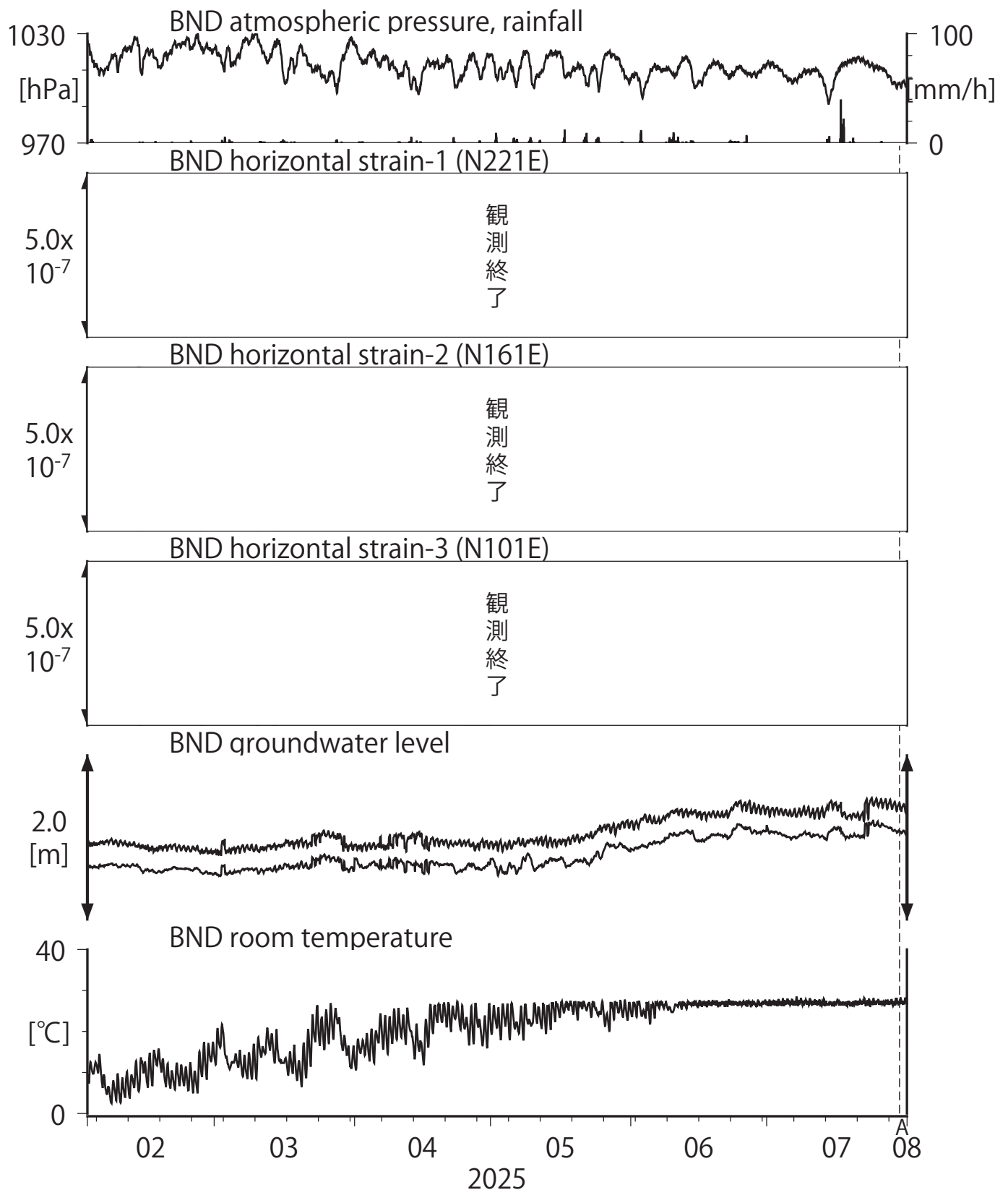
第19図 Crustal strains and groundwater level at BND (時間値) (2025/02/01 00:00 - 2025/08/01 00:00 (JST))
