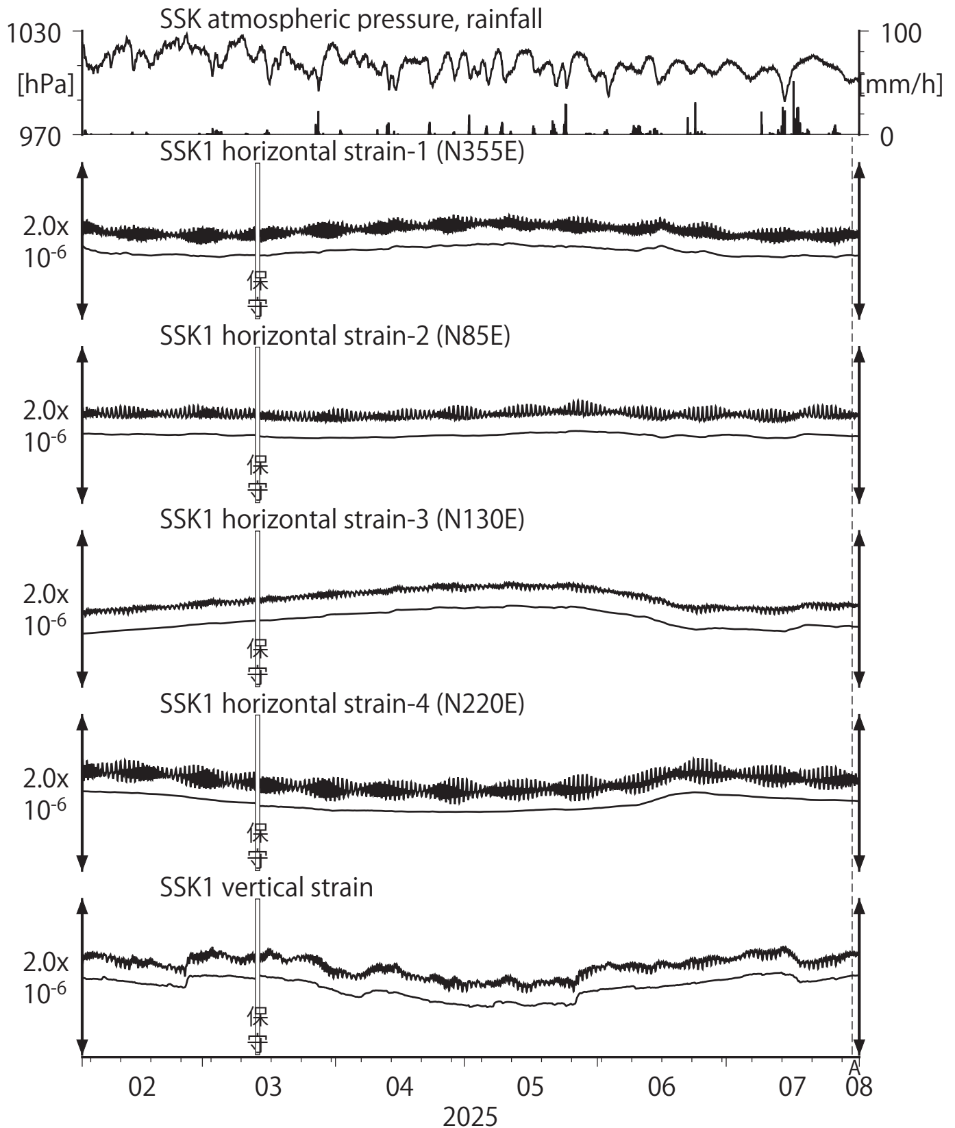
第24図 Crustal strains at SSK (時間値) (2025/02/01 00:00 - 2025/08/01 00:00 (JST))
