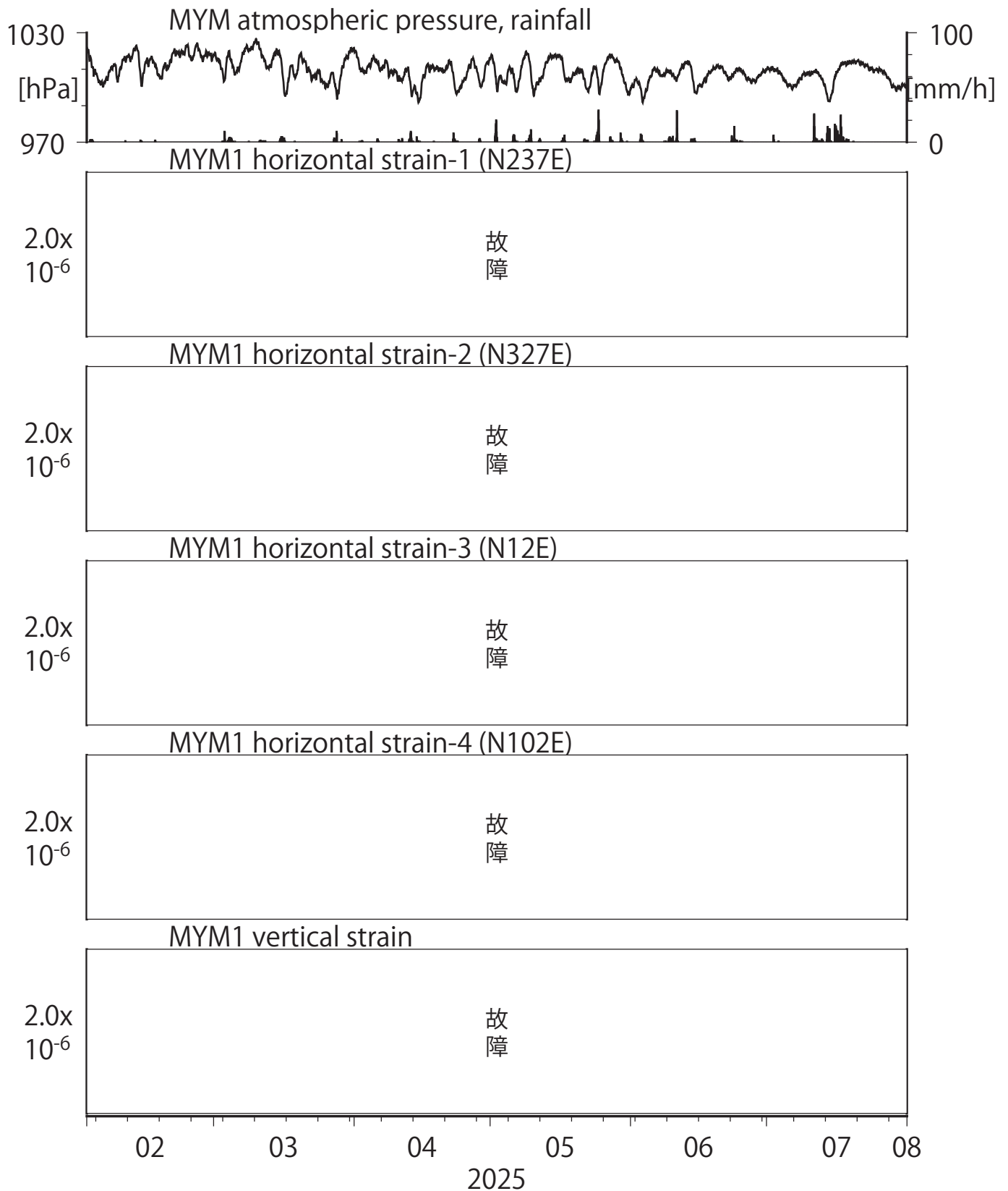
第11図 Crustal strains at MYM (時間値) (2025/02/01 00:00 - 2025/08/01 00:00 (JST))
