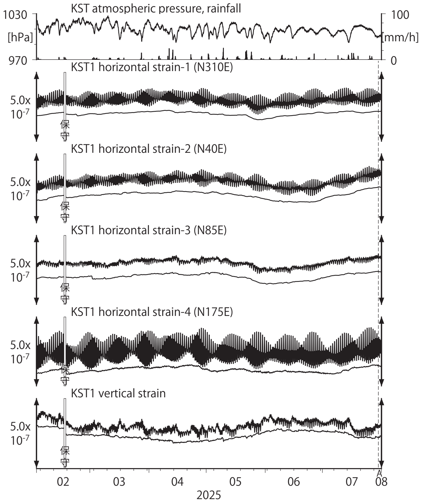
第17図 Crustal strains at KST (時間値) (2025/02/01 00:00 - 2025/08/01 00:00 (JST))
