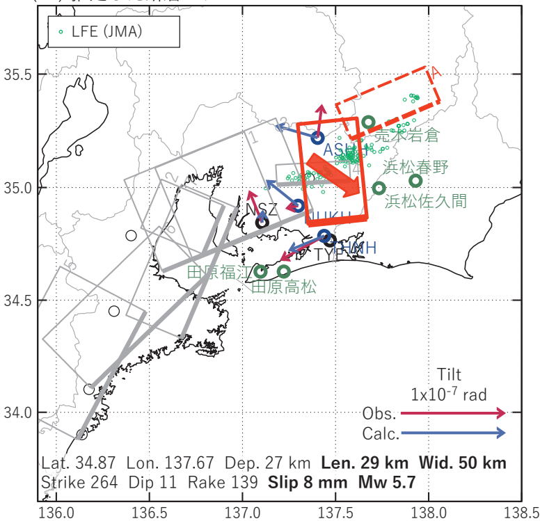
第54図 2025/07/07-10の歪・傾斜変化（第52図[B]）を説明する断層モデル。
