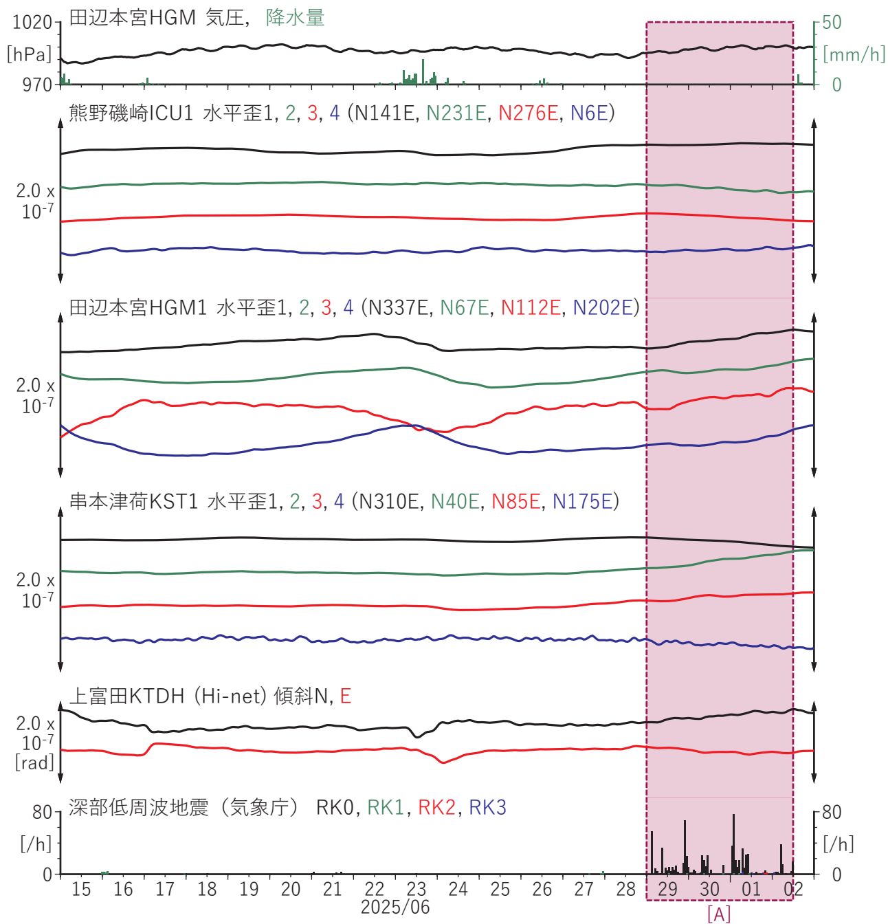
第49図 紀伊半島における歪・傾斜観測結果 (2025/06/15 00:00 - 2025/07/03 00:00 (JST))
