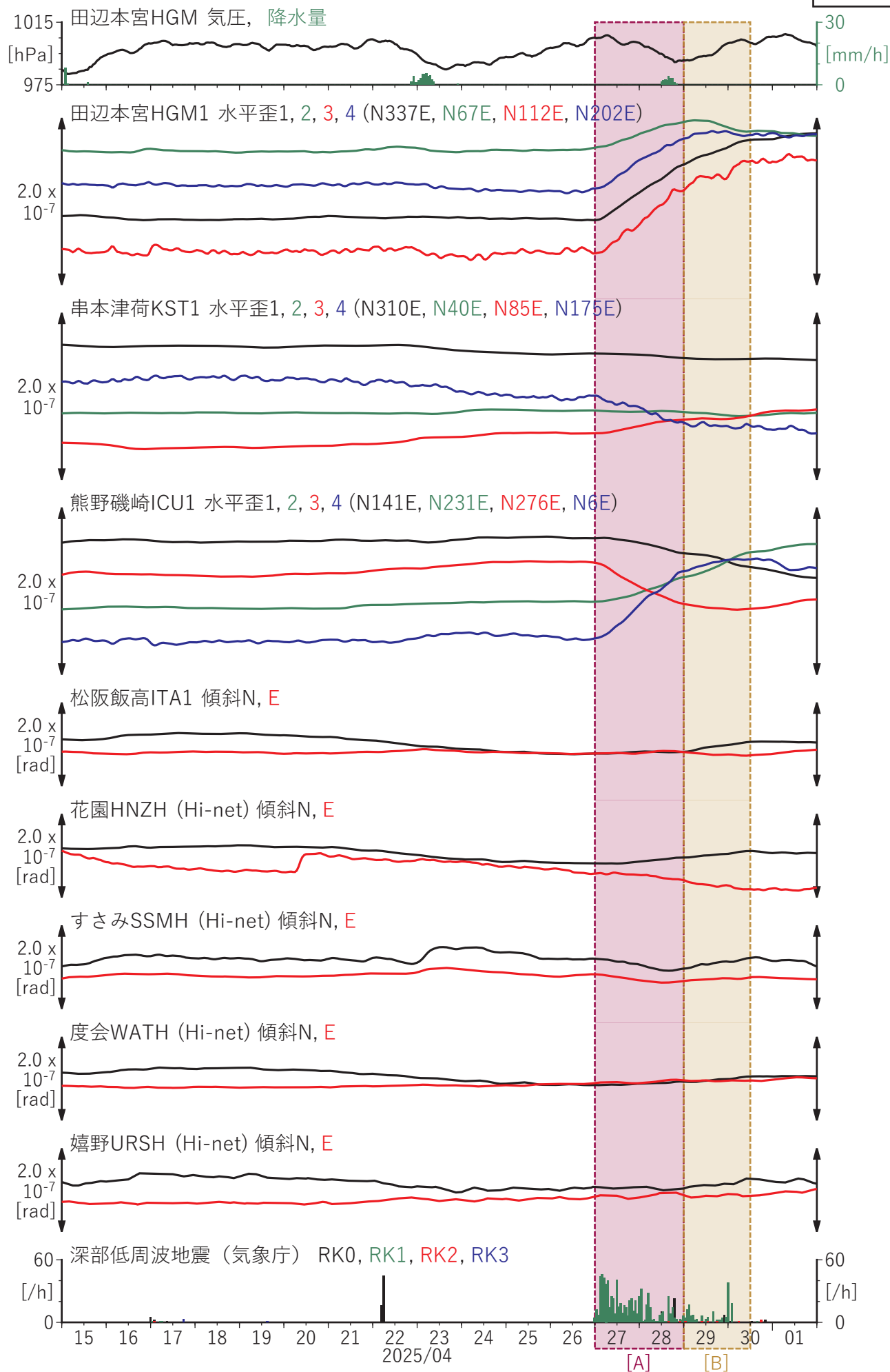
第34図 紀伊半島における歪・傾斜の時間変化 (2025/04/15 00:00 - 2025/05/02 00:00 (JST))
