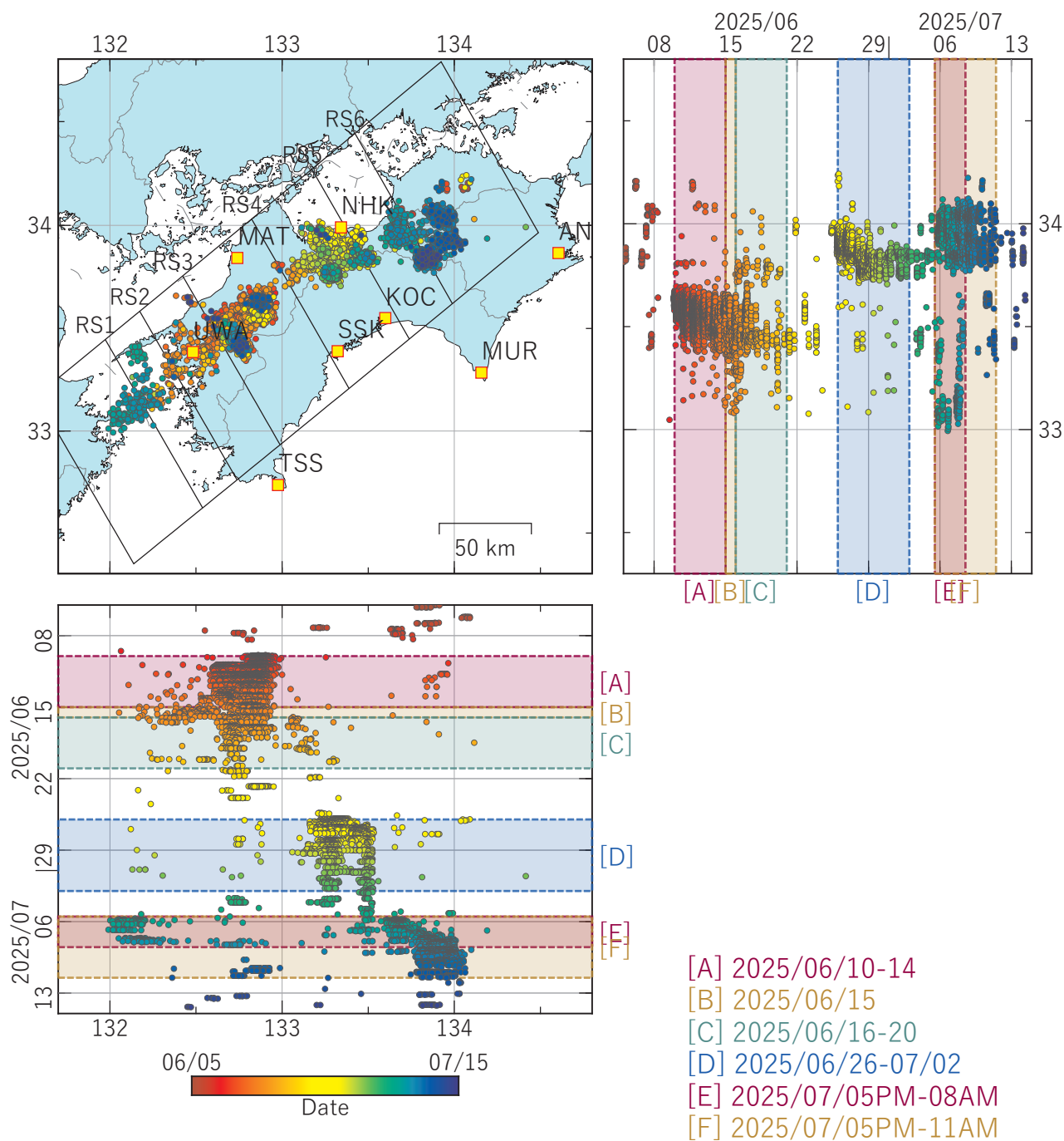
第40図 四国地方における低周波地震の時空間分布図 (2025/06/05 00:00 - 2025/07/15 00:00 (JST))。気象庁カタログによる。 (観測点名) ANK: 阿南桑野, MUR: 室戸岬, NHK: 新居浜黒島, KOC: 高知五台山, SSK: 須崎大谷, MAT: 松山南江戸, UWA: 西予宇和, TSS: 土佐清水松尾
