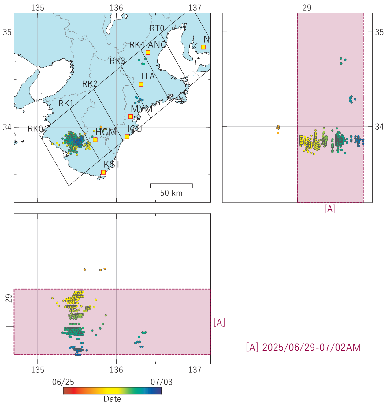
第48図 紀伊半島における低周波地震の時空間分布図（2025/06/25 00:00 - 2025/07/03 00:00 (JST)）。気象庁カタログによる。 （観測点名）NSZ: 西尾善明, ANO: 津安濃, ITA: 松阪飯高, MYM: 紀北海山, ICU: 熊野磯崎, HGM: 田辺本宮, KST: 串本津荷
