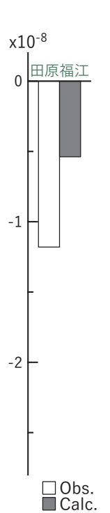
第56図 2025/07/15PM-18の歪・傾斜変化 (第52図[D]) を説明する断層モデル。
