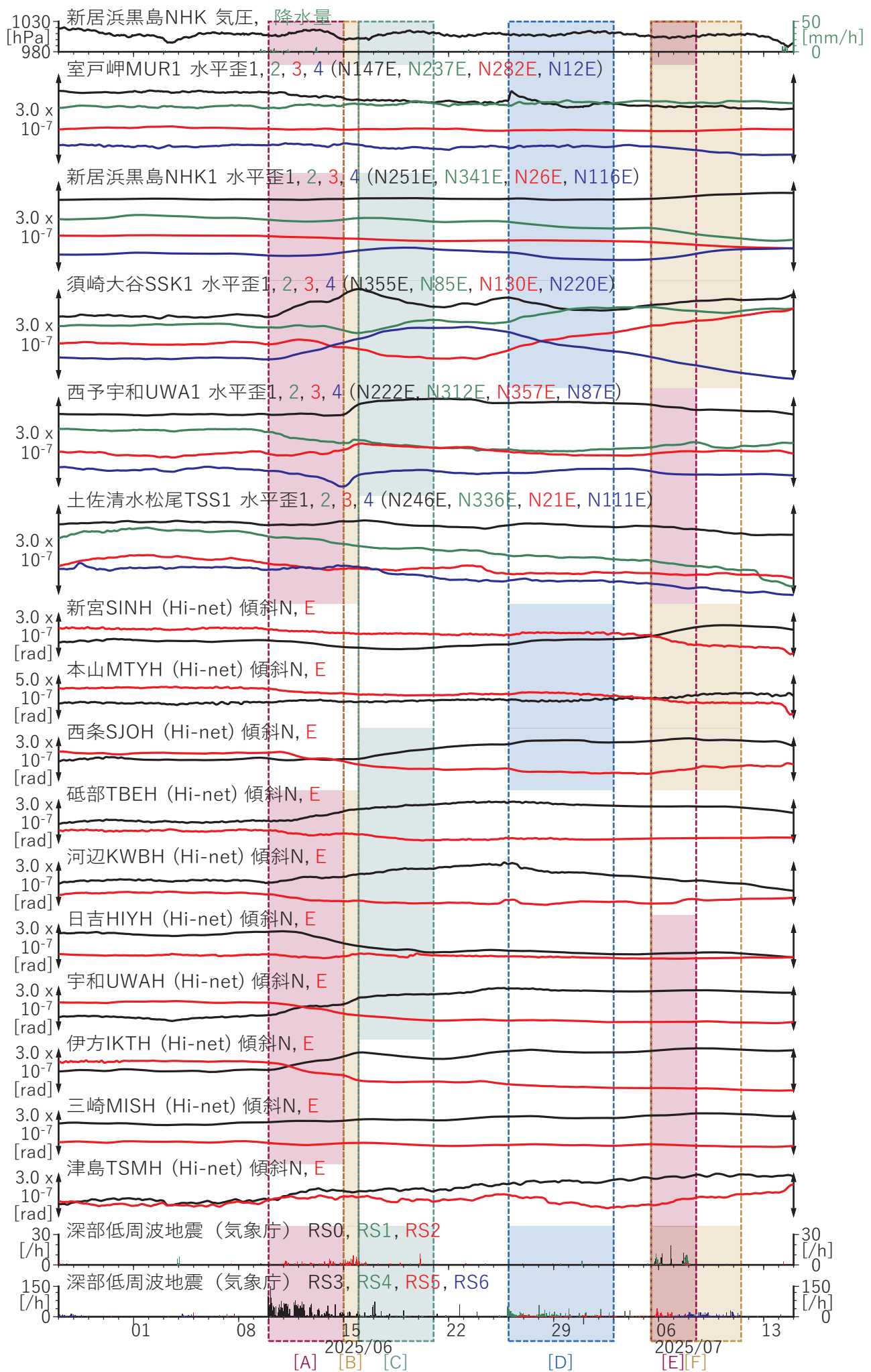
第41図 四国地方における歪・傾斜観測結果 (2025/05/27 00:00 - 2025/07/15 00:00 (JST))
