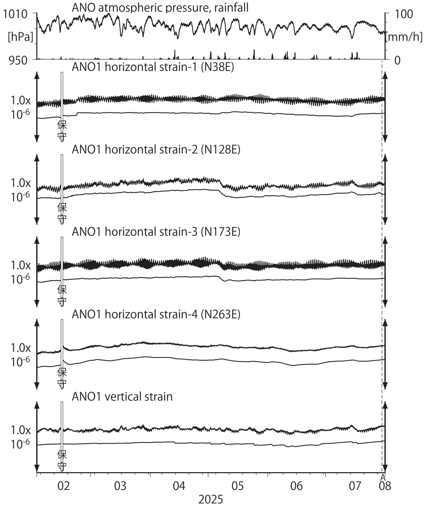
第8図 Crustal strains at ANO (時間値) (2025/02/01 00:00 - 2025/08/01 00:00 (JST))
