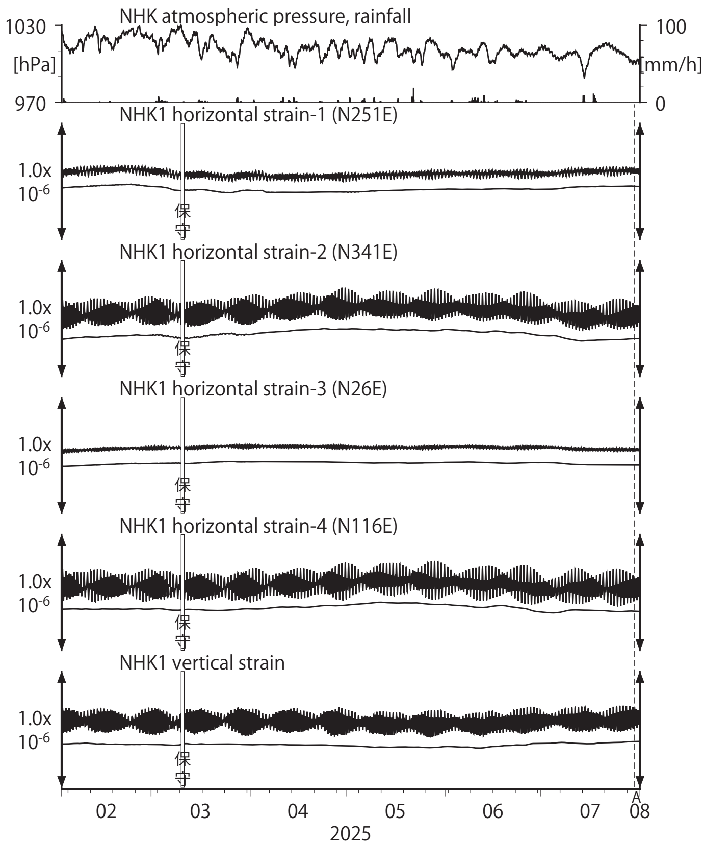
第31図 Crustal strains at NHK (時間値) (2025/02/01 00:00 - 2025/08/01 00:00 (JST))
