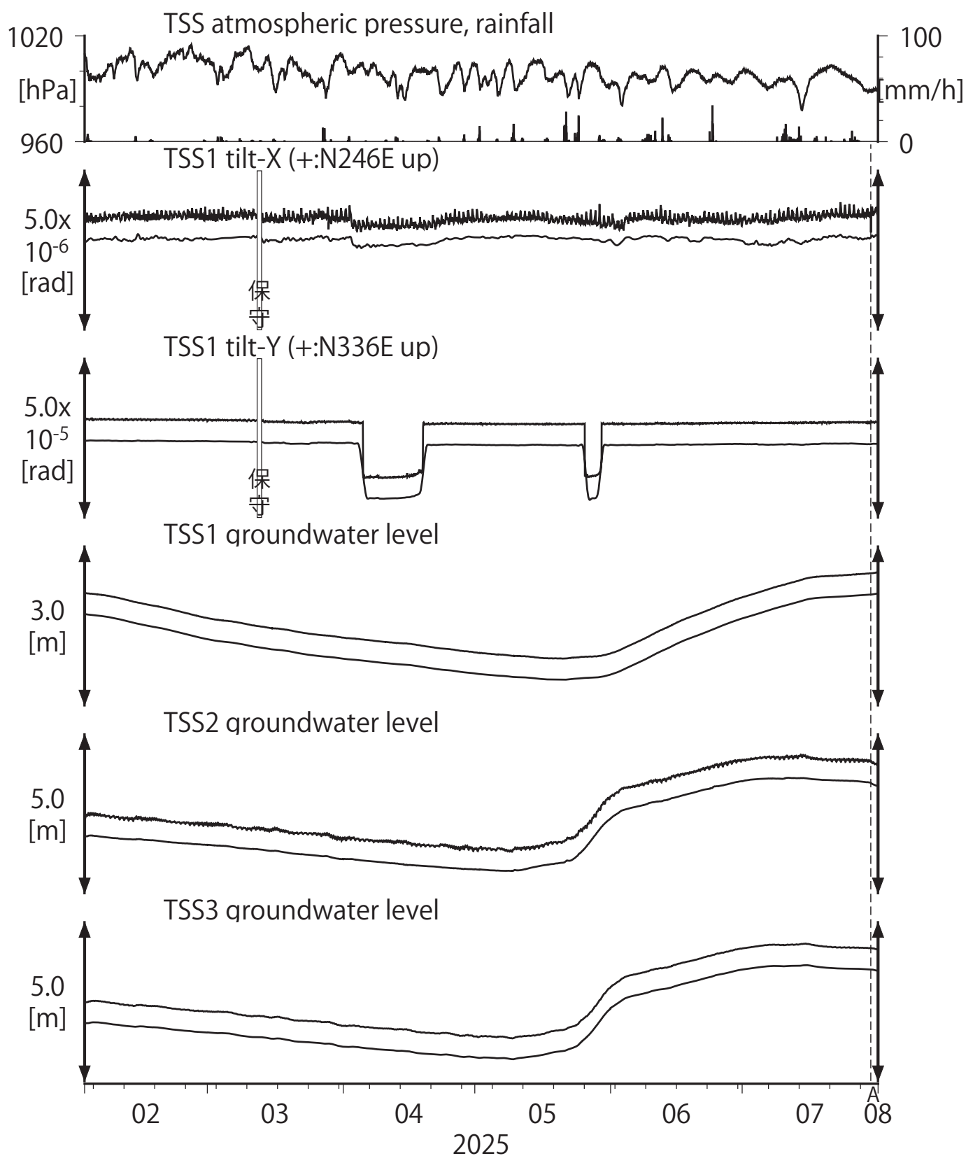
第27図 Tilt and groundwater level at TSS (時間値) (2025/02/01 00:00 - 2025/08/01 00:00 (JST))
