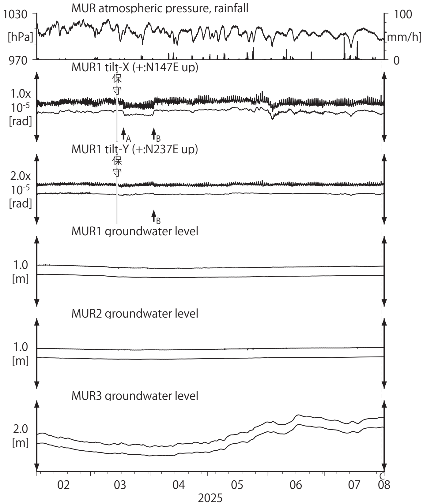
第22図 Tilt and groundwater level at MUR (時間値) (2025/02/01 00:00 - 2025/08/01 00:00 (JST))
