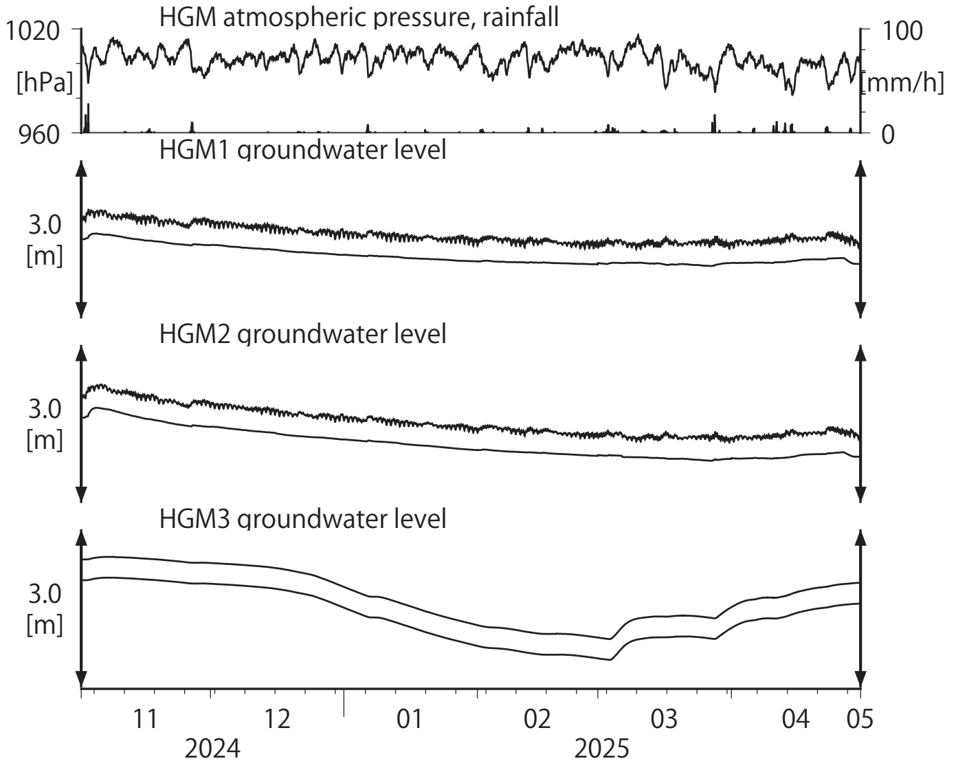
第16図 Tilt and groundwater level at HGM (時間値) (2024/11/01 00:00 - 2025/05/01 00:00 (JST))
