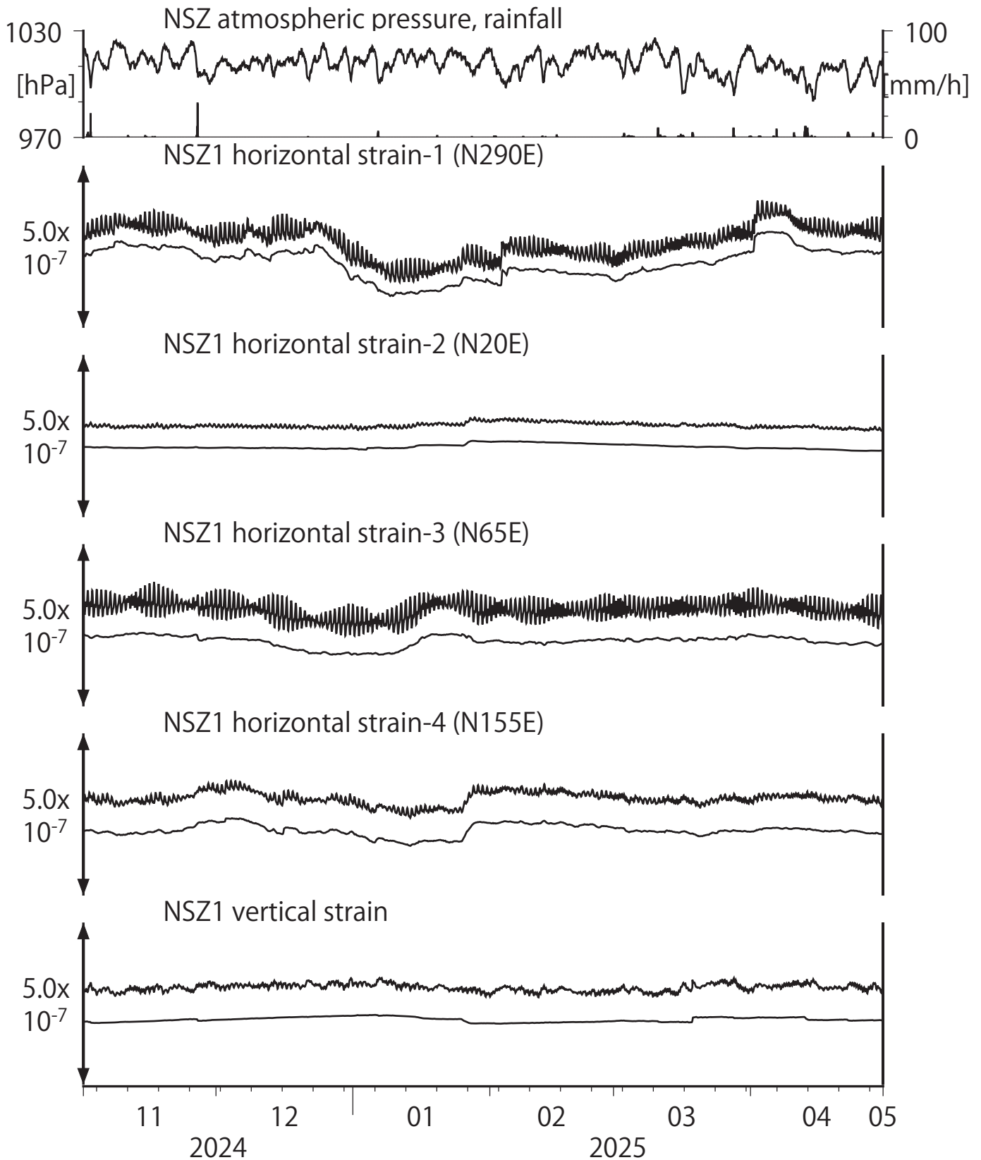
第4図 Crustal strains at NSZ (時間値) (2024/11/01 00:00 - 2025/05/01 00:00 (JST))
