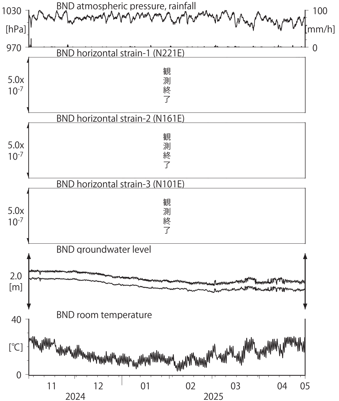
第19図 Crustal strains and groundwater level at BND (時間値) (2024/11/01 00:00 - 2025/05/01 00:00 (JST))
