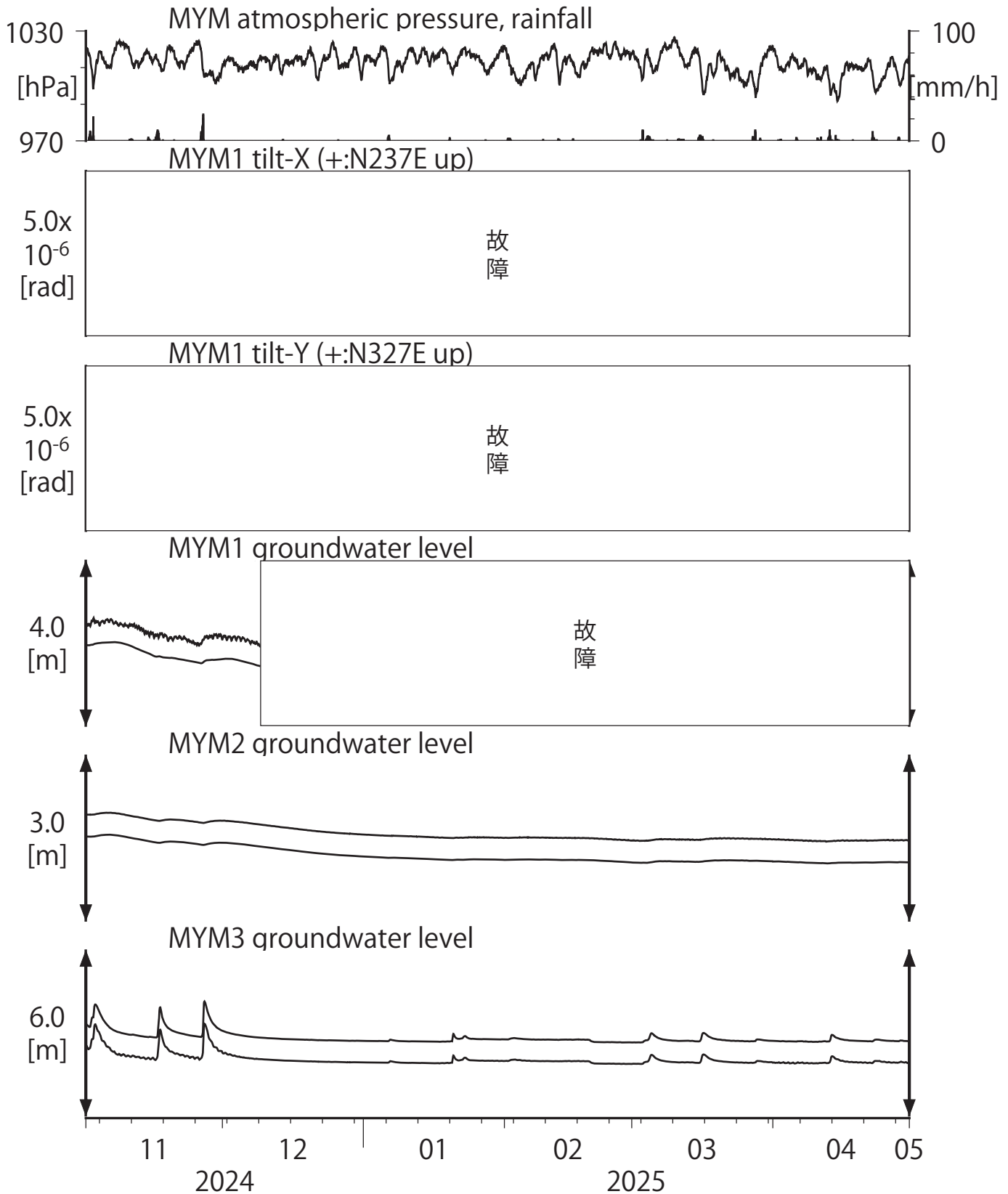
第12図 Tilt and groundwater level at MYM (時間値) (2024/11/01 00:00 - 2025/05/01 00:00 (JST))
