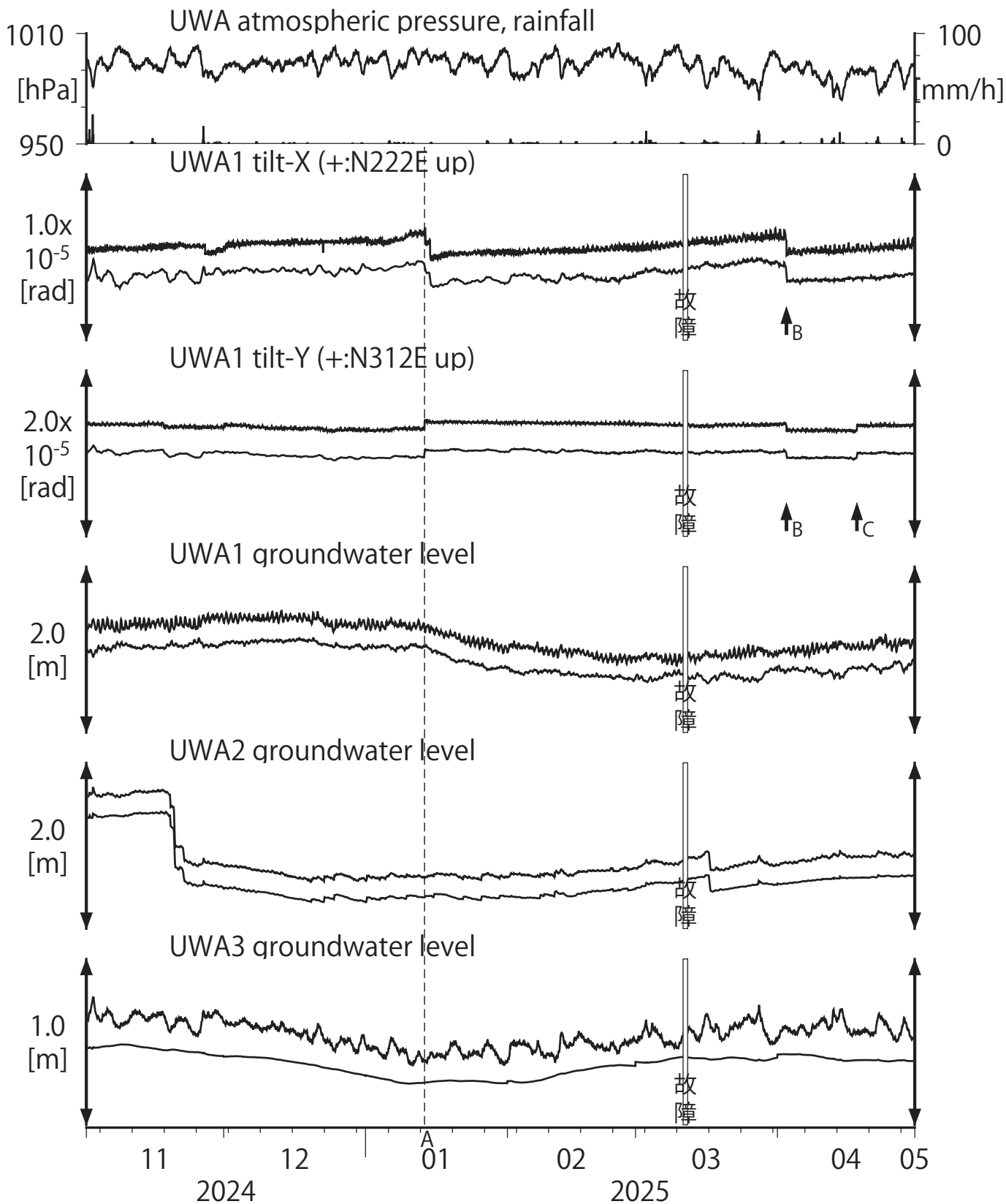
第29図 Tilt and groundwater level at UWA (時間値) (2024/11/01 00:00 - 2025/05/01 00:00 (JST))
