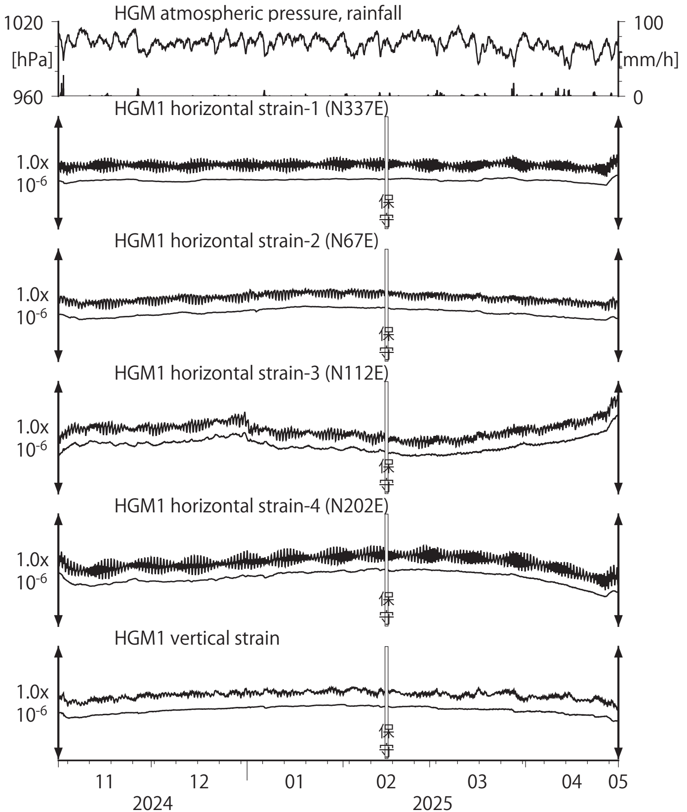
第15図 Crustal strains at HGM (時間値) (2024/11/01 00:00 - 2025/05/01 00:00 (JST))
