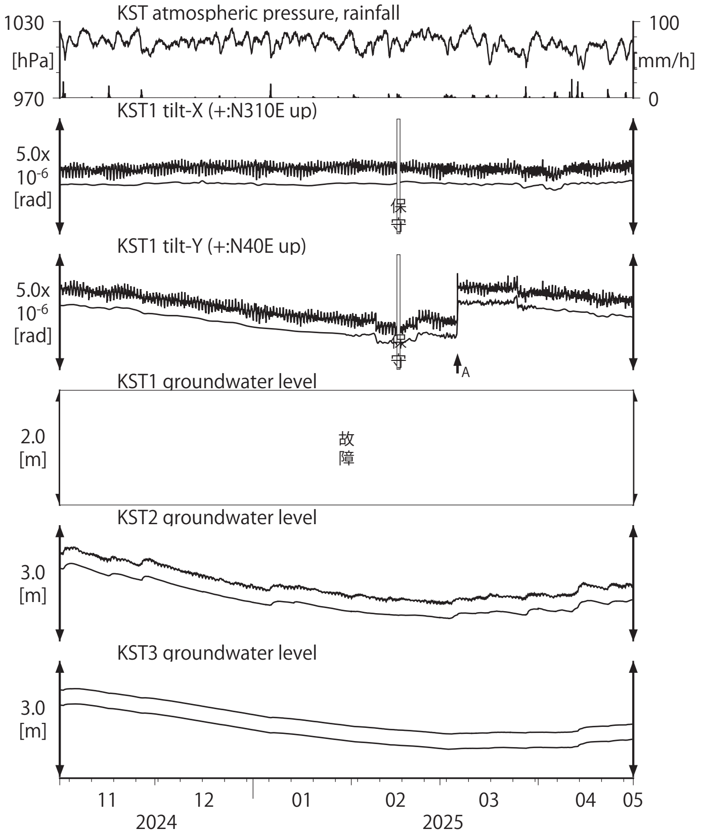
第18図 Tilt and groundwater level at KST (時間値) (2024/11/01 00:00 - 2025/05/01 00:00 (JST))
