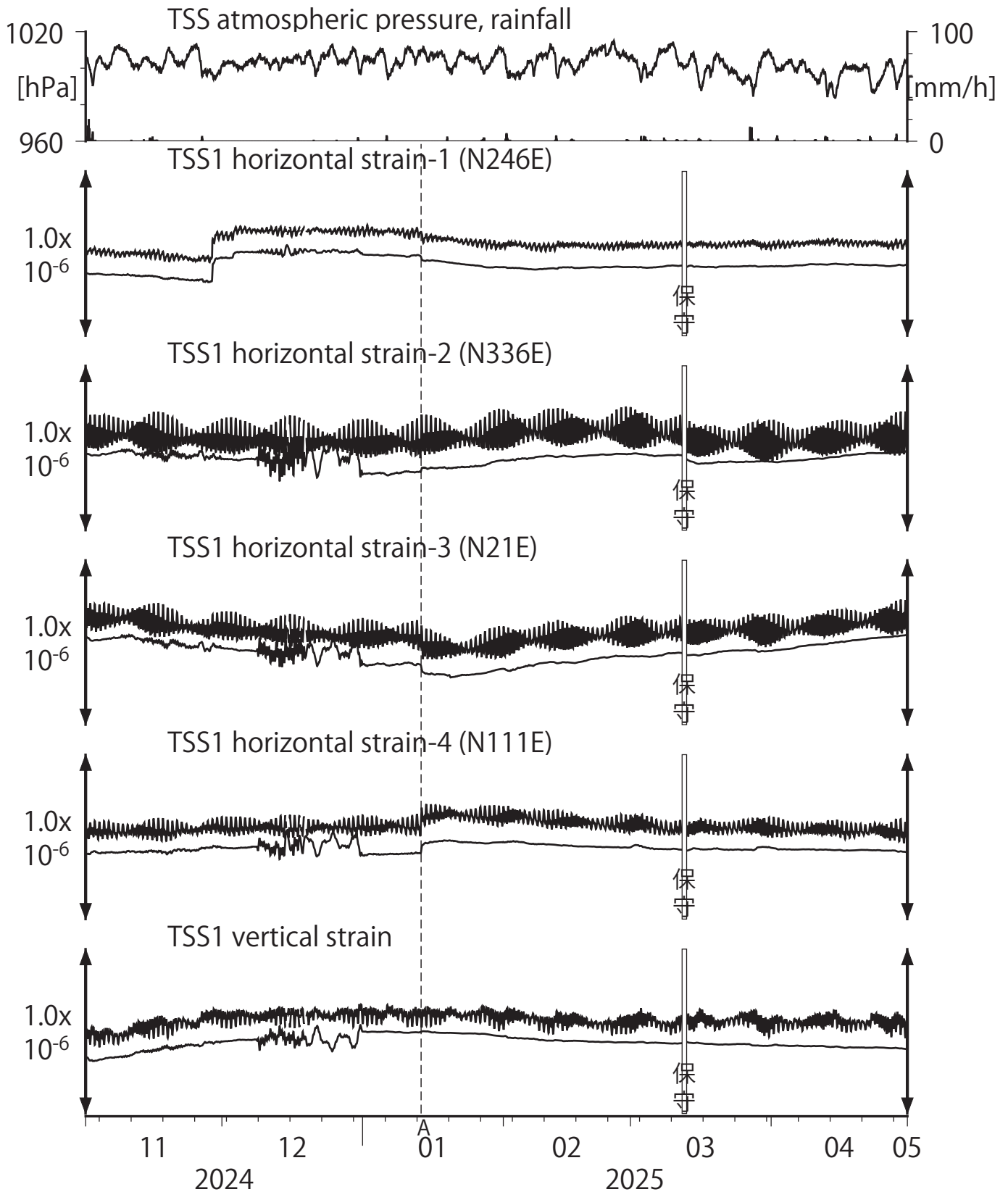
第26図 Crustal strains at TSS (時間値) (2024/11/01 00:00 - 2025/05/01 00:00 (JST))
