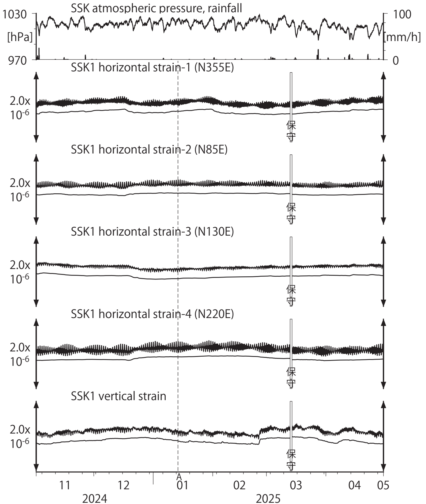
第24図 Crustal strains at SSK (時間値) (2024/11/01 00:00 - 2025/05/01 00:00 (JST))
