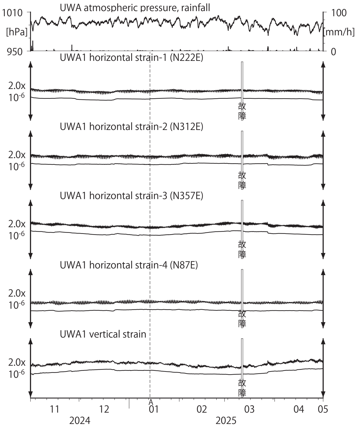
第28図 Crustal strains at UWA (時間値) (2024/11/01 00:00 - 2025/05/01 00:00 (JST))
