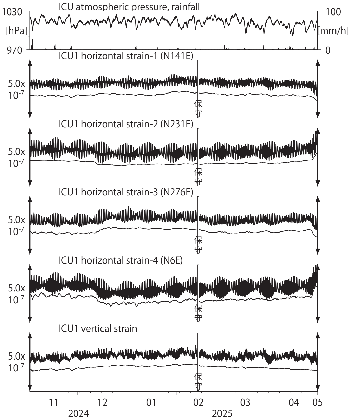
第13図 Crustal strains at ICU (時間値) (2024/11/01 00:00 - 2025/05/01 00:00 (JST))
