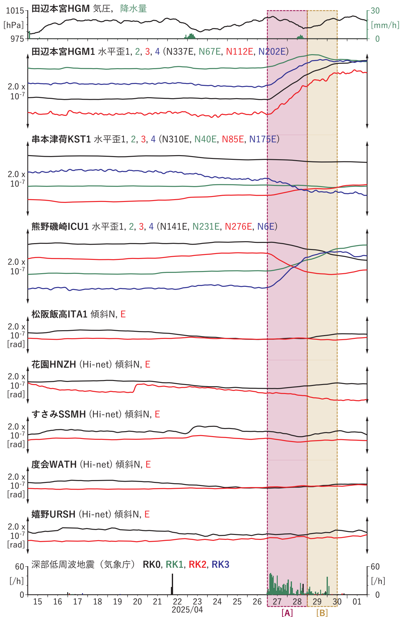
第42図 紀伊半島における歪・傾斜の時間変化 (2025/04/15 00:00 - 2025/05/02 00:00 (JST))
