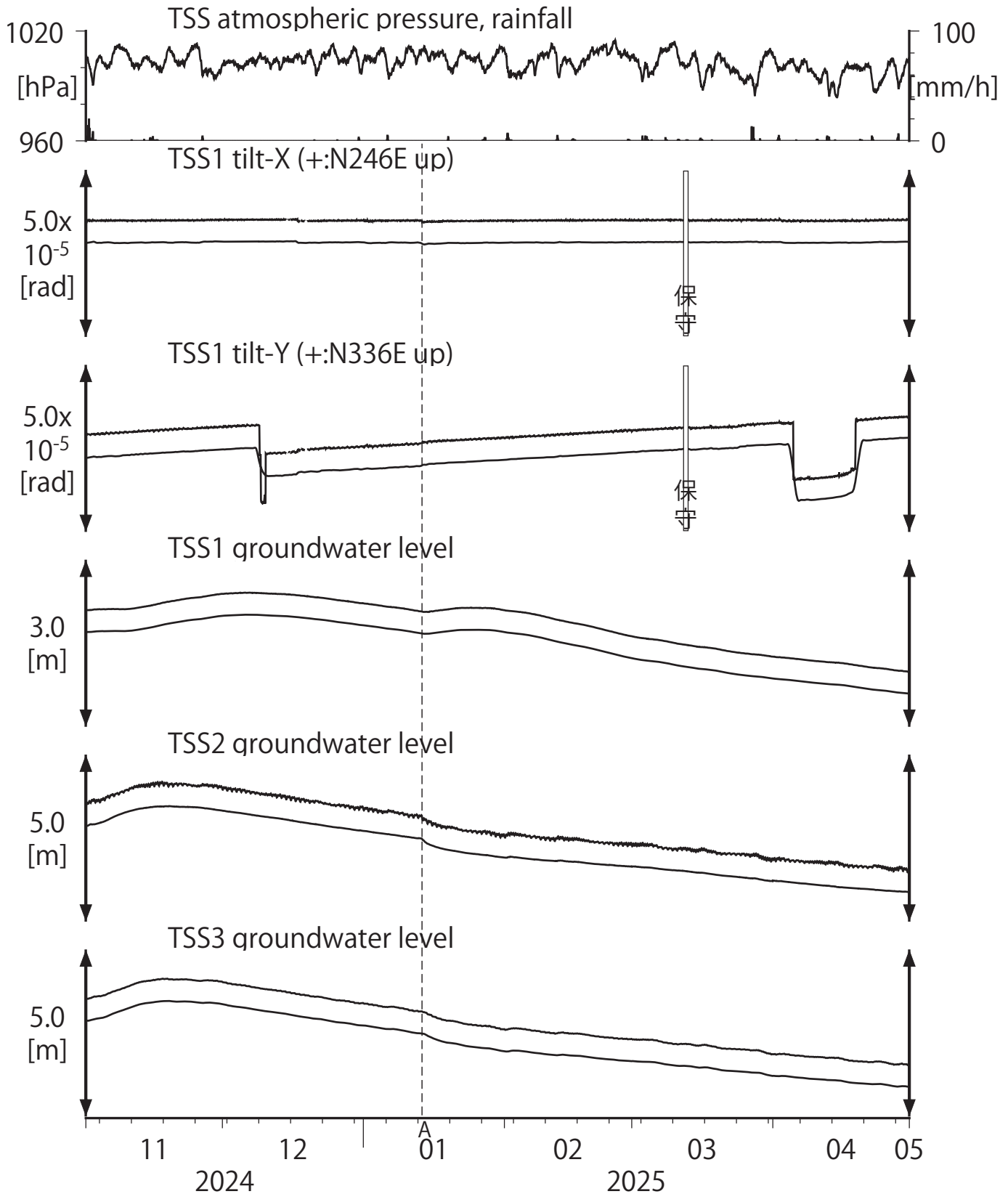
第27図 Tilt and groundwater level at TSS (時間値) (2024/11/01 00:00 - 2025/05/01 00:00 (JST))
