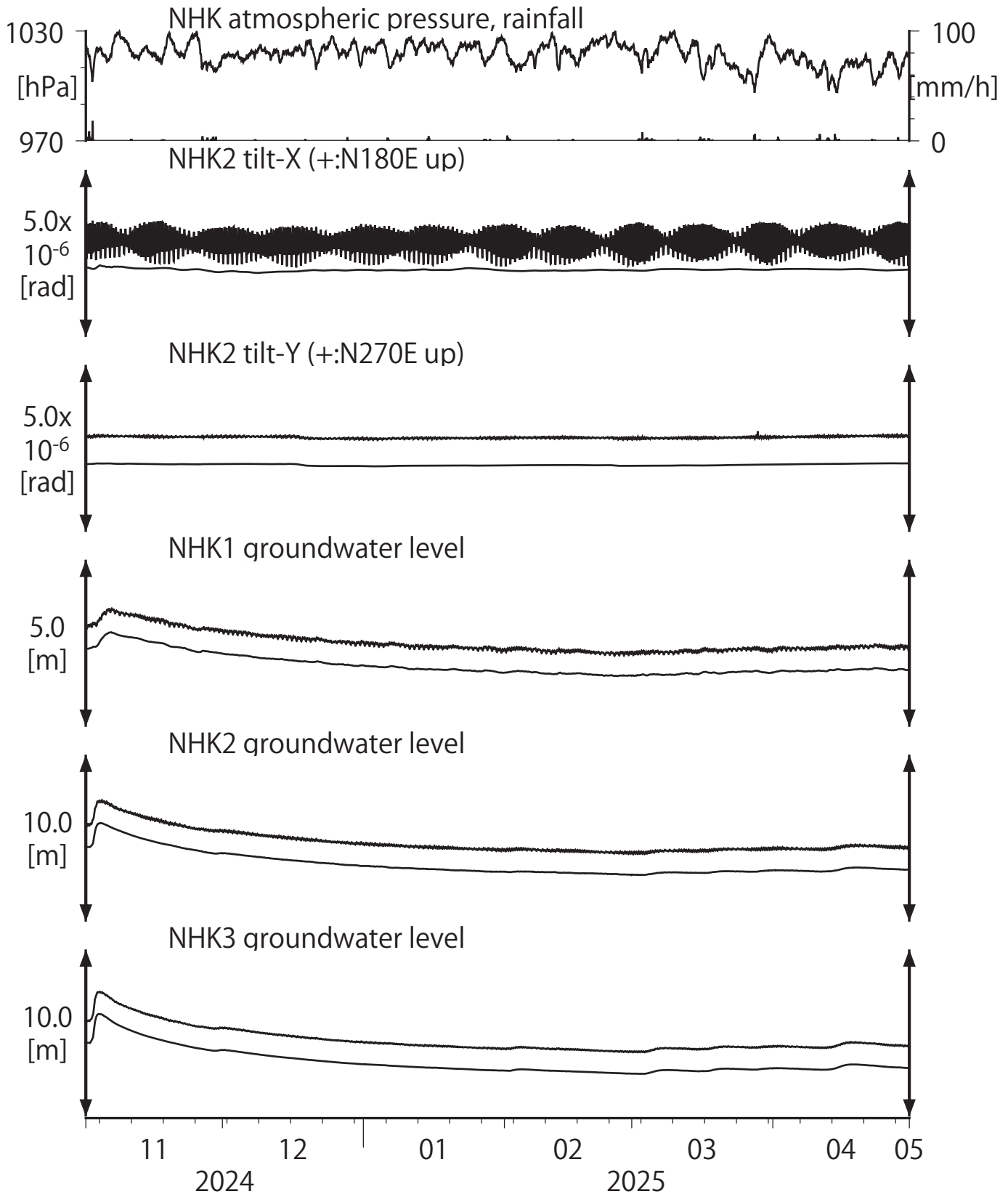
第32図 Tilt and groundwater level at NHK (時間値) (2024/11/01 00:00 - 2025/05/01 00:00 (JST))
