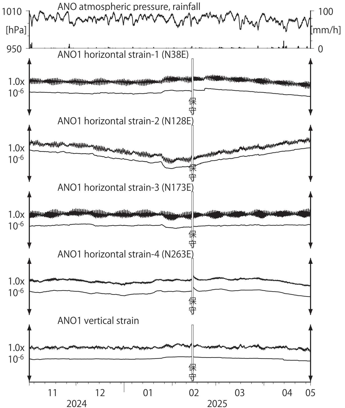
第8図 Crustal strains at ANO (時間値) (2024/11/01 00:00 - 2025/05/01 00:00 (JST))
