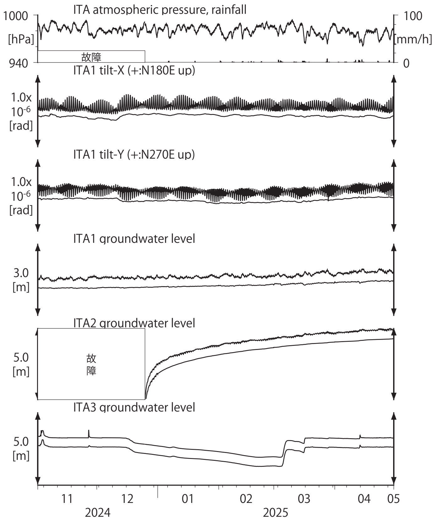
第10図 Tilt and groundwater level at ITA (時間値) (2024/11/01 00:00 - 2025/05/01 00:00 (JST))
