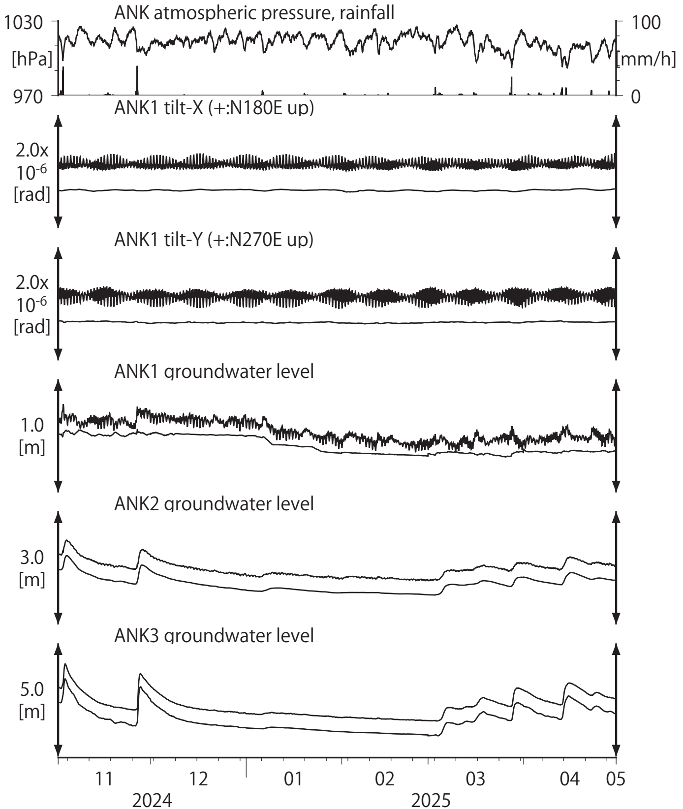
第20図 Tilt and groundwater level at ANK (時間値) (2024/11/01 00:00 - 2025/05/01 00:00 (JST))
