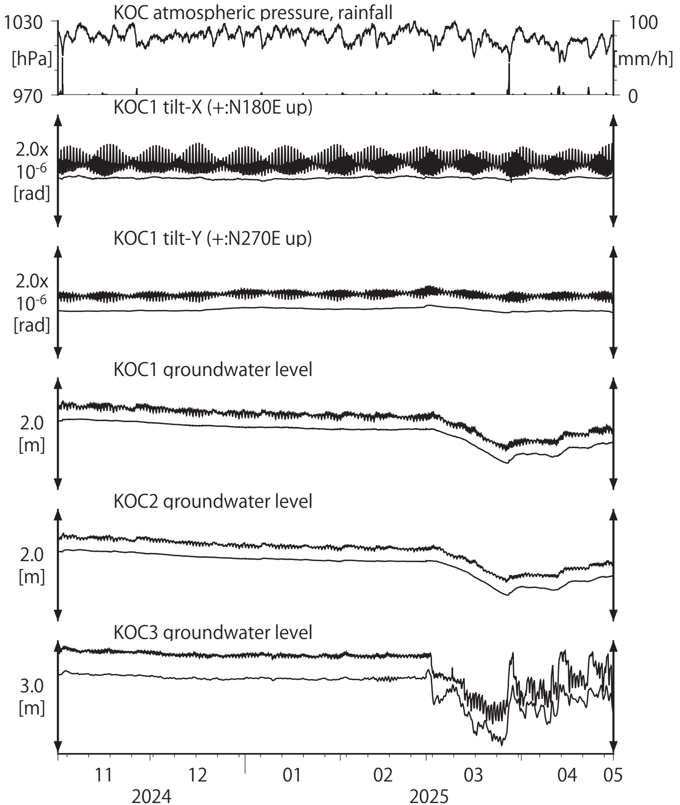
第23図 Tilt and groundwater level at KOC (時間値) (2024/11/01 00:00 - 2025/05/01 00:00 (JST))
