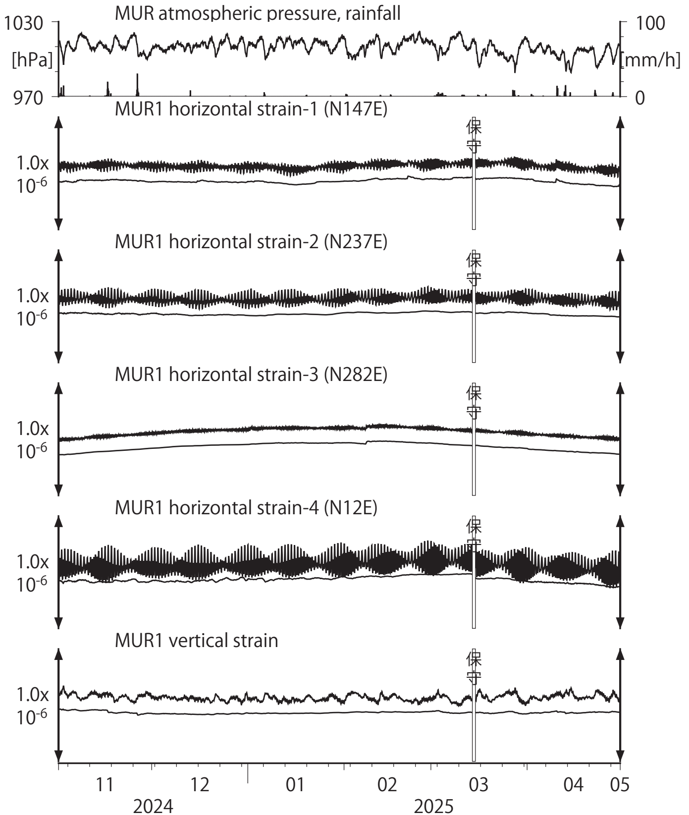
第21図 Crustal strains at MUR (時間値) (2024/11/01 00:00 - 2025/05/01 00:00 (JST))
