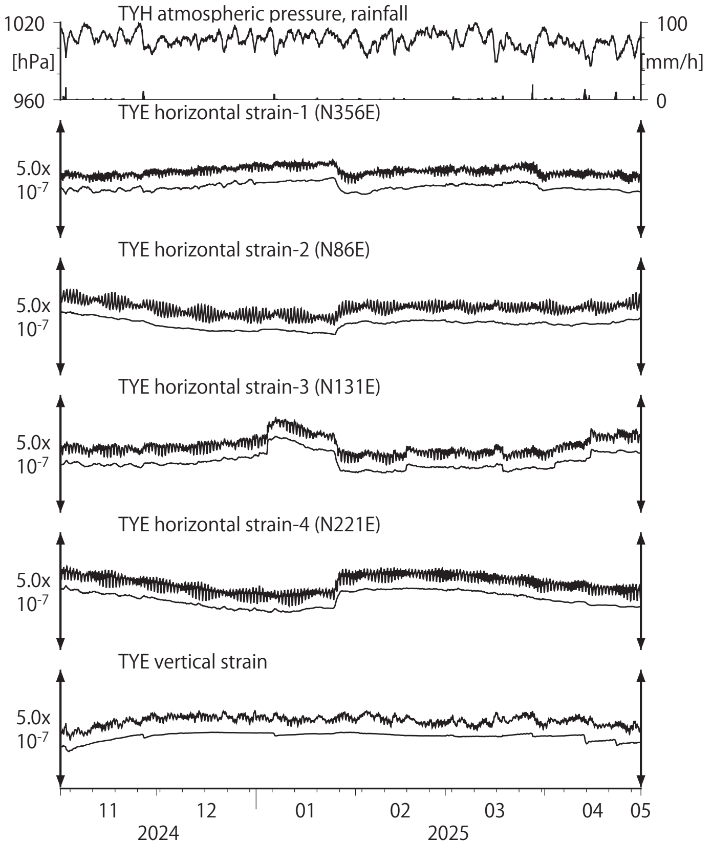
第6図 Crustal strain at TYE (時間値) (2024/11/01 00:00 - 2025/05/01 00:00 (JST))
