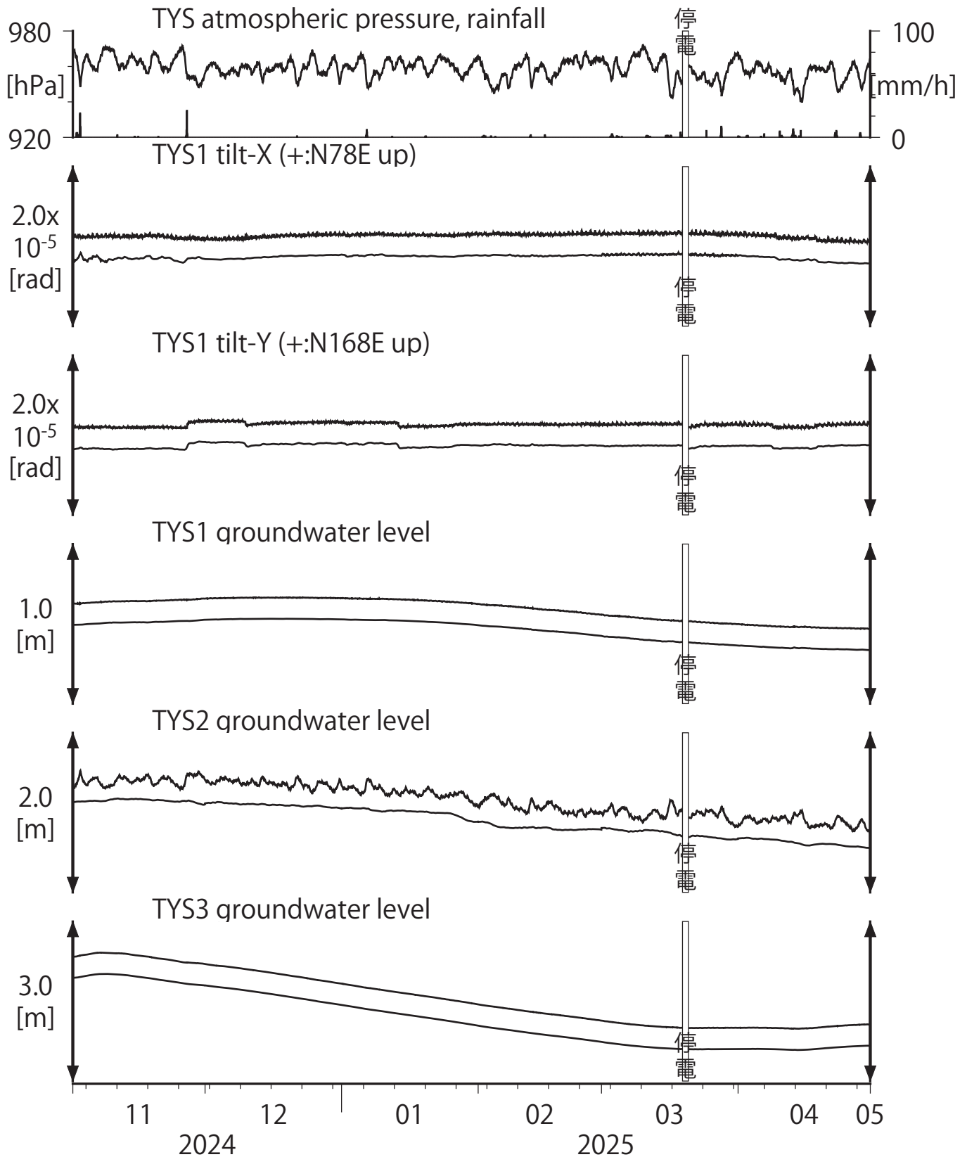
第3図 Tilt and groundwater level at TYS (時間値) (2024/11/01 00:00 - 2025/05/01 00:00 (JST))
