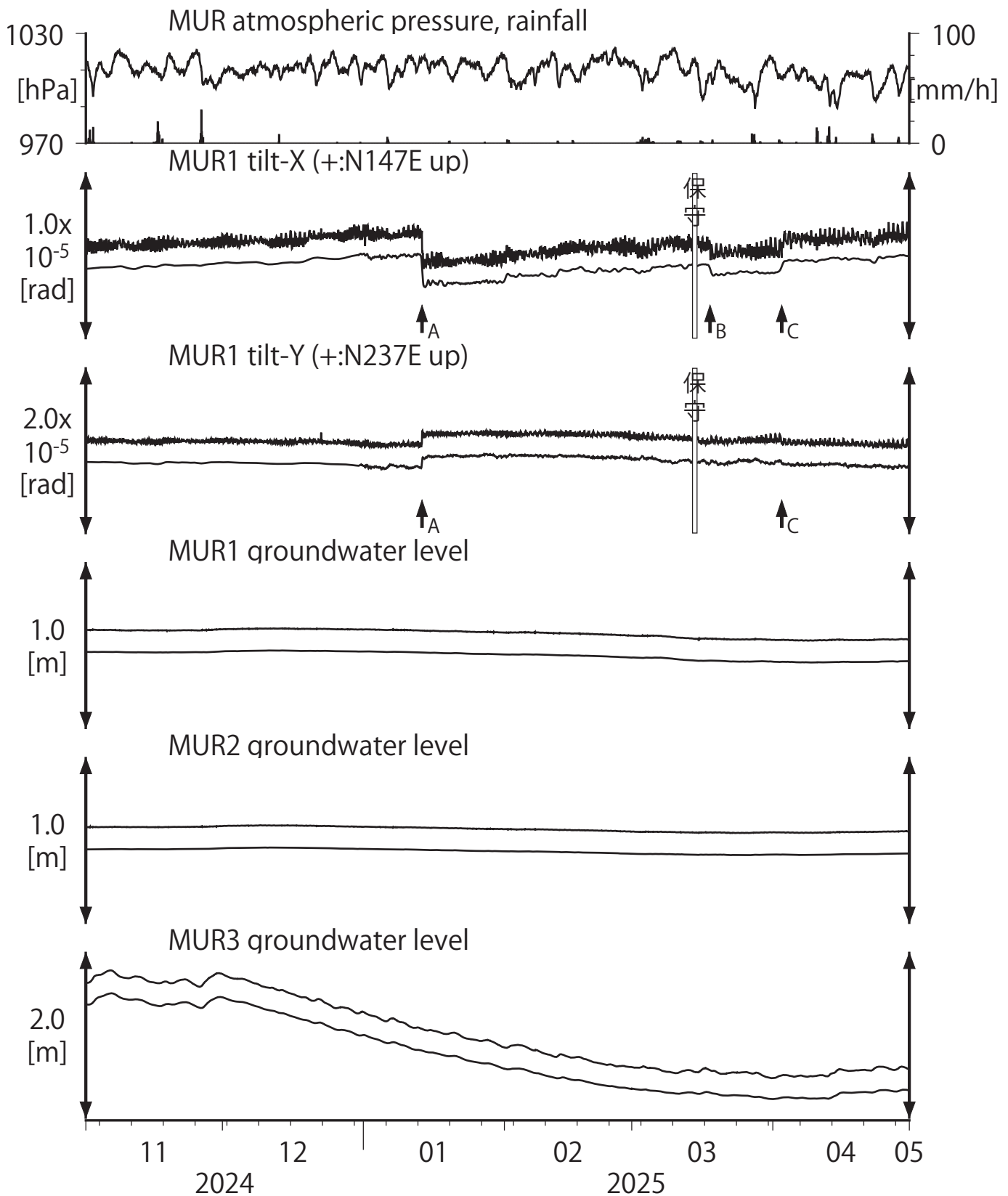
第22図 Tilt and groundwater level at MUR (時間値) (2024/11/01 00:00 - 2025/05/01 00:00 (JST))
