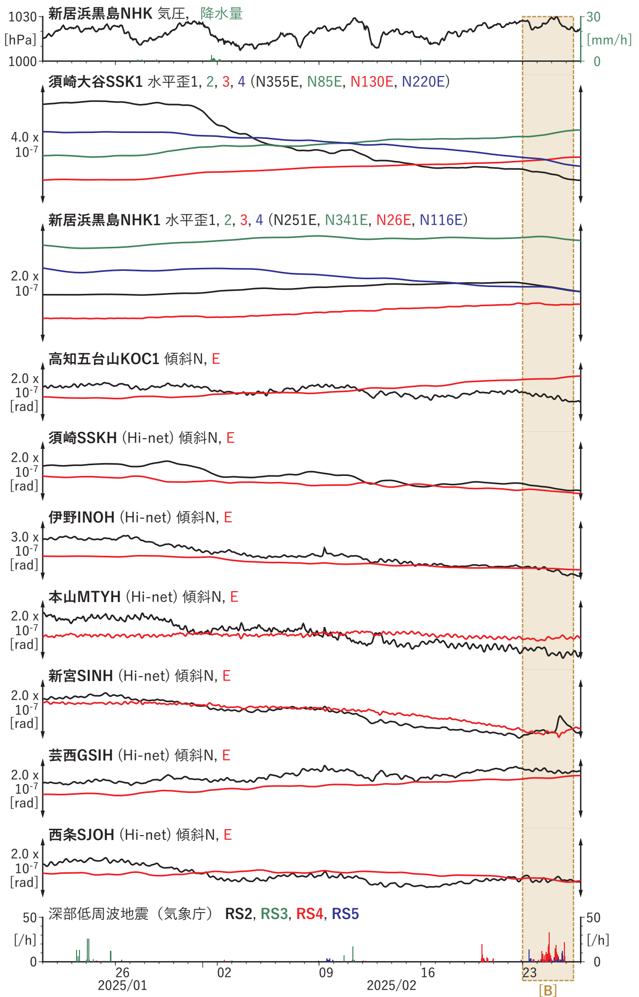
第35図 四国地方中部における歪・傾斜の時間変化 (2025/01/21 00:00 - 2025/02/27 00:00 (JST))
