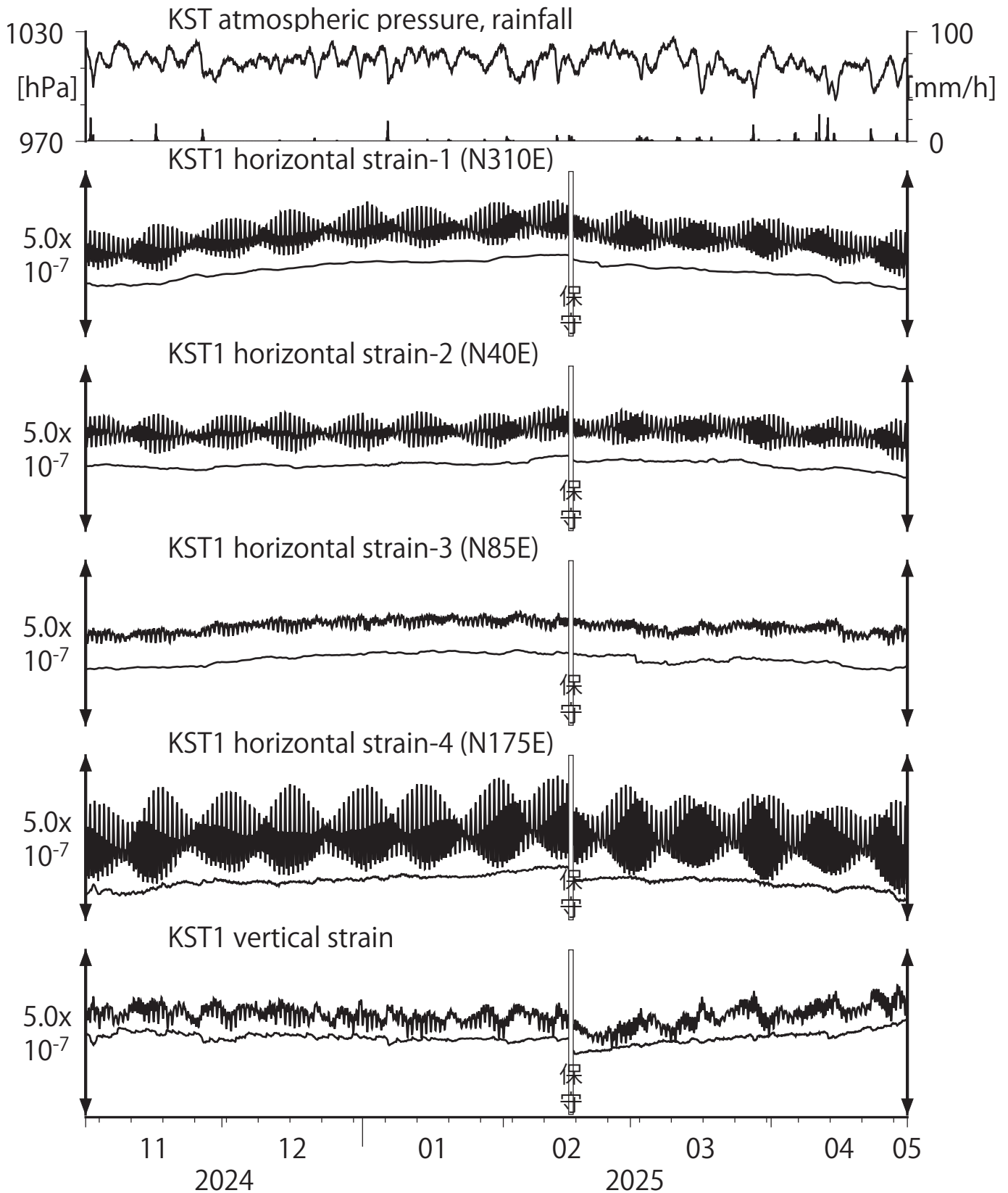
第17図 Crustal strains at KST (時間値) (2024/11/01 00:00 - 2025/05/01 00:00 (JST))
