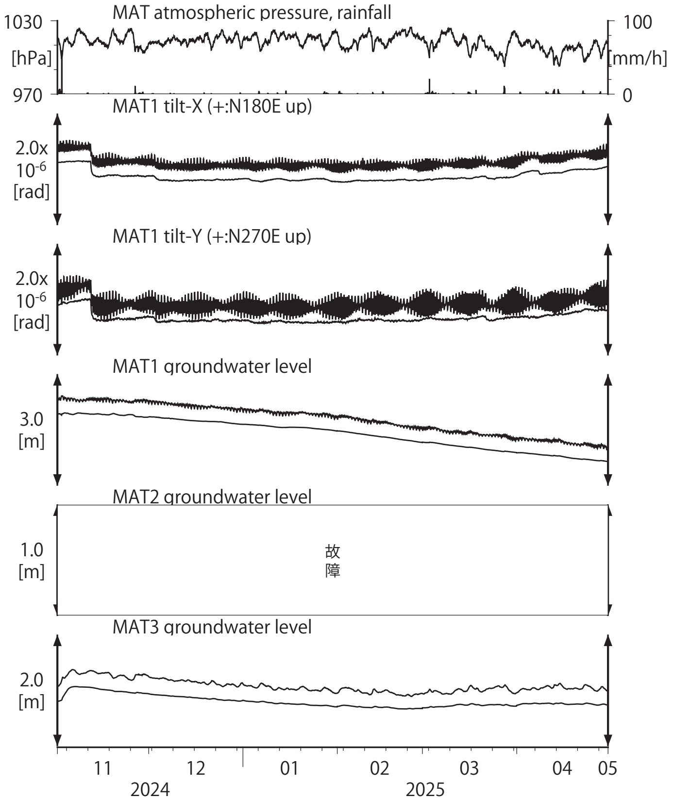
第30図 Tilt and groundwater level at MAT (時間値) (2024/11/01 00:00 - 2025/05/01 00:00 (JST))
