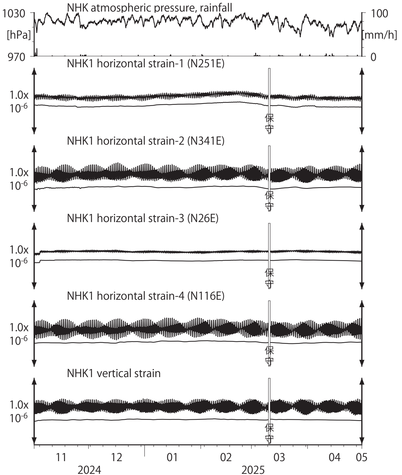
第31図 Crustal strains at NHK (時間値) (2024/11/01 00:00 - 2025/05/01 00:00 (JST))
