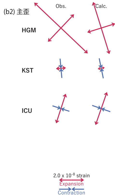
第43図 2025/04/27 - 28 の歪・傾斜変化（第42図 [A]）を説明する断層モデル。
