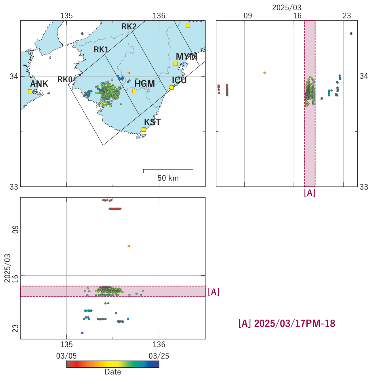
第38図 紀伊半島における深部低周波地震の時空間分布図。 (2025/03/05 00:00 - 2025/03/25 00:00 (JST)) 気象庁カタログによる。
