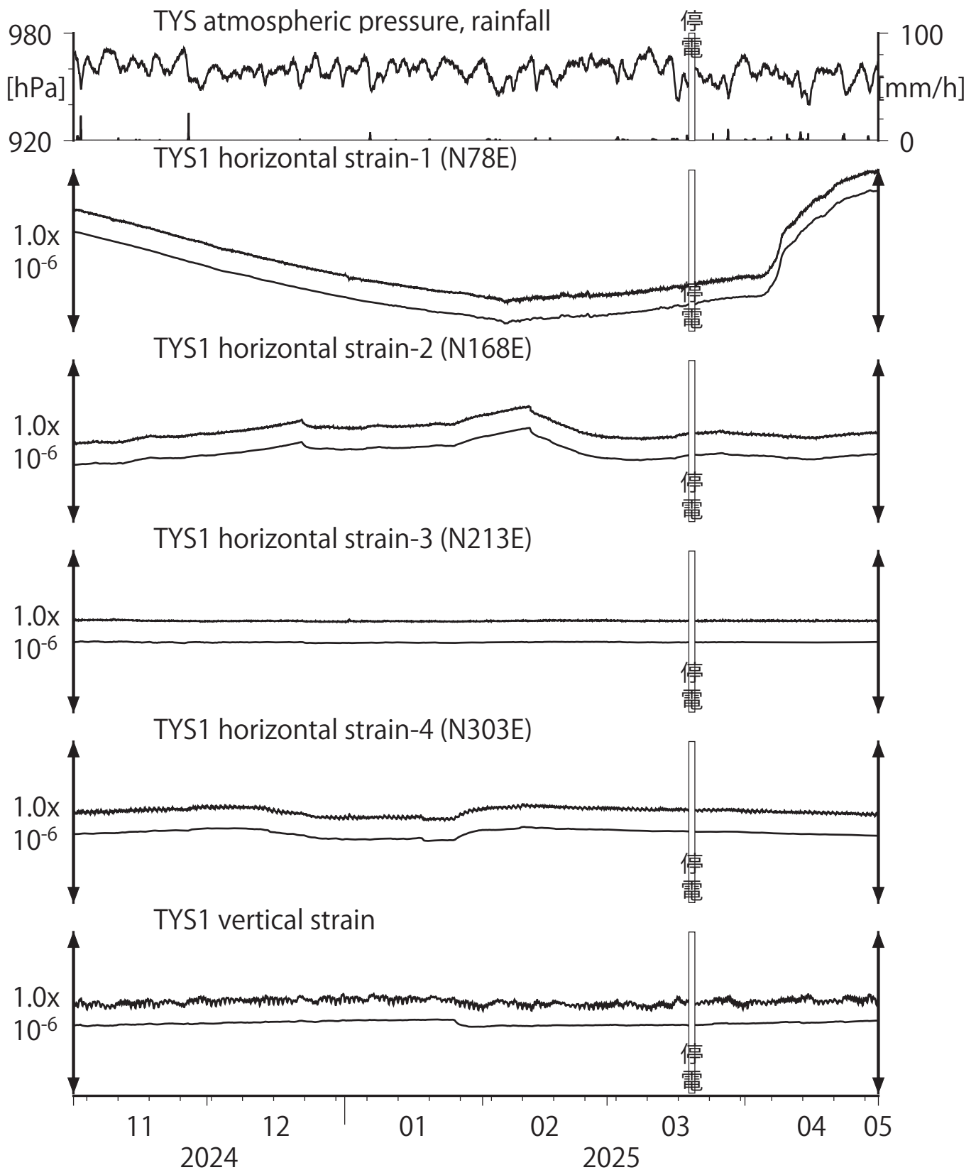
第2図 Crustal strains at TYS (時間値) (2024/11/01 00:00 - 2025/05/01 00:00 (JST))
