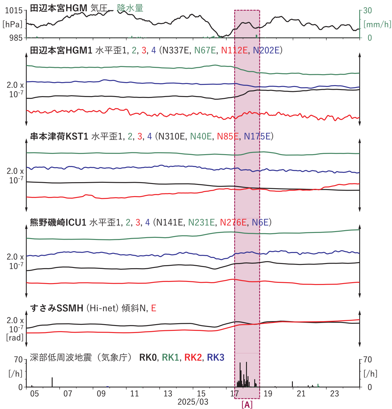
第39図 紀伊半島における歪・傾斜の時間変化 (2025/03/05 00:00 - 2025/03/25 00:00 (JST))
