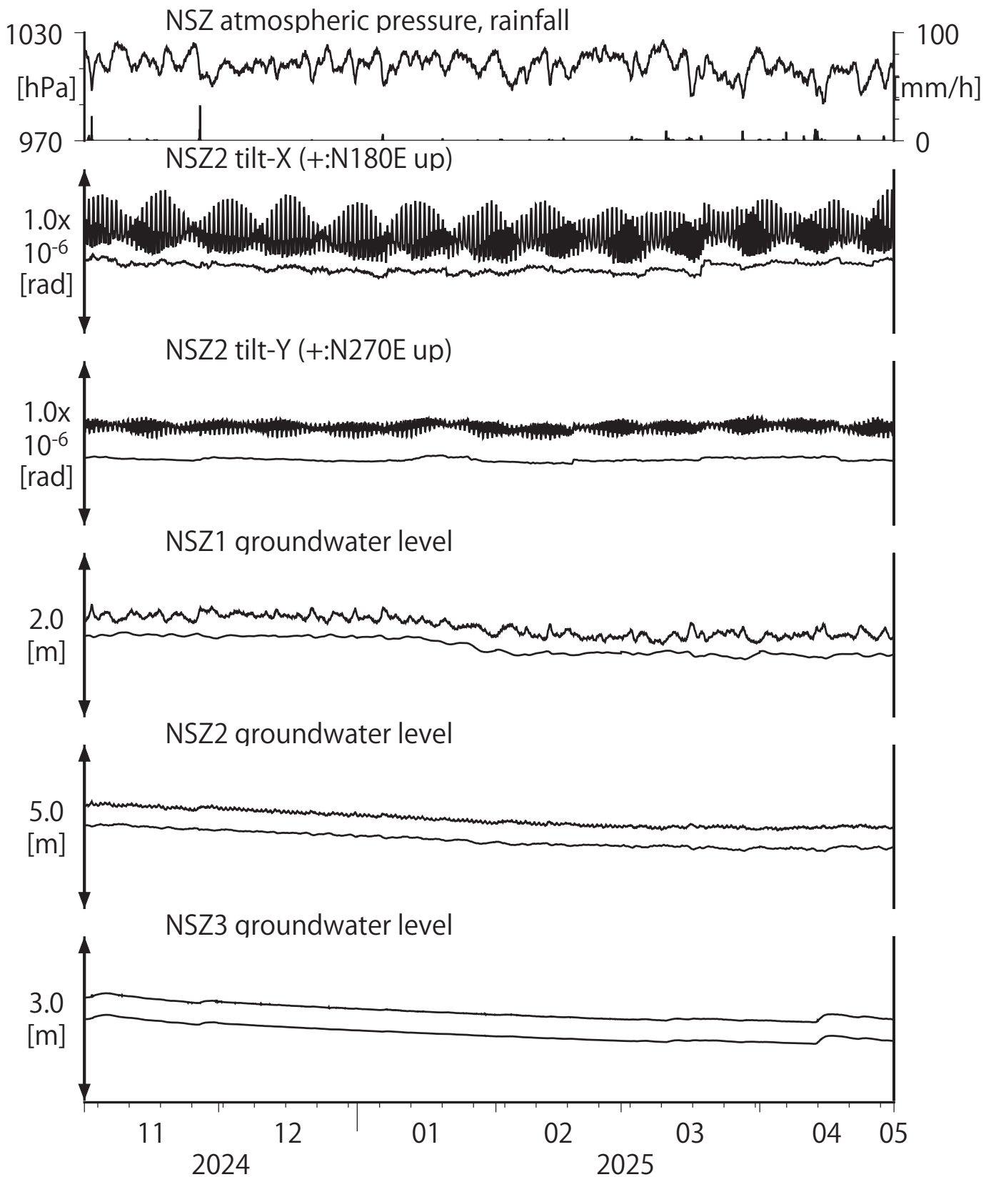
第5図 Tilt and groundwater level at NSZ (時間値) (2024/11/01 00:00 - 2025/05/01 00:00 (JST))
