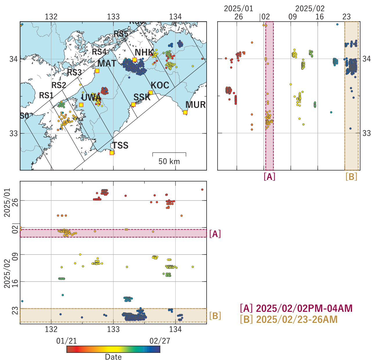
第33図 四国地方における深部低周波地震の時空間分布図。 (2025/01/21 00:00 - 2025/02/27 00:00 (JST)) 気象庁カタログによる。
