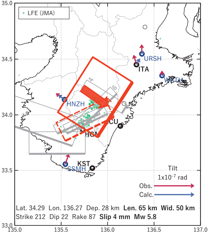
第44図 2025/04/29-30AM の歪・傾斜変化（第42図 [B]）を説明する断層モデル。 (a) プレート境界面に沿って分布させた20×20kmの矩形断層面を移動させ、各位置で残差の総和を最小とするすべり量を選んだ時の残差の総和の分布。赤色矩形が残差の総和が最小となる断層面の位置。 (b1) (a)の位置付近をグリッドサーチして推定した断層面（赤色矩形）と断層パラメータ。灰色矩形は最近周辺で発生したイベントの推定断層面。 1: 2025/03/17PM-18 (Mw5.3), 2: 2024/09/07-09AM (Mw5.6), 3: 2024/09/21-24 (Mw5.7), 4: 2024/08/07-08 (Mw5.6), 5: 2024/05/30PM-06/01 (Mw5.7), 6: 2024/01/02PM-03AM (Mw5.7) A: 2025/04/27-28 (Mw5.8) (b2) 主歪の観測値と(b1)に示した断層モデルから求めた計算値との比較。
