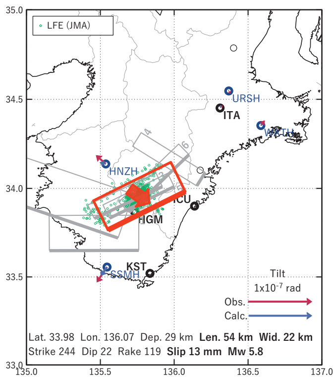
第43図 2025/04/27 - 28 の歪・傾斜変化（第42図 [A]）を説明する断層モデル。
