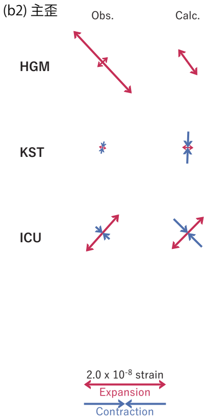
第44図 2025/04/29-30AM の歪・傾斜変化（第42図 [B]）を説明する断層モデル。 (a) プレート境界面に沿って分布させた20×20kmの矩形断層面を移動させ、各位置で残差の総和を最小とするすべり量を選んだ時の残差の総和の分布。赤色矩形が残差の総和が最小となる断層面の位置。 (b1) (a)の位置付近をグリッドサーチして推定した断層面（赤色矩形）と断層パラメータ。灰色矩形は最近周辺で発生したイベントの推定断層面。 1: 2025/03/17PM-18 (Mw5.3), 2: 2024/09/07-09AM (Mw5.6), 3: 2024/09/21-24 (Mw5.7), 4: 2024/08/07-08 (Mw5.6), 5: 2024/05/30PM-06/01 (Mw5.7), 6: 2024/01/02PM-03AM (Mw5.7) A: 2025/04/27-28 (Mw5.8) (b2) 主歪の観測値と(b1)に示した断層モデルから求めた計算値との比較。
