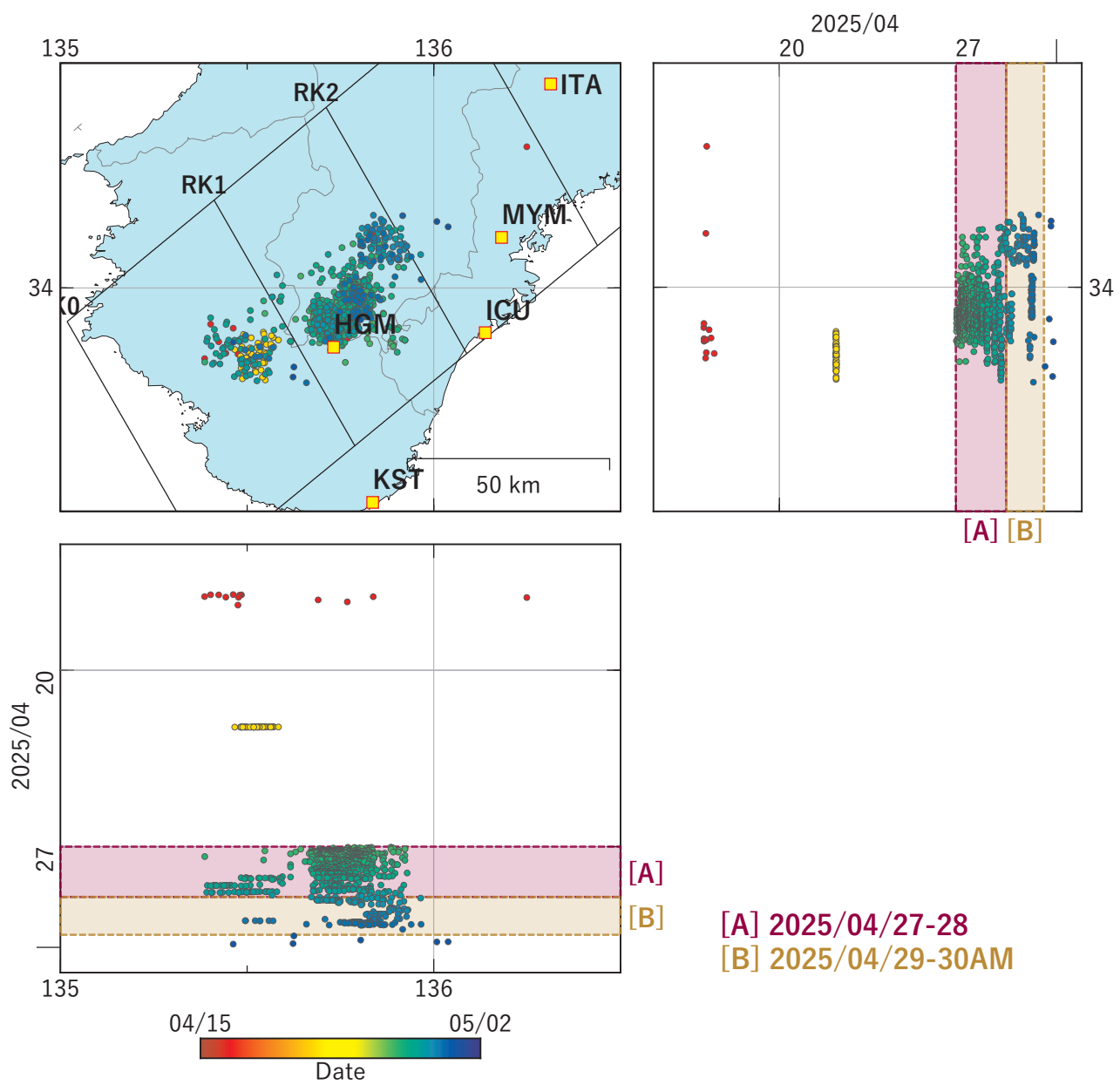
第41図 紀伊半島における深部低周波地震の時空間分布図。 (2025/04/15 00:00 - 2025/05/02 00:00 (JST)) 気象庁カタログによる。
