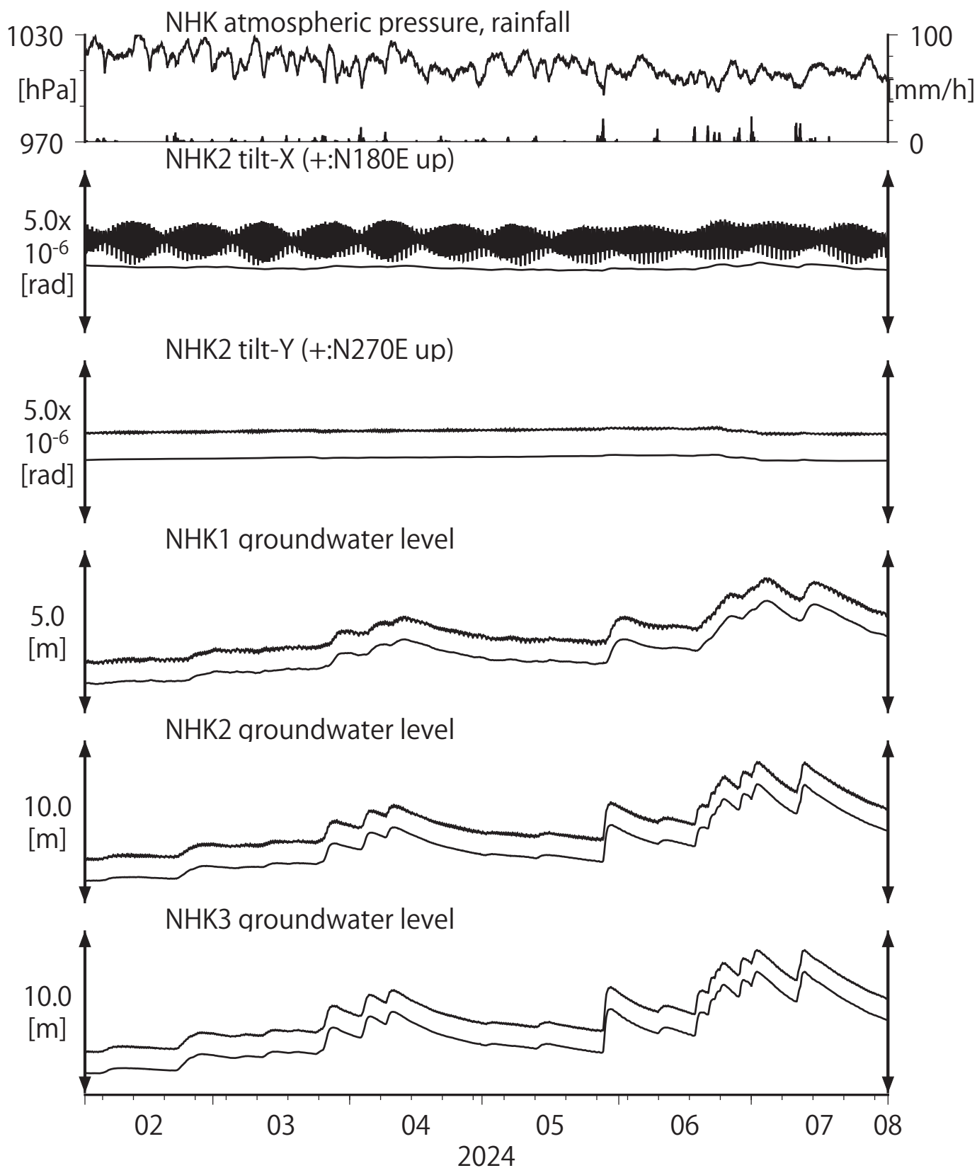
第32図 Tilt and groundwater level at NHK (時間値) (2024/02/01 00:00 - 2024/08/01 00:00 (JST))
