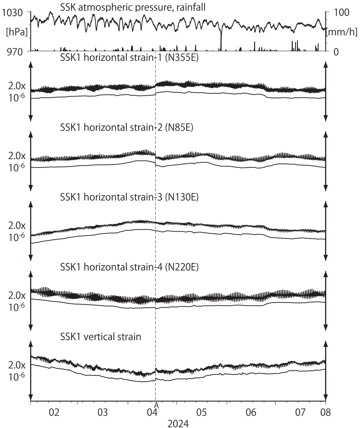
第24図 Crustal strains at SSK (時間値) (2024/02/01 00:00 - 2024/08/01 00:00 (JST))
