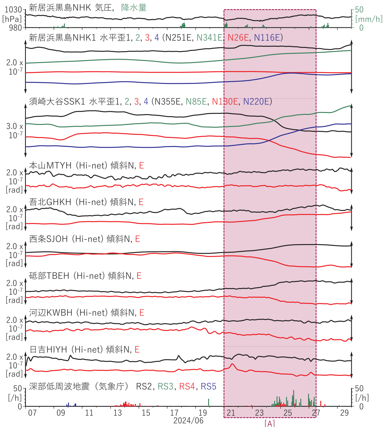
第44図 四国における歪・傾斜観測結果 (2024/06/02 00:00 - 2024/06/31 00:00 (JST))
