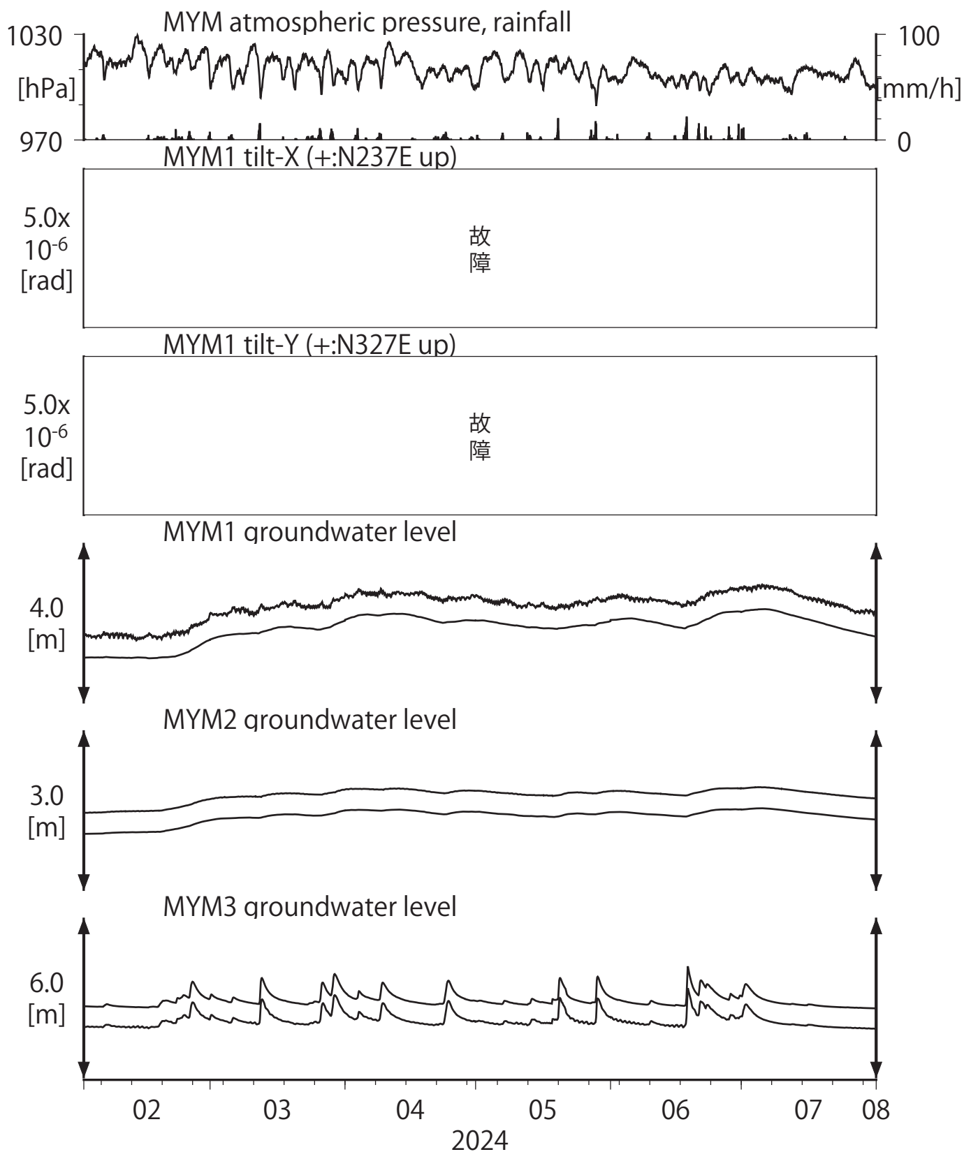
第12図 Tilt and groundwater level at MYM (時間値) (2024/02/01 00:00 - 2024/08/01 00:00 (JST))
