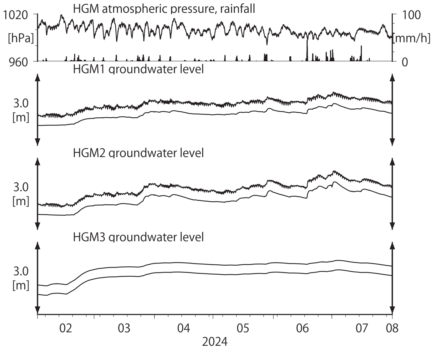
第16図 Tilt and groundwater level at HGM (時間値) (2024/02/01 00:00 - 2024/08/01 00:00 (JST))
