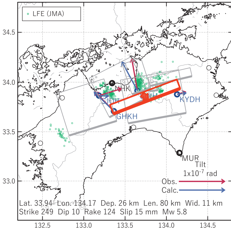
第48図 2024/07/04-06の歪・傾斜変化 (第47図[A]) を説明する断層モデル。
