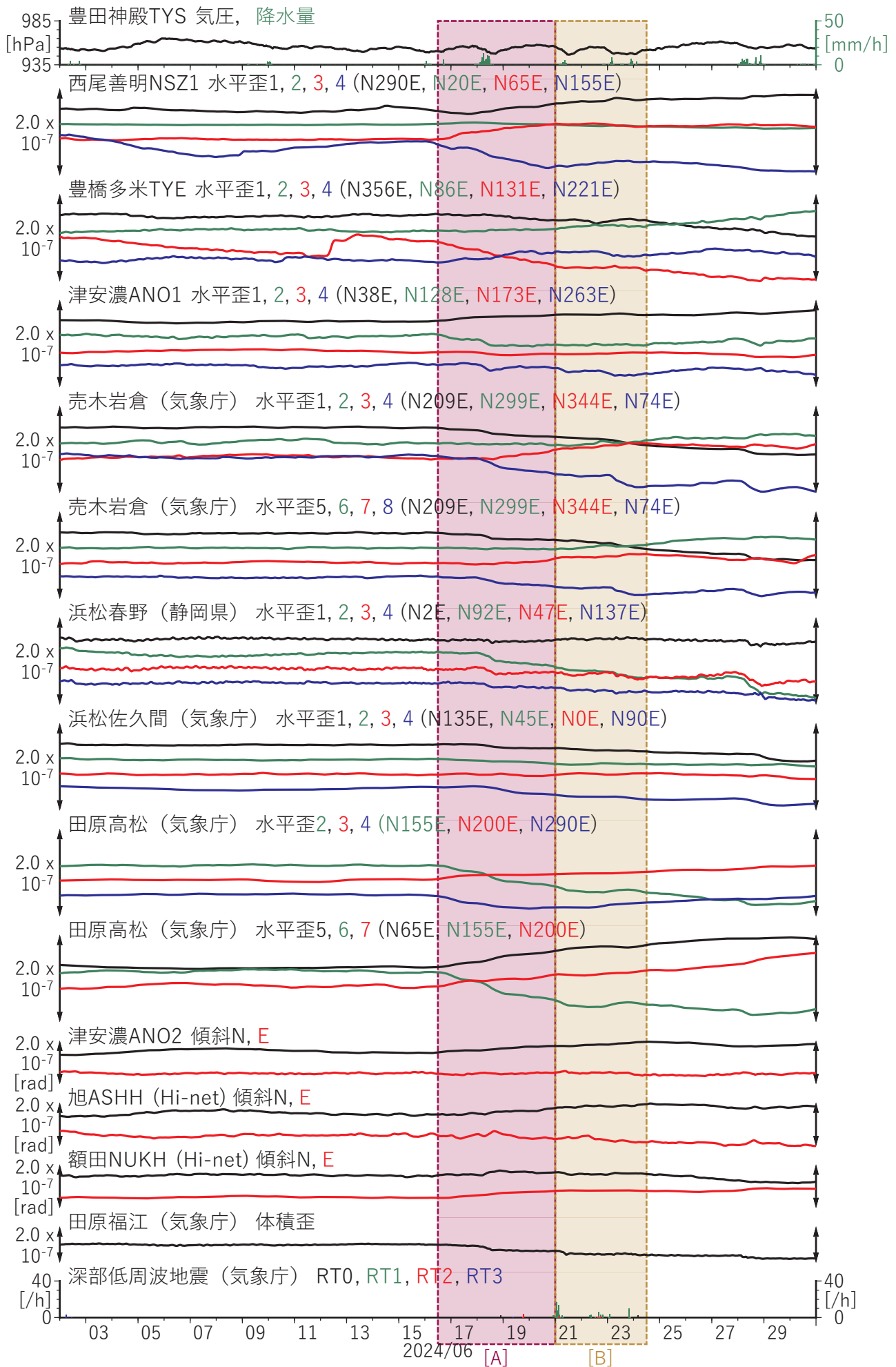
第40図 東海・紀伊半島における歪・傾斜観測結果 (2024/06/02 00:00 - 2024/06/31 00:00 (JST))
