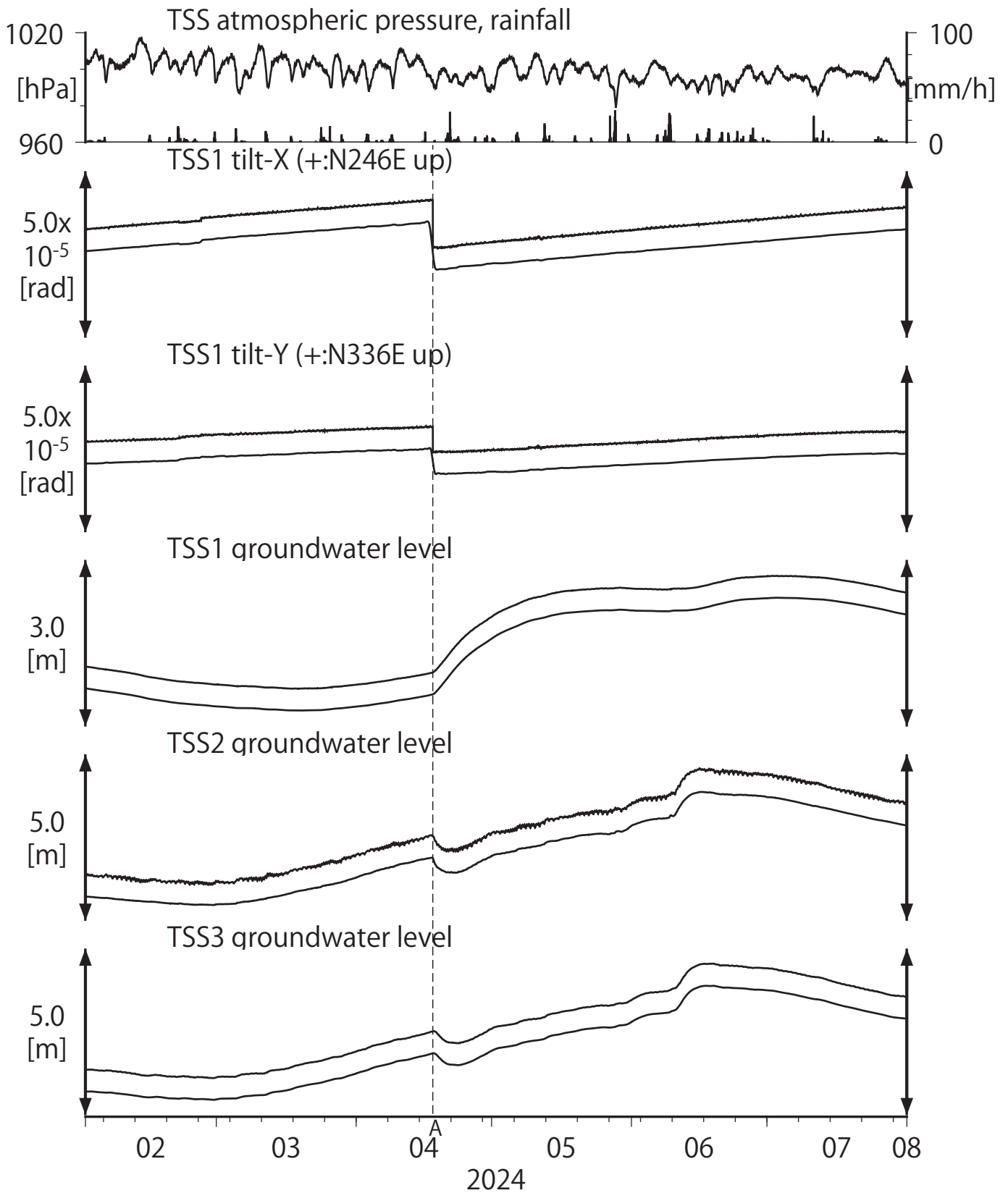
第27図 Tilt and groundwater level at TSS (時間値) (2024/02/01 00:00 - 2024/08/01 00:00 (JST))
