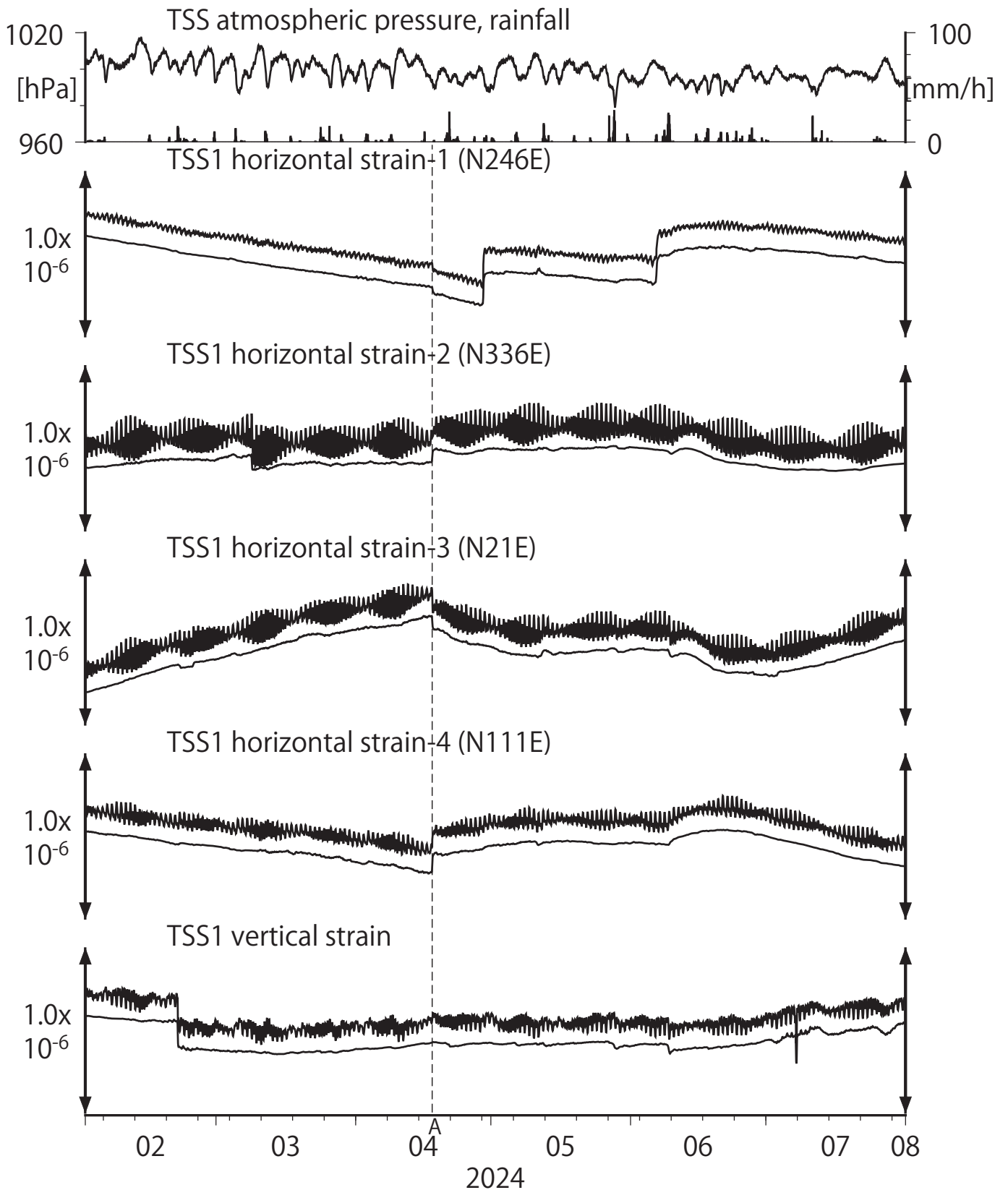
第26図 Crustal strains at TSS (時間値) (2024/02/01 00:00 - 2024/08/01 00:00 (JST))
