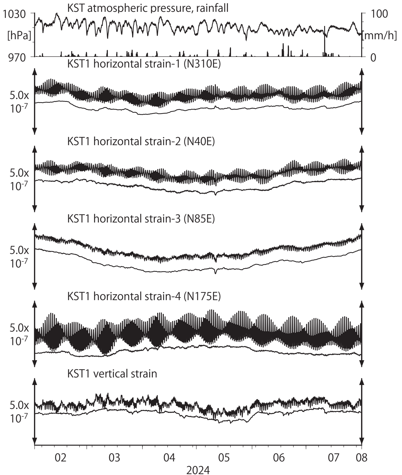
第17図 Crustal strains at KST (時間値) (2024/02/01 00:00 - 2024/08/01 00:00 (JST))
