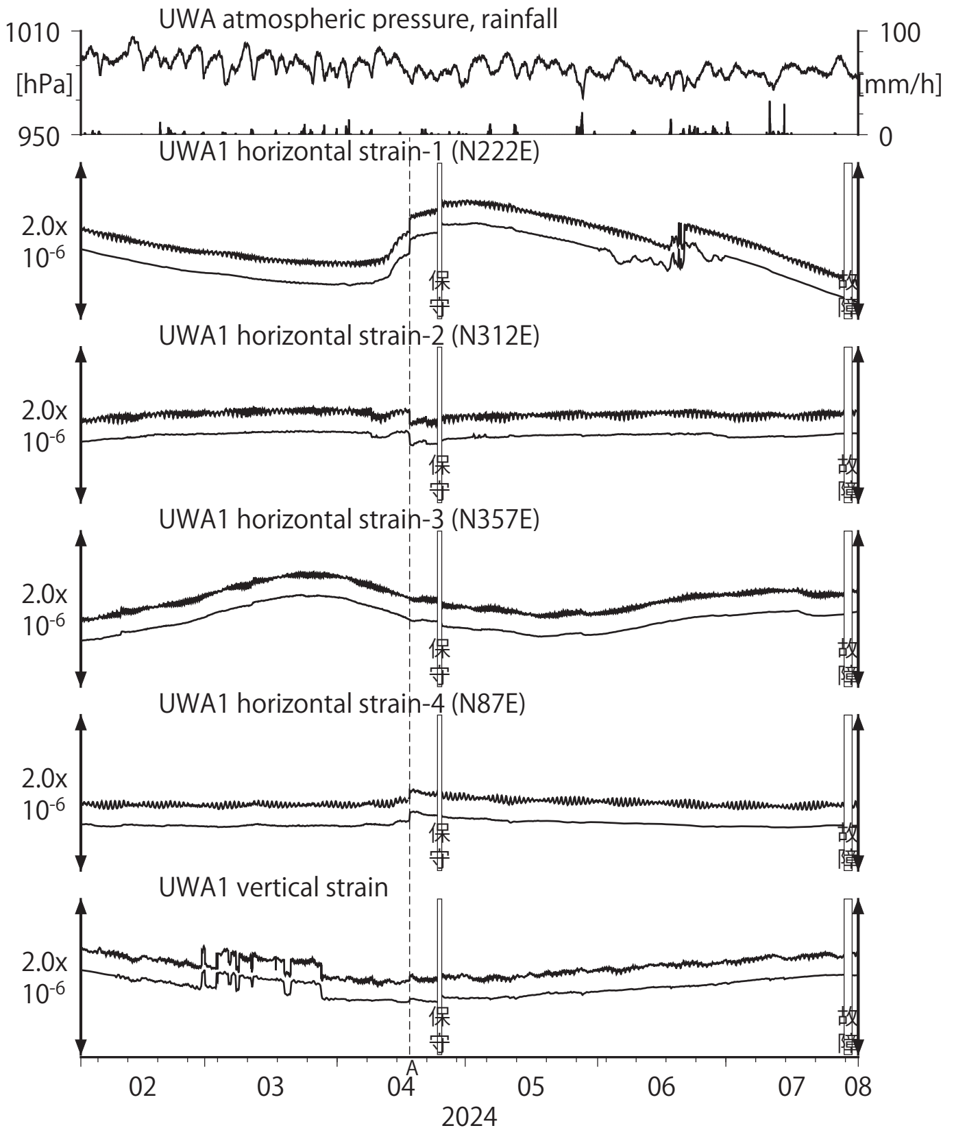
第28図 Crustal strains at UWA (時間値) (2024/02/01 00:00 - 2024/08/01 00:00 (JST))
