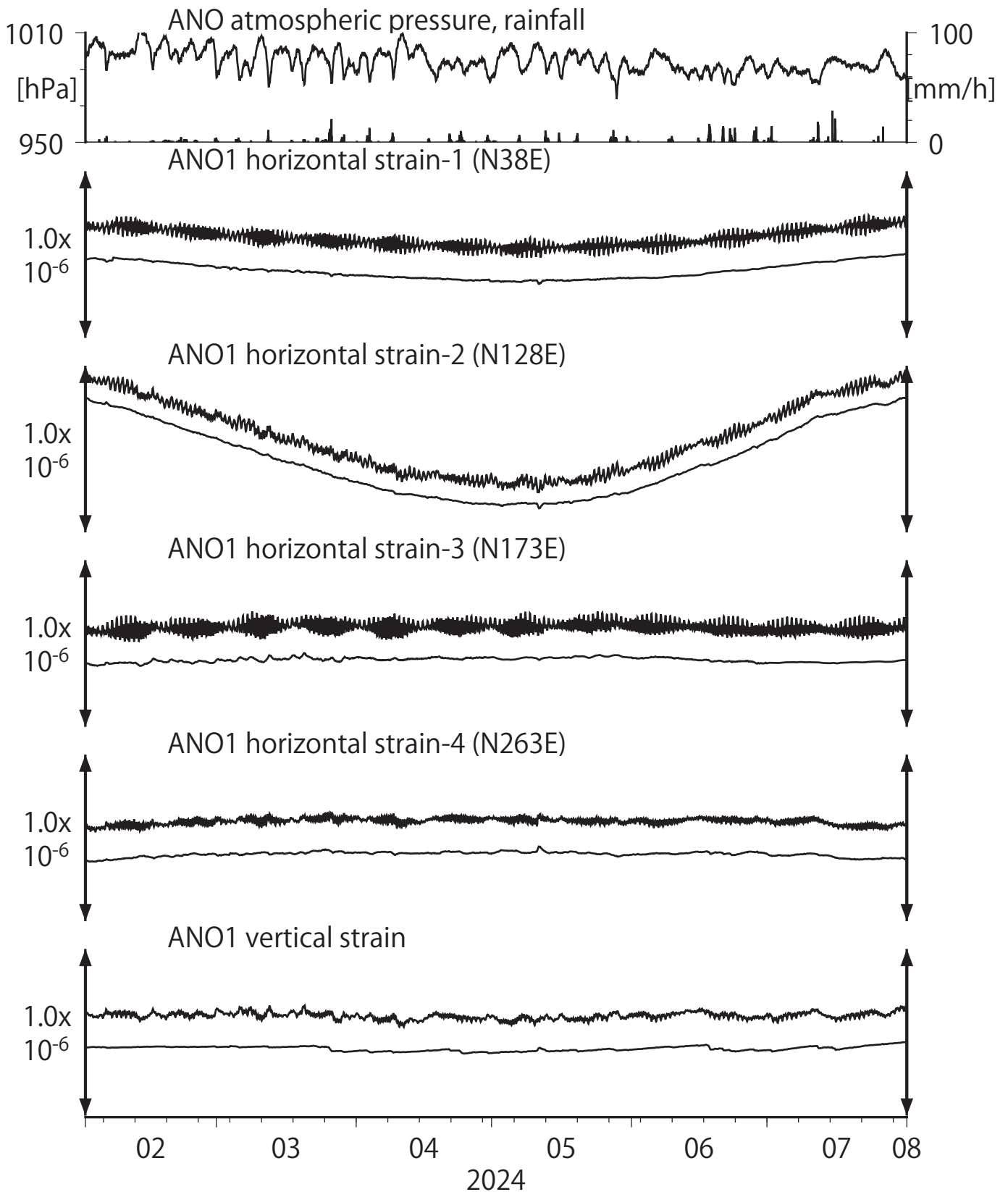
第8図 Crustal strains at ANO (時間値) (2024/02/01 00:00 - 2024/08/01 00:00 (JST))
