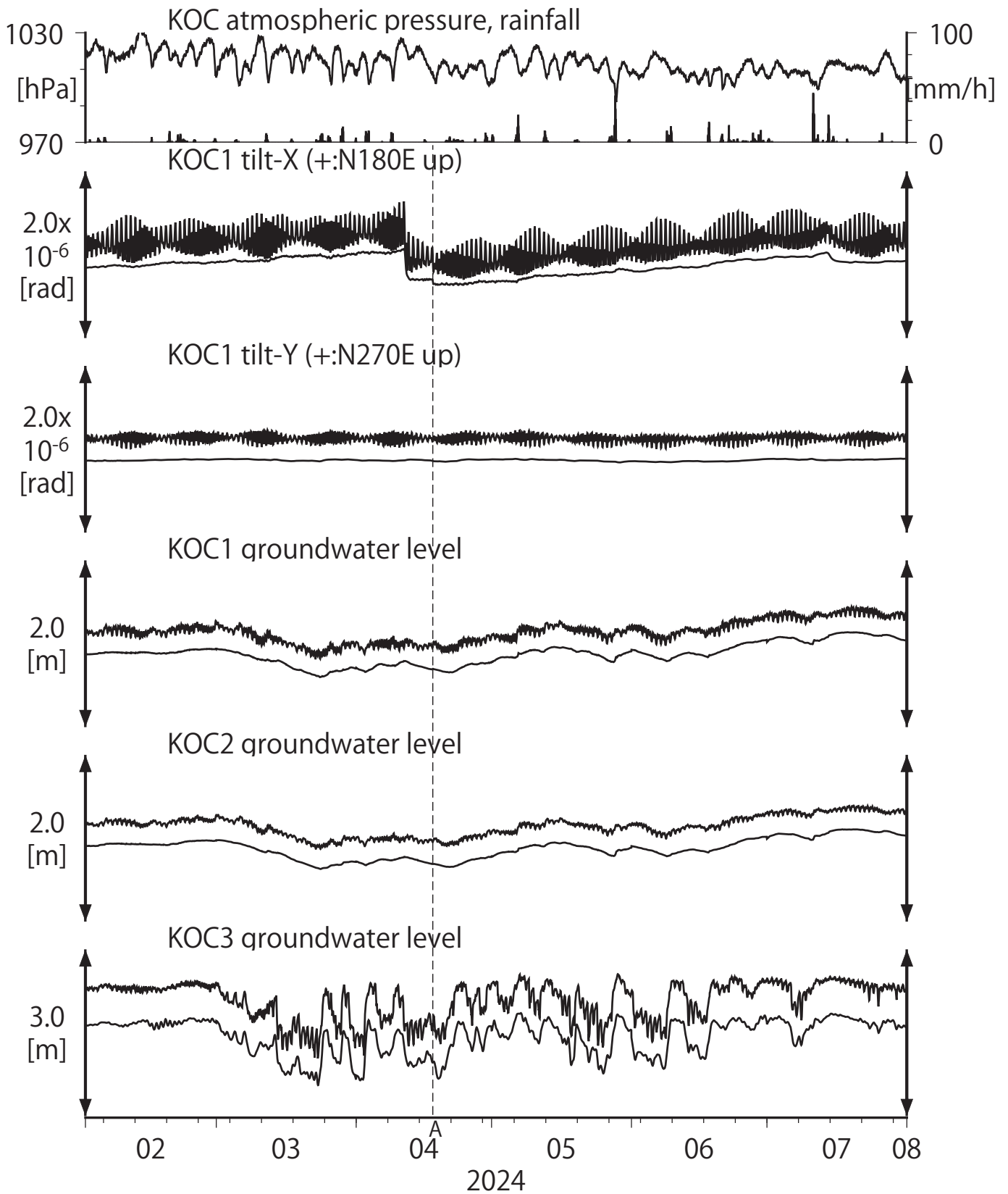
第23図 Tilt and groundwater level at KOC (時間値) (2024/02/01 00:00 - 2024/08/01 00:00 (JST))
