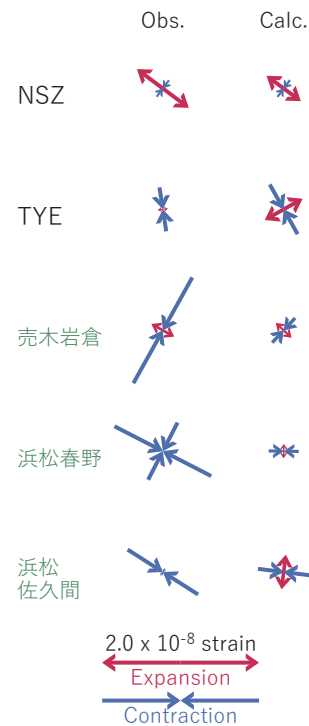
第42図 2024/06/21-24AMの歪変化 (第40図[B]) を説明する断層モデル。
