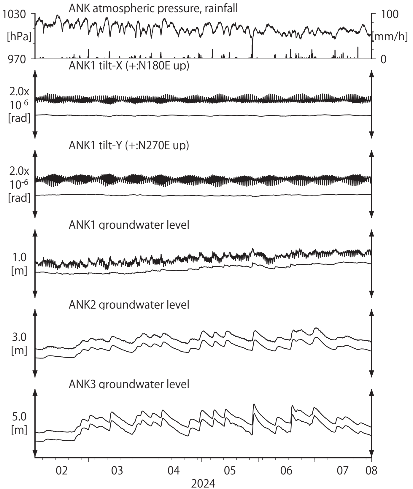
第20図 Tilt and groundwater level at ANK (時間値) (2024/02/01 00:00 - 2024/08/01 00:00 (JST))
