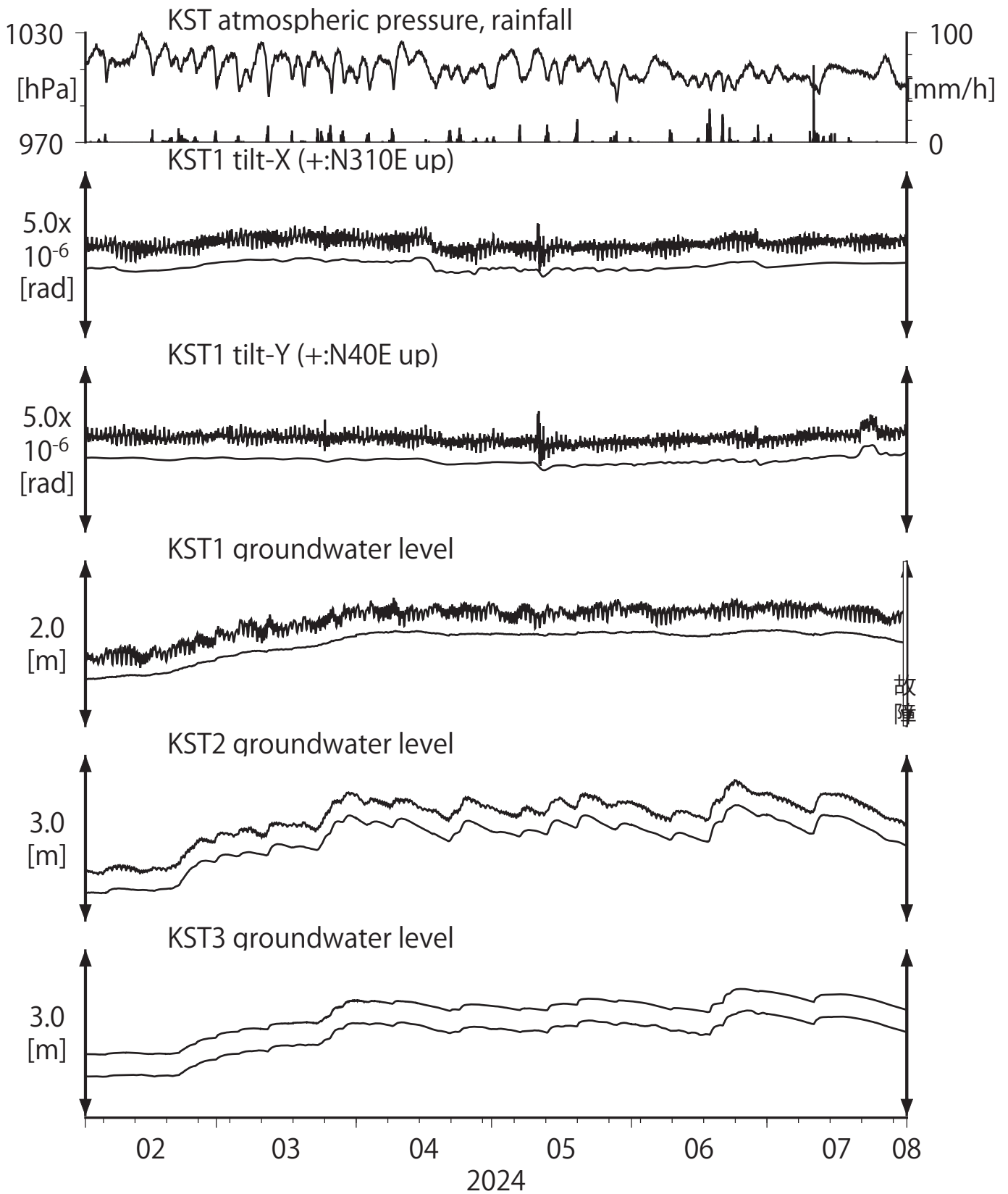
第18図 Tilt and groundwater level at KST (時間値) (2024/02/01 00:00 - 2024/08/01 00:00 (JST))
