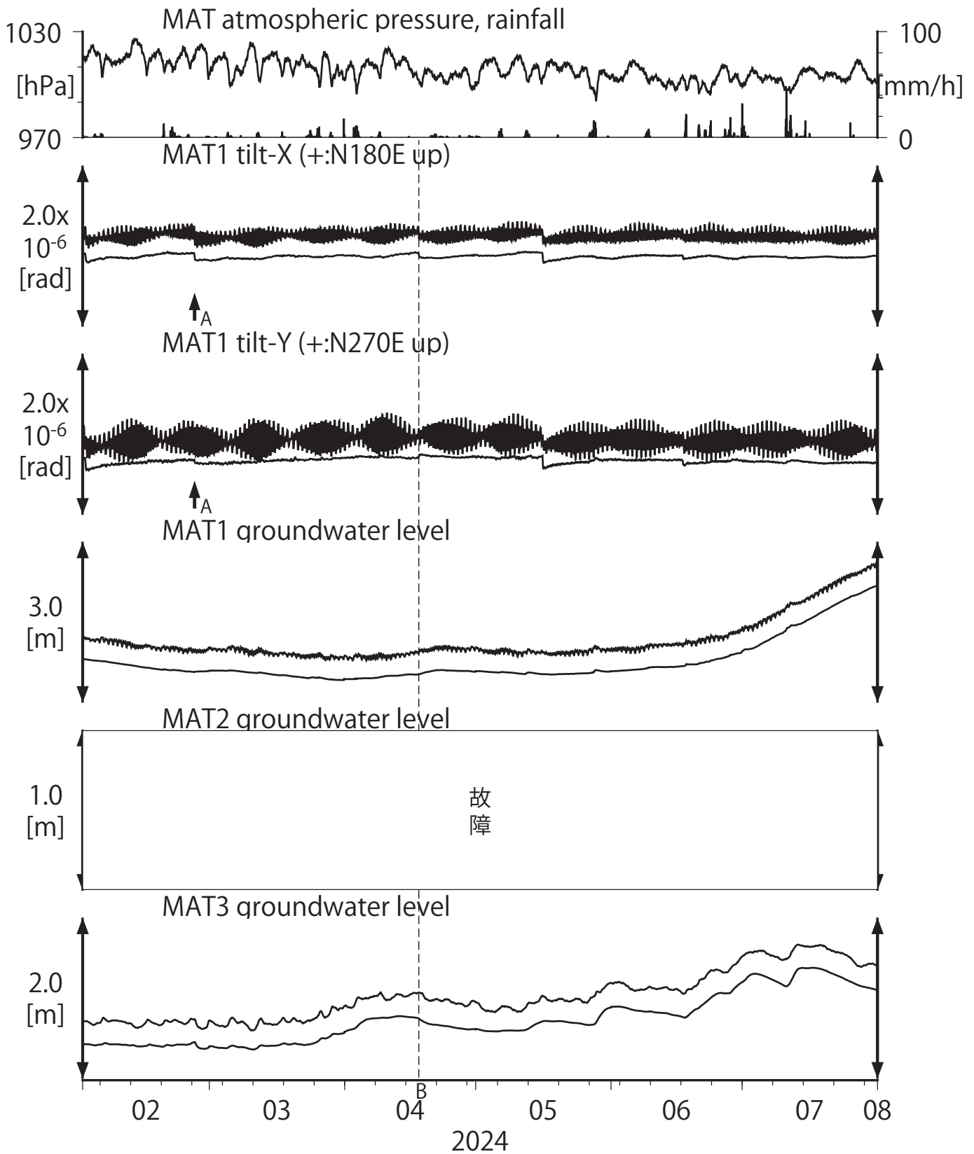
第30図 Tilt and groundwater level at MAT (時間値) (2024/02/01 00:00 - 2024/08/01 00:00 (JST))
