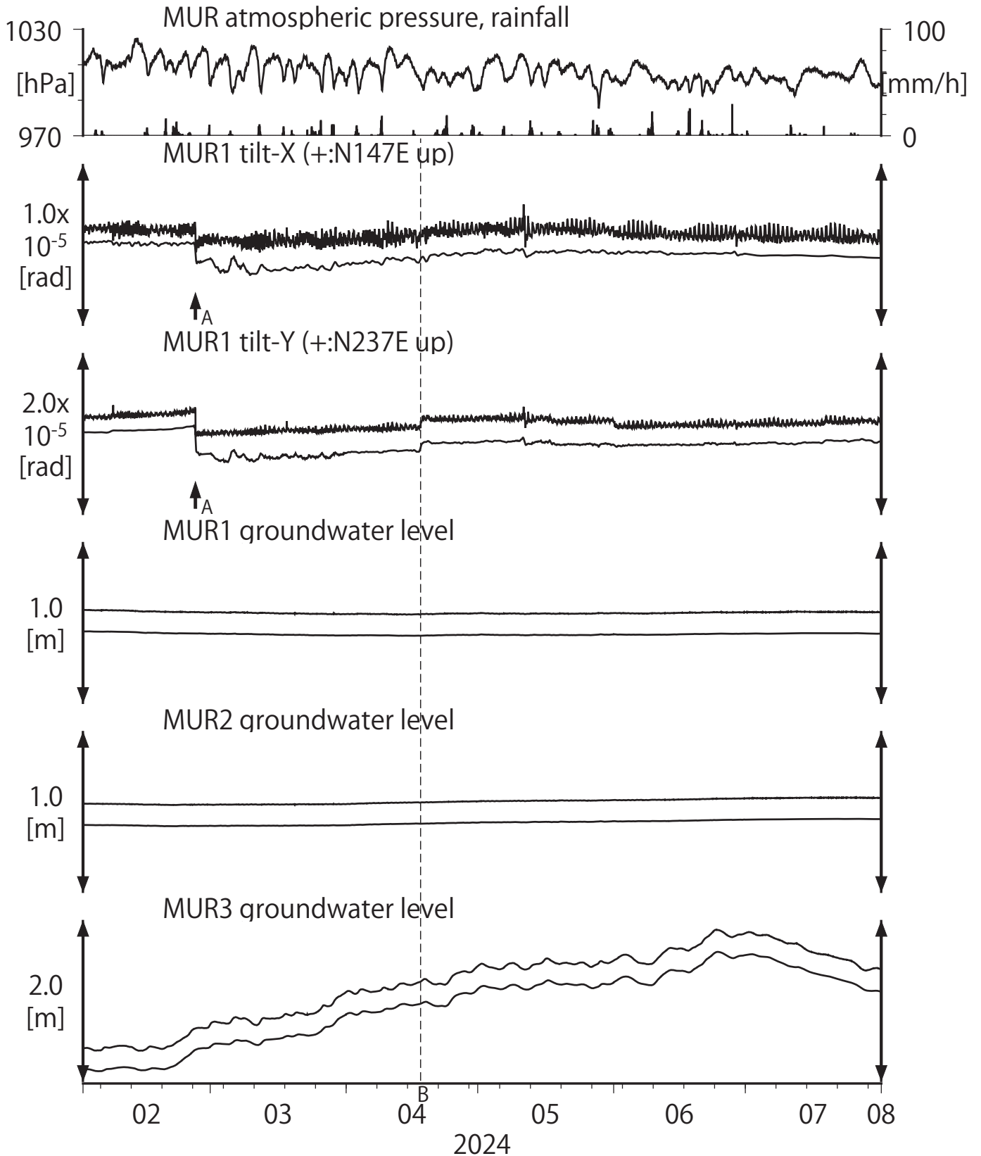
第22図 Tilt and groundwater level at MUR (時間値) (2024/02/01 00:00 - 2024/08/01 00:00 (JST))
