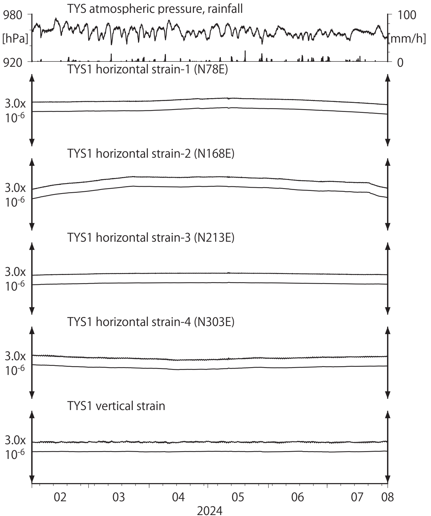
第2図 Crustal strains at TYS (時間値) (2024/02/01 00:00 - 2024/08/01 00:00 (JST))
