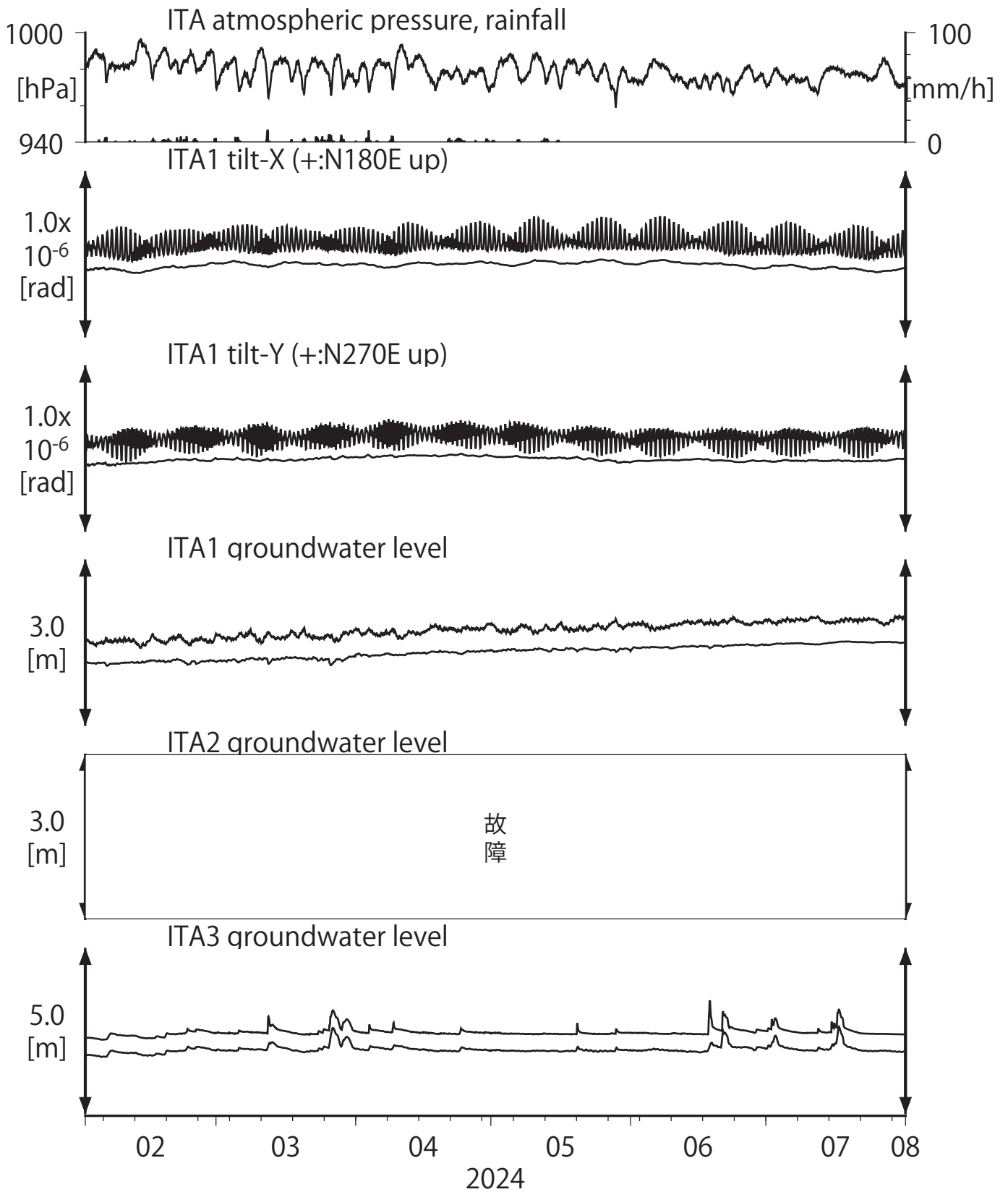
第10図 Tilt and groundwater level at ITA (時間値) (2024/02/01 00:00 - 2024/08/01 00:00 (JST))
