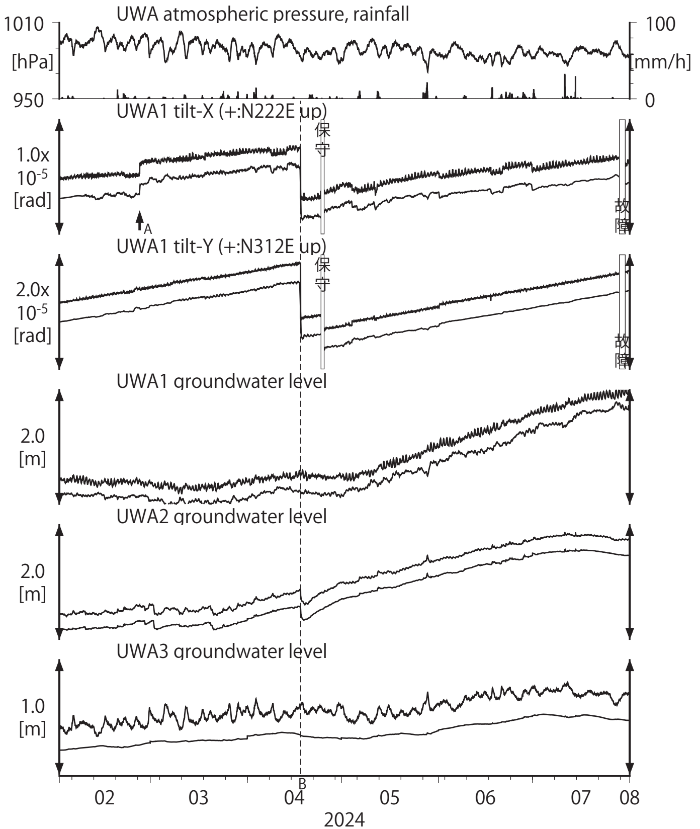
第29図 Tilt and groundwater level at UWA (時間値) (2024/02/01 00:00 - 2024/08/01 00:00 (JST))
