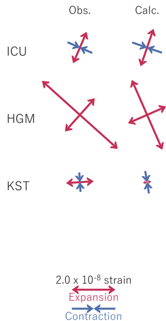
第35図 2024/05/30PM-06/01の歪・傾斜変化（第34図[A]）を説明する断層モデル。
