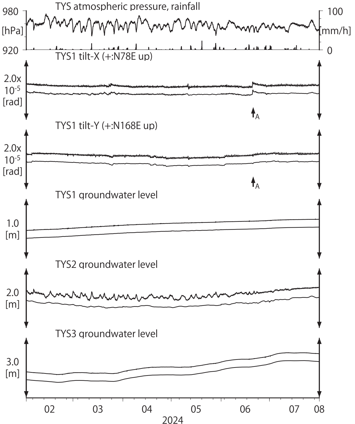
第3図 Tilt and groundwater level at TYS (時間値) (2024/02/01 00:00 - 2024/08/01 00:00 (JST))
