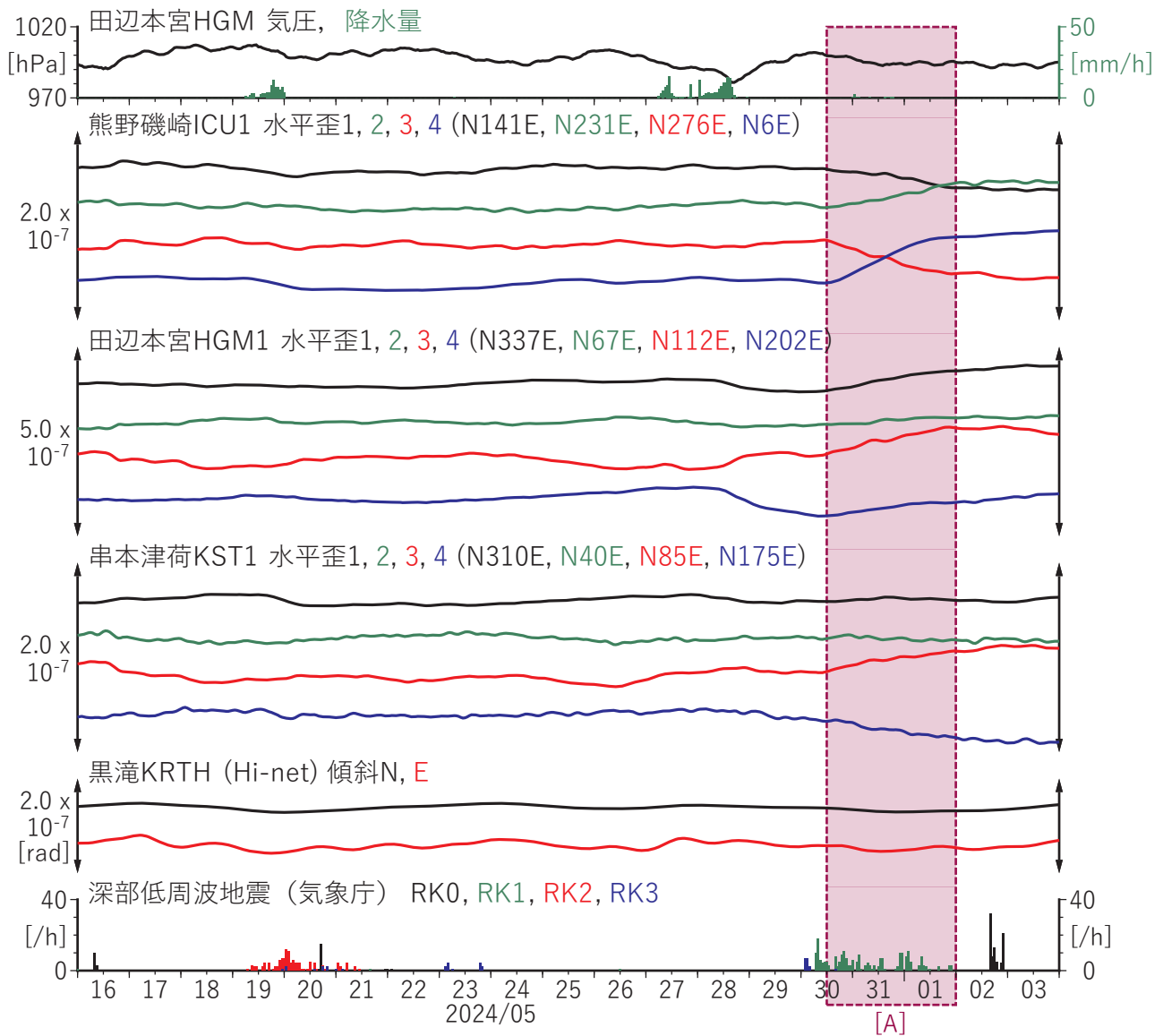
第34図 紀伊半島における歪・傾斜観測結果 (2024/05/16 00:00 - 2024/06/04 00:00 (JST))
