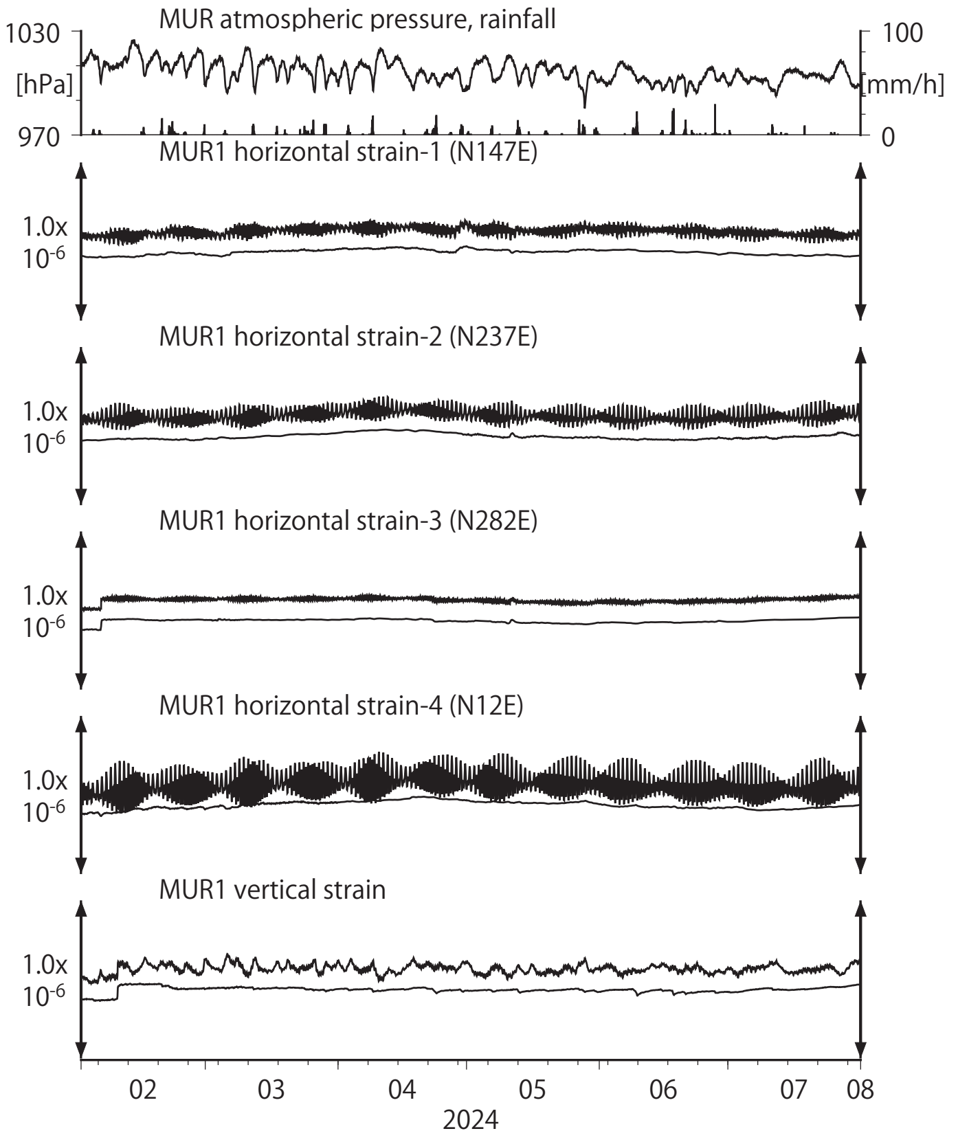
第21図 Crustal strains at MUR (時間値) (2024/02/01 00:00 - 2024/08/01 00:00 (JST))
