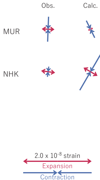
第48図 2024/07/04-06の歪・傾斜変化 (第47図[A]) を説明する断層モデル。
