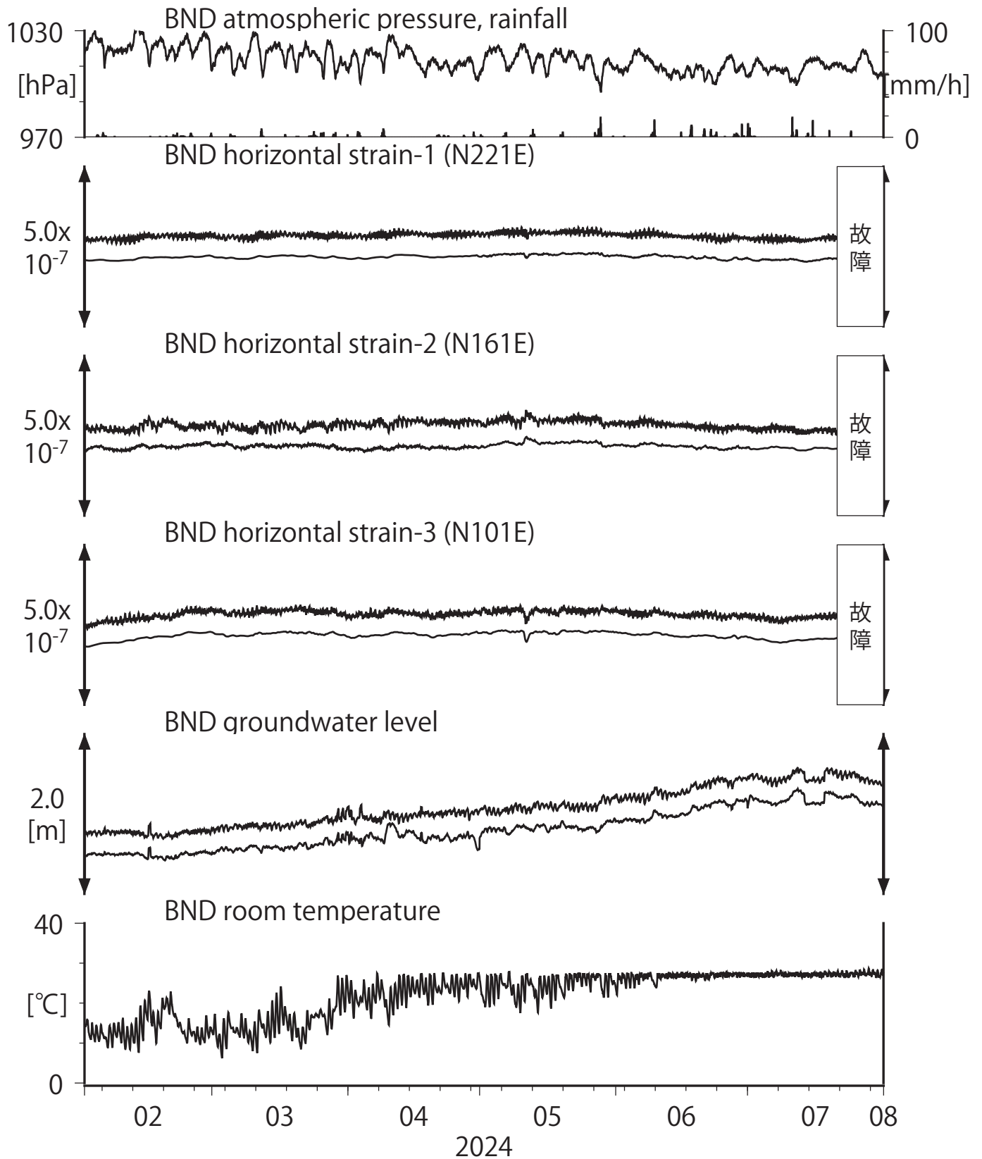
第19図 Crustal strains and groundwater level at BND (時間値) (2024/02/01 00:00 - 2024/08/01 00:00 (JST))
