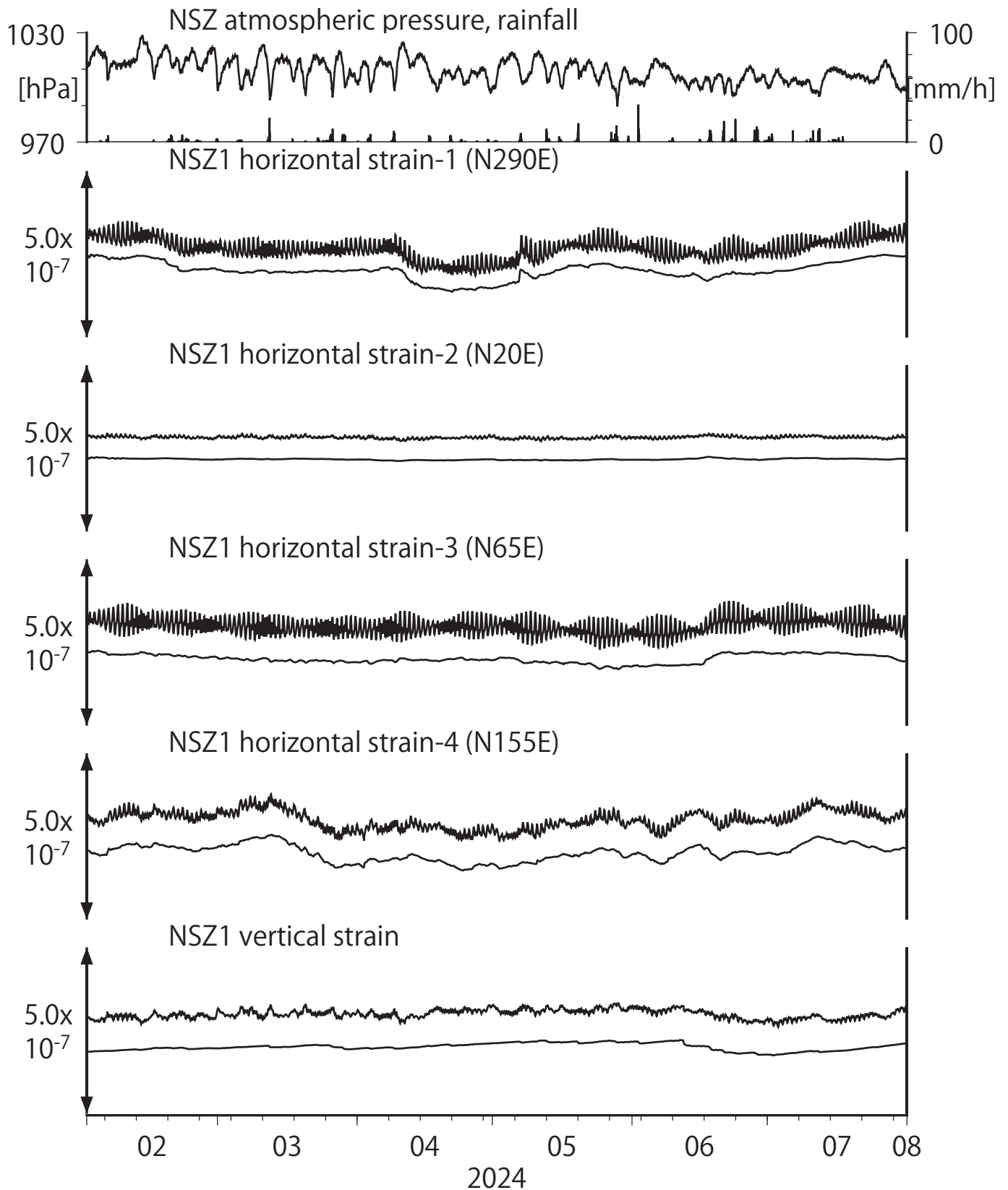
第4図 Crustal strains at NSZ (時間値) (2024/02/01 00:00 - 2024/08/01 00:00 (JST))
