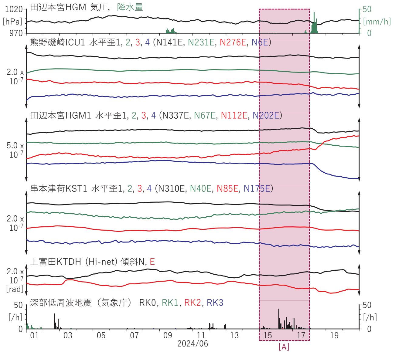
第37図 紀伊半島における歪・傾斜観測結果 (2024/06/01 00:00 - 2024/06/21 00:00 (JST))
