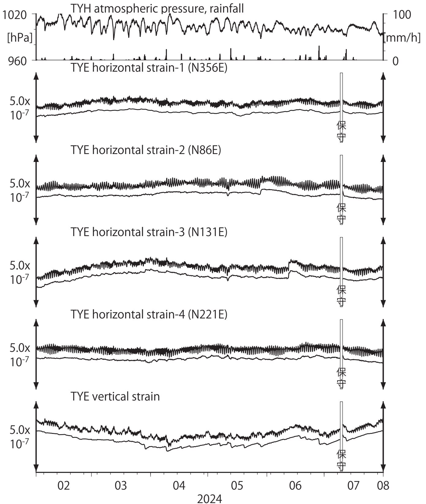
第6図 Crustal strain at TYE (時間値) (2024/02/01 00:00 - 2024/08/01 00:00 (JST))
