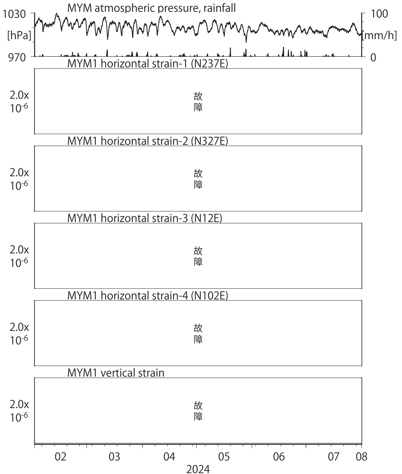
第11図 Crustal strains at MYM (時間値) (2024/02/01 00:00 - 2024/08/01 00:00 (JST))
