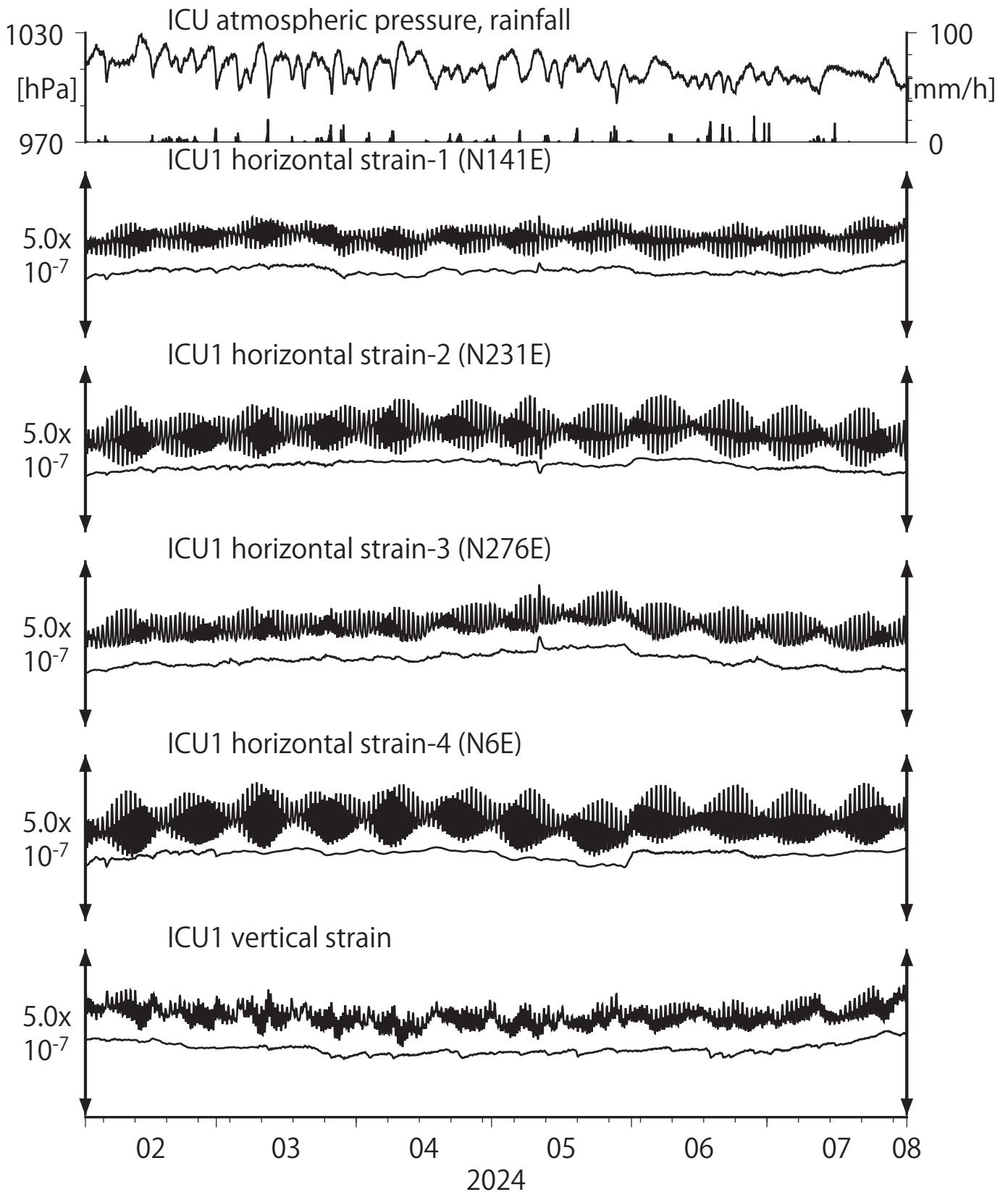
第13図 Crustal strains at ICU (時間値) (2024/02/01 00:00 - 2024/08/01 00:00 (JST))
