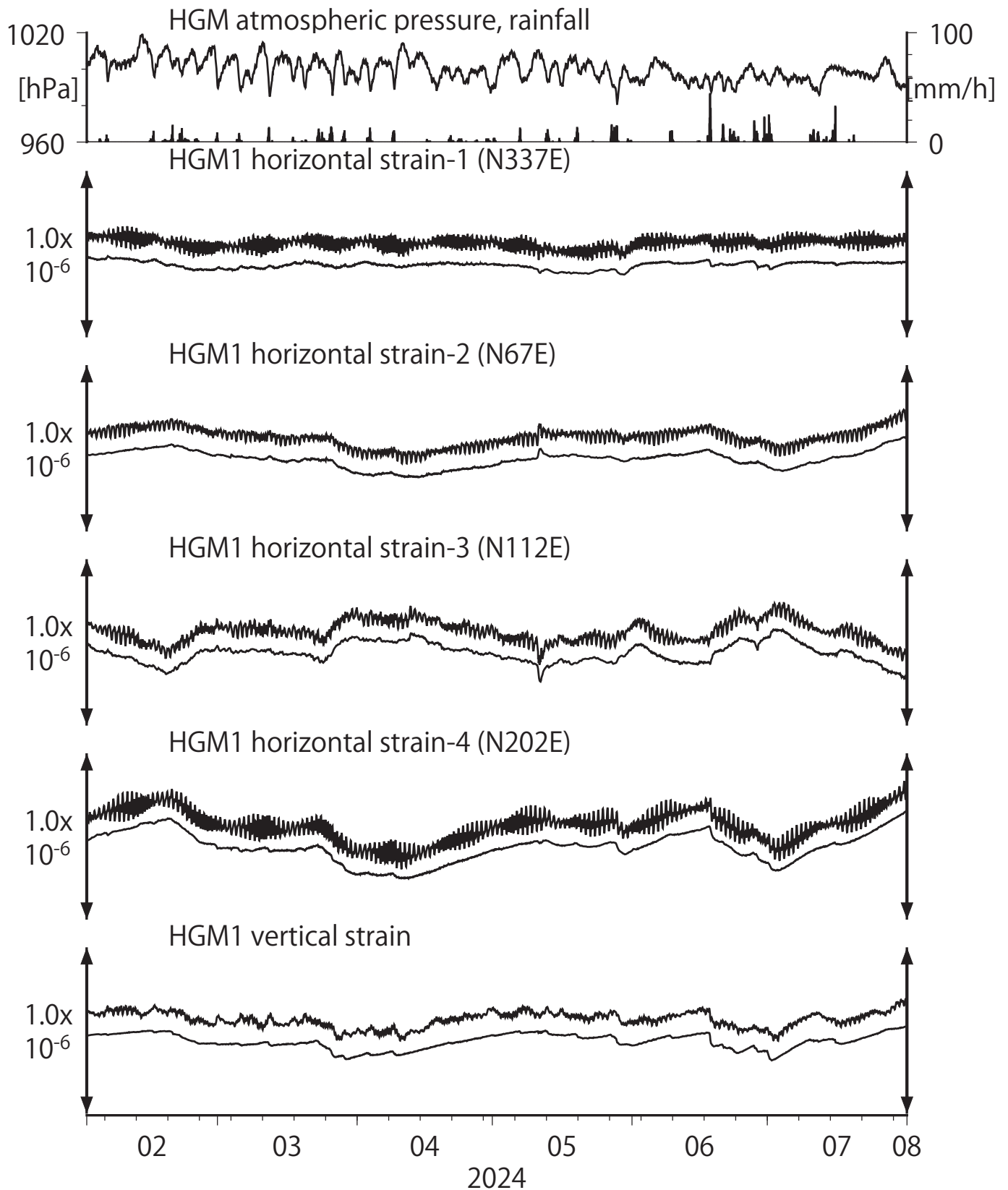
第15図 Crustal strains at HGM (時間値) (2024/02/01 00:00 - 2024/08/01 00:00 (JST))
