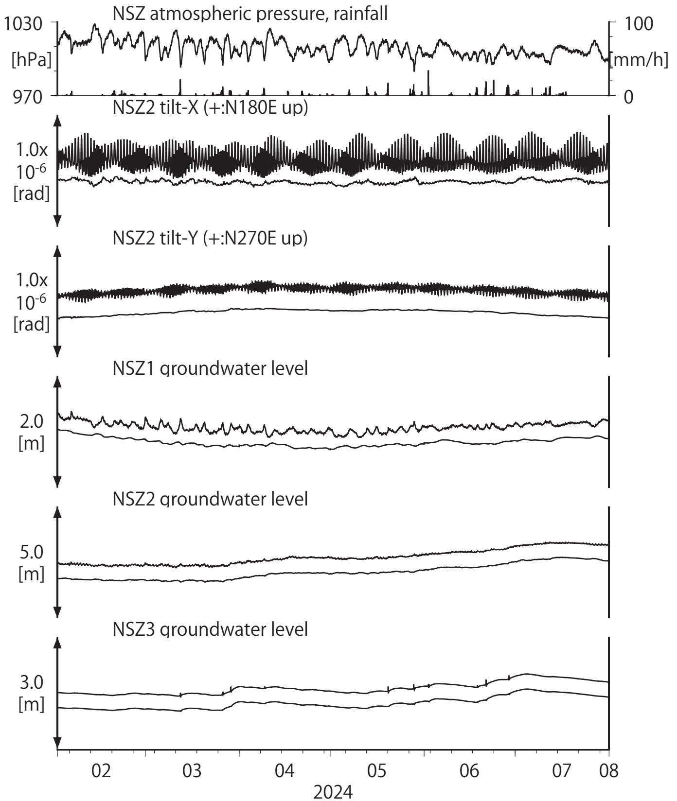
第5図 Tilt and groundwater level at NSZ (時間値) (2024/02/01 00:00 - 2024/08/01 00:00 (JST))
