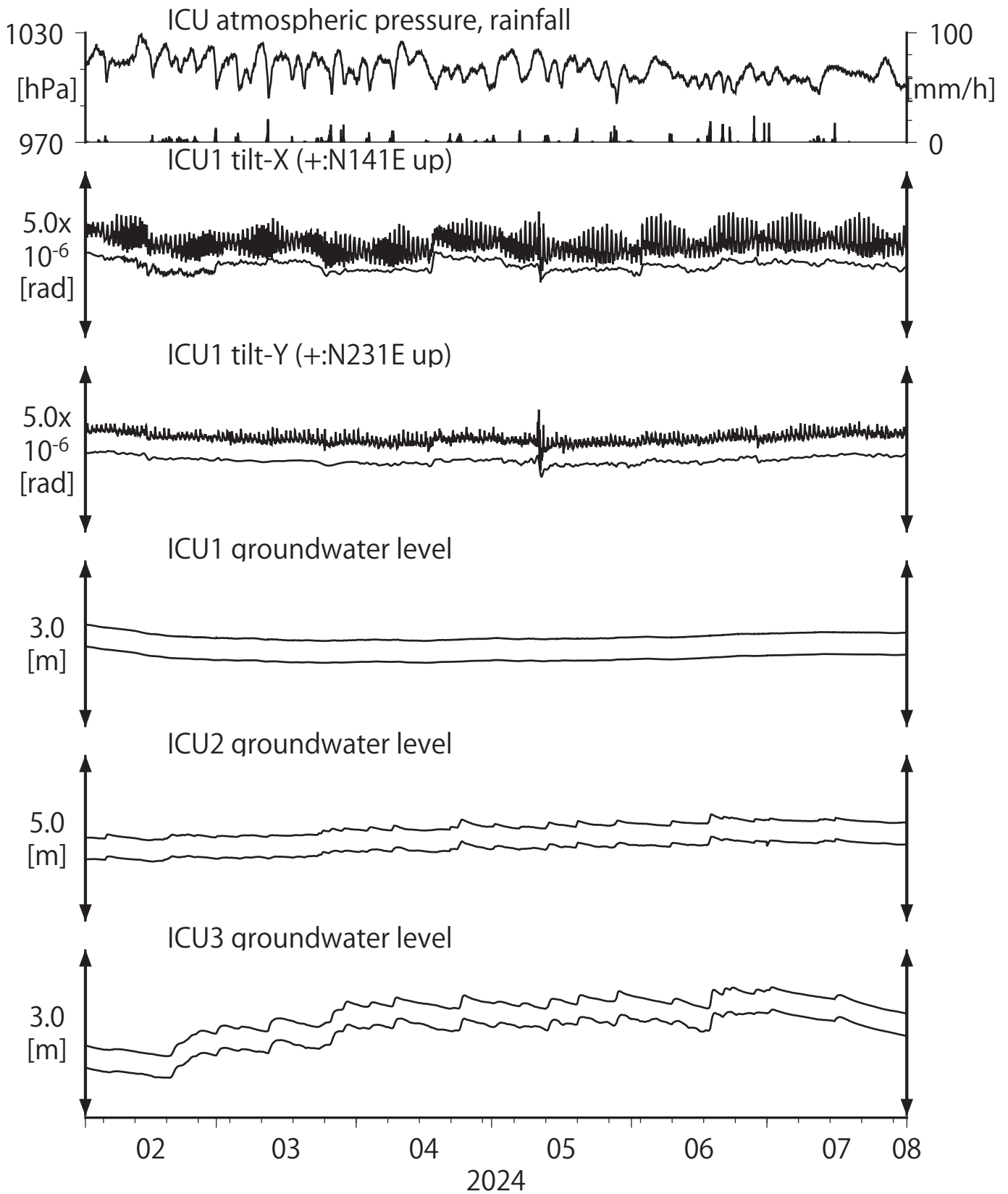
第14図 Tilt and groundwater level at ICU (時間値) (2024/02/01 00:00 - 2024/08/01 00:00 (JST))
