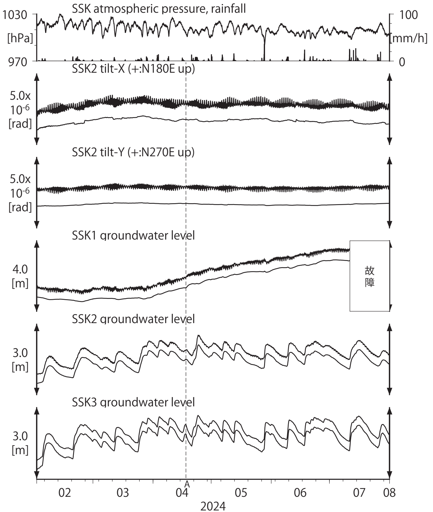
第25図 Tilt and groundwater level at SSK (時間値) (2024/02/01 00:00 - 2024/08/01 00:00 (JST))
