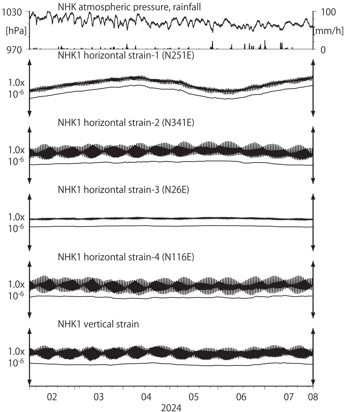
第31図 Crustal strains at NHK (時間値) (2024/02/01 00:00 - 2024/08/01 00:00 (JST))
