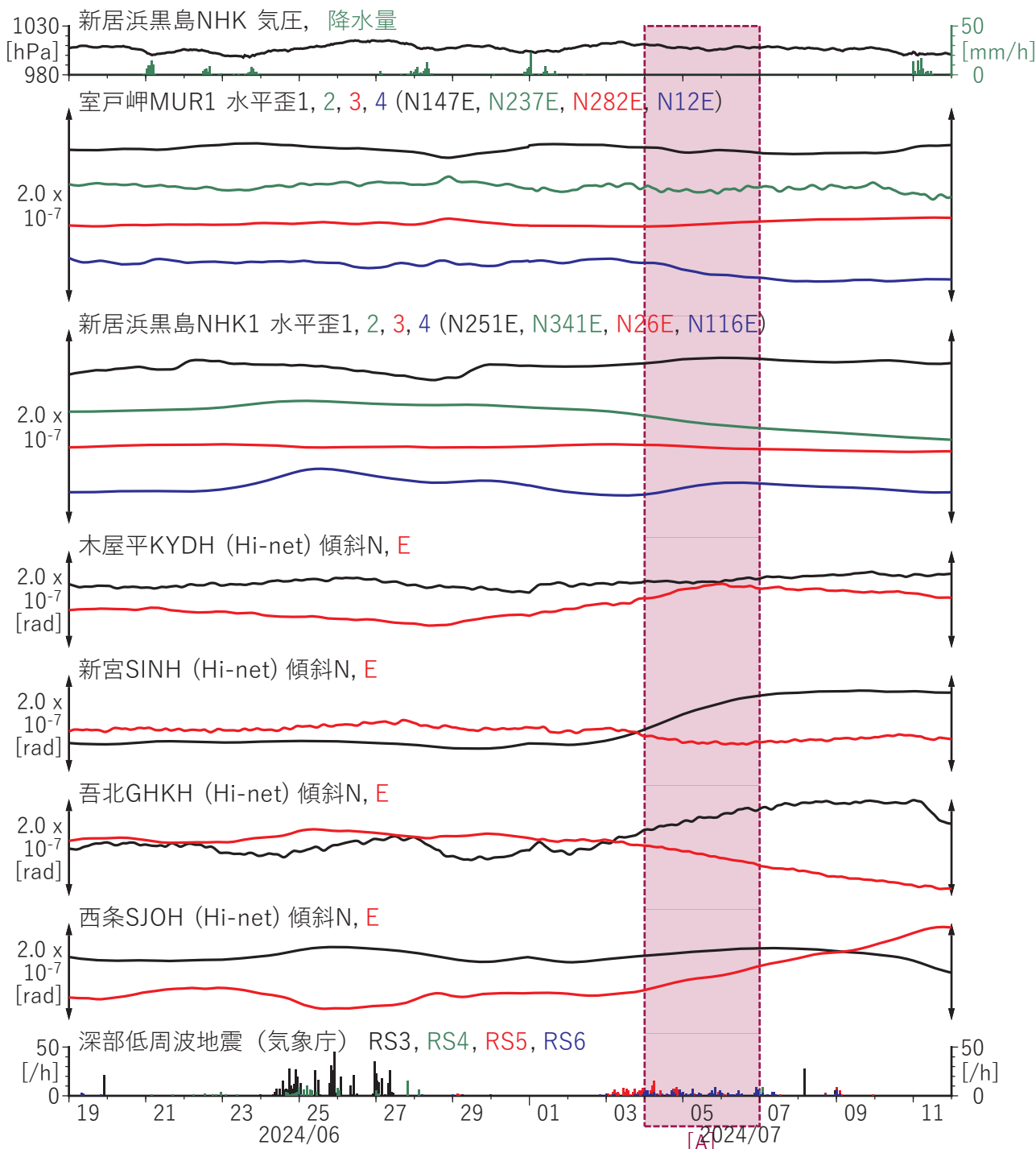
第47図 四国における歪・傾斜観測結果 (2024/06/19 00:00 - 2024/07/12 00:00 (JST))
