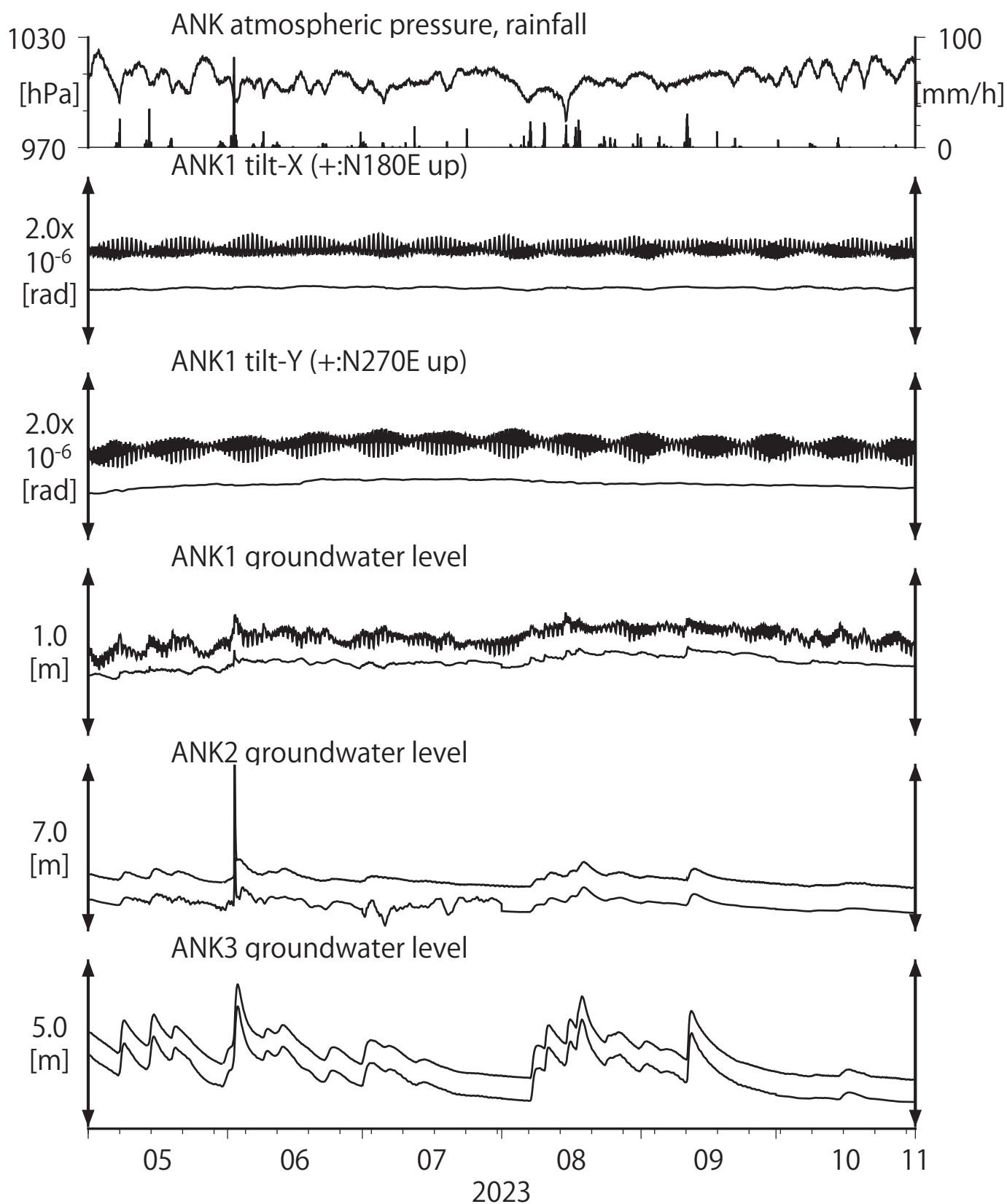
第20図 Tilt and groundwater level at ANK (時間値) (2023/05/01 00:00 - 2023/11/01 00:00 (JST))
