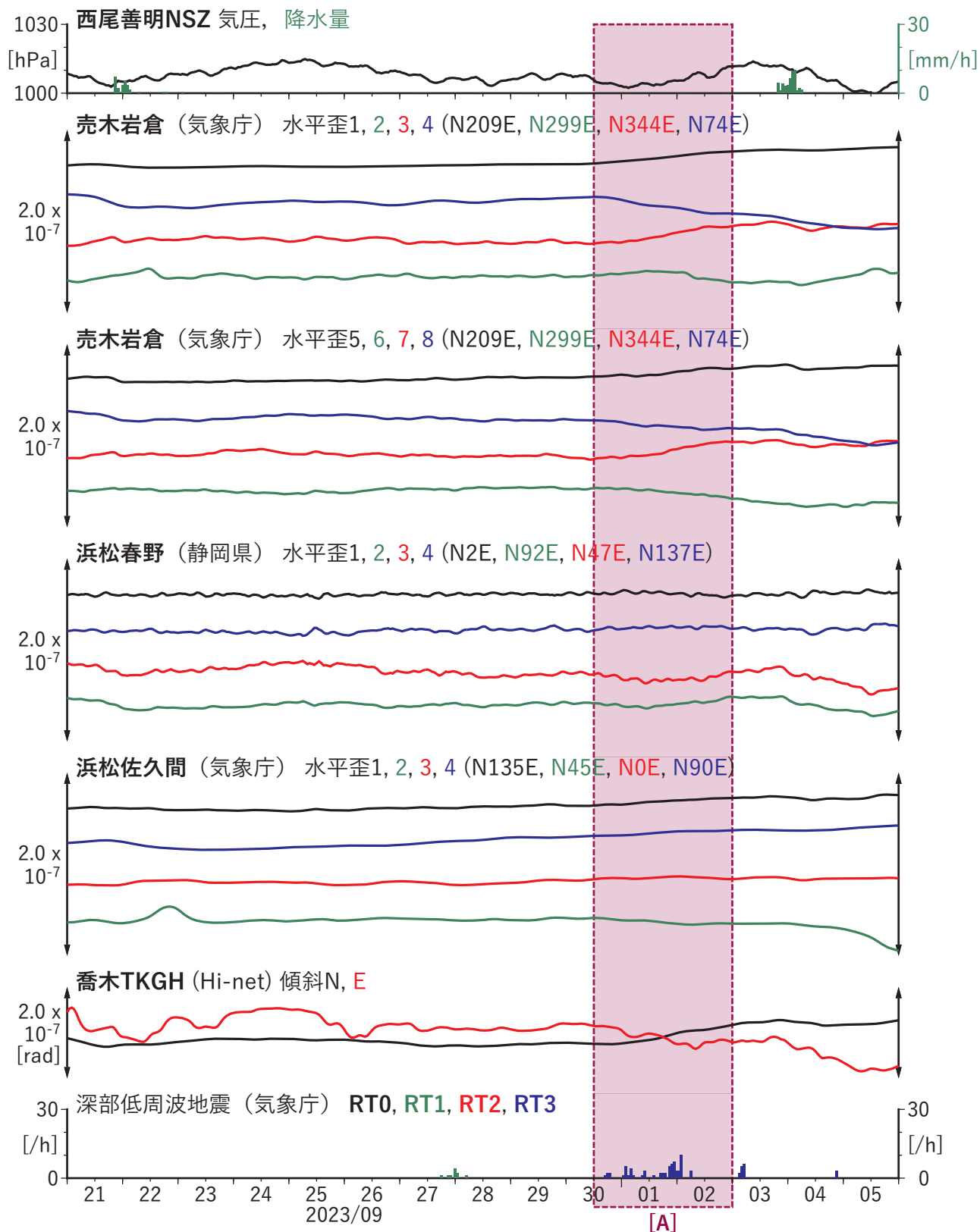
第52図 東海地方における歪・傾斜の時間変化 (2023/09/21 00:00 - 2023/10/06 00:00 (JST))
