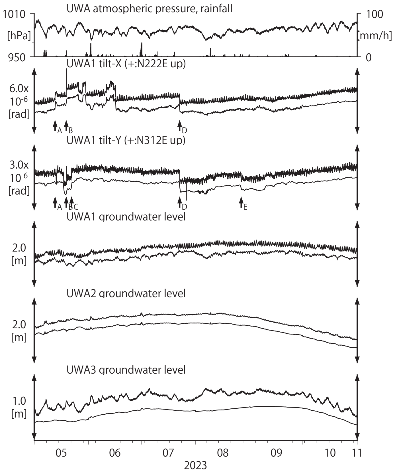
第29図 Tilt and groundwater level at UWA (時間値) (2023/05/01 00:00 - 2023/11/01 00:00 (JST))
