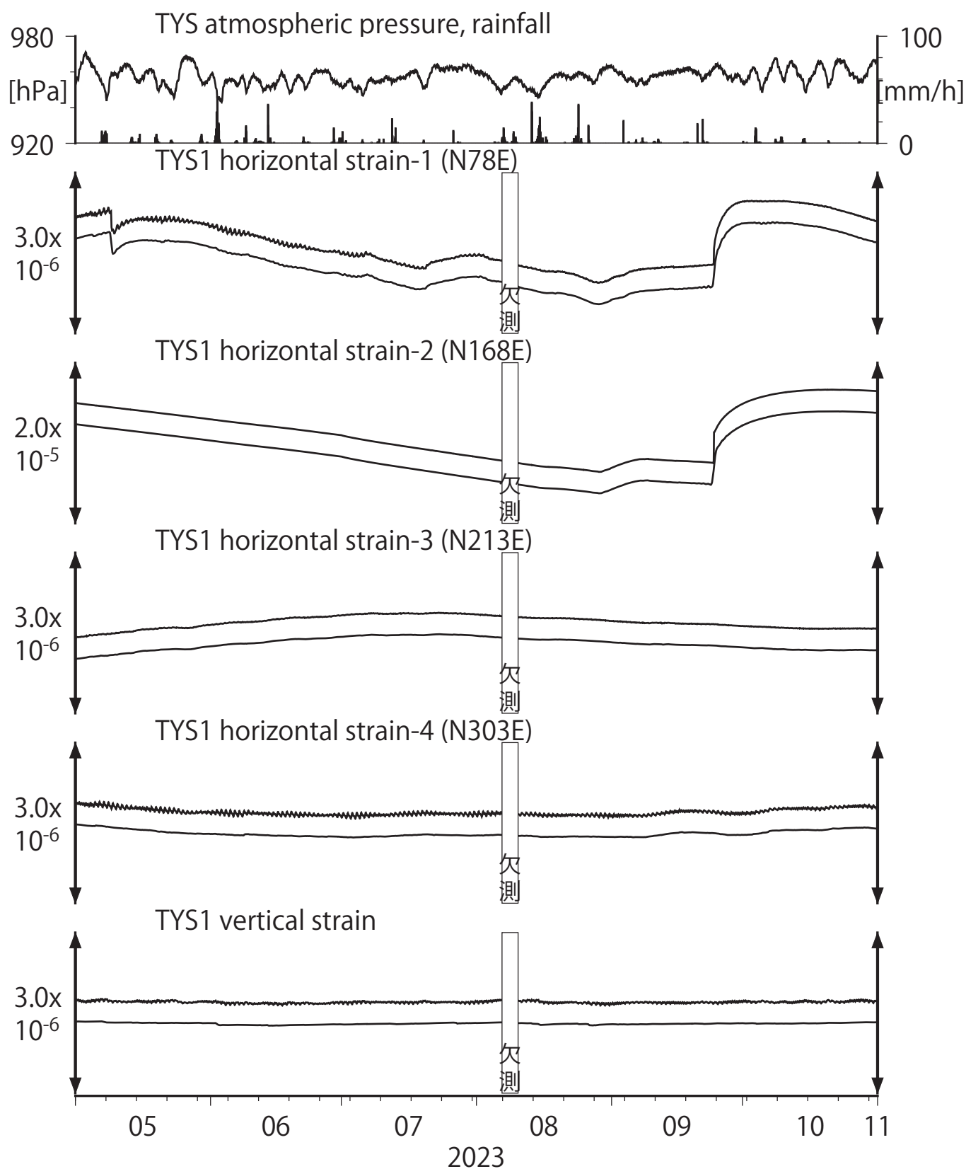
第2図 Crustal strains at TYS (時間値) (2023/05/01 00:00 - 2023/11/01 00:00 (JST))
