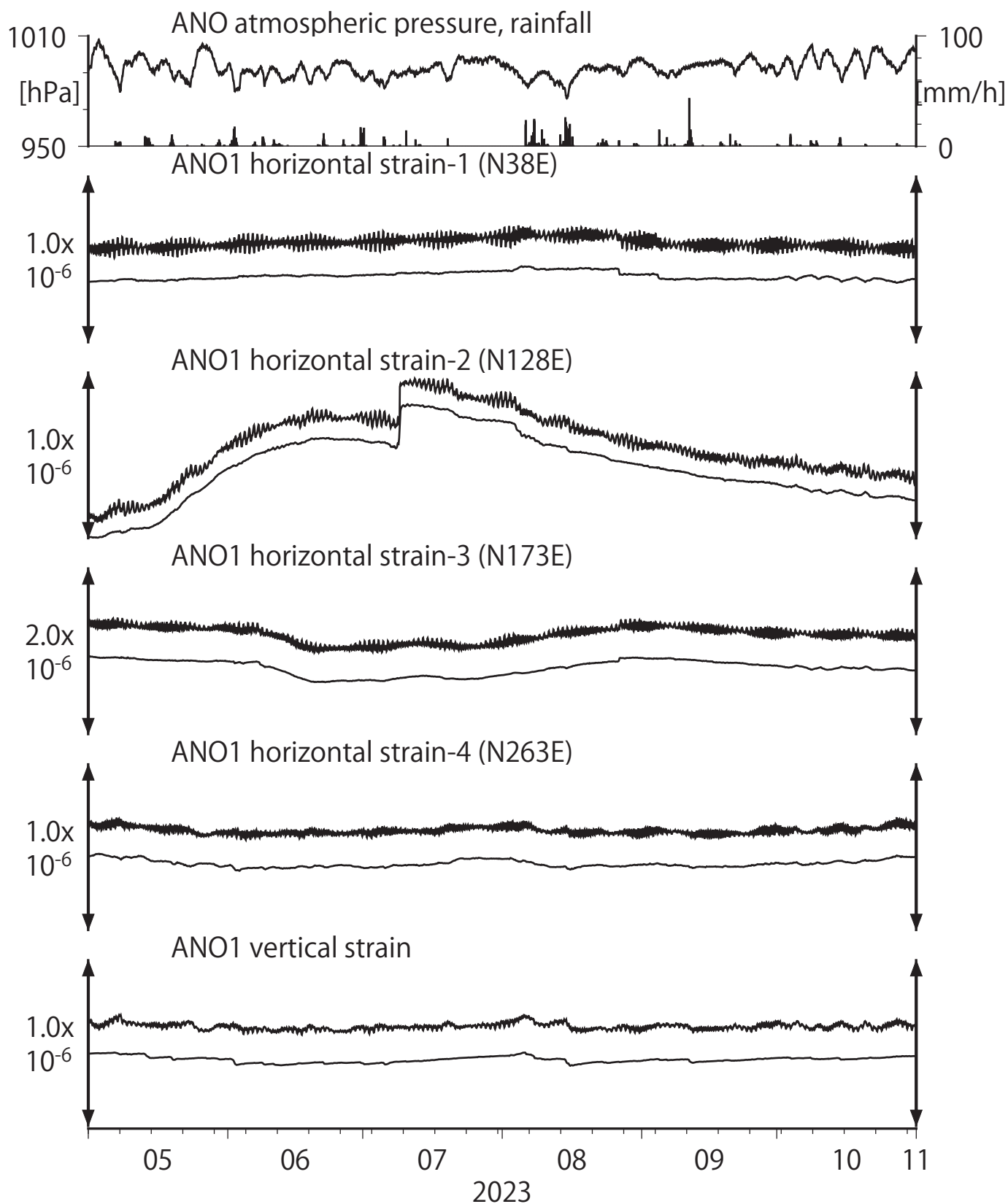
第8図 Crustal strains at ANO (時間値) (2023/05/01 00:00 - 2023/11/01 00:00 (JST))
