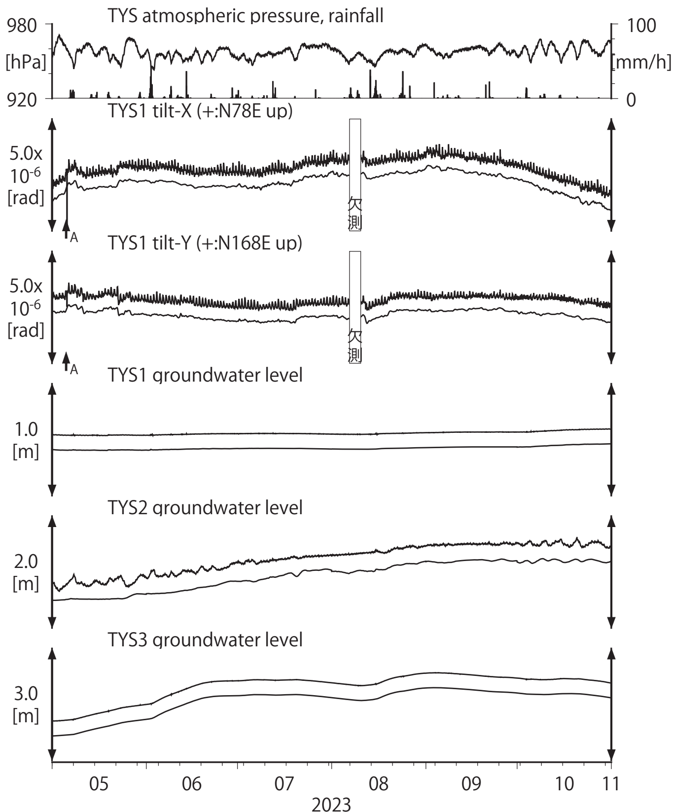
第3図 Tilt and groundwater level at TYS (時間値) (2023/05/01 00:00 - 2023/11/01 00:00 (JST))
