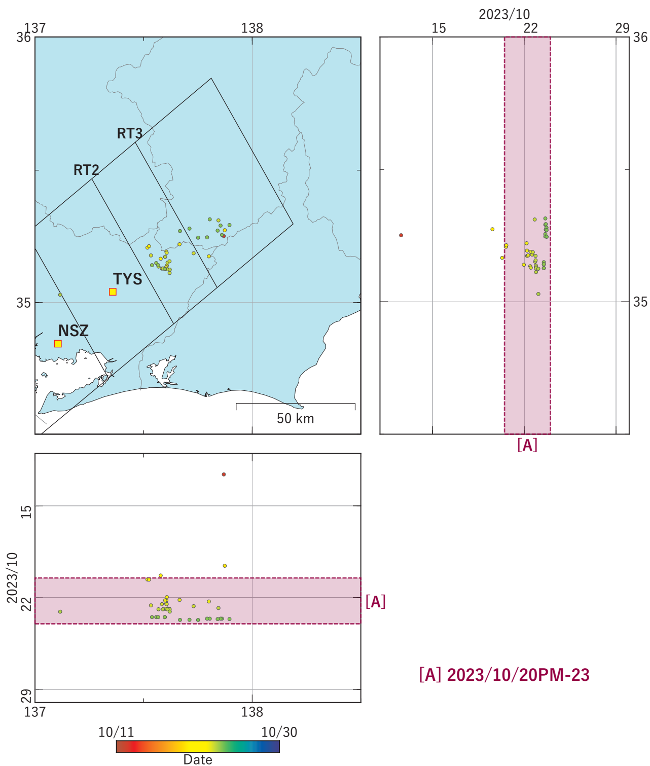
第57図 東海地方における深部低周波地震の時空間分布図。 (2023/10/11 00:00 - 2023/10/30 00:00 (JST)) 気象庁カタログによる。
