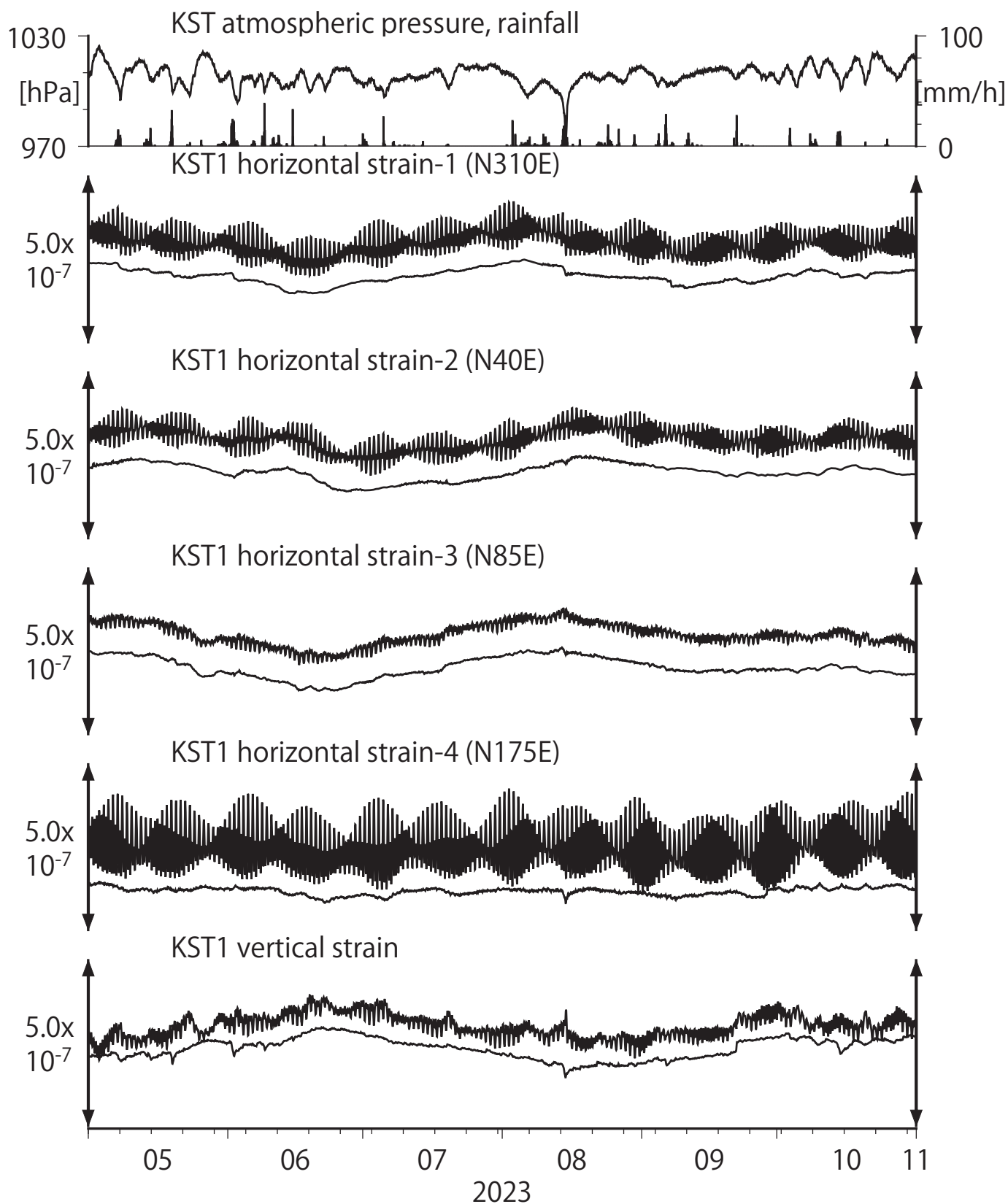
第17図 Crustal strains at KST (時間値) (2023/05/01 00:00 - 2023/11/01 00:00 (JST))
