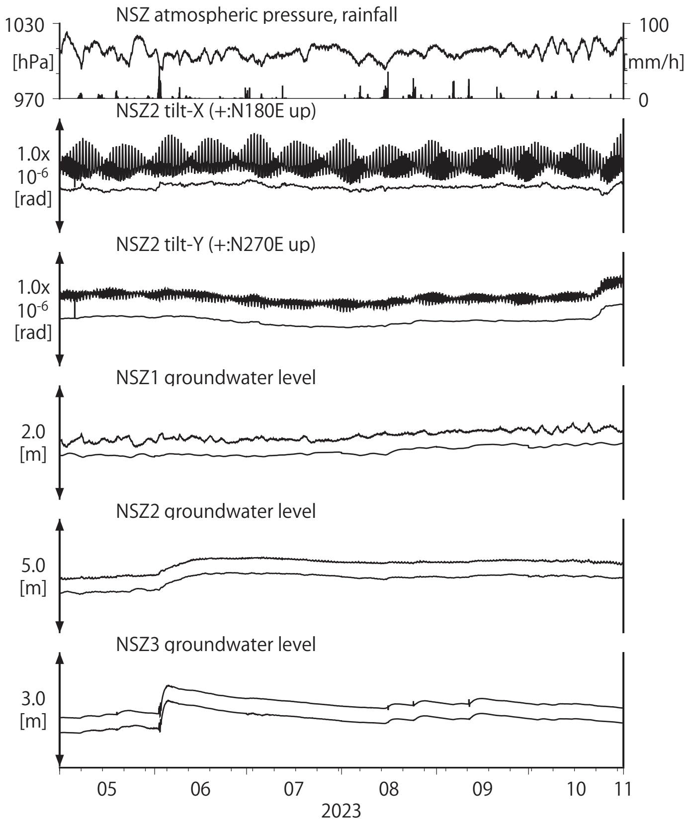
第5図 Tilt and groundwater level at NSZ (時間値) (2023/05/01 00:00 - 2023/11/01 00:00 (JST))
