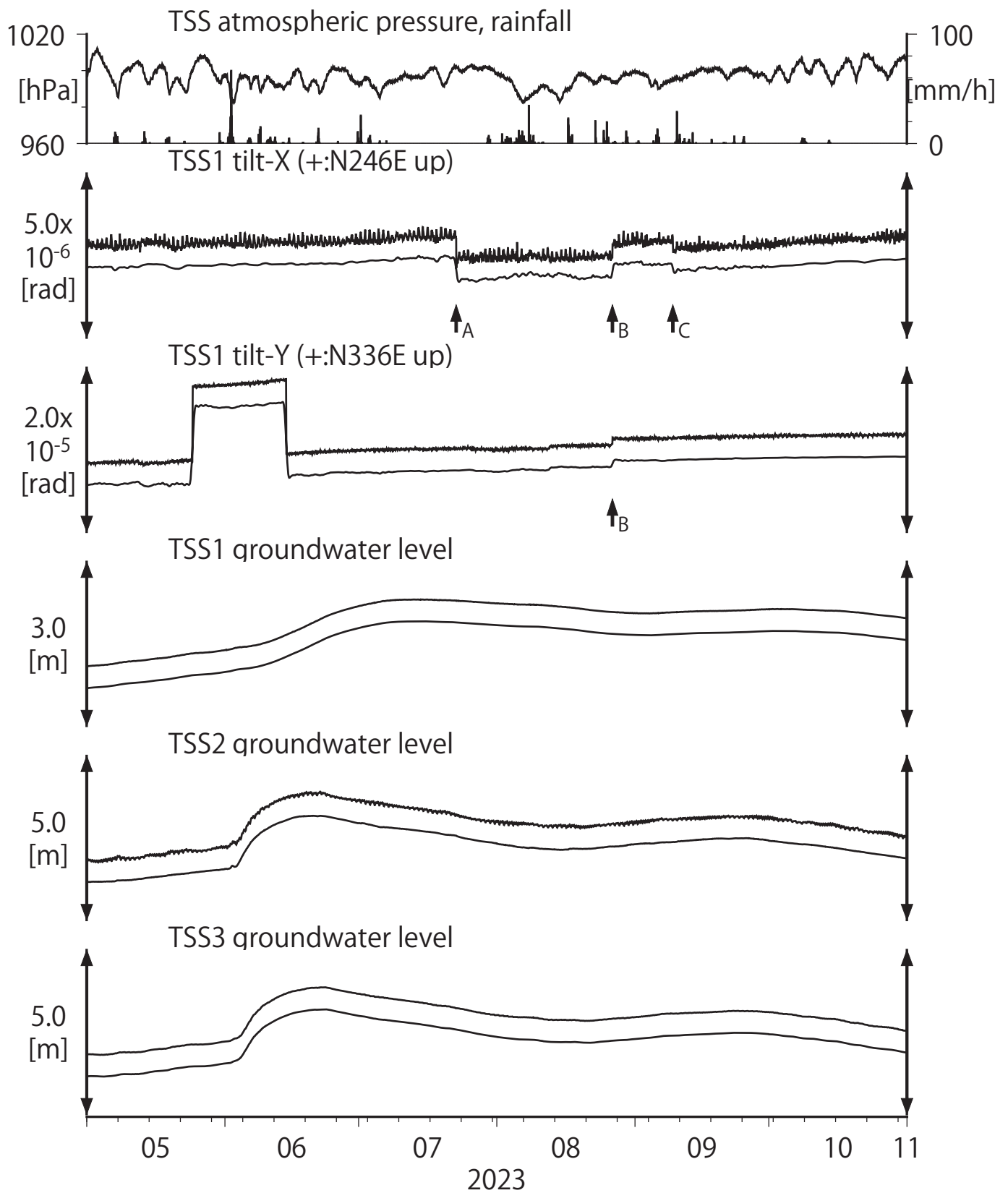
第27図 Tilt and groundwater level at TSS (時間値) (2023/05/01 00:00 - 2023/11/01 00:00 (JST))
