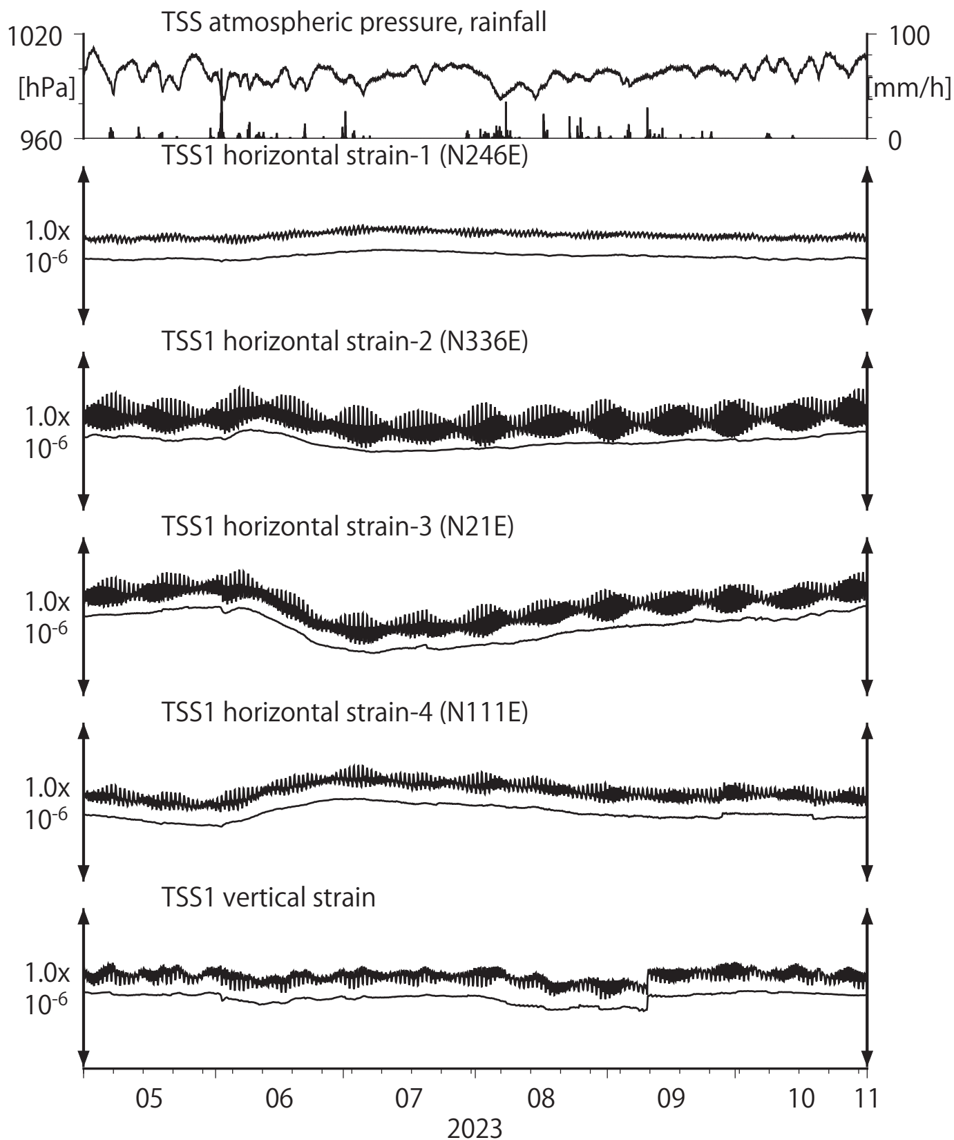
第26図 Crustal strains at TSS (時間値) (2023/05/01 00:00 - 2023/11/01 00:00 (JST))
