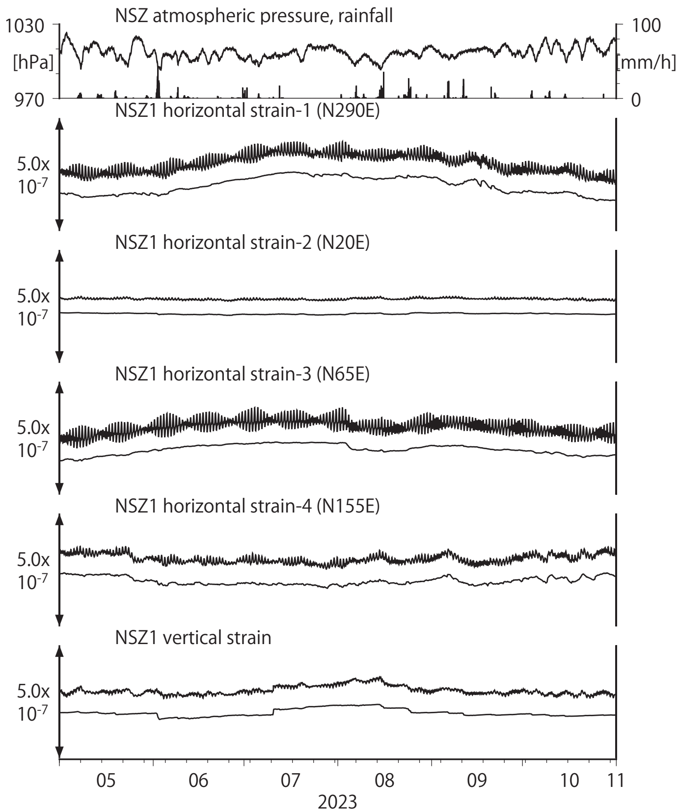
第4図 Crustal strains at NSZ (時間値) (2023/05/01 00:00 - 2023/11/01 00:00 (JST))
