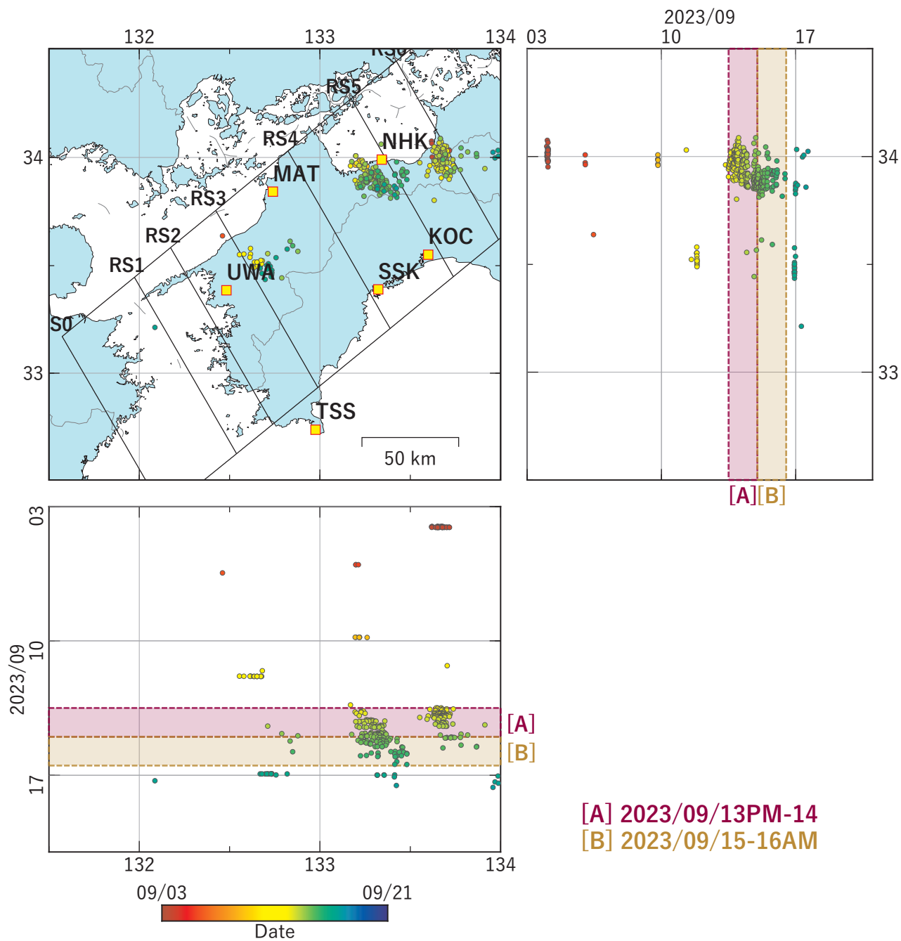
第44図 四国地方における深部低周波地震の時空間分布図。 (2023/09/03 00:00 - 2023/09/21 00:00 (JST)) 気象庁カタログによる。
