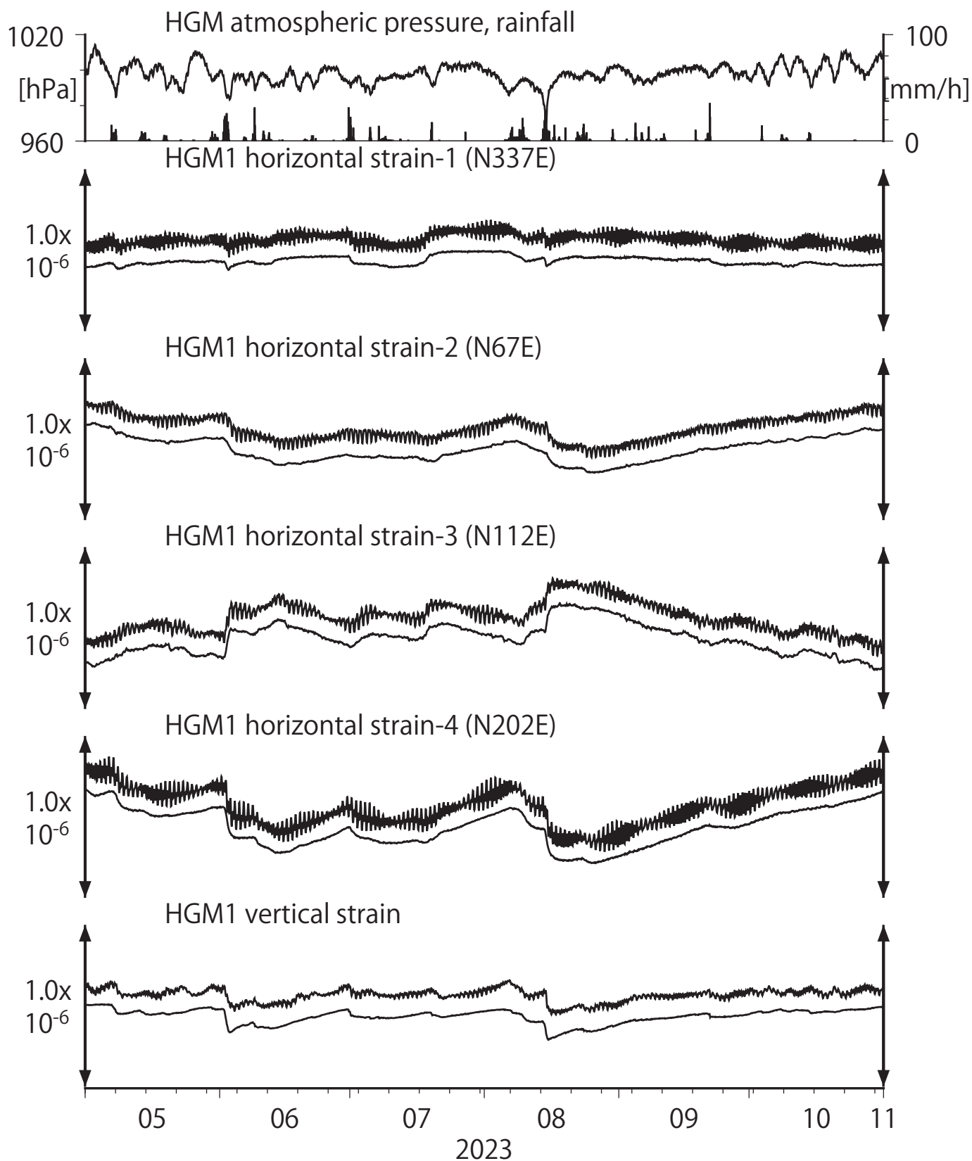
第15図 Crustal strains at HGM (時間値) (2023/05/01 00:00 - 2023/11/01 00:00 (JST))
