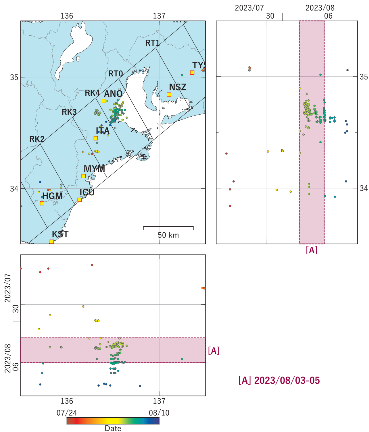
第33図 紀伊半島から東海地方における深部低周波地震の時空間分布図。 (2023/07/24 00:00 - 2023/08/10 00:00 (JST)) 気象庁カタログによる。
