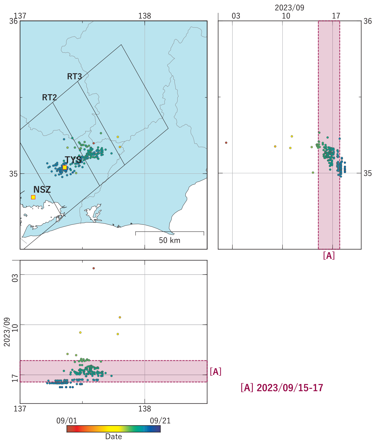
第48図 東海地方における深部低周波地震の時空間分布図。 (2023/09/01 00:00 - 2023/09/21 00:00 (JST)) 気象庁カタログによる。
