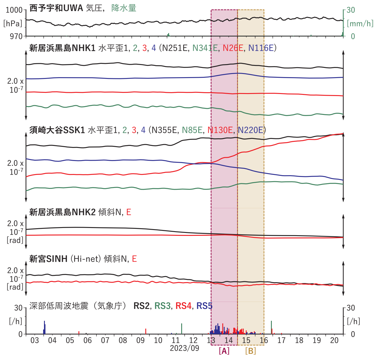
第45図 四国地方における歪・傾斜の時間変化 (2023/09/03 00:00 - 2023/09/21 00:00 (JST))
