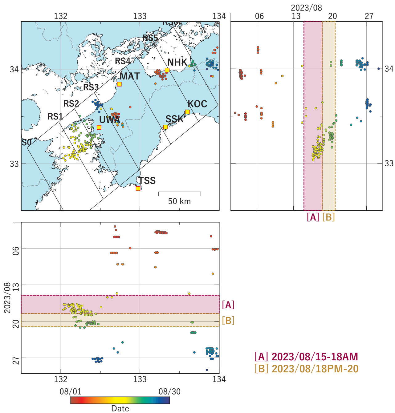
第36図 四国地方における深部低周波地震の時空間分布図。 (2023/08/01 00:00 - 2023/08/30 00:00 (JST)) 気象庁カタログによる。
