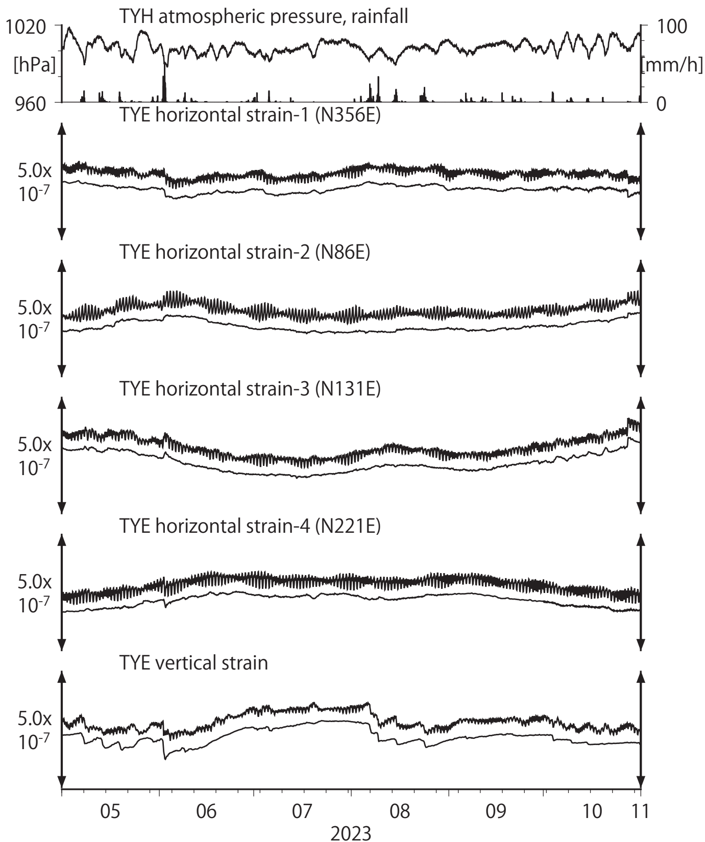
第6図 Crustal strain at TYE (時間値) (2023/05/01 00:00 - 2023/11/01 00:00 (JST))
