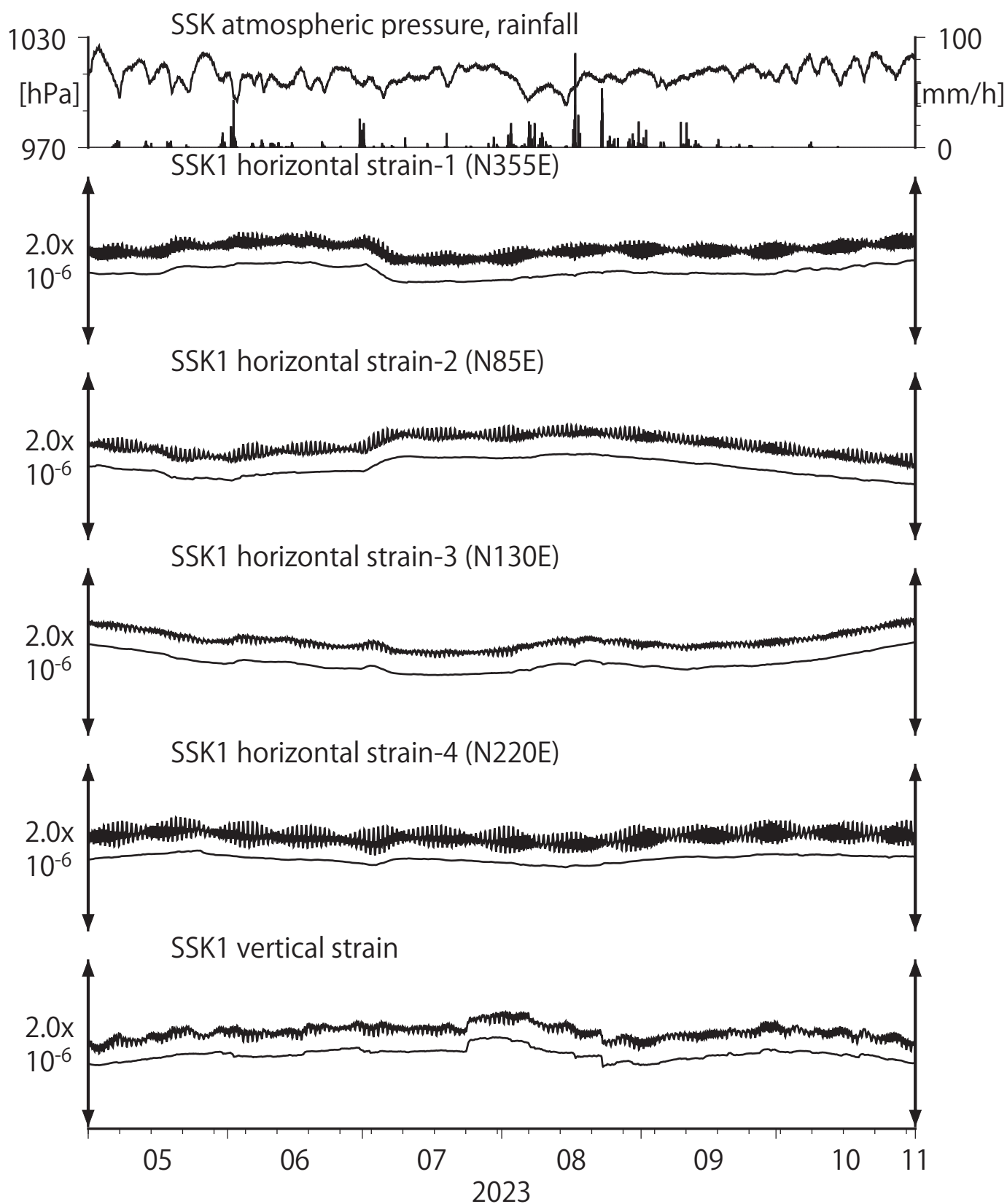
第24図 Crustal strains at SSK (時間値) (2023/05/01 00:00 - 2023/11/01 00:00 (JST))
