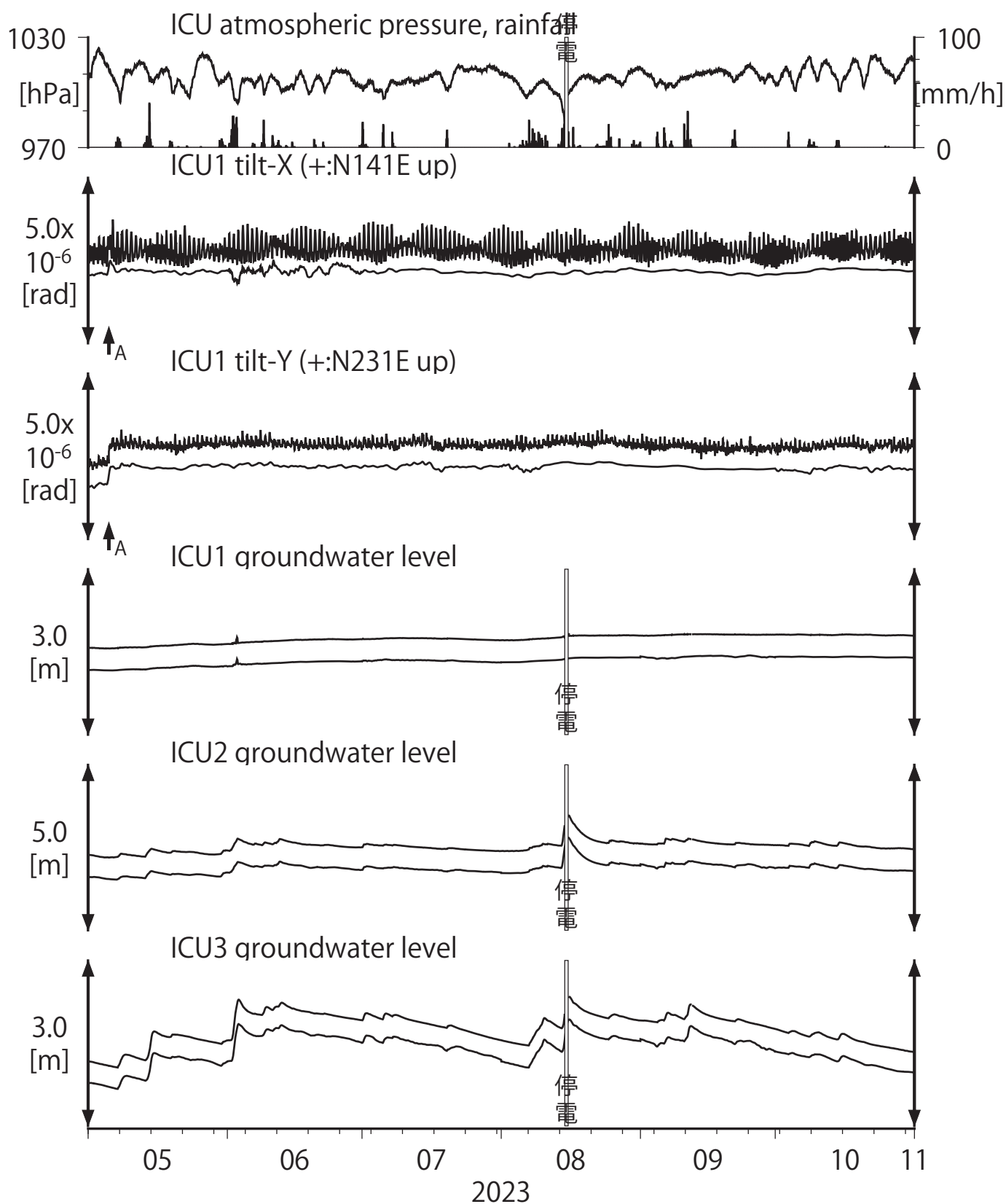
第14図 Tilt and groundwater level at ICU (時間値) (2023/05/01 00:00 - 2023/11/01 00:00 (JST))
