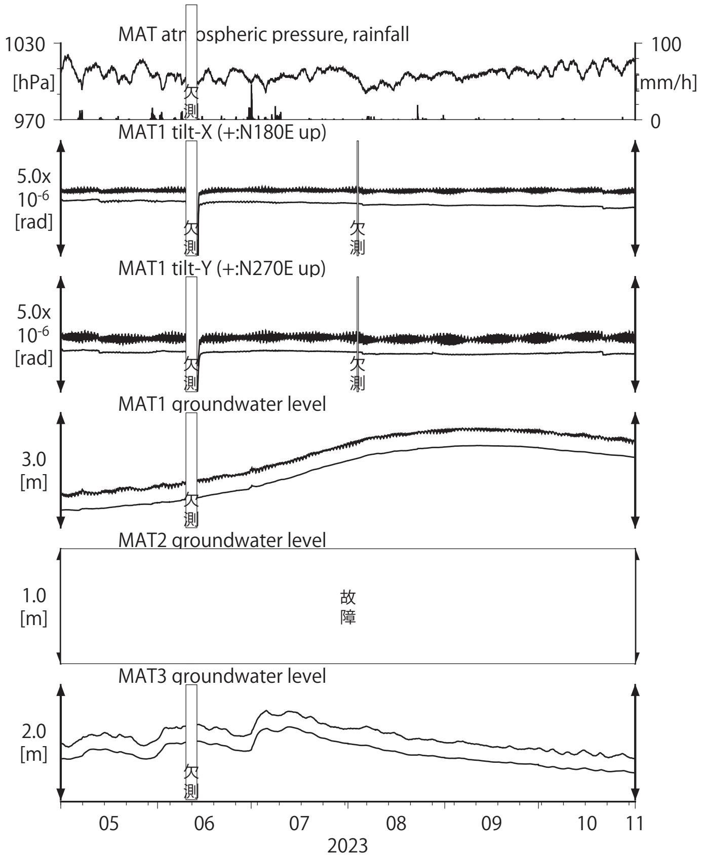
第30図 Tilt and groundwater level at MAT (時間値) (2023/05/01 00:00 - 2023/11/01 00:00 (JST))
