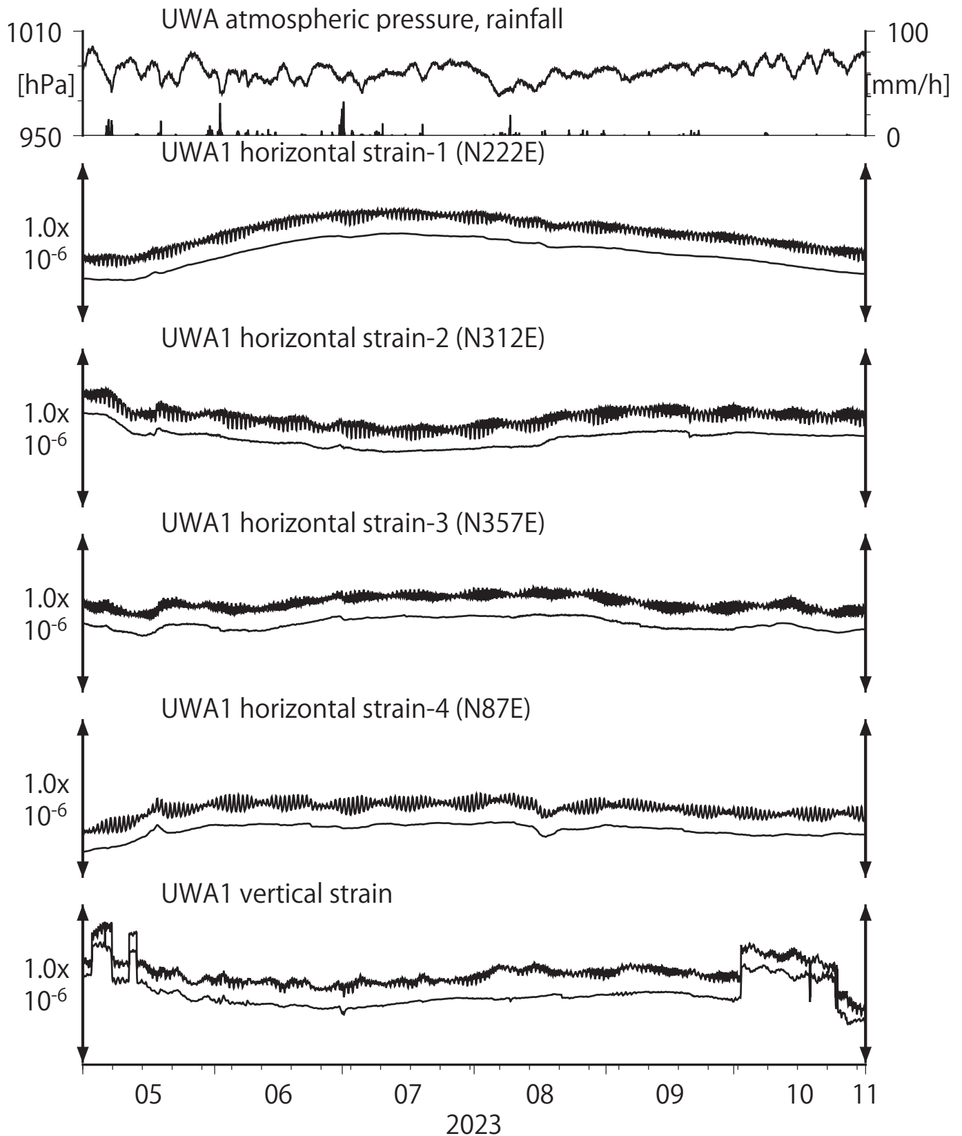
第28図 Crustal strains at UWA (時間値) (2023/05/01 00:00 - 2023/11/01 00:00 (JST))
