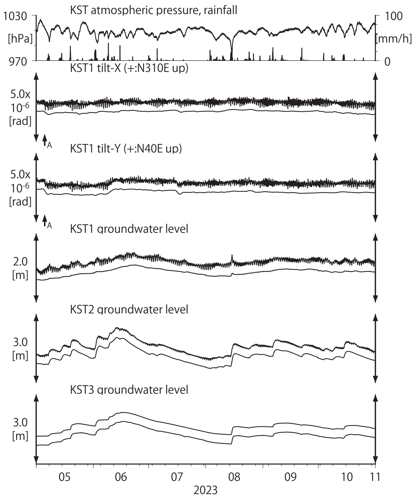
第18図 Tilt and groundwater level at KST (時間値) (2023/05/01 00:00 - 2023/11/01 00:00 (JST))
