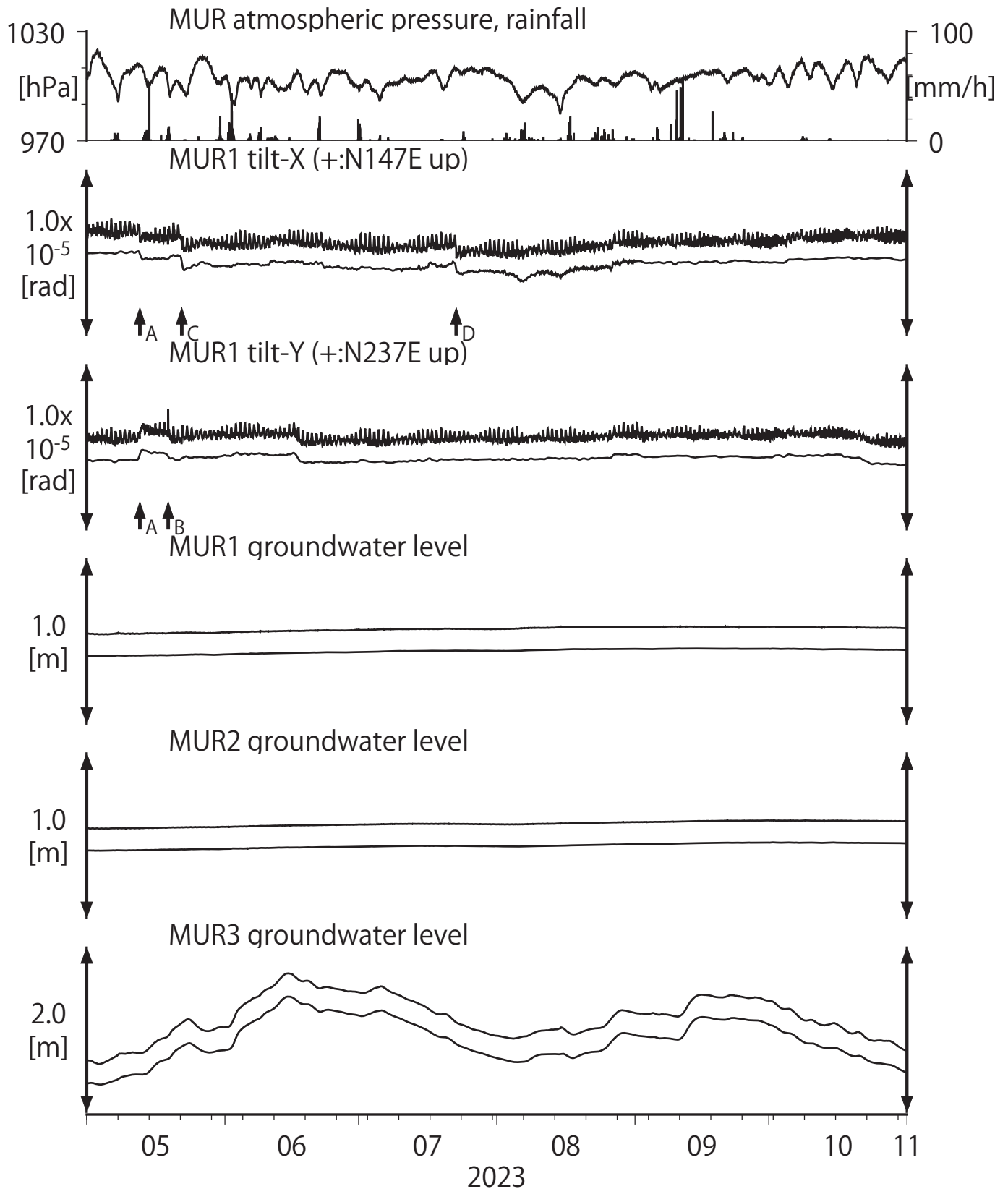
第22図 Tilt and groundwater level at MUR (時間値) (2023/05/01 00:00 - 2023/11/01 00:00 (JST))
