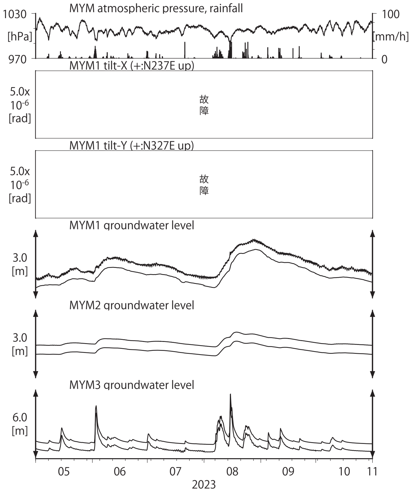
第12図 Tilt and groundwater level at MYM (時間値) (2023/05/01 00:00 - 2023/11/01 00:00 (JST))
