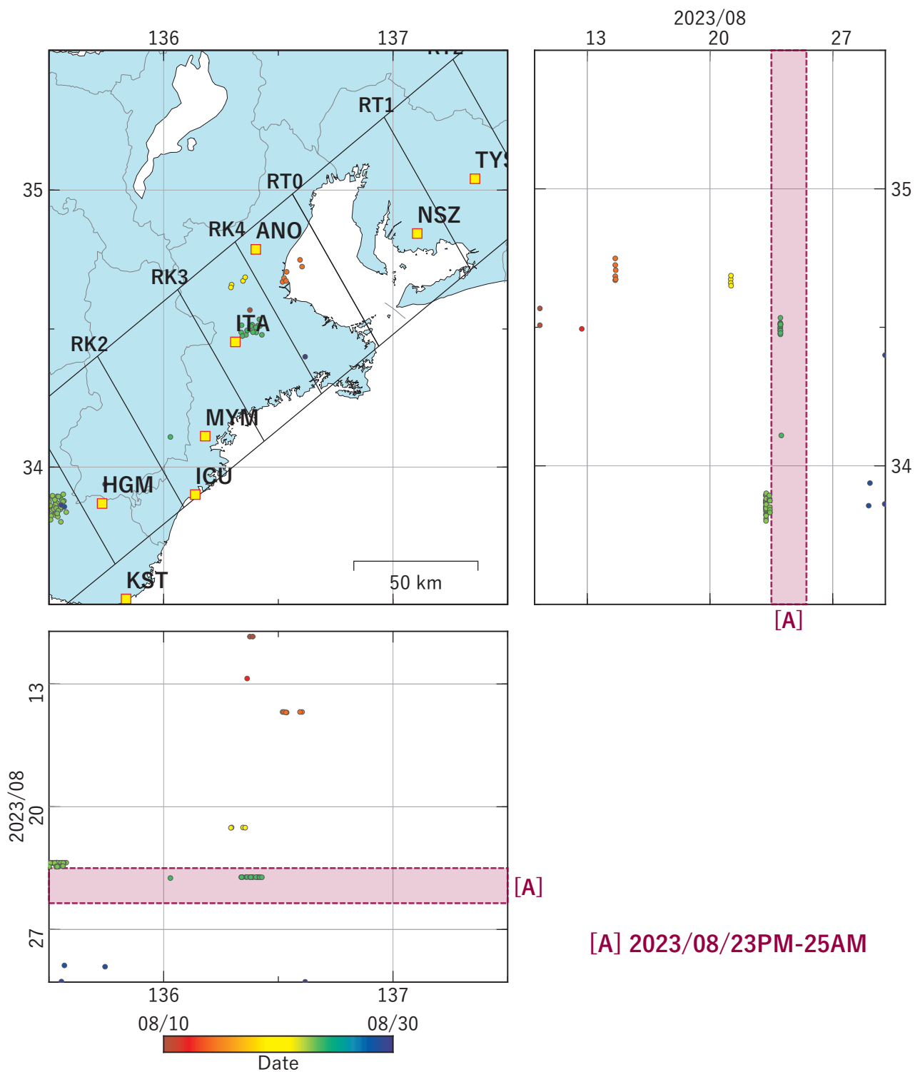
第40図 紀伊半島から東海地方における深部低周波地震の時空間分布図。 (2023/08/10 00:00 - 2023/08/30 00:00 (JST)) 気象庁カタログによる。
