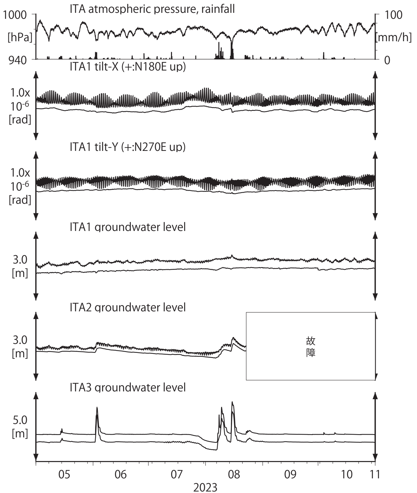
第10図 Tilt and groundwater level at ITA (時間値) (2023/05/01 00:00 - 2023/11/01 00:00 (JST))
