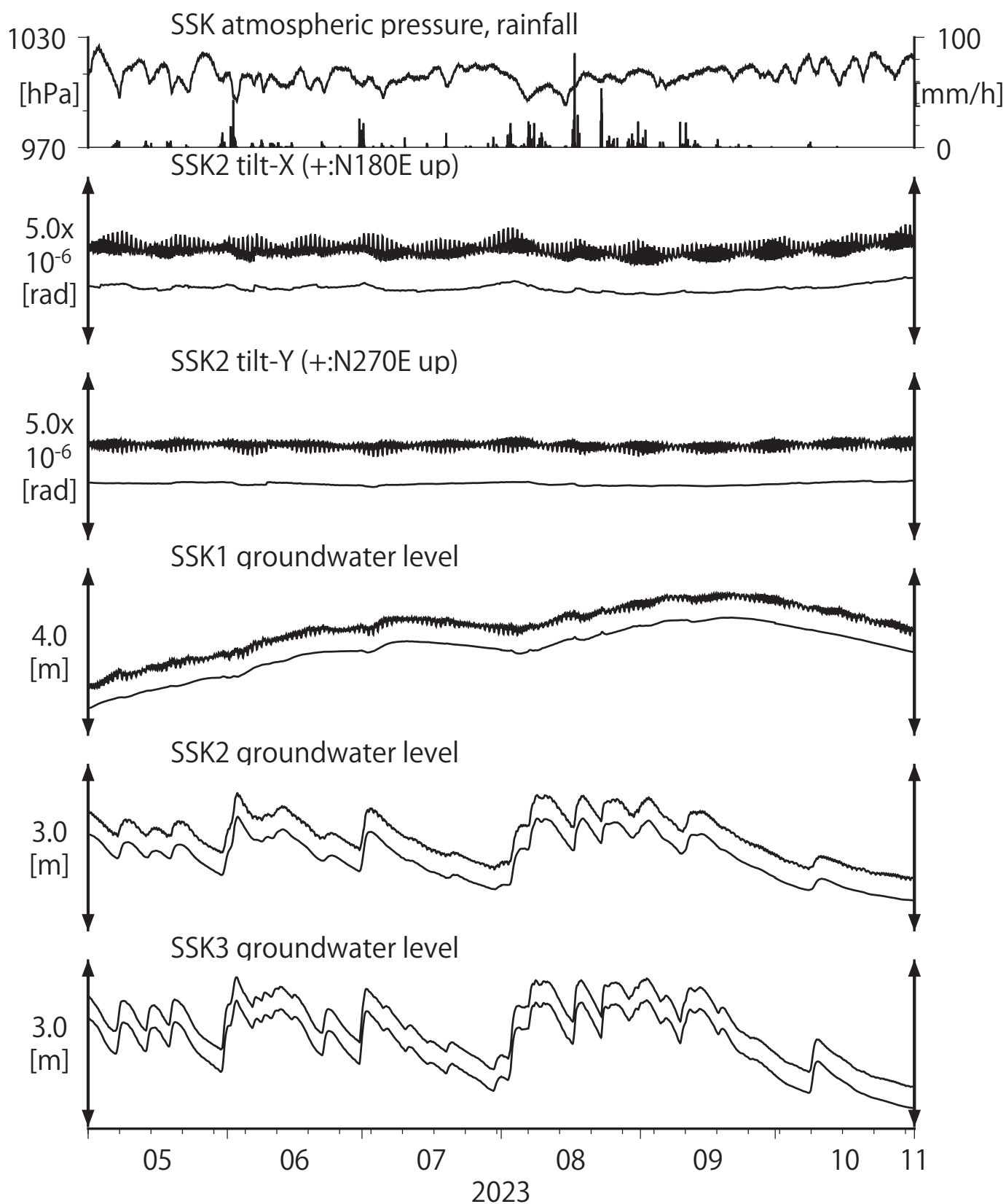
第25図 Tilt and groundwater level at SSK (時間値) (2023/05/01 00:00 - 2023/11/01 00:00 (JST))
