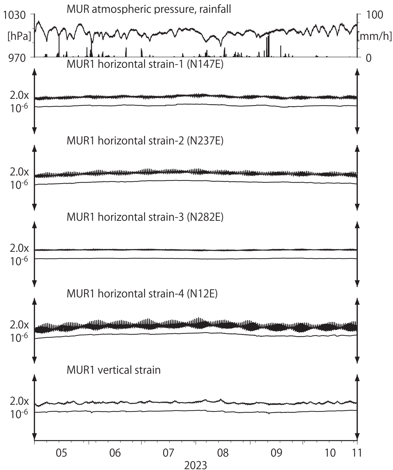
第21図 Crustal strains at MUR (時間値) (2023/05/01 00:00 - 2023/11/01 00:00 (JST))
