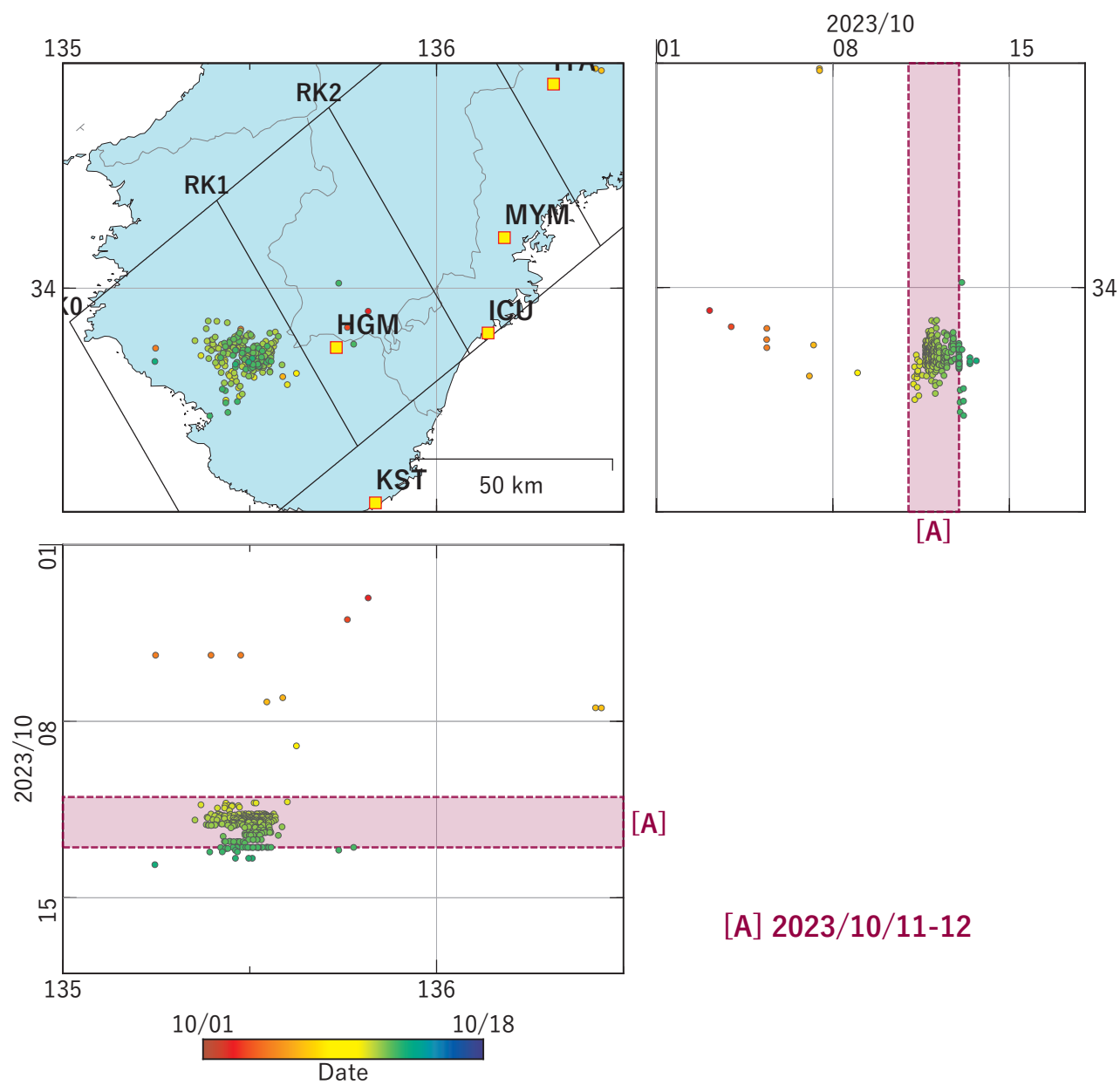
第54図 紀伊半島における深部低周波地震の時空間分布図。 (2023/10/01 00:00 - 2023/10/18 00:00 (JST)) 気象庁カタログによる。
