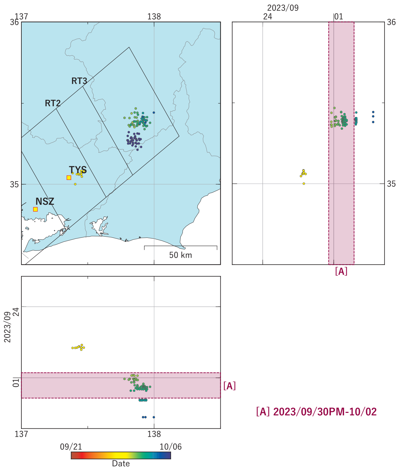
第51図 東海地方における深部低周波地震の時空間分布図。 (2023/09/21 00:00 - 2023/10/06 00:00 (JST)) 気象庁カタログによる。
