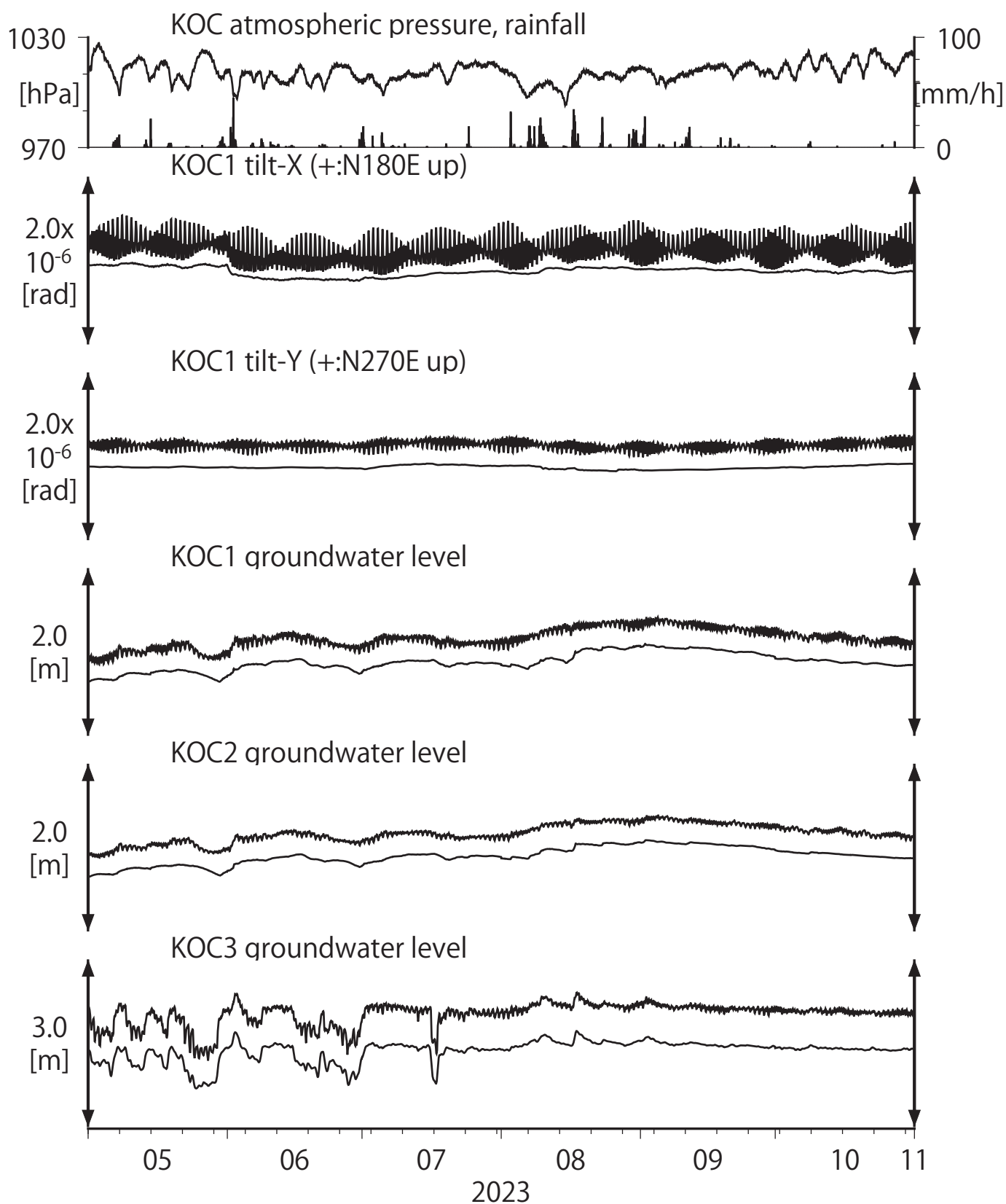
第23図 Tilt and groundwater level at KOC (時間値) (2023/05/01 00:00 - 2023/11/01 00:00 (JST))
