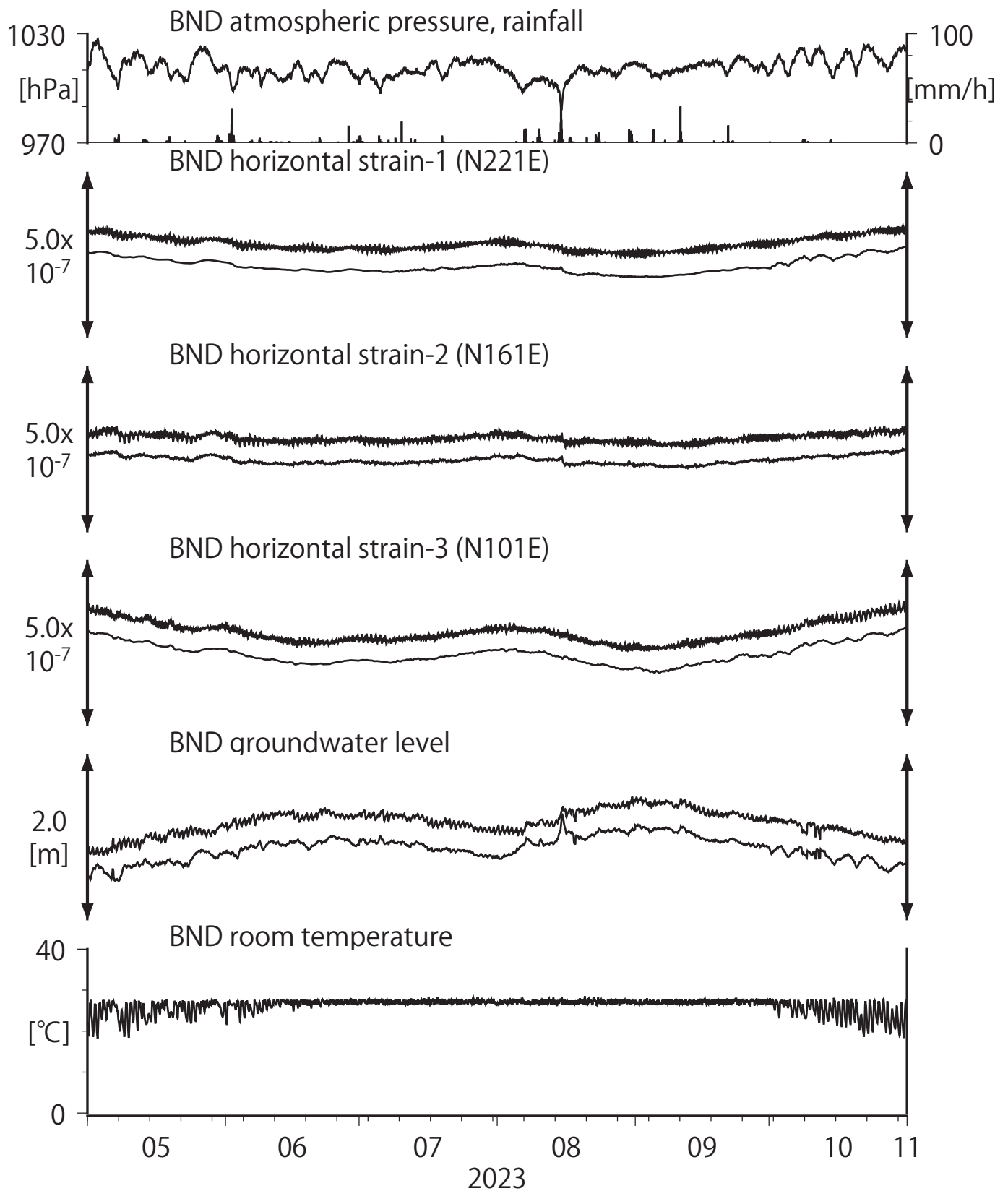
第19図 Crustal strains and groundwater level at BND (時間値) (2023/05/01 00:00 - 2023/11/01 00:00 (JST))
