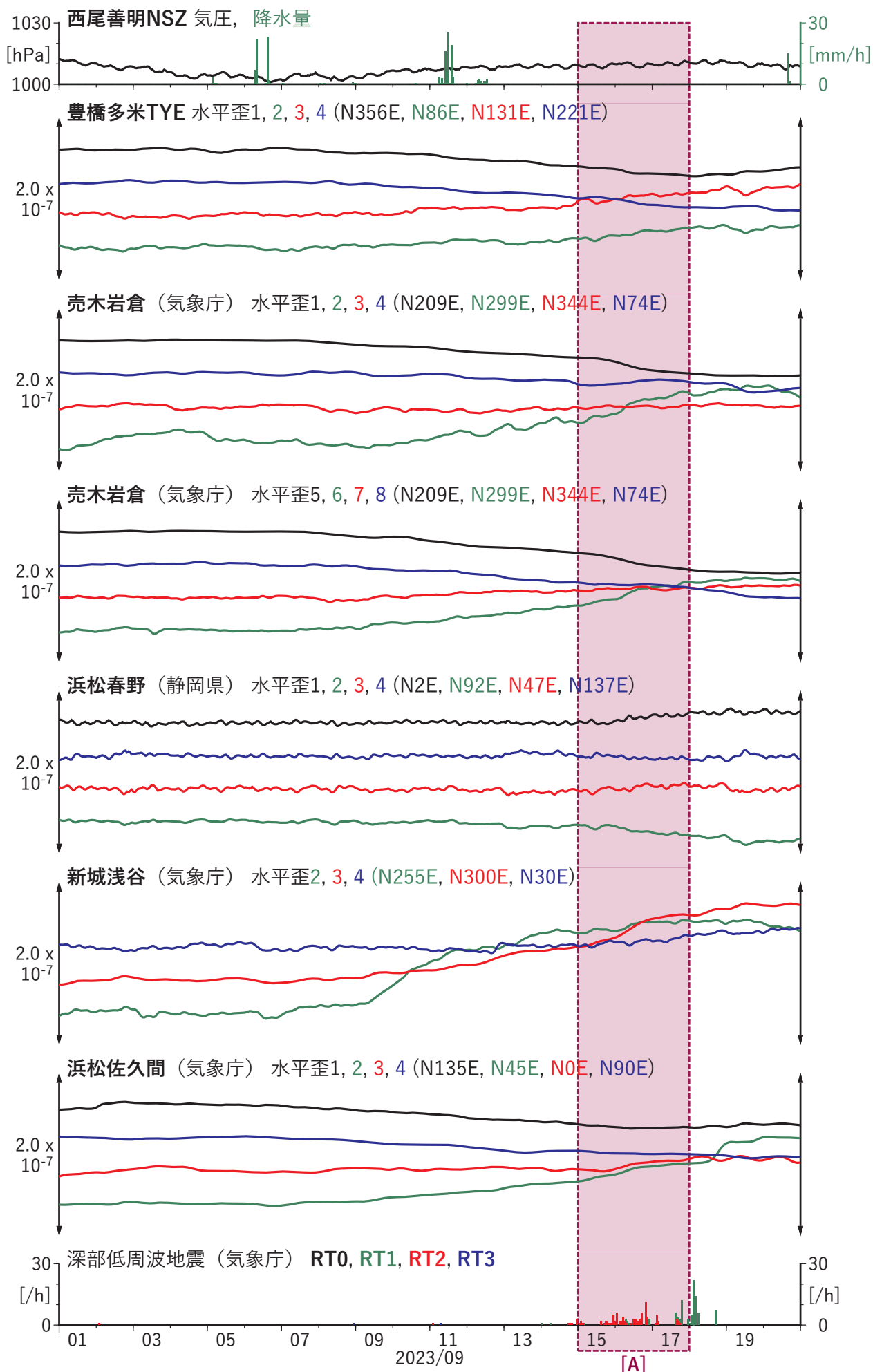
第49図 東海地方における歪の時間変化 (2023/09/01 00:00 - 2023/09/21 00:00 (JST))
