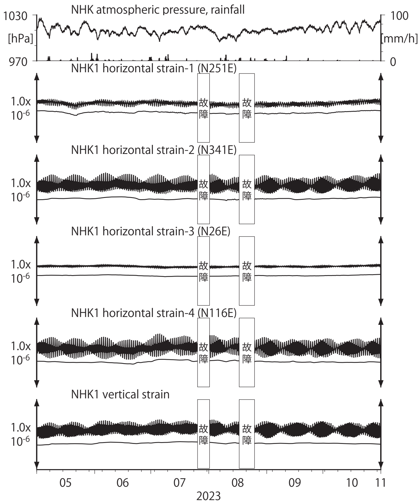
第31図 Crustal strains at NHK (時間値) (2023/05/01 00:00 - 2023/11/01 00:00 (JST))
