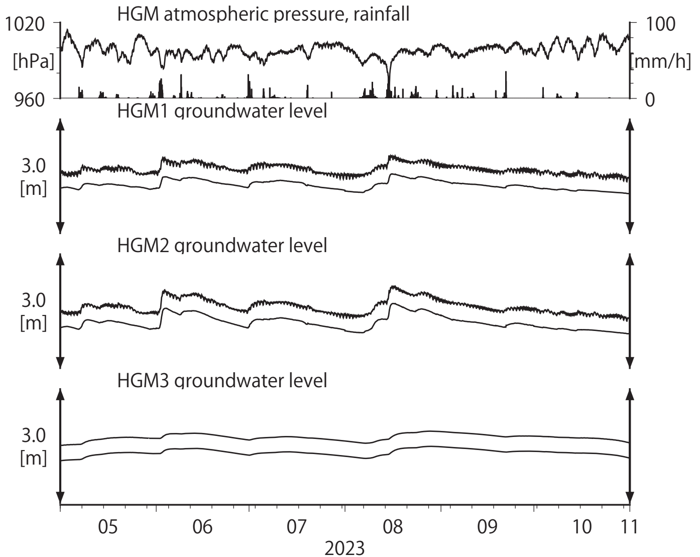
第16図 Tilt and groundwater level at HGM (時間値) (2023/05/01 00:00 - 2023/11/01 00:00 (JST))
