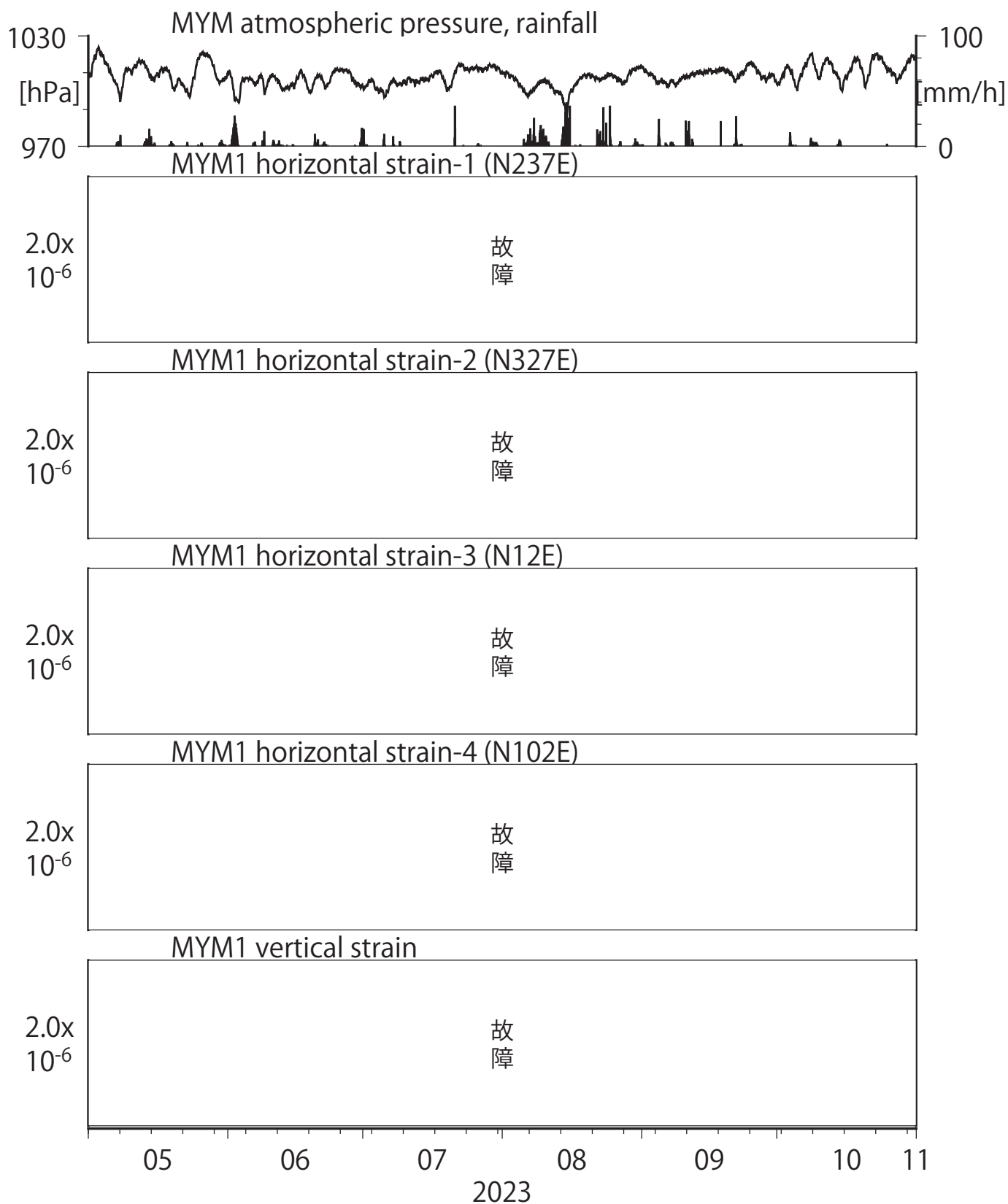
第11図 Crustal strains at MYM (時間値) (2023/05/01 00:00 - 2023/11/01 00:00 (JST))
