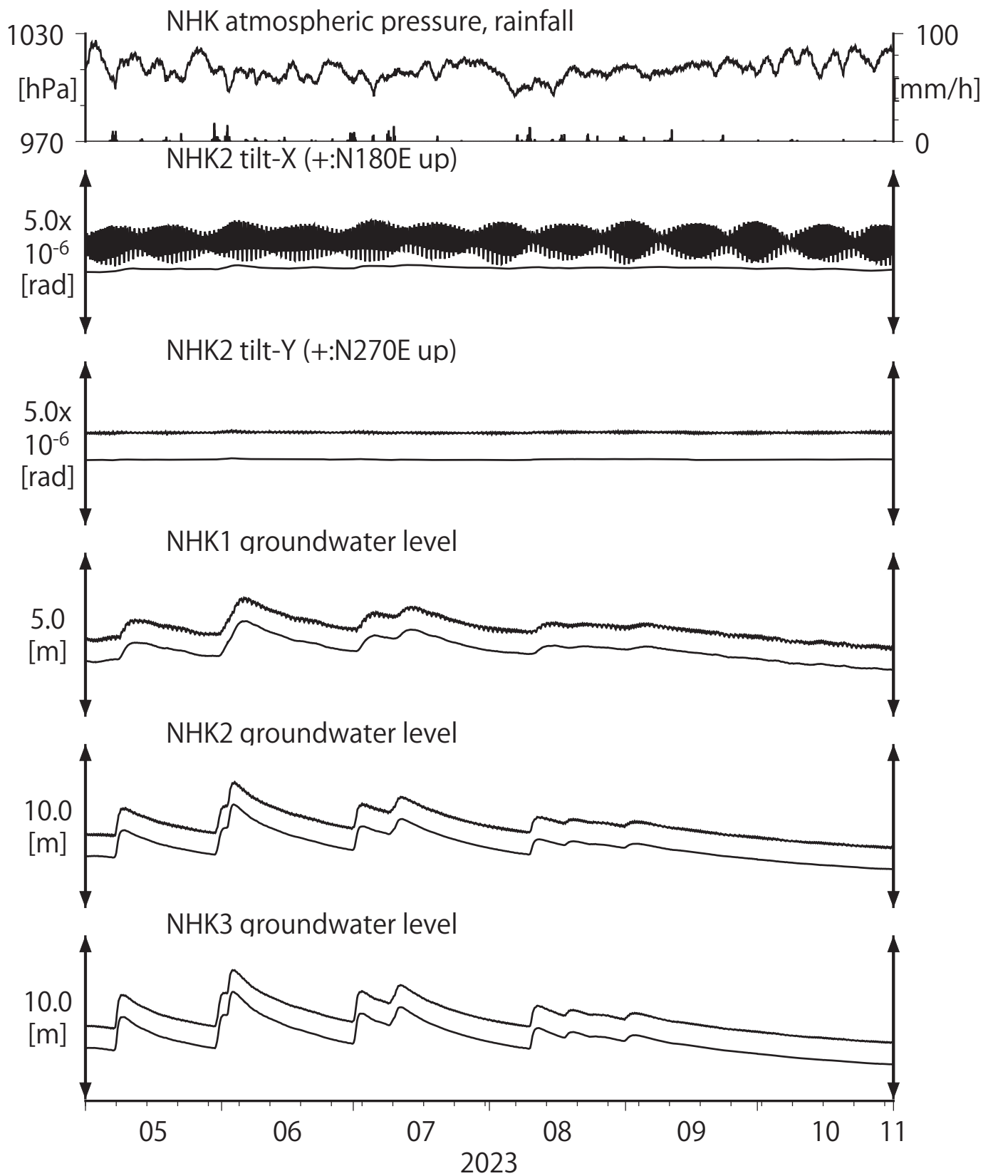
第32図 Tilt and groundwater level at NHK (時間値) (2023/05/01 00:00 - 2023/11/01 00:00 (JST))
