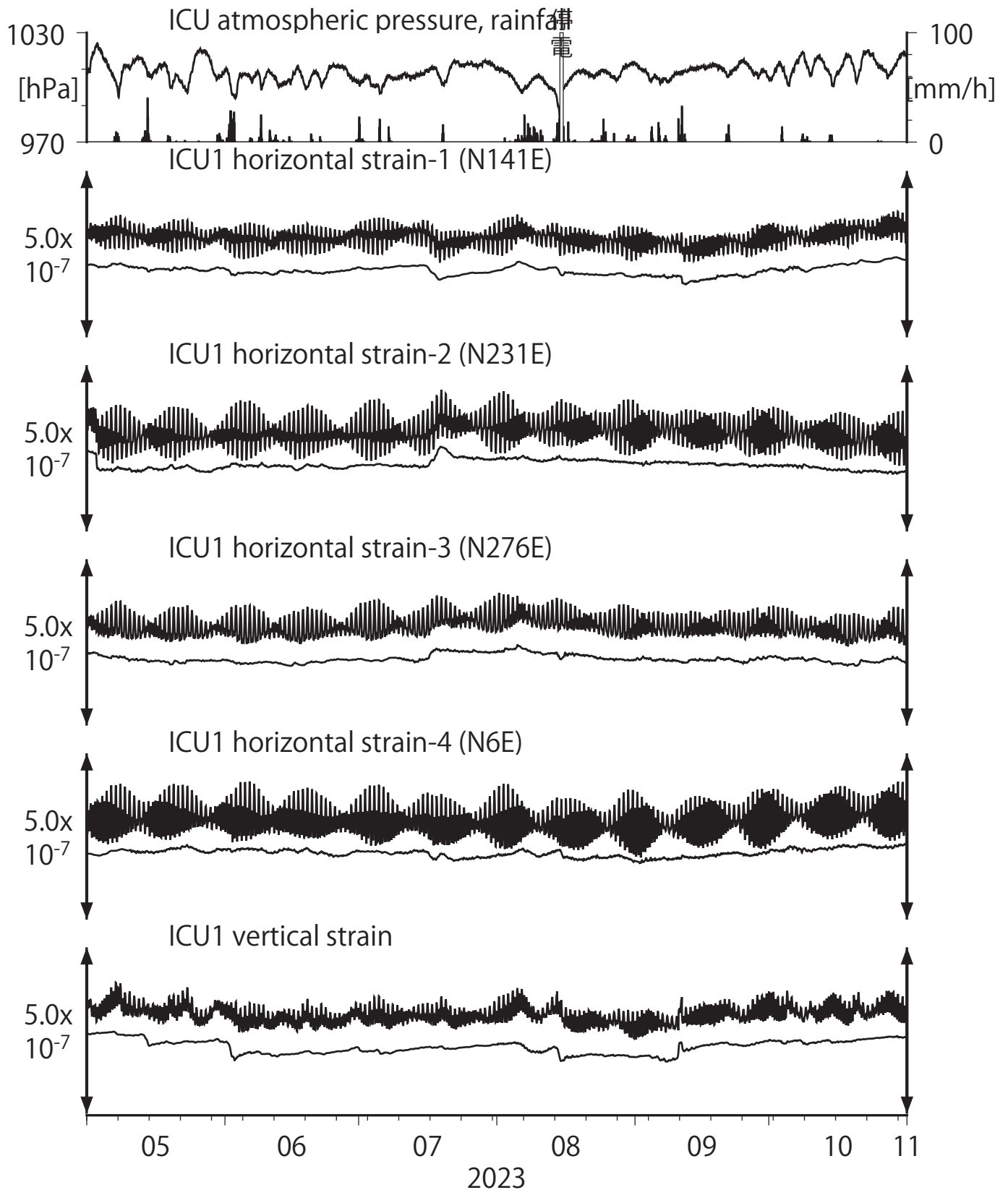
第13図 Crustal strains at ICU (時間値) (2023/05/01 00:00 - 2023/11/01 00:00 (JST))
