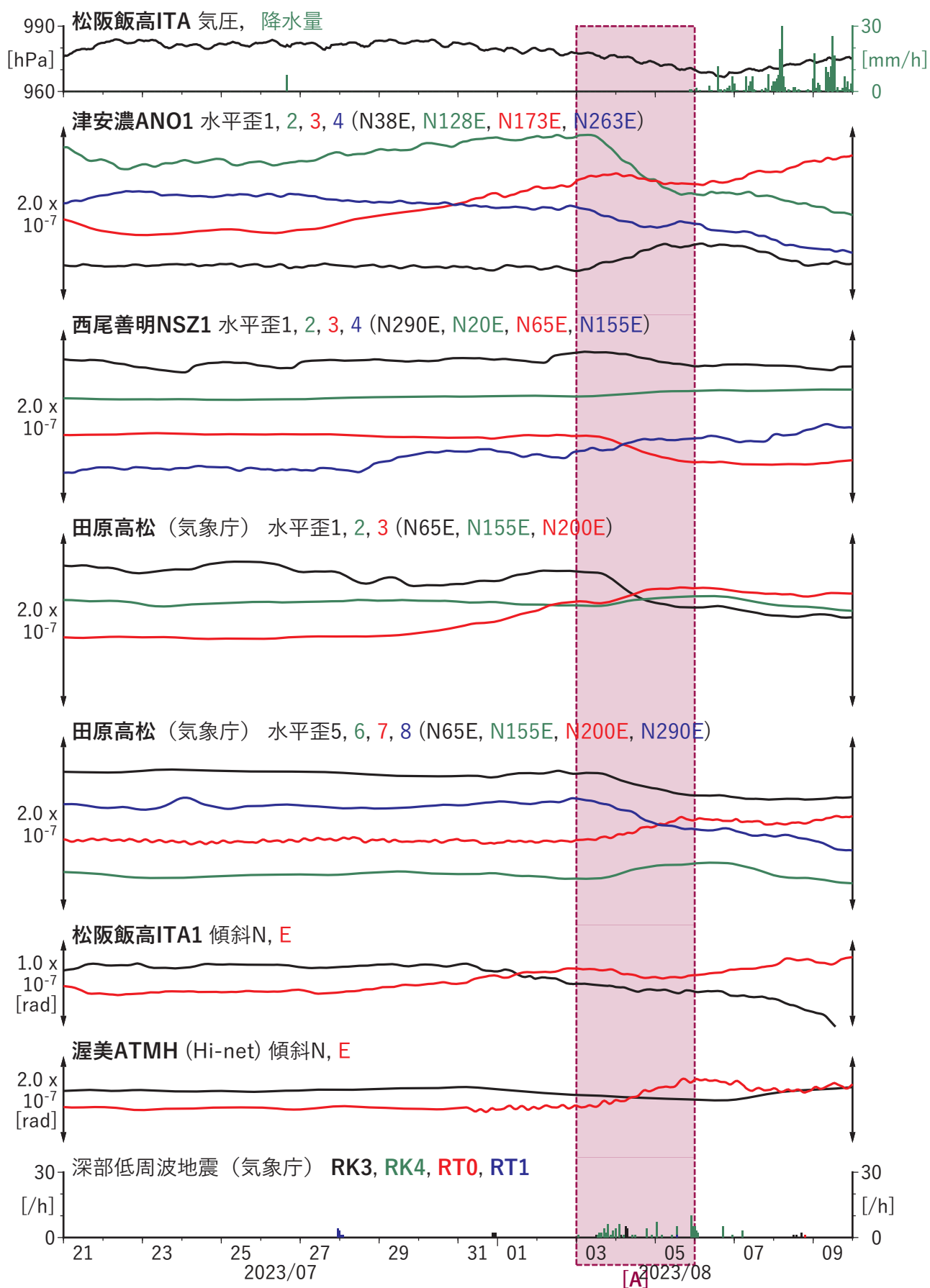
第34図 紀伊半島から東海地方における歪・傾斜の時間変化 (2023/07/21 00:00 - 2023/08/10 00:00 (JST))
