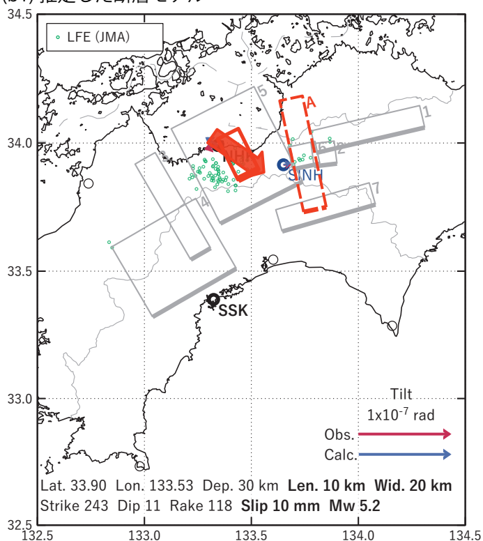
第47図 2023/09/15 - 16AM の歪・傾斜変化（第45図 [B]）を説明する断層モデル。
