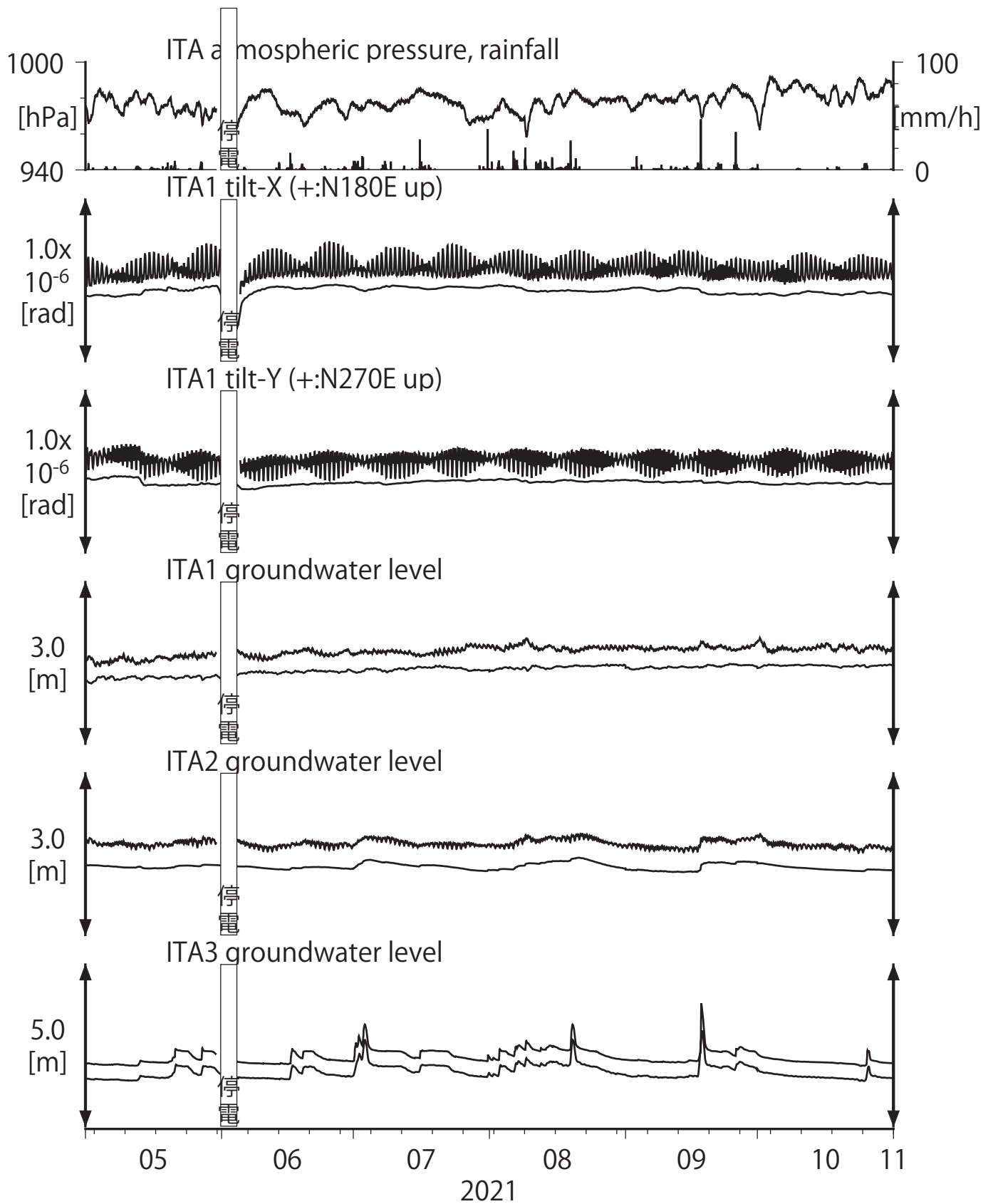
第11図 Tilt and groundwater level at ITA (時間値) (2021/05/01 00:00 - 2021/11/01 00:00 (JST))
