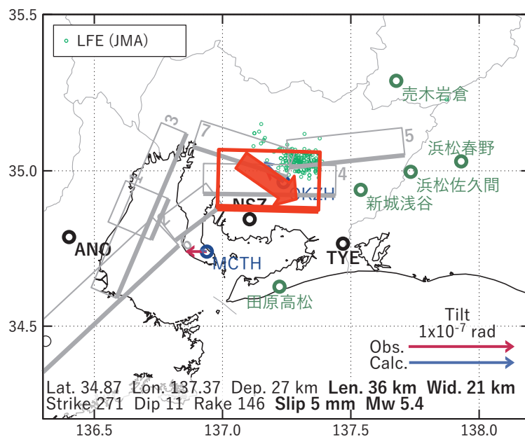
第40図 2021/09/21-22 の歪・傾斜変化 (図2, 3[A]) を説明する断層モデル。
