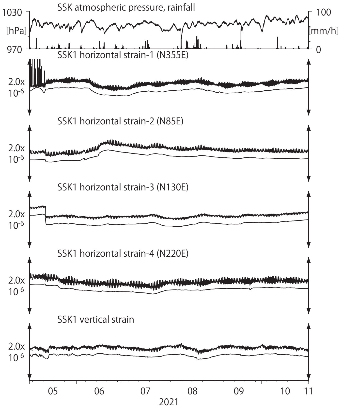
第27図 Crustal strains at SSK (時間値) (2021/05/01 00:00 - 2021/11/01 00:00 (JST))
