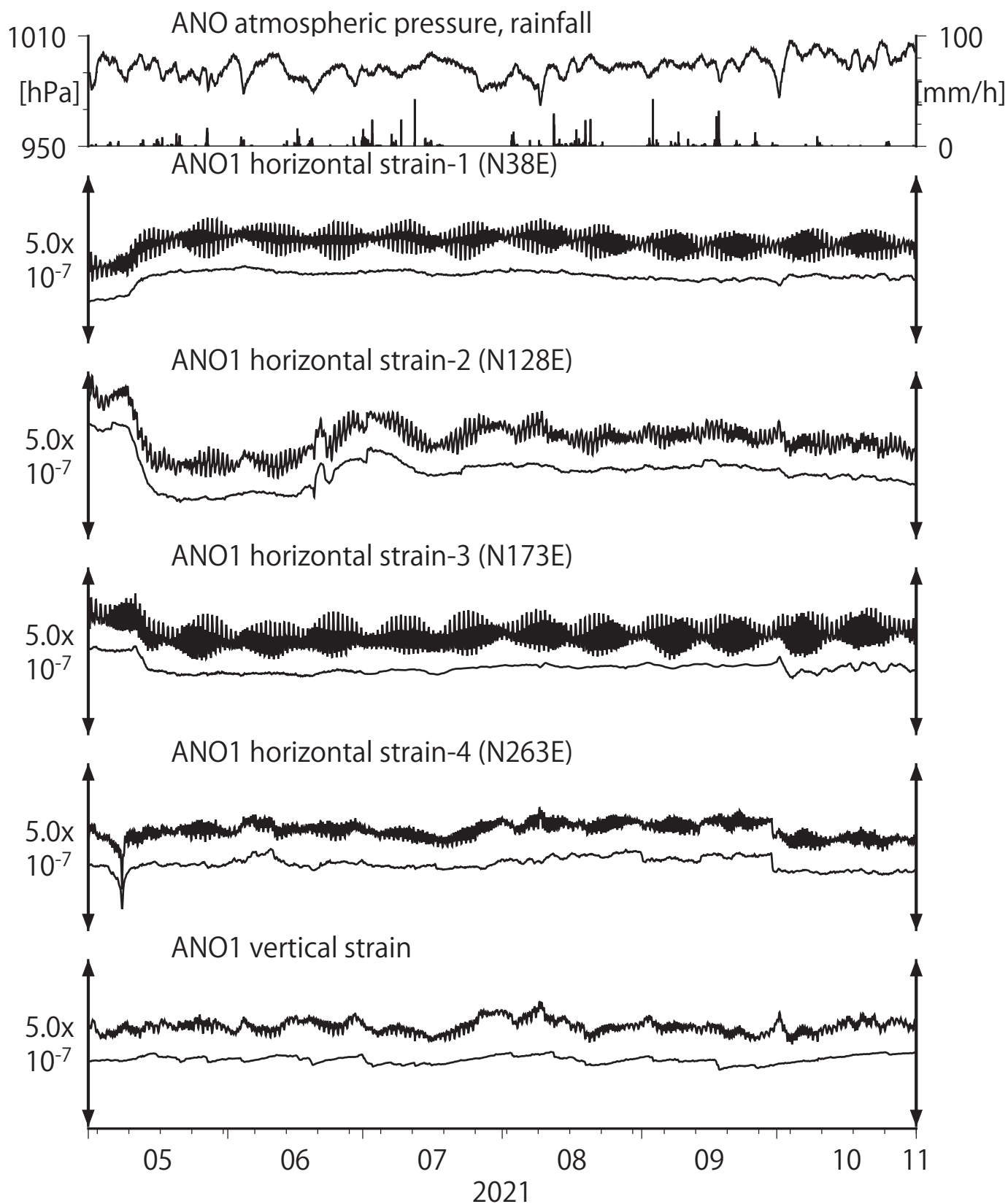
第8図 Crustal strains at ANO (時間値) (2021/05/01 00:00 - 2021/11/01 00:00 (JST))
