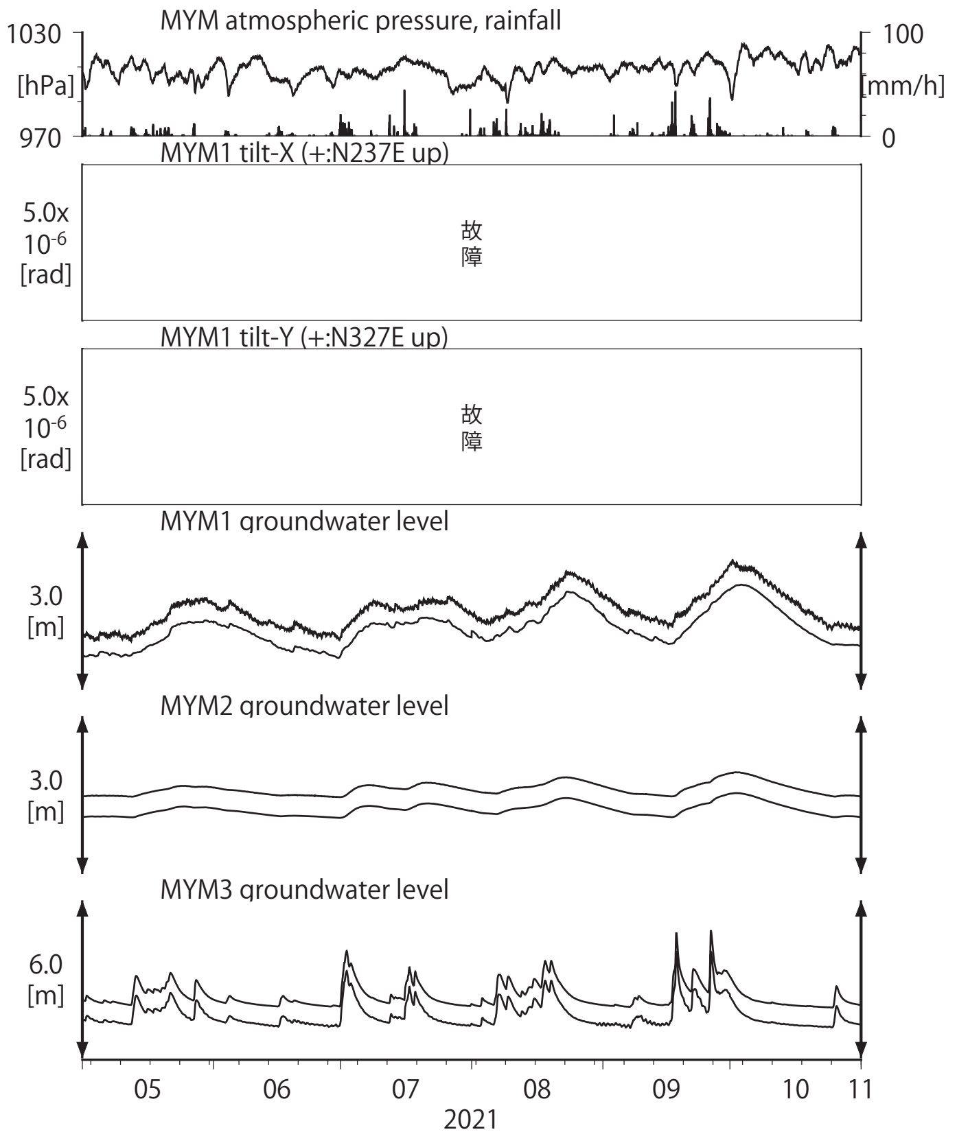
第13図 Tilt and groundwater level at MYM (時間値) (2021/05/01 00:00 - 2021/11/01 00:00 (JST))
