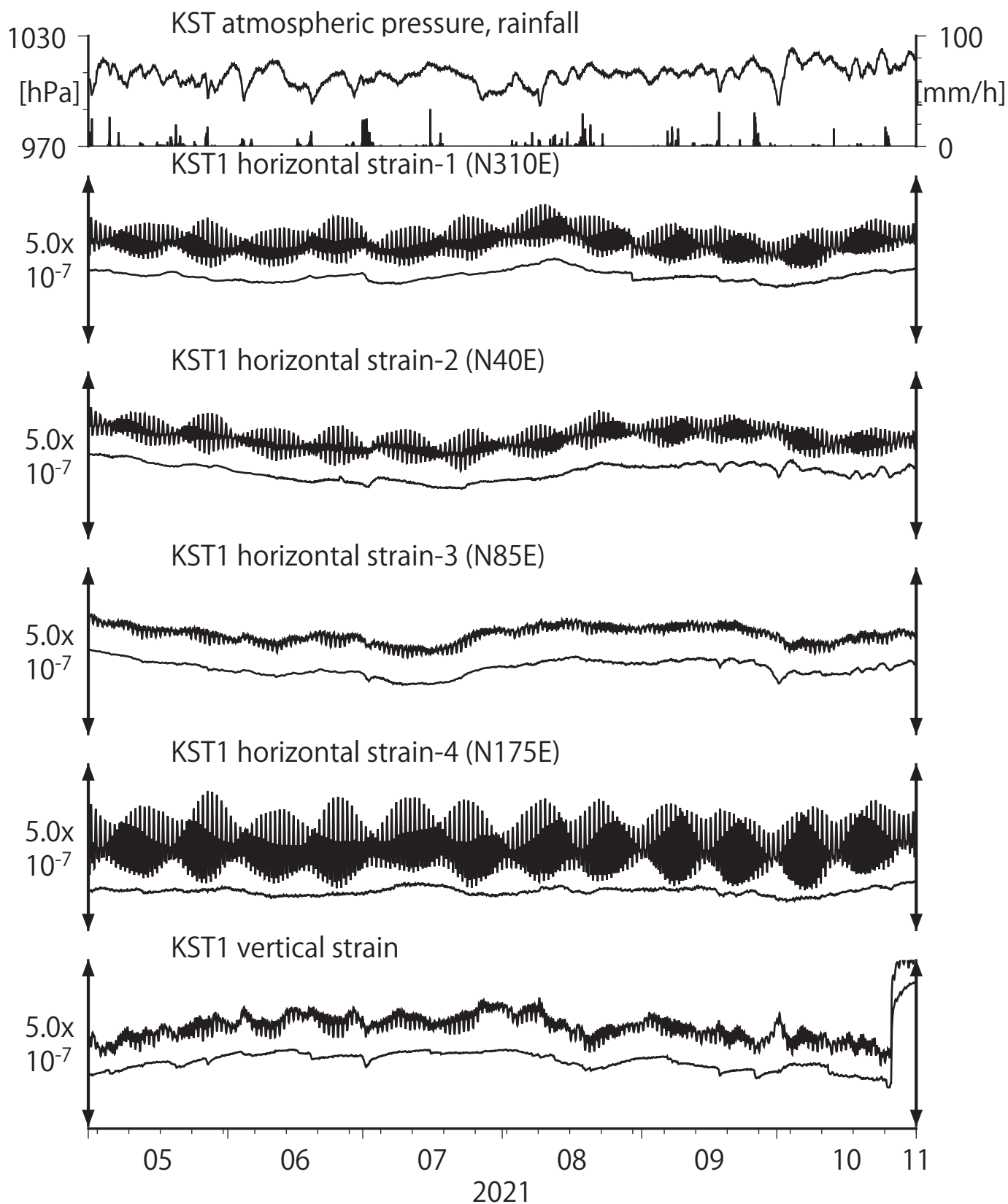
第18図 Crustal strains at KST (時間値) (2021/05/01 00:00 - 2021/11/01 00:00 (JST))
