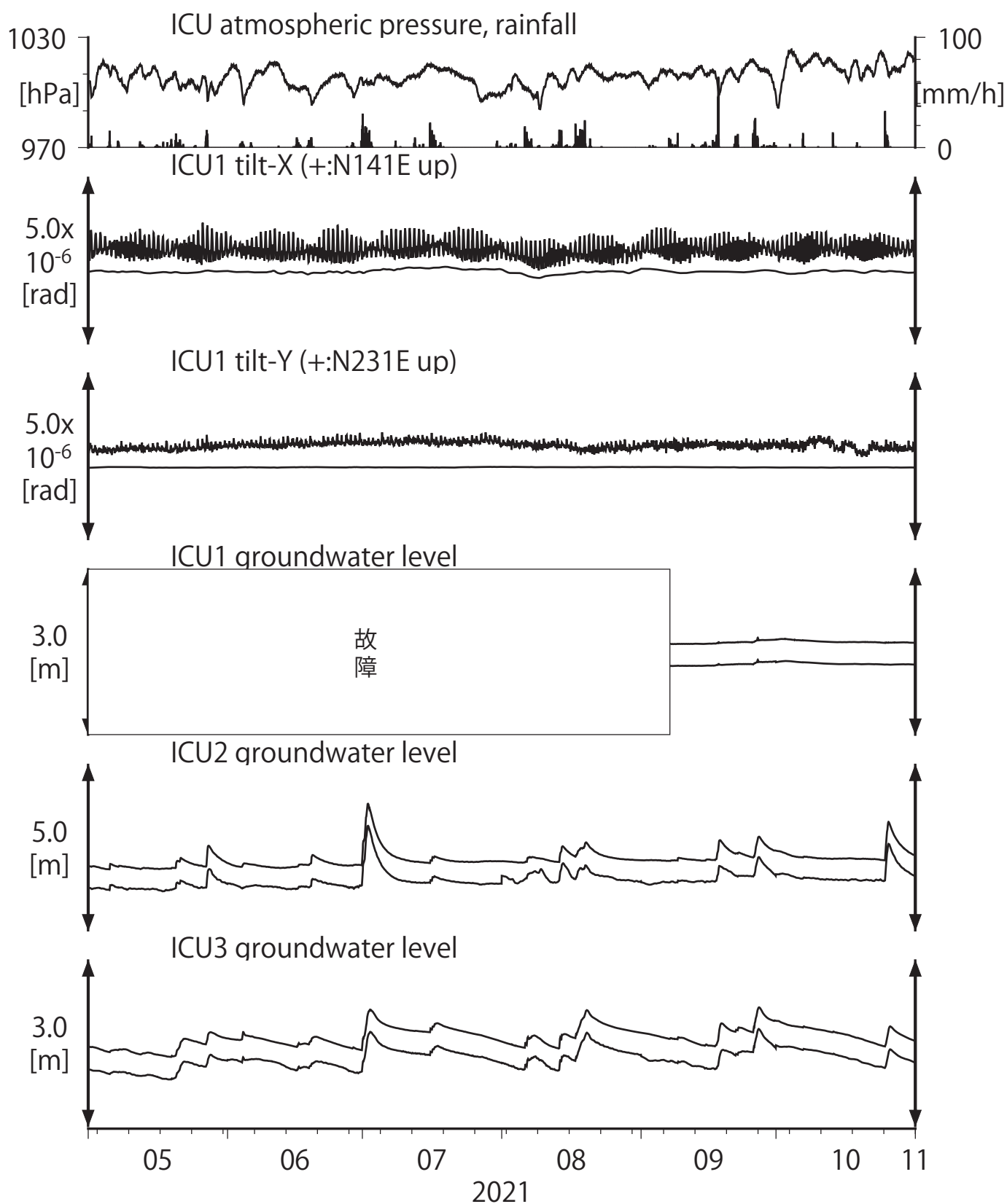
第15図 Tilt and groundwater level at ICU (時間値) (2021/05/01 00:00 - 2021/11/01 00:00 (JST))
