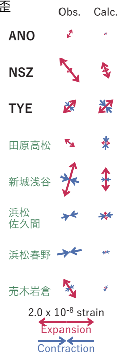
第40図 2021/09/21-22 の歪・傾斜変化 (図2, 3[A]) を説明する断層モデル。
