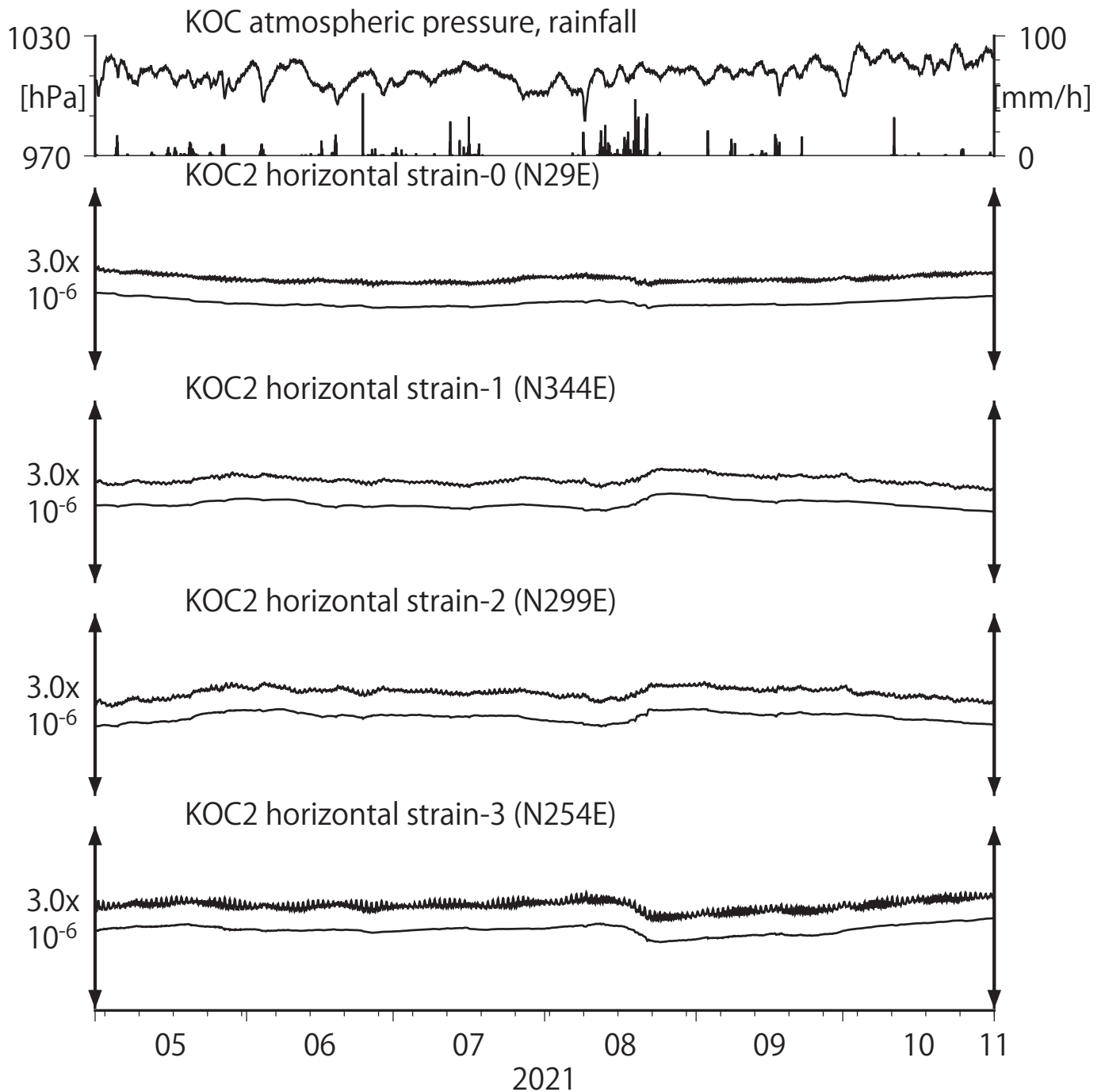
第25図 Crustal strains at KOC (時間値) (2021/05/01 00:00 - 2021/11/01 00:00 (JST))
