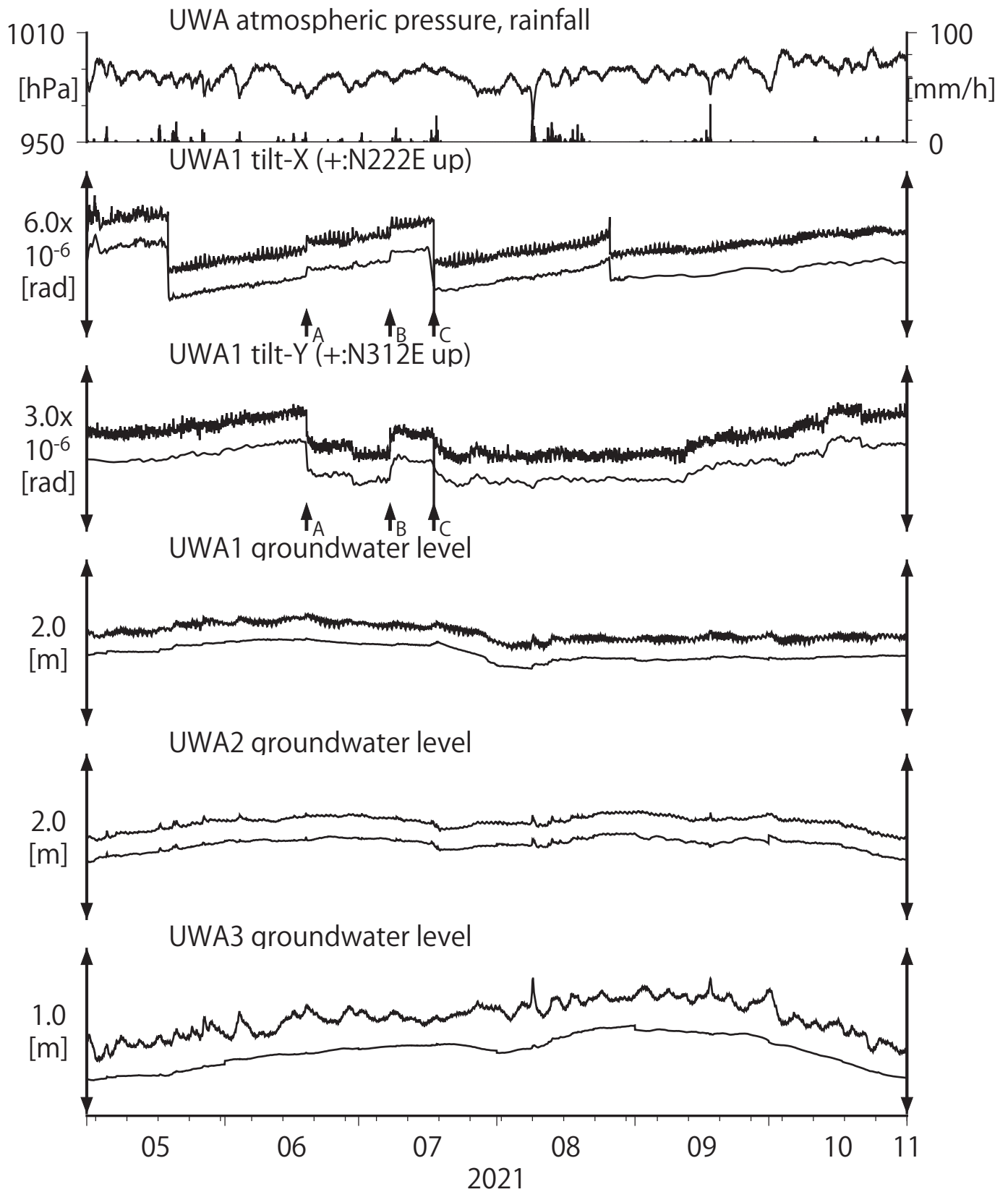
第32図 Tilt and groundwater level at UWA (時間値) (2021/05/01 00:00 - 2021/11/01 00:00 (JST))
