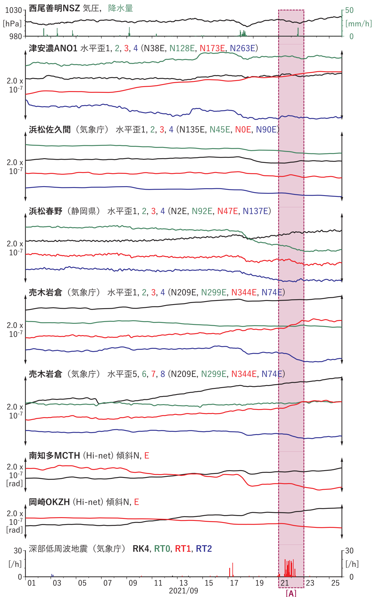
第39図 歪・傾斜の時間変化 (2021/09/01 00:00 - 2021/09/26 00:00 (JST))
