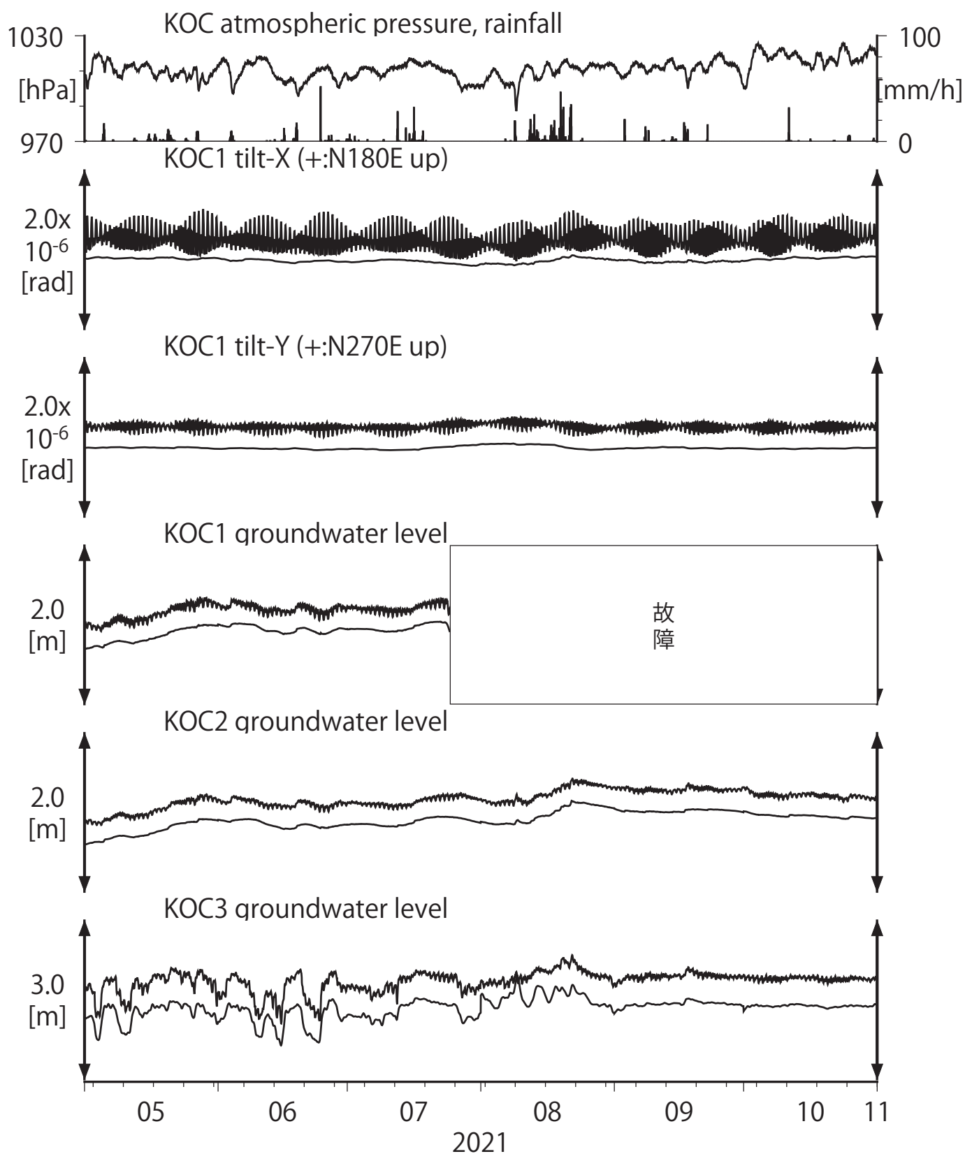
第26図 Tilt and groundwater level at KOC (時間値) (2021/05/01 00:00 - 2021/11/01 00:00 (JST))
