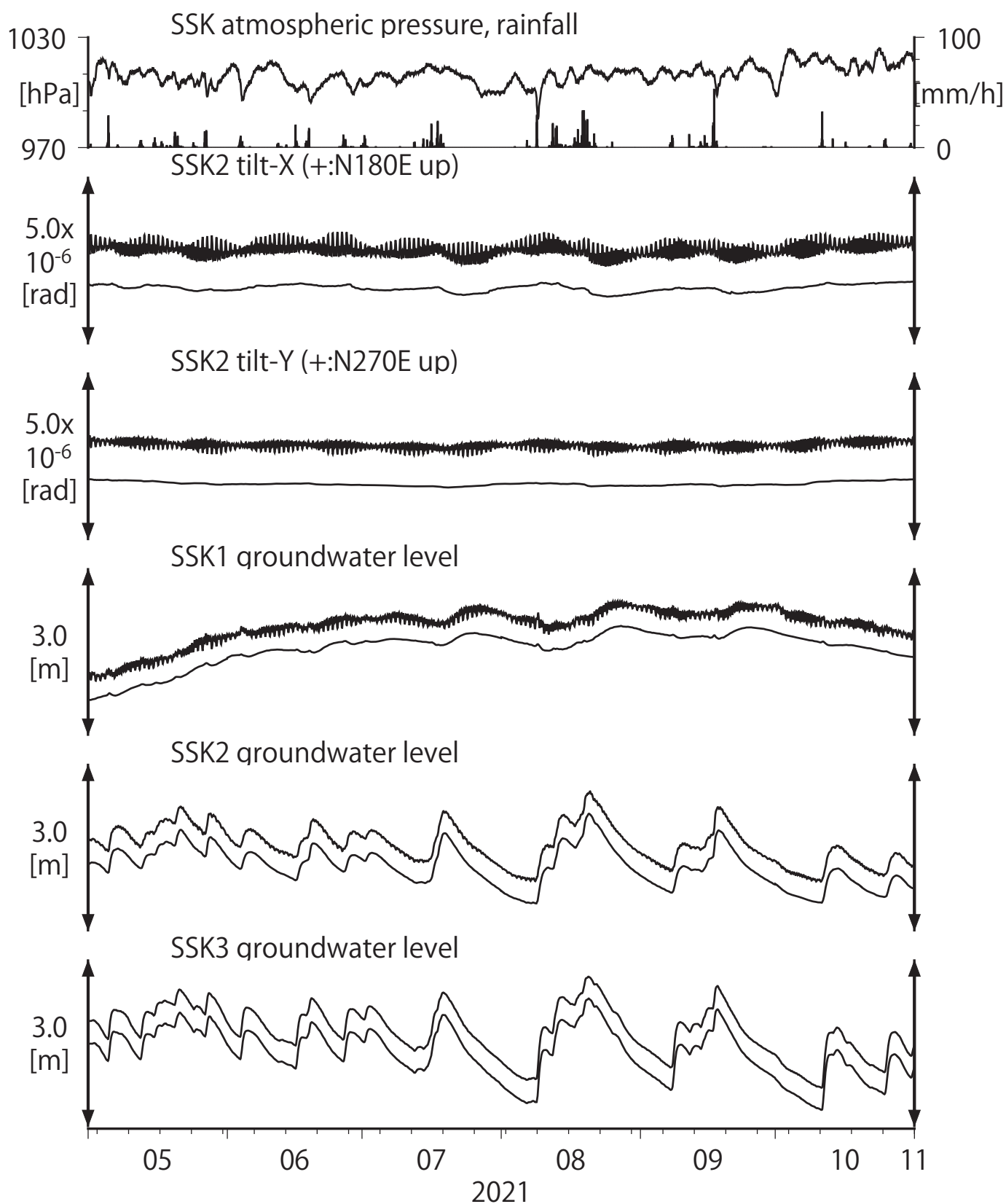
第28図 Tilt and groundwater level at SSK (時間値) (2021/05/01 00:00 - 2021/11/01 00:00 (JST))
