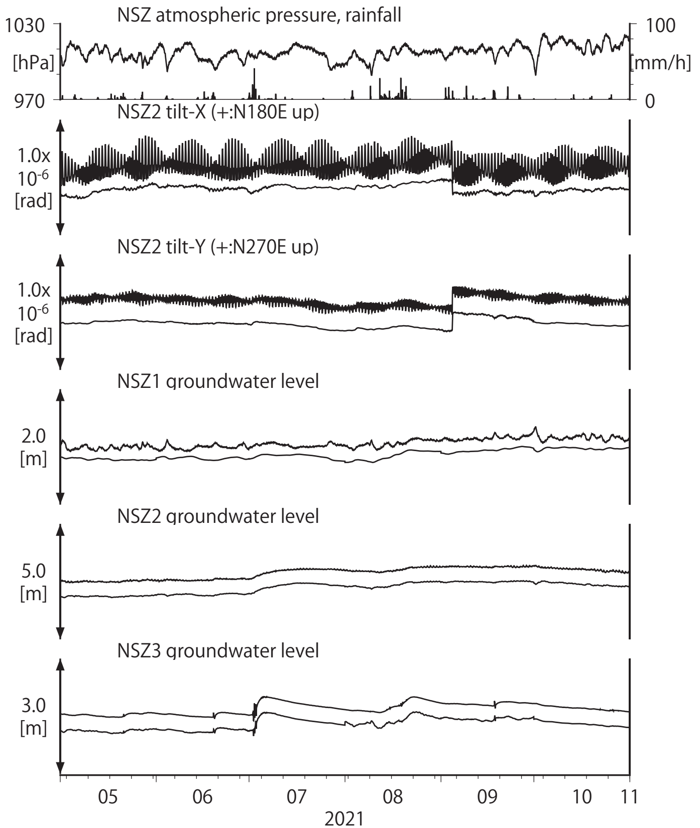
第5図 Tilt and groundwater level at NSZ (時間値) (2021/05/01 00:00 - 2021/11/01 00:00 (JST))
