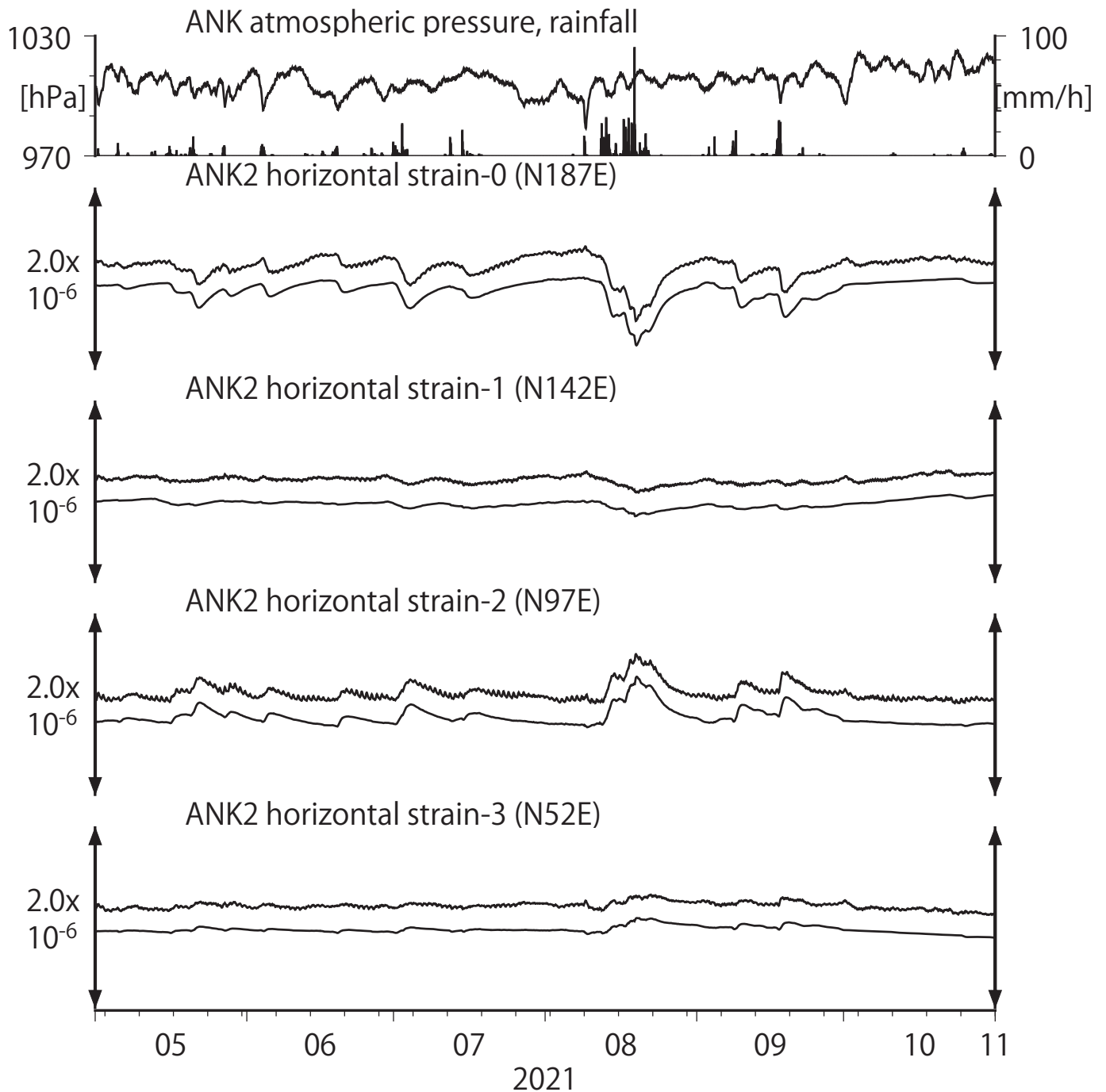
第21図 Crustal strains at ANK (時間値) (2021/05/01 00:00 - 2021/11/01 00:00 (JST))
