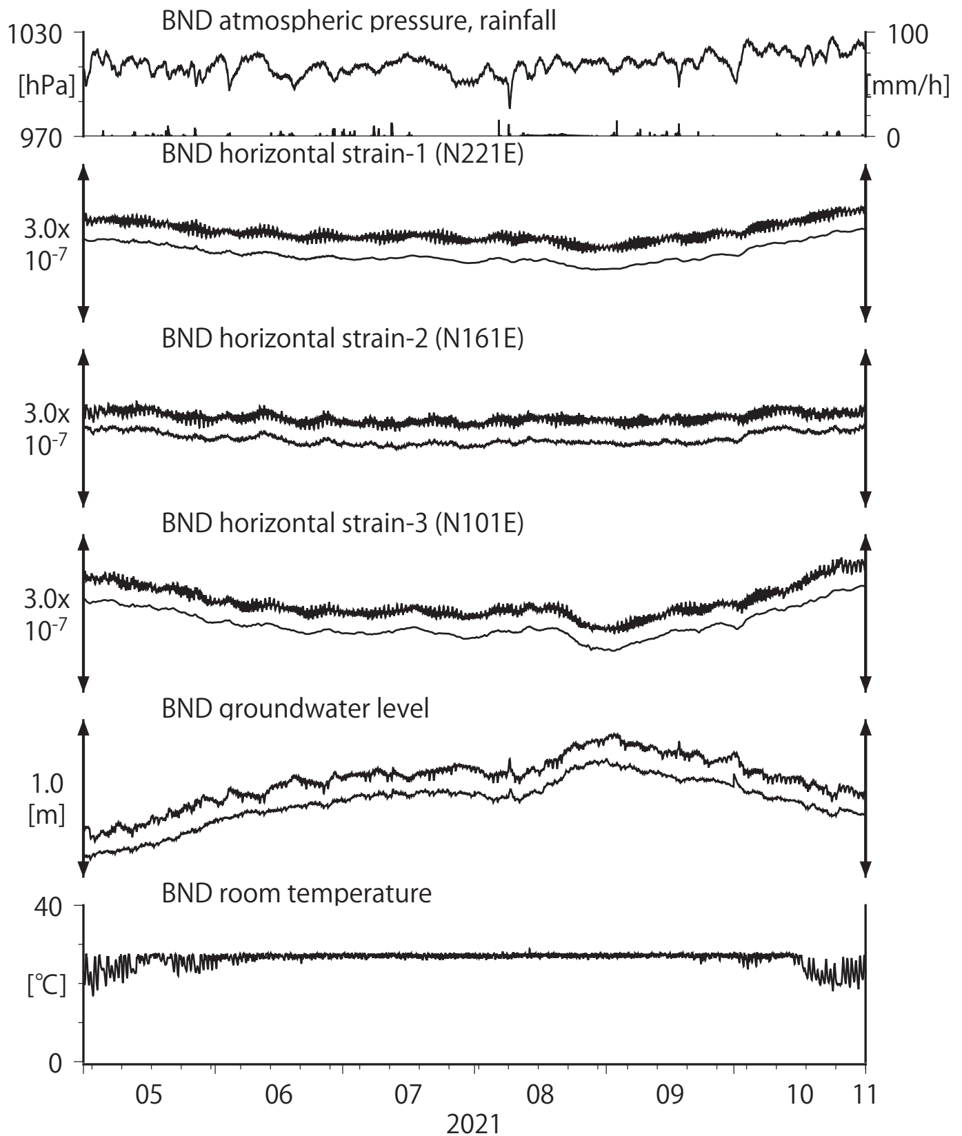
第20図 Crustal strains and groundwater level at BND (時間値) (2021/05/01 00:00 - 2021/11/01 00:00 (JST))
