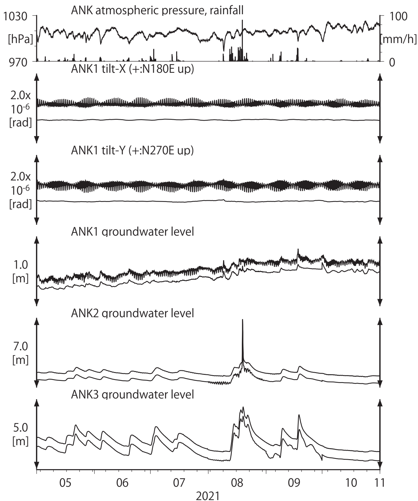
第22図 Tilt and groundwater level at ANK (時間値) (2021/05/01 00:00 - 2021/11/01 00:00 (JST))
