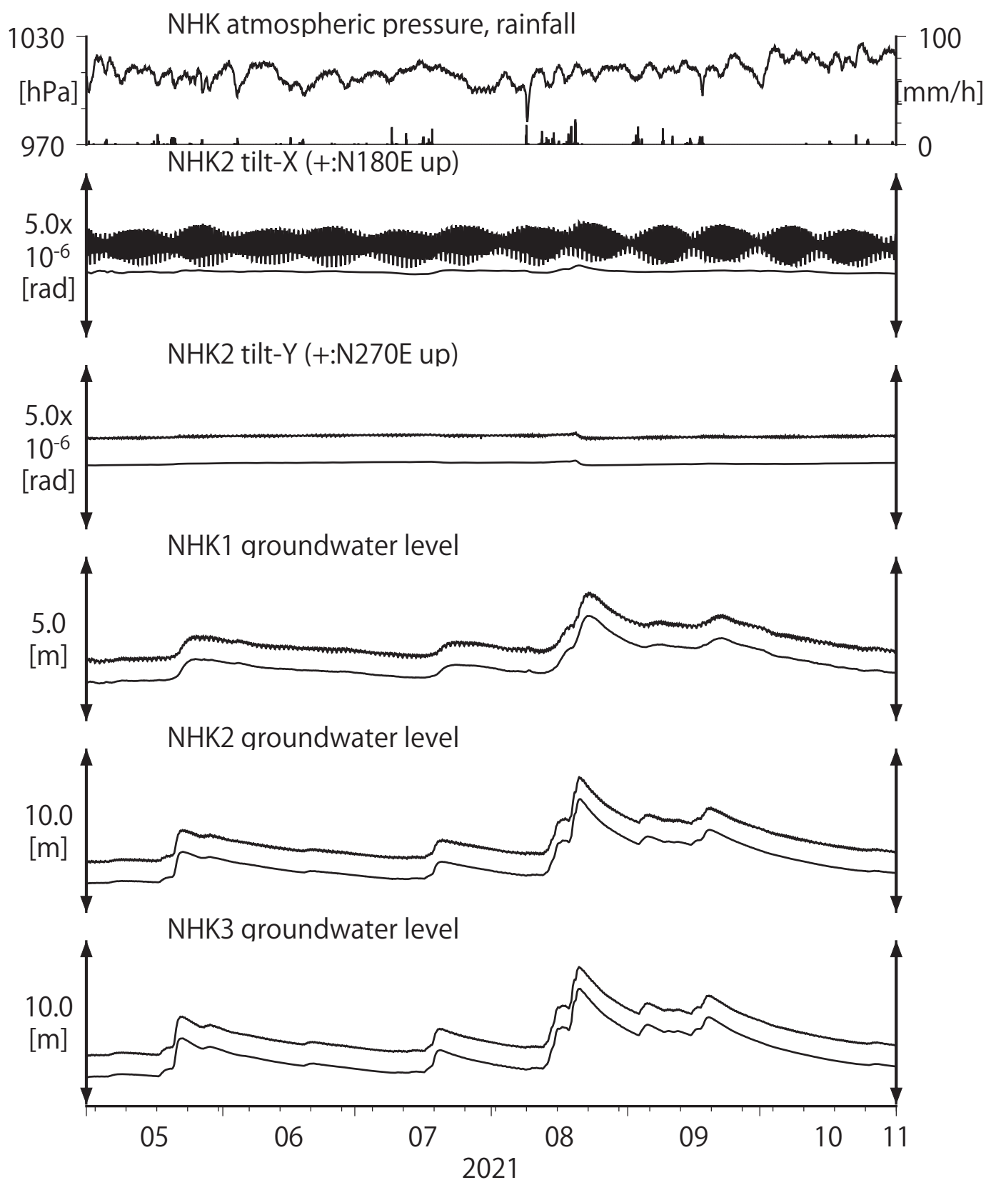
第36図 Tilt and groundwater level at NHK (時間値) (2021/05/01 00:00 - 2021/11/01 00:00 (JST))
