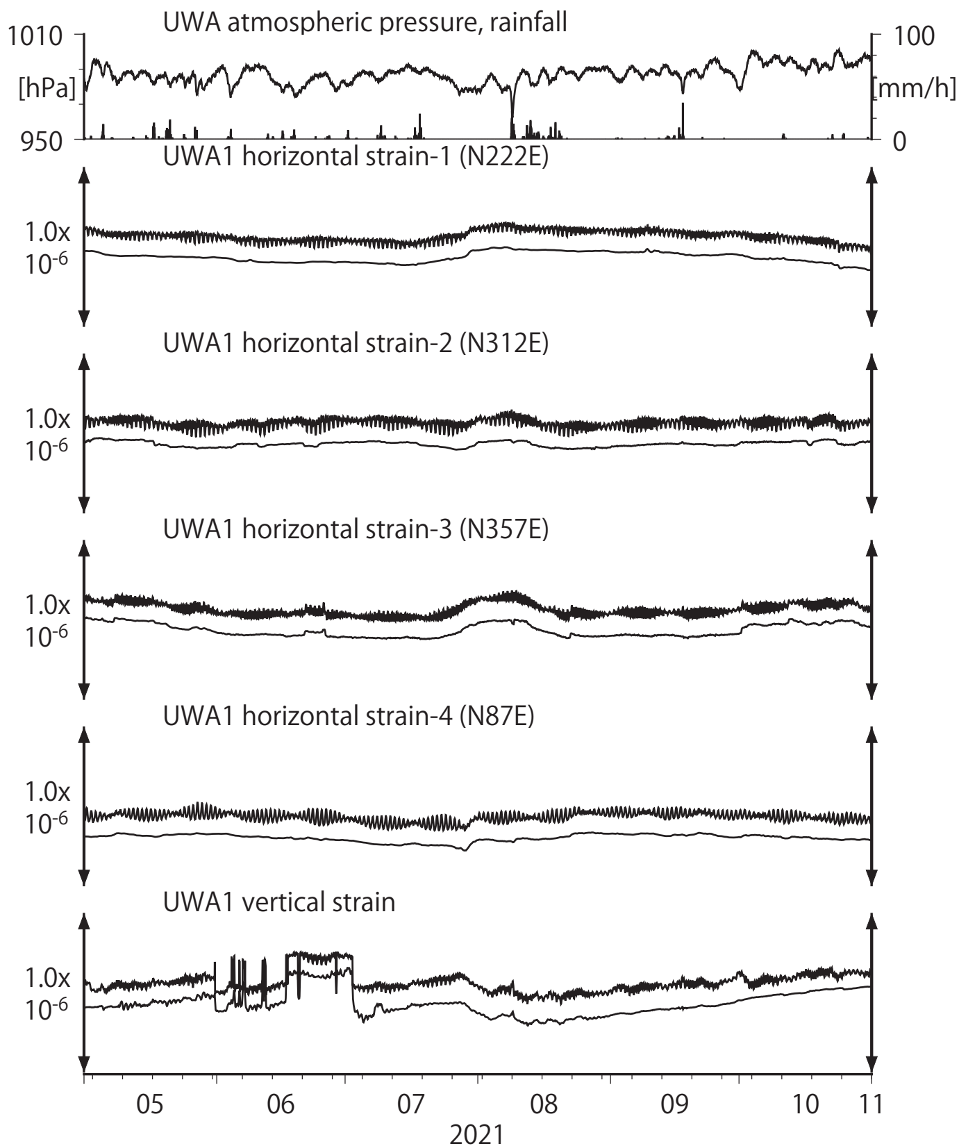
第31図 Crustal strains at UWA (時間値) (2021/05/01 00:00 - 2021/11/01 00:00 (JST))
