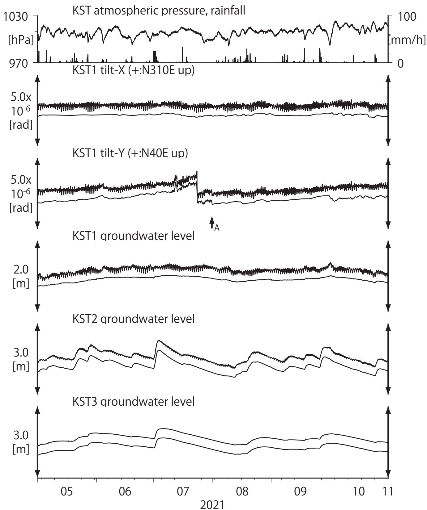
第19図 Tilt and groundwater level at KST (時間値) (2021/05/01 00:00 - 2021/11/01 00:00 (JST))
