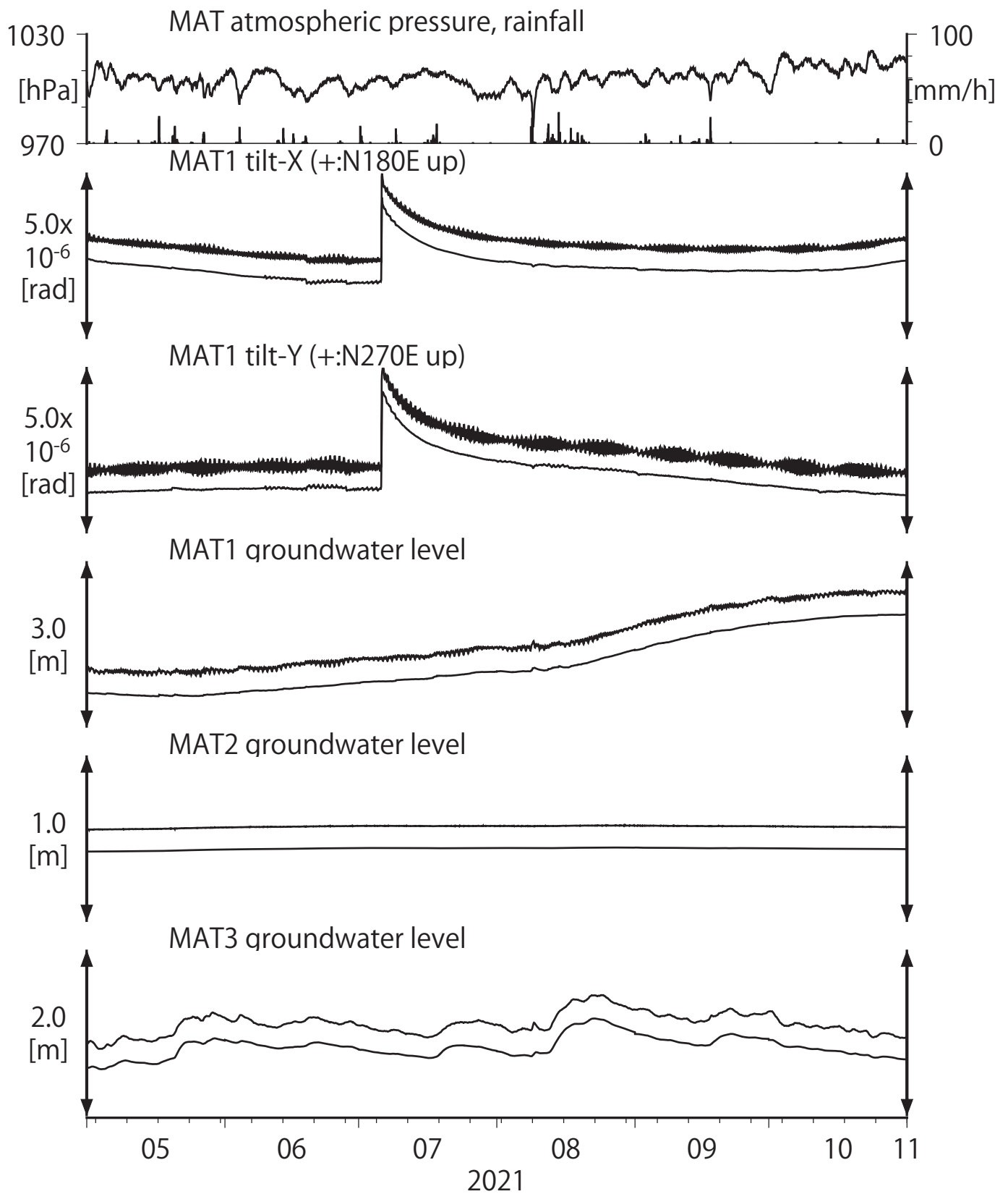
第34図 Tilt and groundwater level at MAT (時間値) (2021/05/01 00:00 - 2021/11/01 00:00 (JST))
