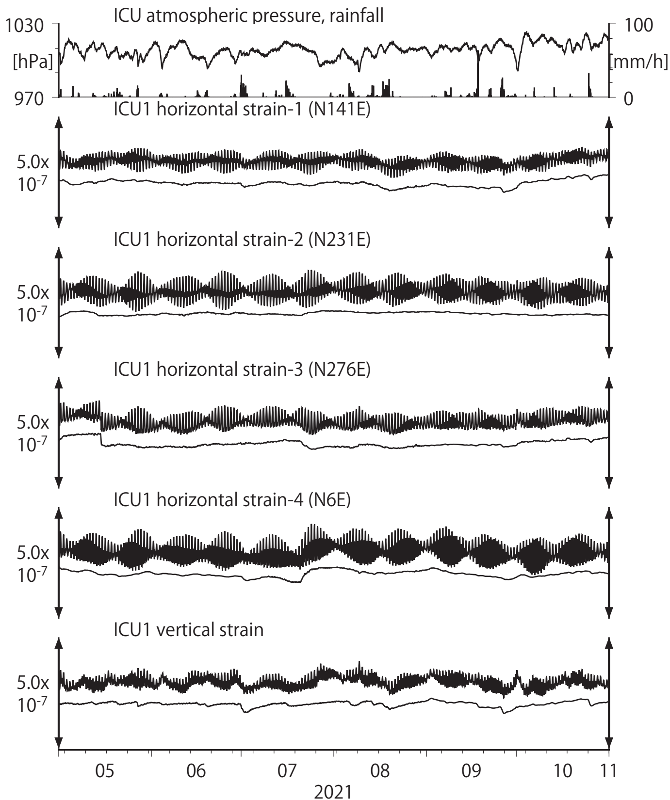
第14図 Crustal strains at ICU (時間値) (2021/05/01 00:00 - 2021/11/01 00:00 (JST))
