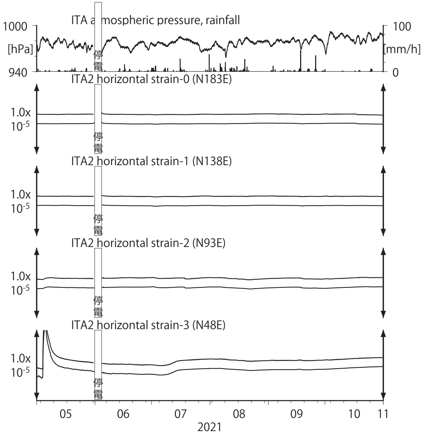
第10図 Crustal strains at ITA (時間値) (2021/05/01 00:00 - 2021/11/01 00:00 (JST))
