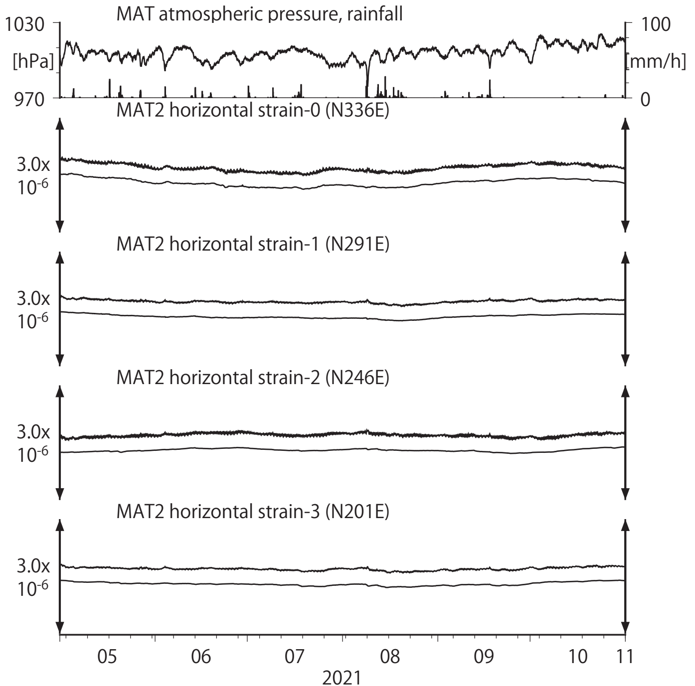
第33図 Crustal strains at MAT (時間値) (2021/05/01 00:00 - 2021/11/01 00:00 (JST))
