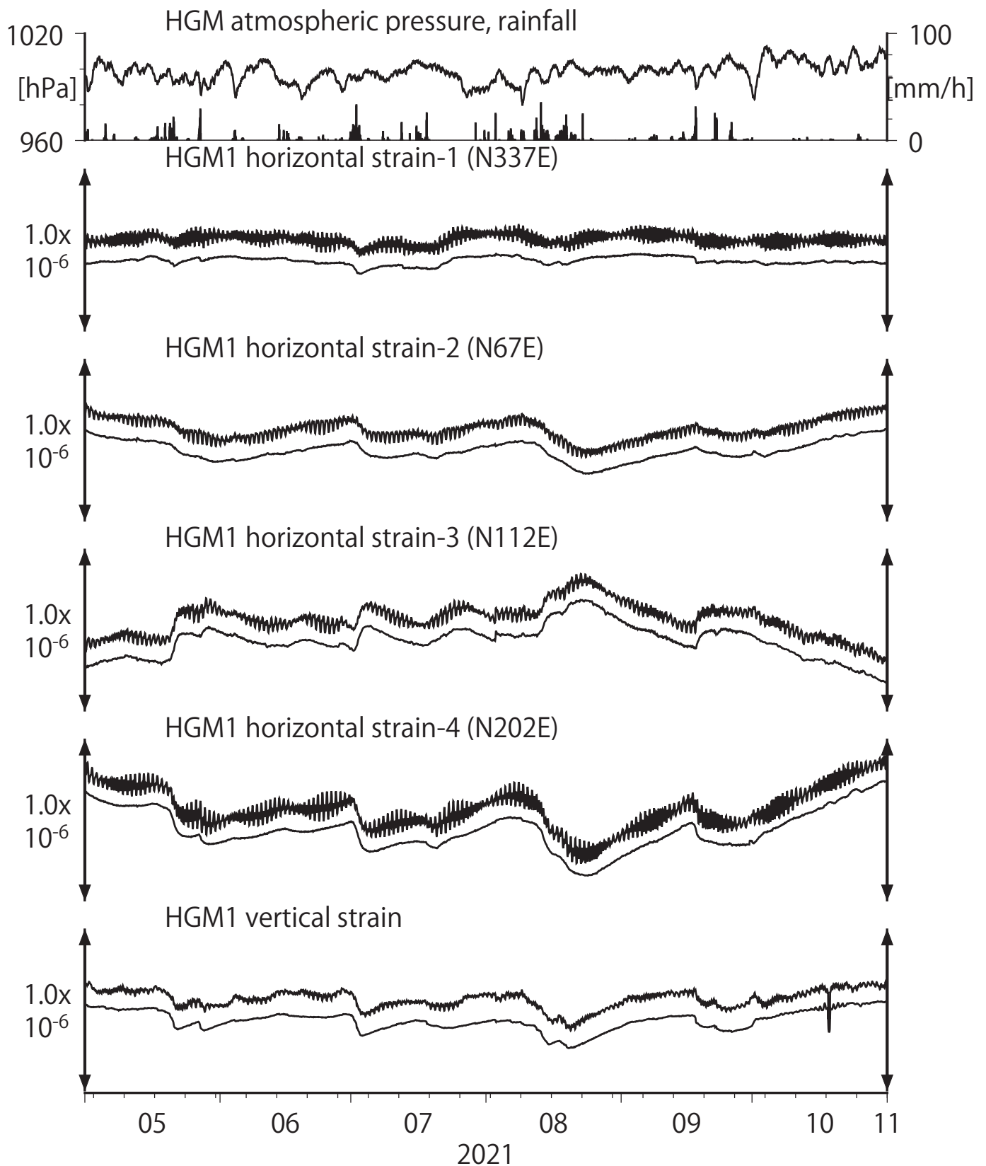
第16図 Crustal strains at HGM (時間値) (2021/05/01 00:00 - 2021/11/01 00:00 (JST))
