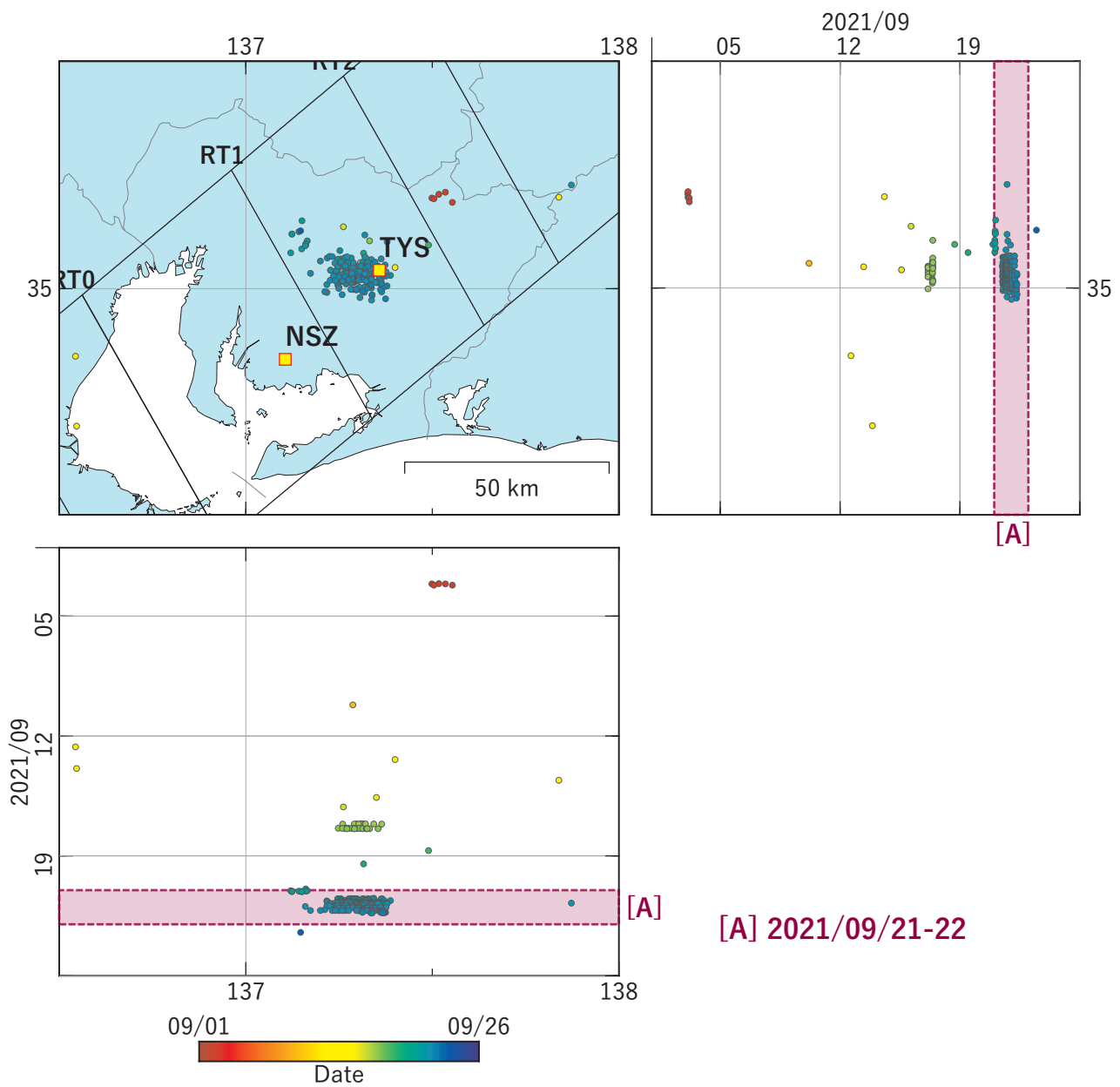
第37図 東海地方における深部低周波地震の時空間分布図。 (2021/09/01 00:00 - 2021/09/26 00:00 (JST)) 気象庁カタログによる。
