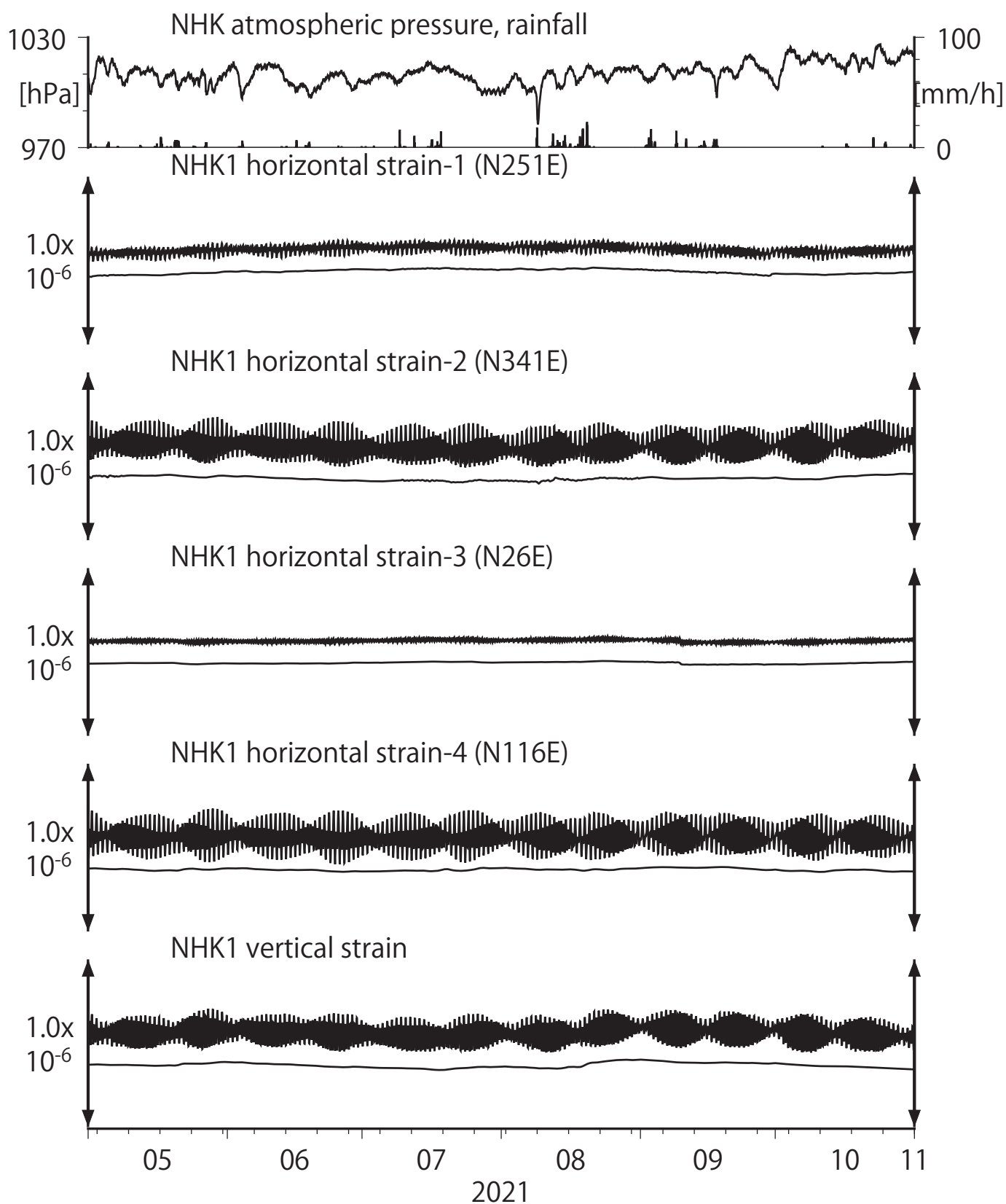
第35図 Crustal strains at NHK (時間値) (2021/05/01 00:00 - 2021/11/01 00:00 (JST))
