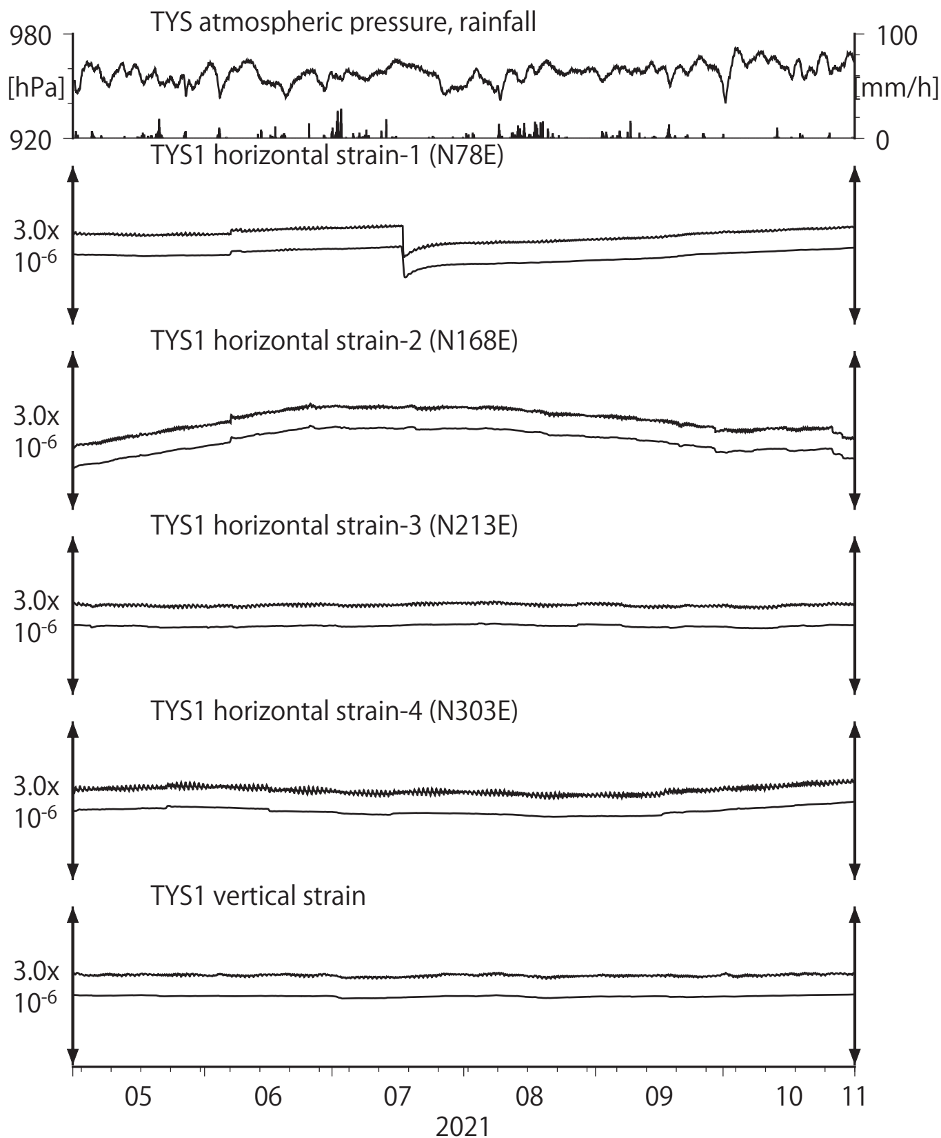
第2図 Crustal strains at TYS (時間値) (2021/05/01 00:00 - 2021/11/01 00:00 (JST))
