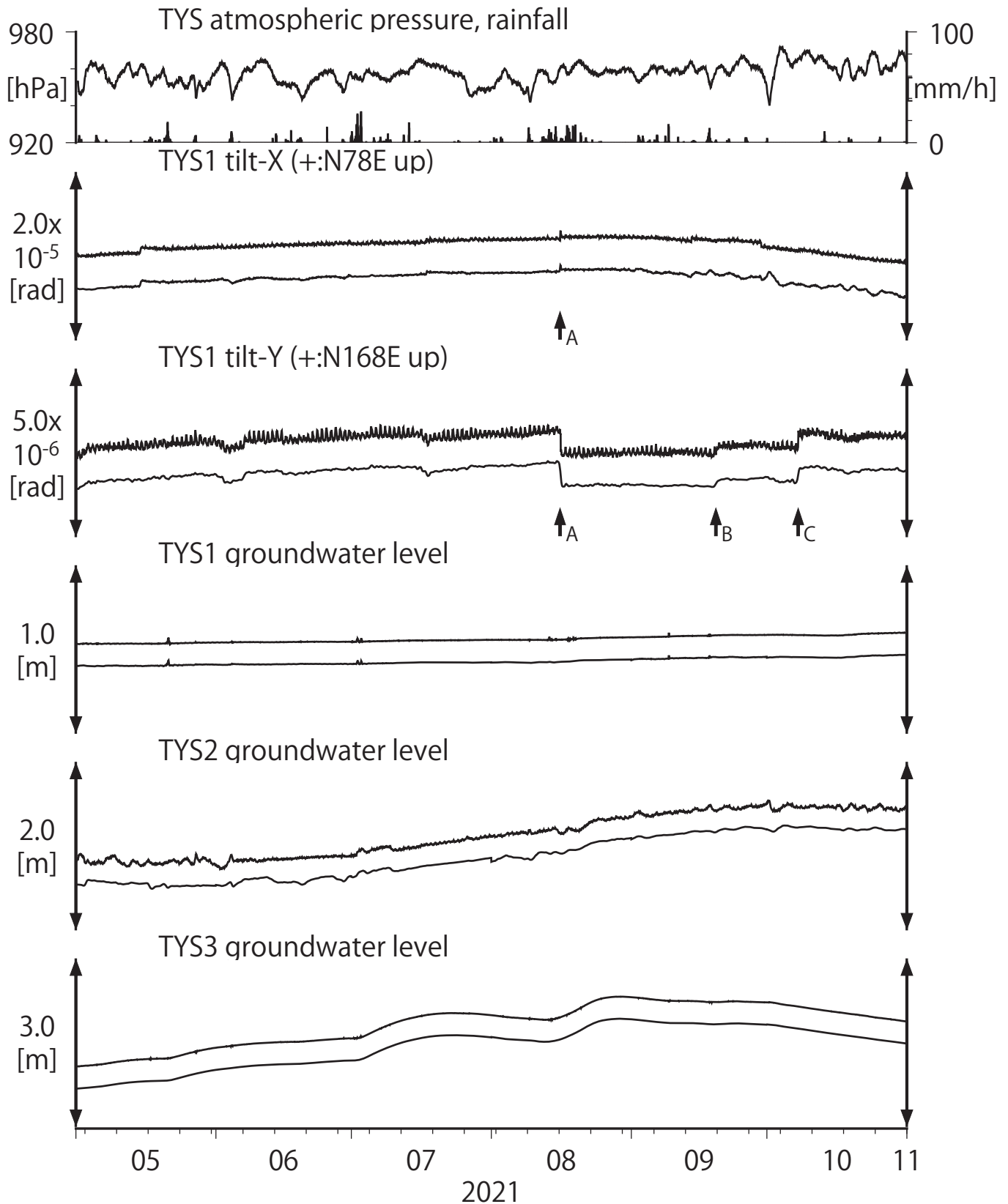
第3図 Tilt and groundwater level at TYS (時間値) (2021/05/01 00:00 - 2021/11/01 00:00 (JST))
