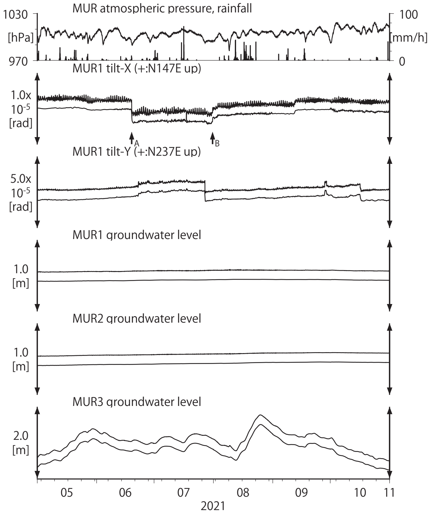
第24図 Tilt and groundwater level at MUR (時間値) (2021/05/01 00:00 - 2021/11/01 00:00 (JST))
