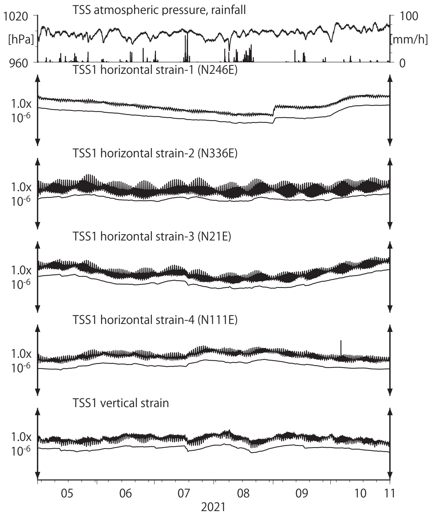
第29図 Crustal strains at TSS (時間値) (2021/05/01 00:00 - 2021/11/01 00:00 (JST))
