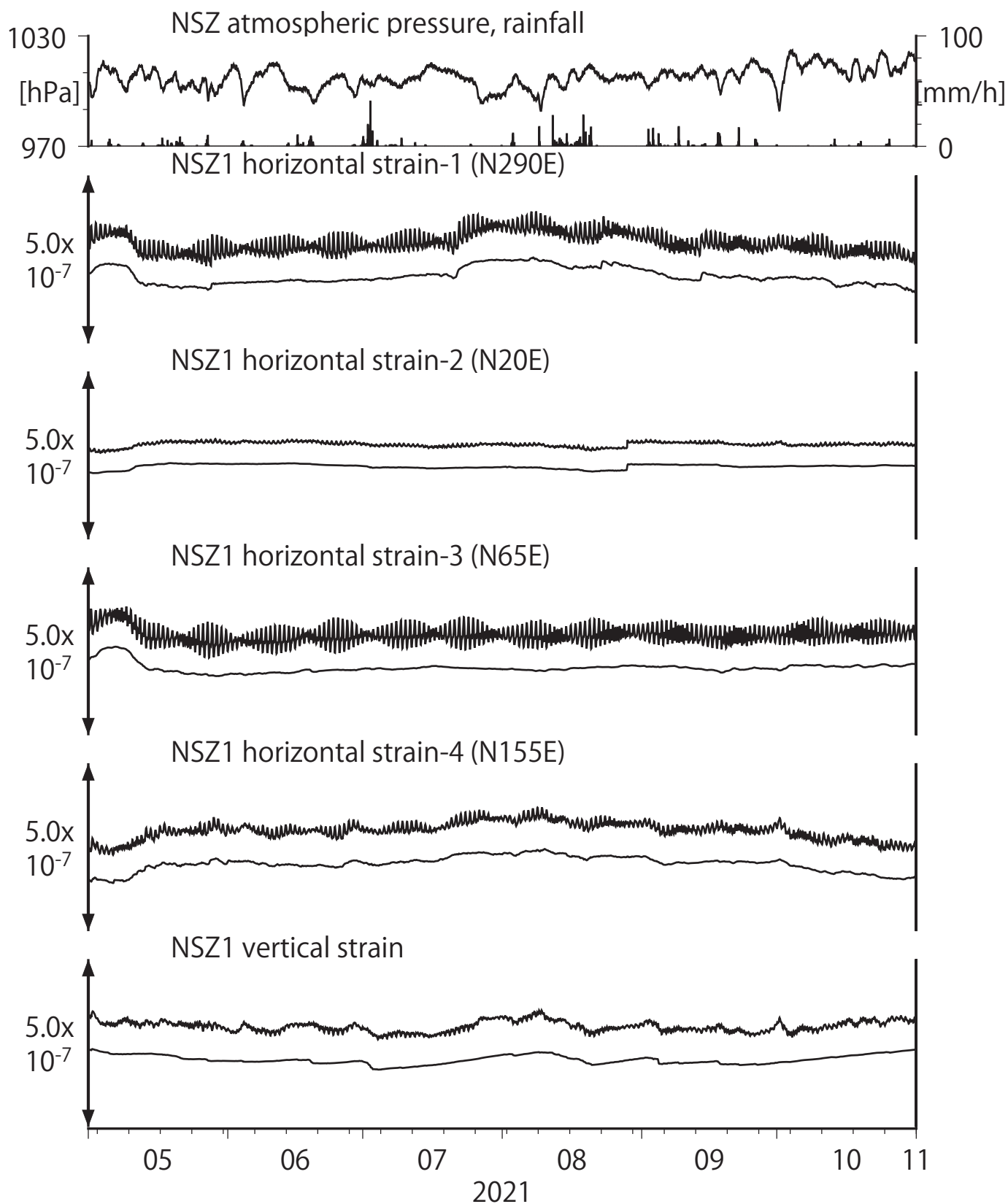
第4図 Crustal strains at NSZ (時間値) (2021/05/01 00:00 - 2021/11/01 00:00 (JST))
