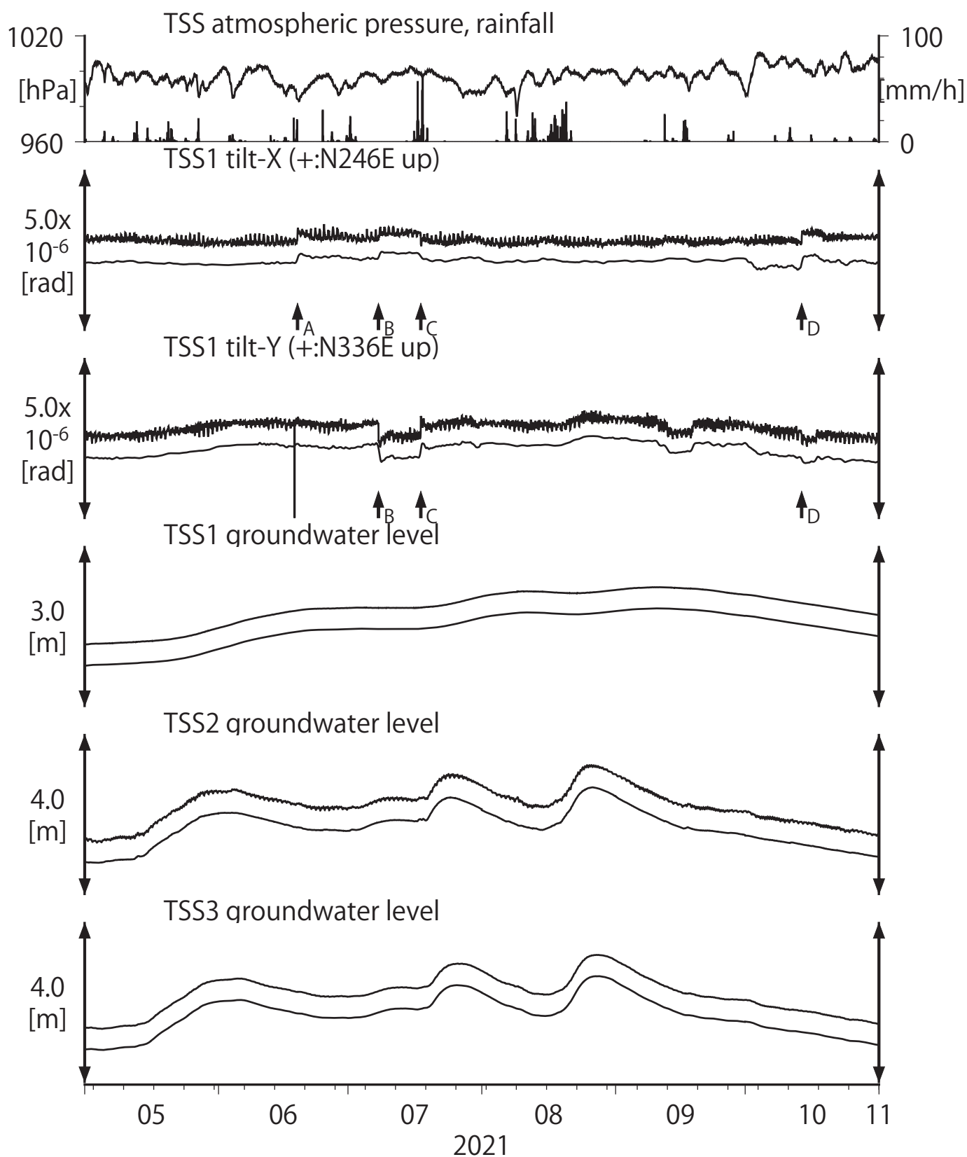
第30図 Tilt and groundwater level at TSS (時間値) (2021/05/01 00:00 - 2021/11/01 00:00 (JST))
