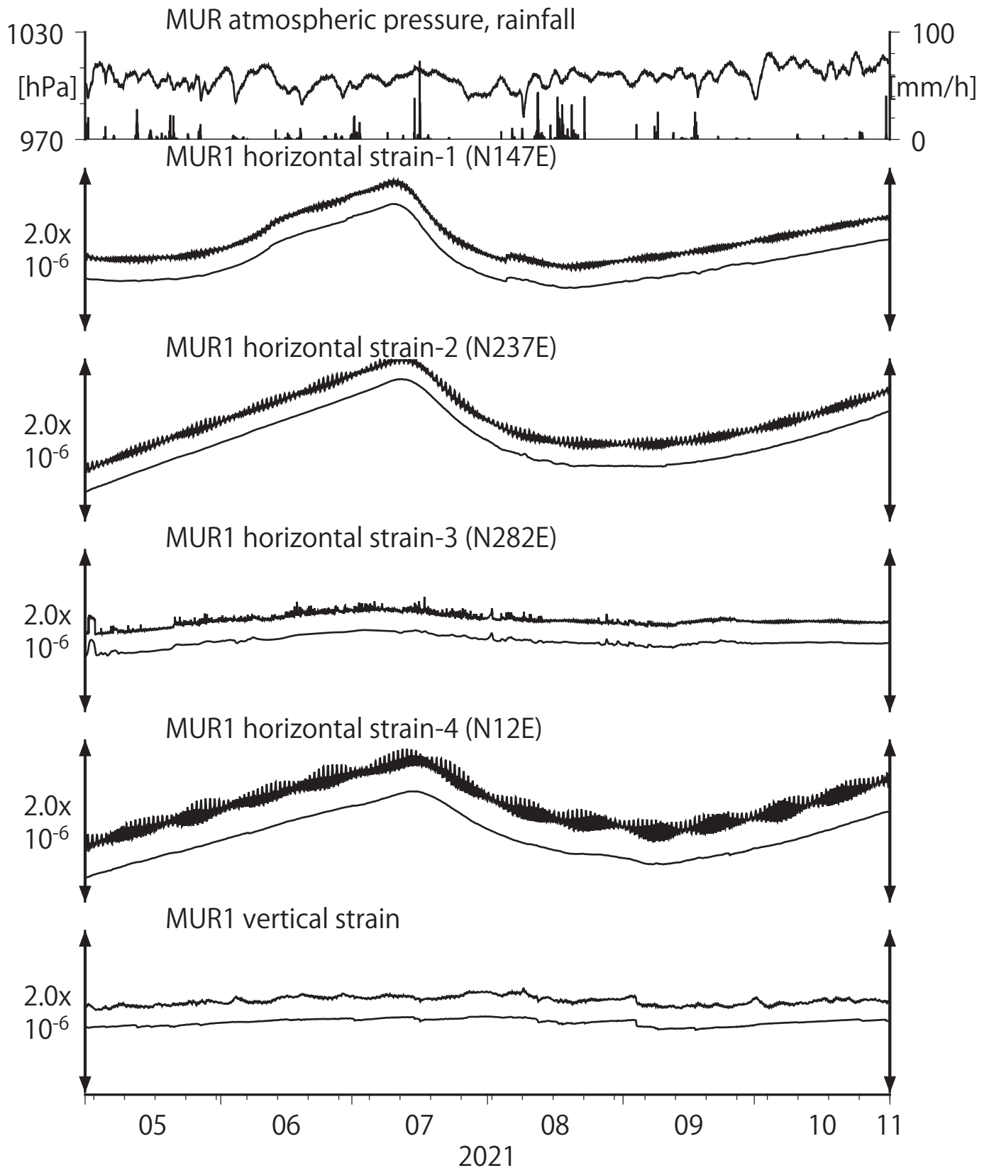
第23図 Crustal strains at MUR (時間値) (2021/05/01 00:00 - 2021/11/01 00:00 (JST))
