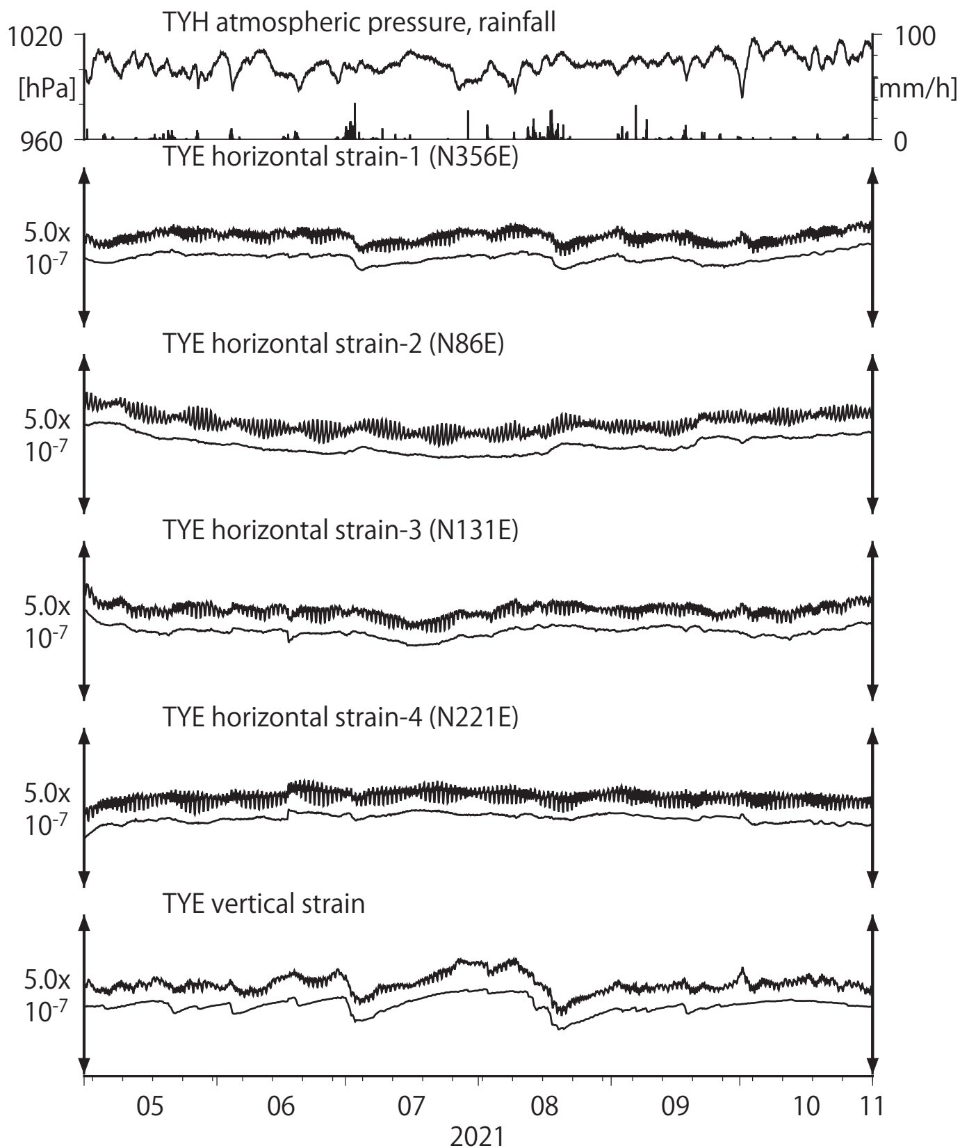
第6図 Crustal strain at TYE (時間値) (2021/05/01 00:00 - 2021/11/01 00:00 (JST))
