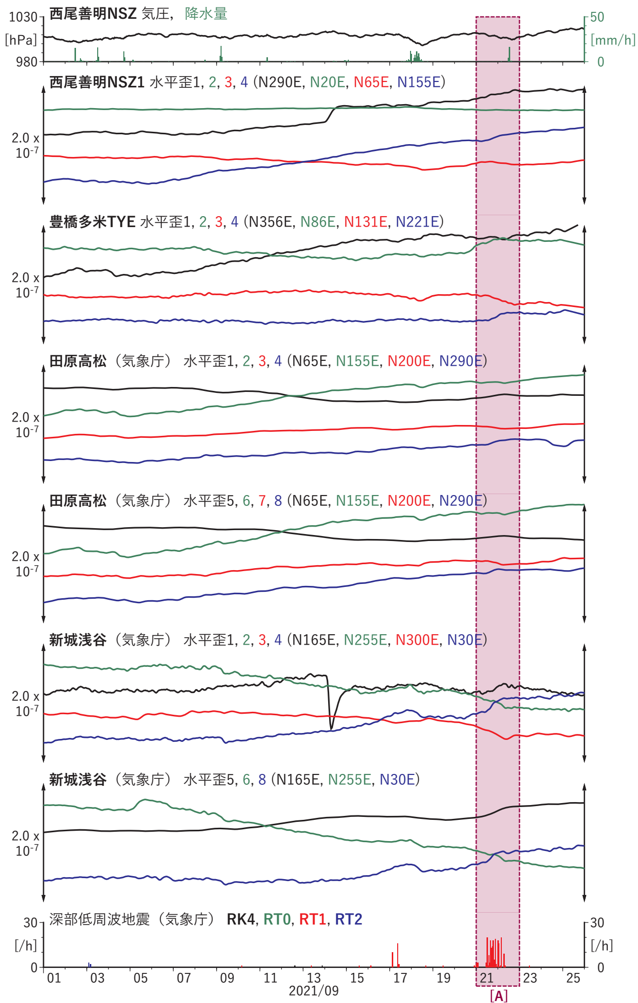
第38図 歪の時間変化 (2021/09/01 00:00 - 2021/09/26 00:00 (JST))
