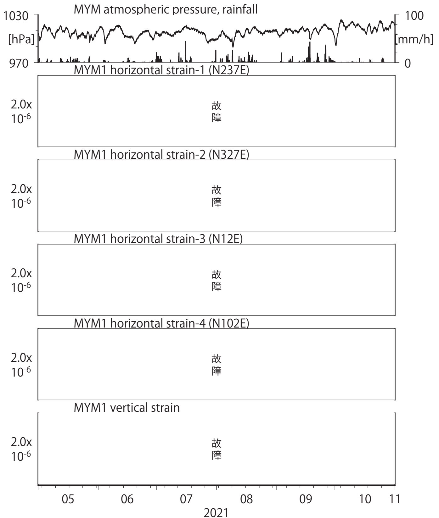
第12図 Crustal strains at MYM (時間値) (2021/05/01 00:00 - 2021/11/01 00:00 (JST))
