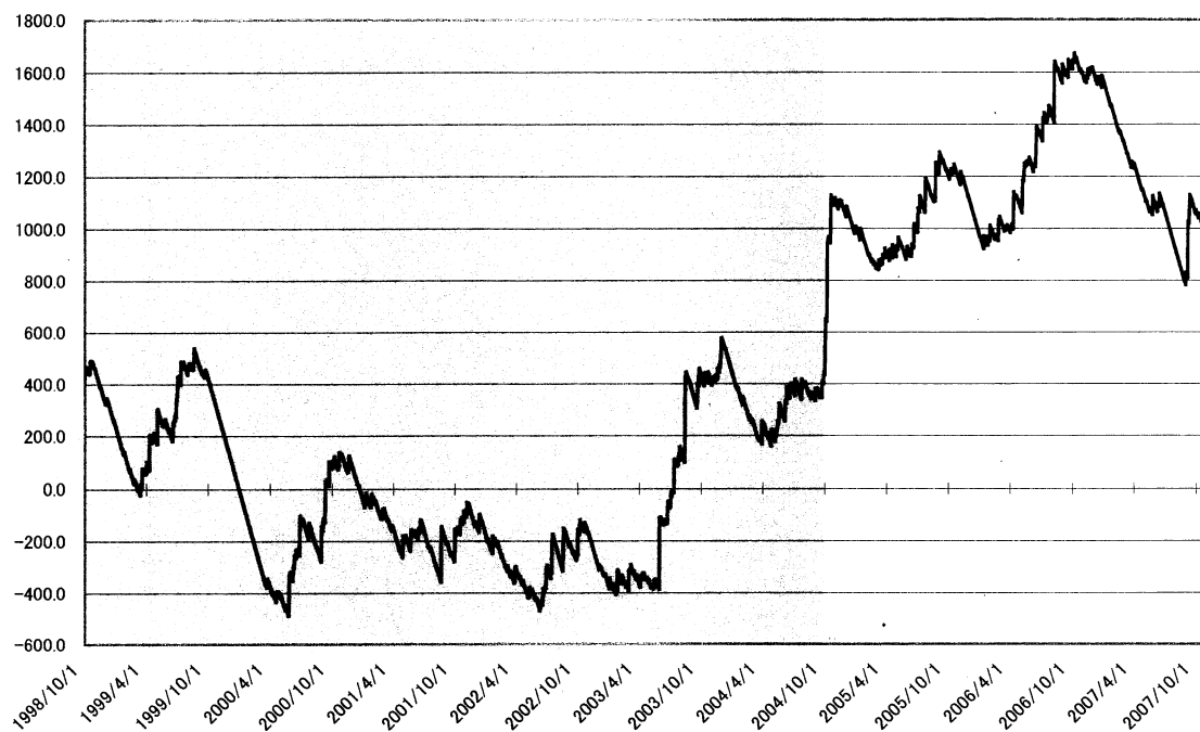
榛原観測井 降雨量の積算からトレンド除去後のグラフ (mm) (1998. 10. 1-2007. 11. 12)
