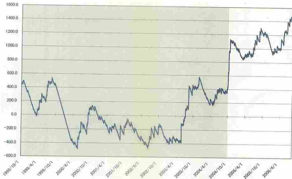
榛原観測井 降雨量の積算からトレンド除去後のグラフ (mm) (1998. 10. 1-2006. 8. 9)
