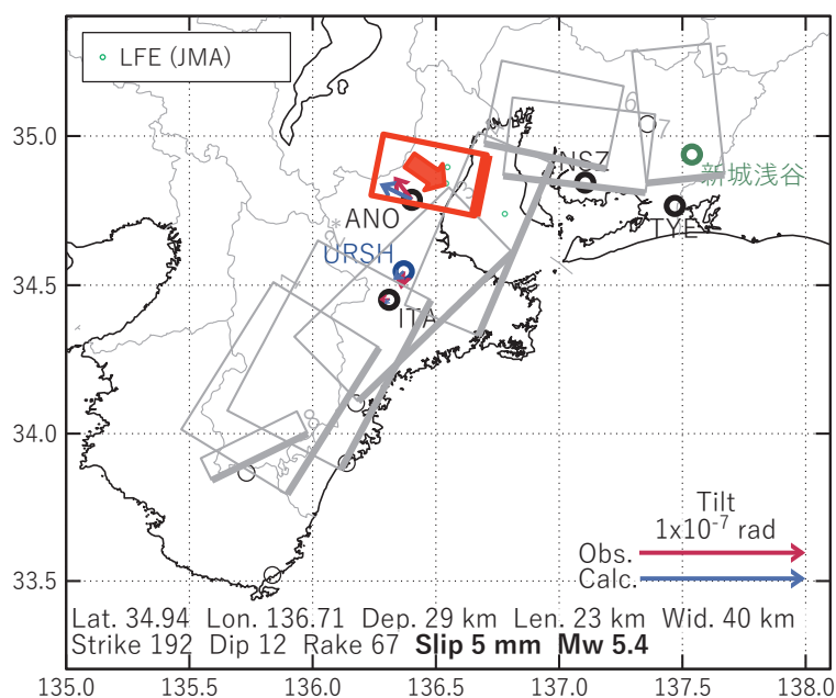
図3 2025/09/01PM-03AMの歪・傾斜変化（図2[A]）を説明する断層モデル。
