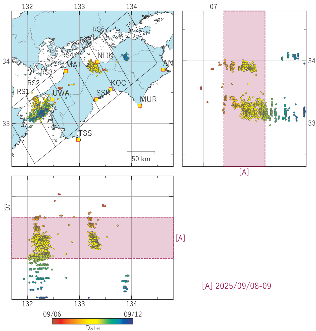
図6 四国地方における低周波地震の時空間分布図（2025/09/06 00:00 - 2025/09/12 00:00 (JST)）。気象庁カタログによる。 (観測点名) ANK: 阿南桑野, MUR: 室戸岬, NHK: 新居浜黒島, KOC: 高知五台山, SSK: 須崎大谷, MAT: 松山南江戸, UWA: 西予宇和, TSS: 土佐清水松尾
