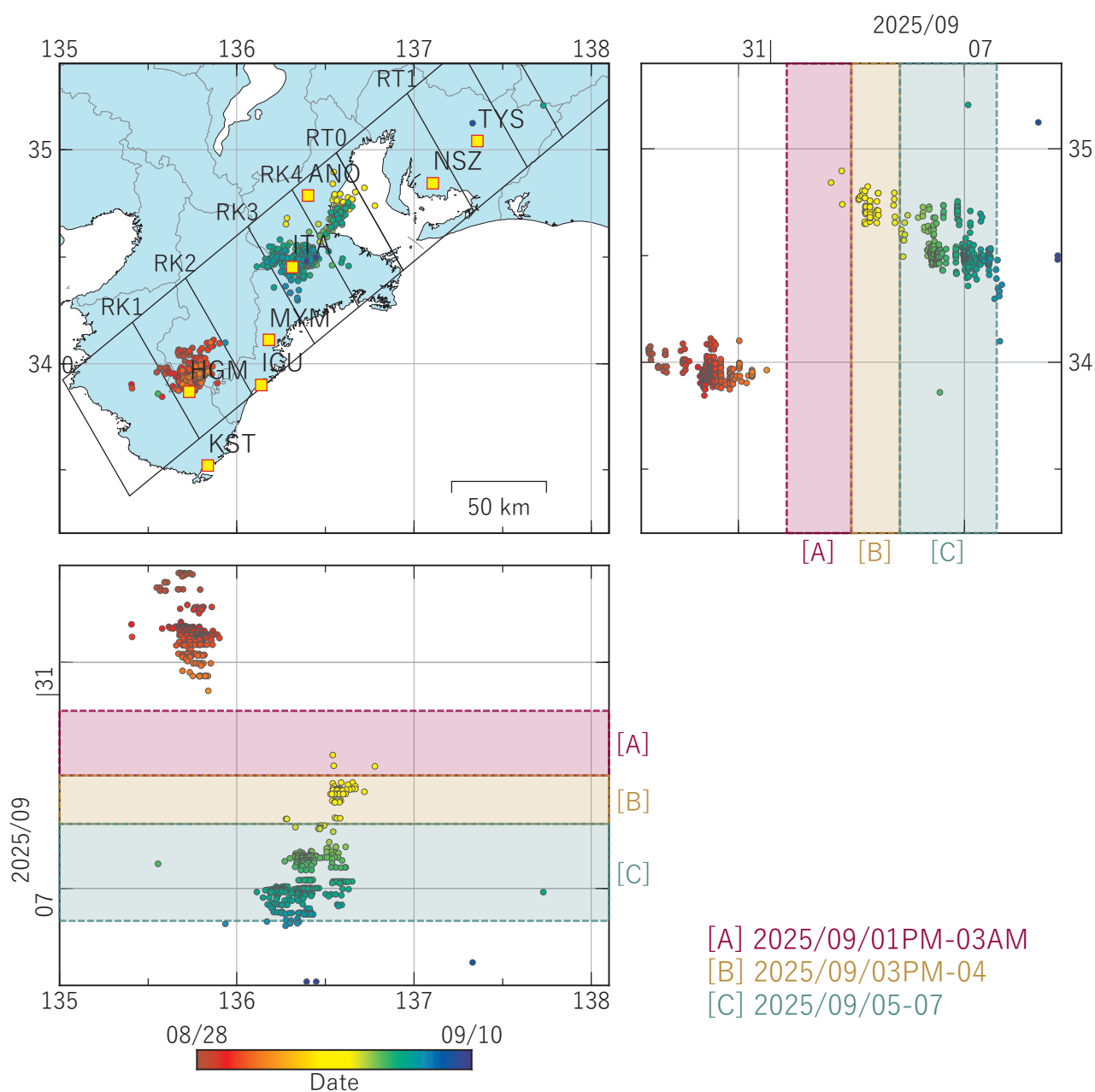
図1 紀伊半島・東海地方における低周波地震の時空間分布図（2025/08/28 00:00 - 2025/09/10 00:00 (JST)）。気象庁カタログによる。 （観測点名）TYS: 豊田神殿, NSZ: 西尾善明, ANO: 津安濃, ITA: 松阪飯高, MYM: 紀北海山, ICU: 熊野磯崎, HGM: 田辺本宮, KST: 串本津荷
