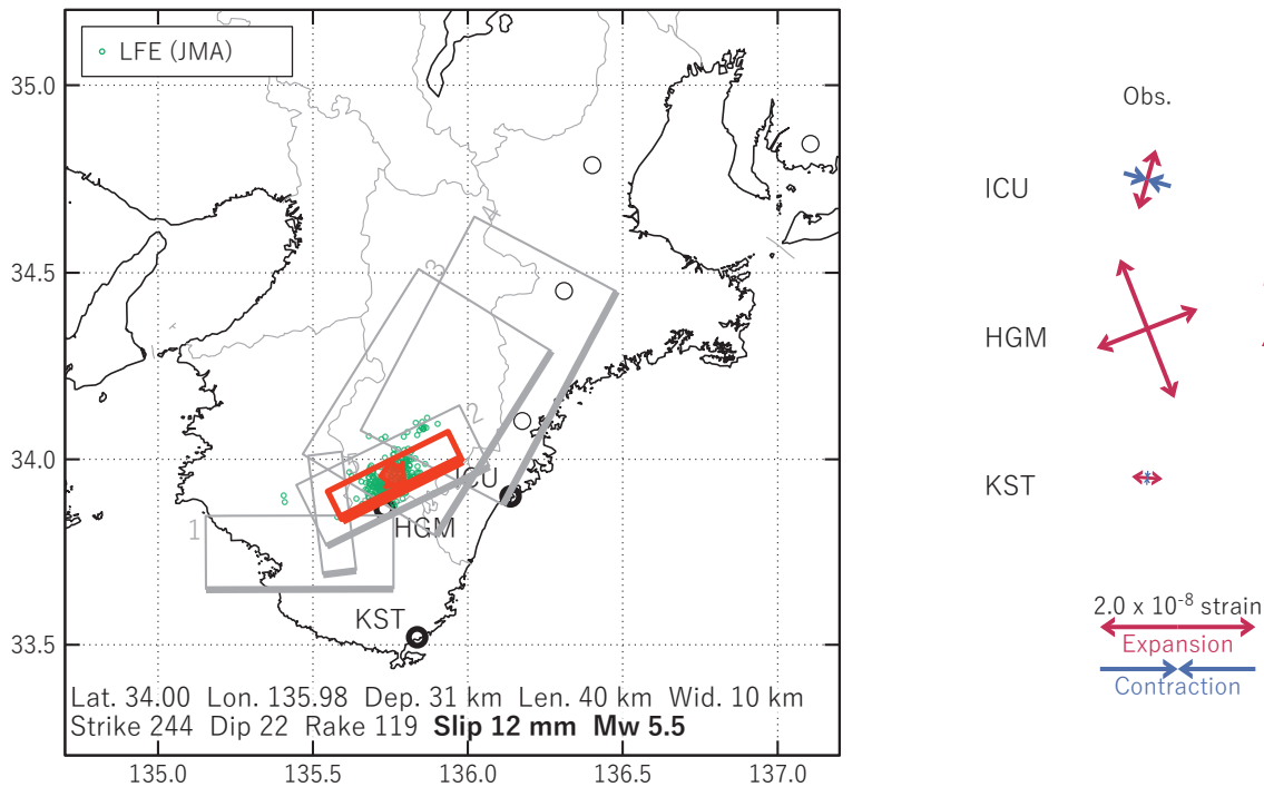
図3 2025/08/29 - 31AMの歪変化（図2[A]）を説明する断層モデル。
