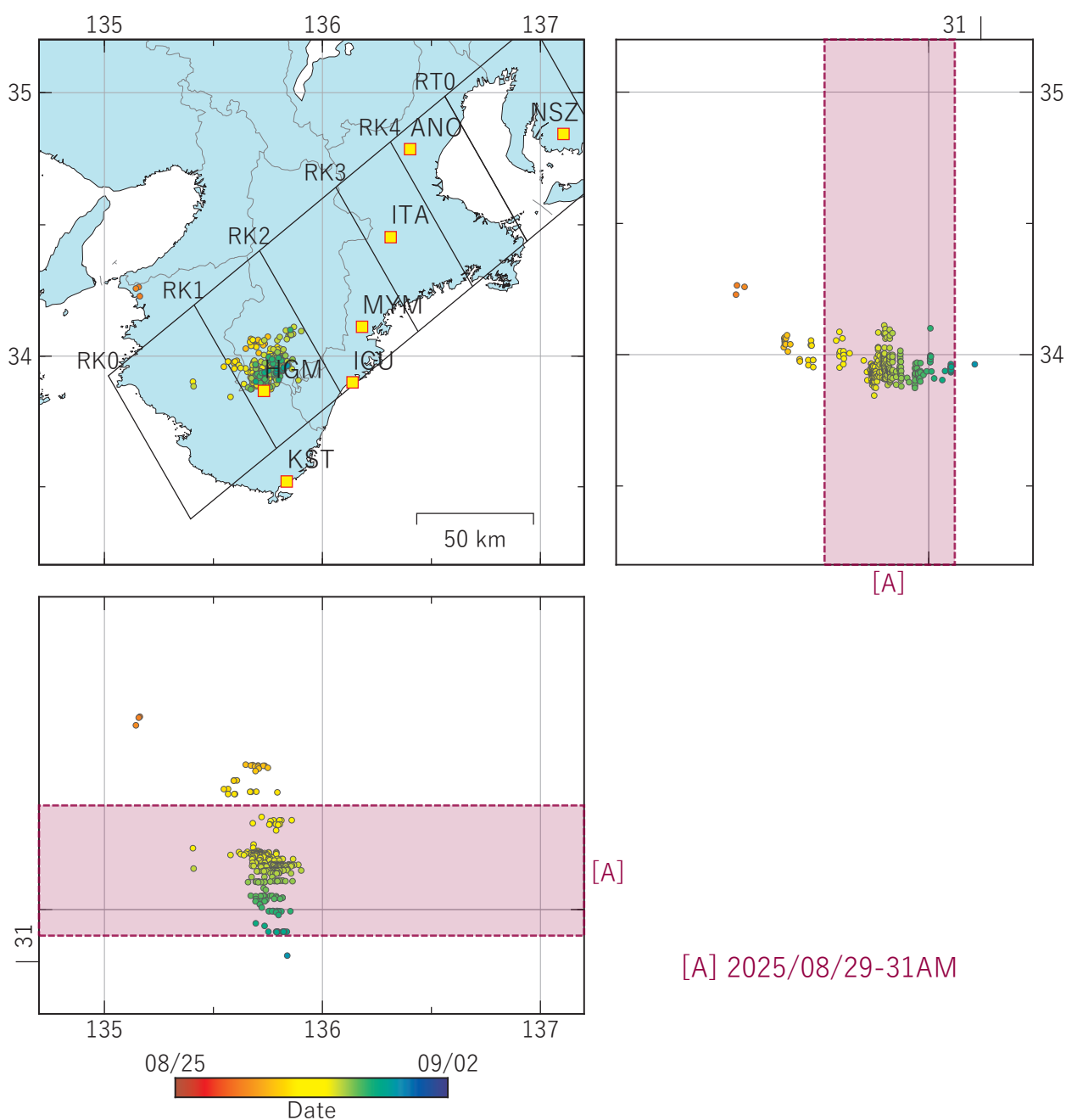
図1 紀伊半島における低周波地震の時空間分布図（2025/08/25 00:00 - 2025/09/02 00:00 (JST)）。気象庁カタログによる。 （観測点名）NSZ: 西尾善明, ANO: 津安濃, ITA: 松阪飯高, MYM: 紀北海山, ICU: 熊野磯崎, HGM: 田辺本宮, KST: 串本津荷
