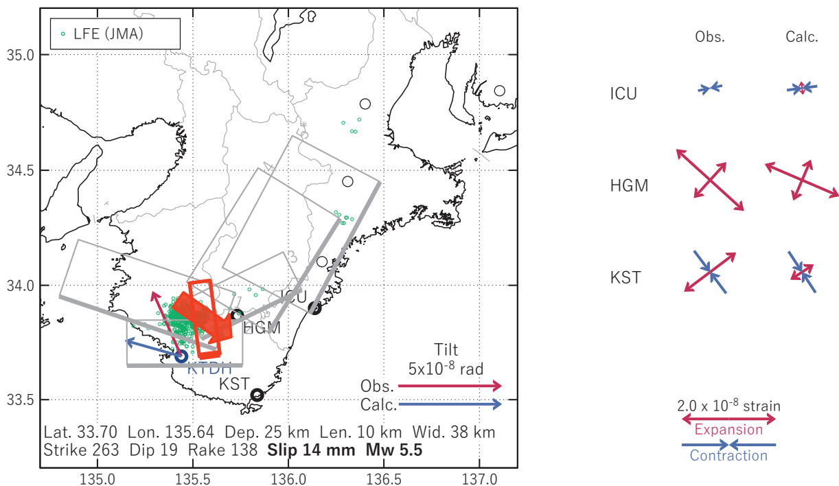
図9 2025/06/29 - 07/02AMの歪・傾斜変化（図8[A]）を説明する断層モデル。
