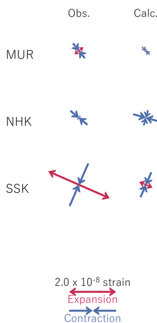
図6 2025/06/26-07/02の歪・傾斜変化（図2[D]）を説明する断層モデル。
