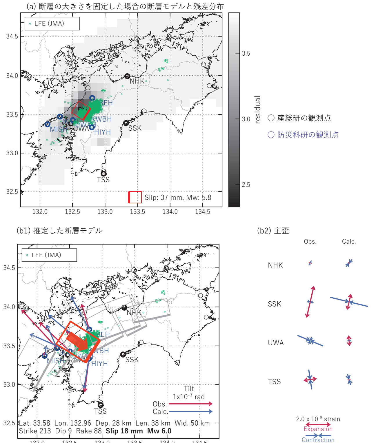
図3 2025/06/10-14の歪・傾斜変化（図2[A]）を説明する断層モデル。
