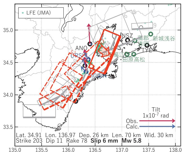
図8 2025/05/09PM-14の歪・傾斜変化（図3[E]）を説明する断層モデル。
