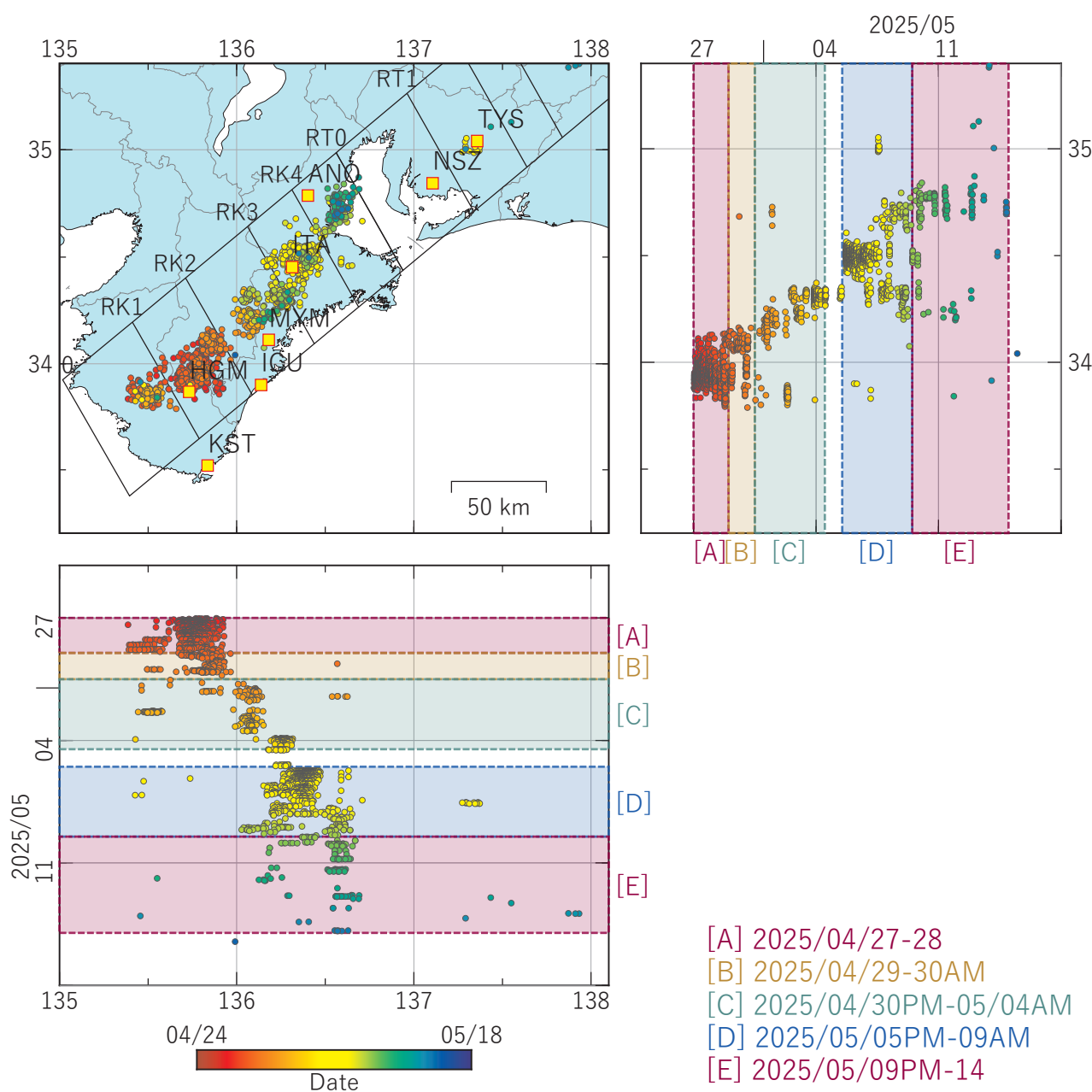
図1 紀伊半島・東海地方における低周波地震の時空間分布図（2025/04/24 00:00 - 2025/05/18 00:00 (JST)）。気象庁カタログによる。 （観測点名）TYS: 豊田神殿, NSZ: 西尾善明, ANO: 津安濃, ITA: 松阪飯高, MYM: 紀北海山, ICU: 熊野磯崎, HCM: 田辺本宮, KST: 串本津荷
