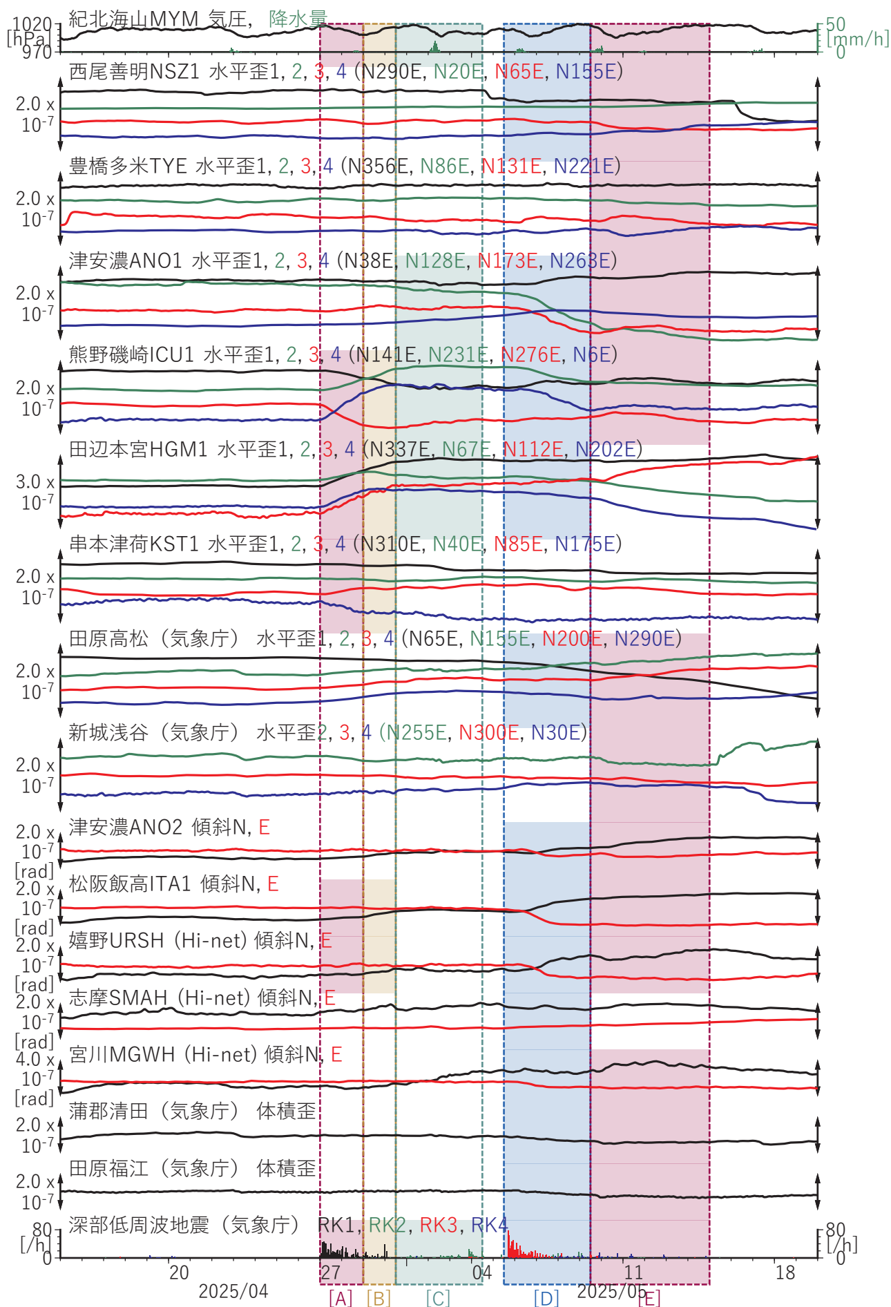
図3 東海・紀伊半島における歪・傾斜観測結果 (2025/04/15 00:00 - 2025/05/20 00:00 (JST))
