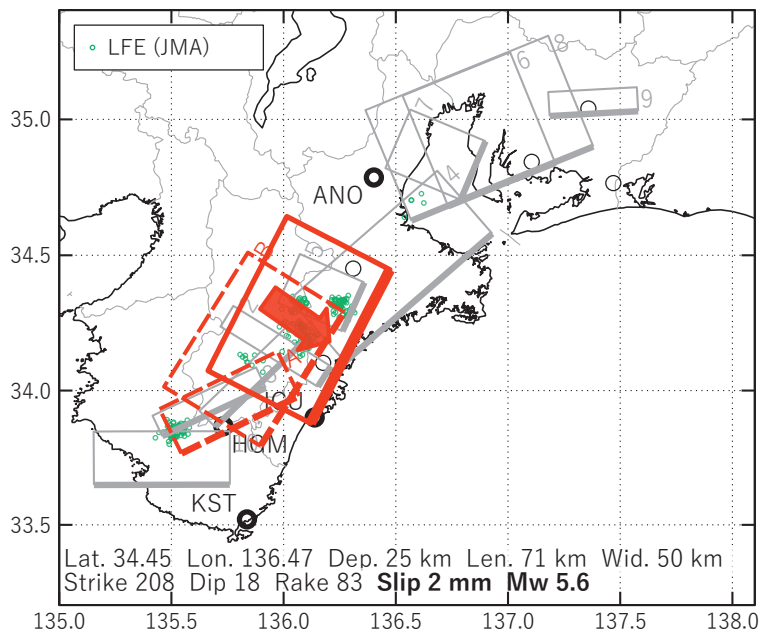
図6 2025/04/30PM-05/04AMの歪変化（図3[C]）を説明する断層モデル。
