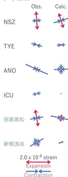
図8 2025/05/09PM-14の歪・傾斜変化（図3[E]）を説明する断層モデル。
