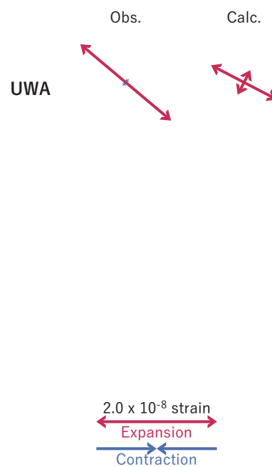
図3 2025/04/23PM - 25AM の歪・傾斜変化（図2 [A]）を説明する断層モデル。
