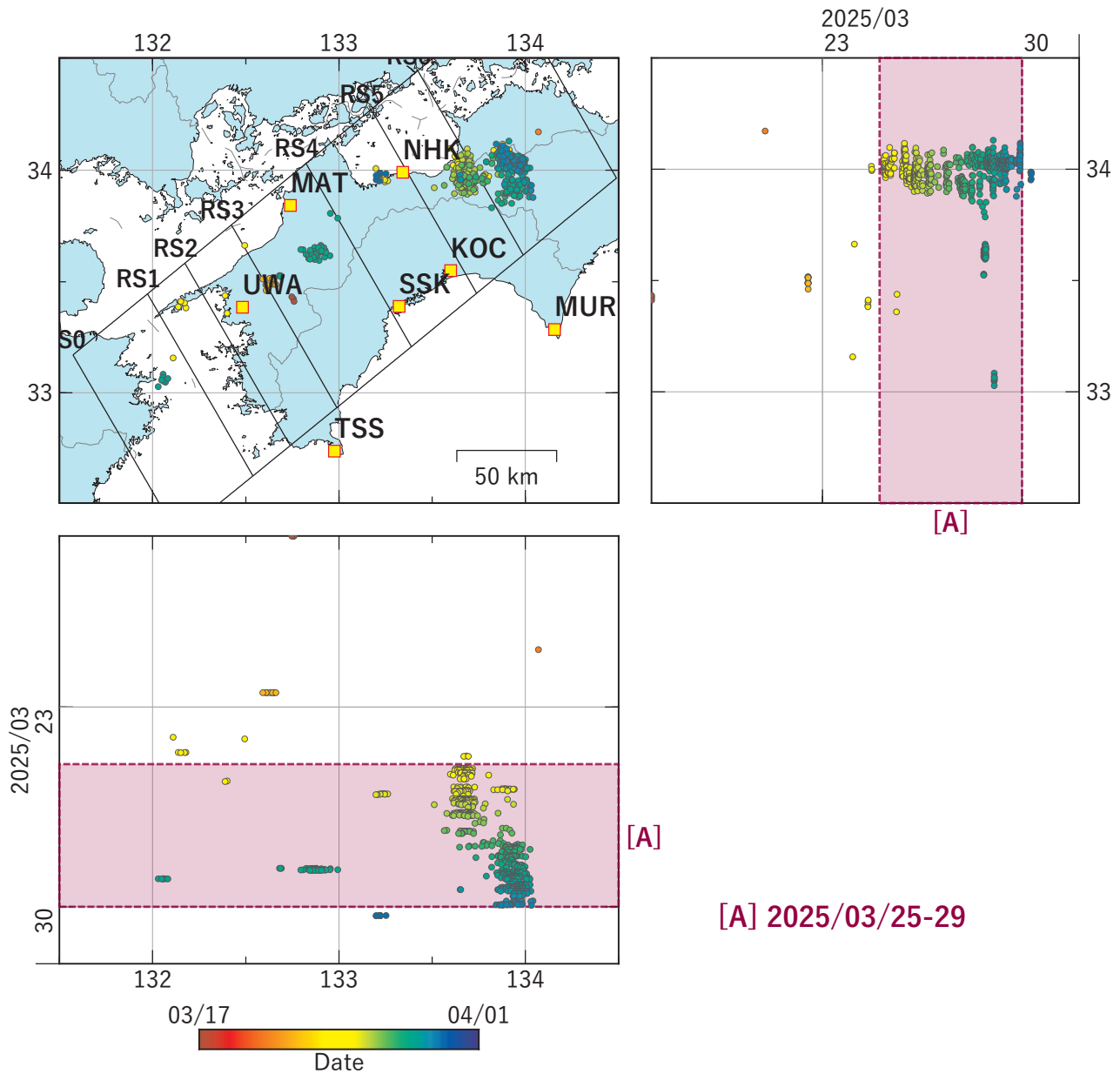
図4 四国地方における深部低周波地震の時空間分布図。 (2025/03/17 00:00 - 2025/04/01 00:00 (JST)) 気象庁カタログによる。
