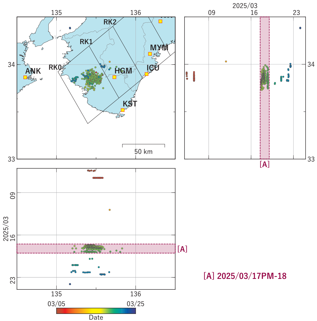
図1 紀伊半島における深部低周波地震の時空間分布図。 (2025/03/05 00:00 - 2025/03/25 00:00 (JST)) 気象庁カタログによる。
