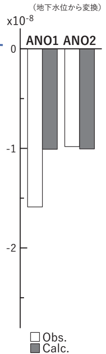
図3 2024/12/11-13AMの歪・傾斜・地下水位の変化(図2[A])を説明する断層モデル。
