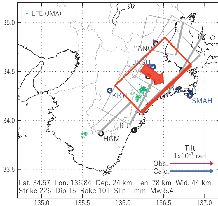
図4 2024/05/19PM-21AMの歪・傾斜変化（図2[A]）を説明する断層モデル。
