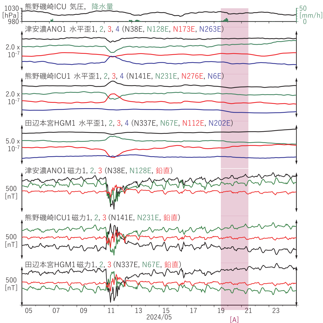
図3 紀伊半島における歪・磁力観測結果 (2024/05/05 00:00 - 2024/05/24 00:00 (JST))
