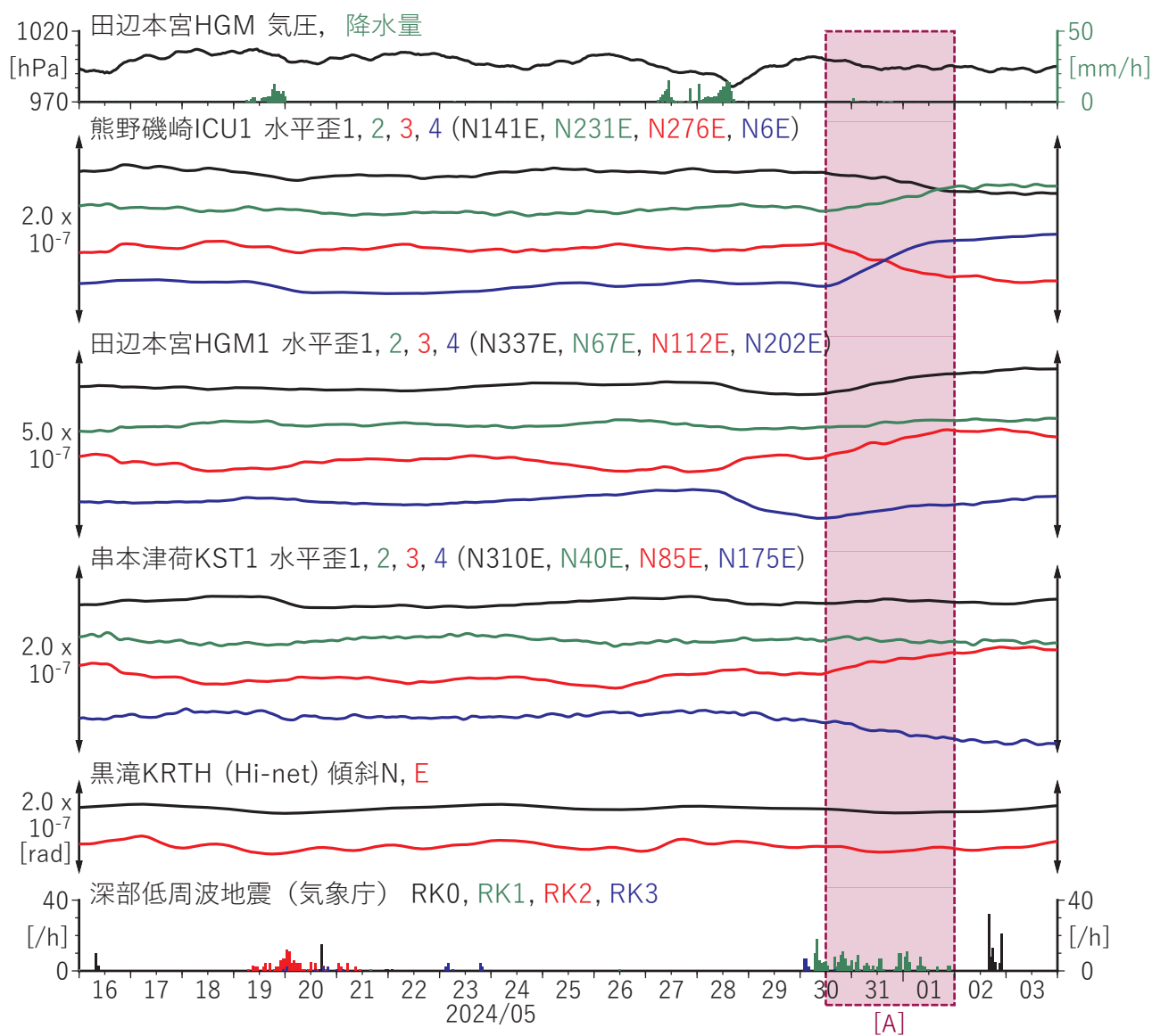
図6 紀伊半島における歪・傾斜観測結果 (2024/05/16 00:00 - 2024/06/04 00:00 (JST))
