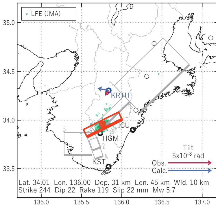
図7 2024/05/30PM-06/01の歪・傾斜変化(図4[A])を説明する断層モデル。
