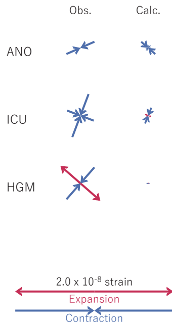
図4 2024/05/19PM-21AMの歪・傾斜変化（図2[A]）を説明する断層モデル。
