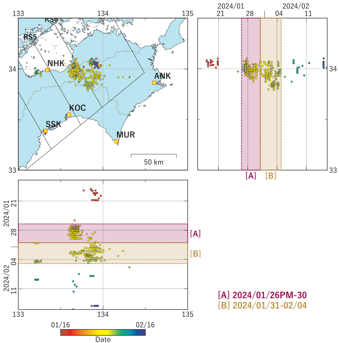
図1 四国地方における深部低周波地震の時空間分布図。 (2024/01/16 00:00 - 2024/02/16 00:00 (JST)) 気象庁カタログによる。
