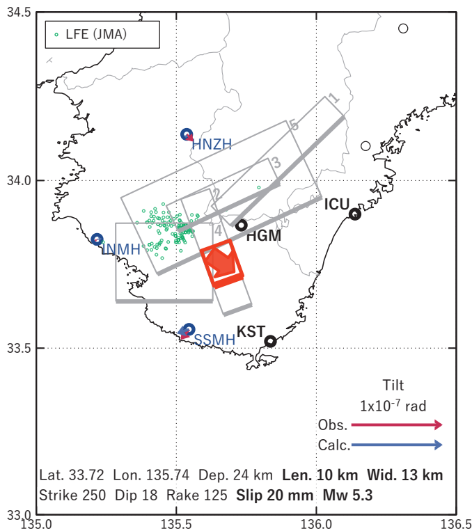
図7 2024/02/20 - 21AM の歪・傾斜変化 (図6 [A]) を説明する断層モデル。
