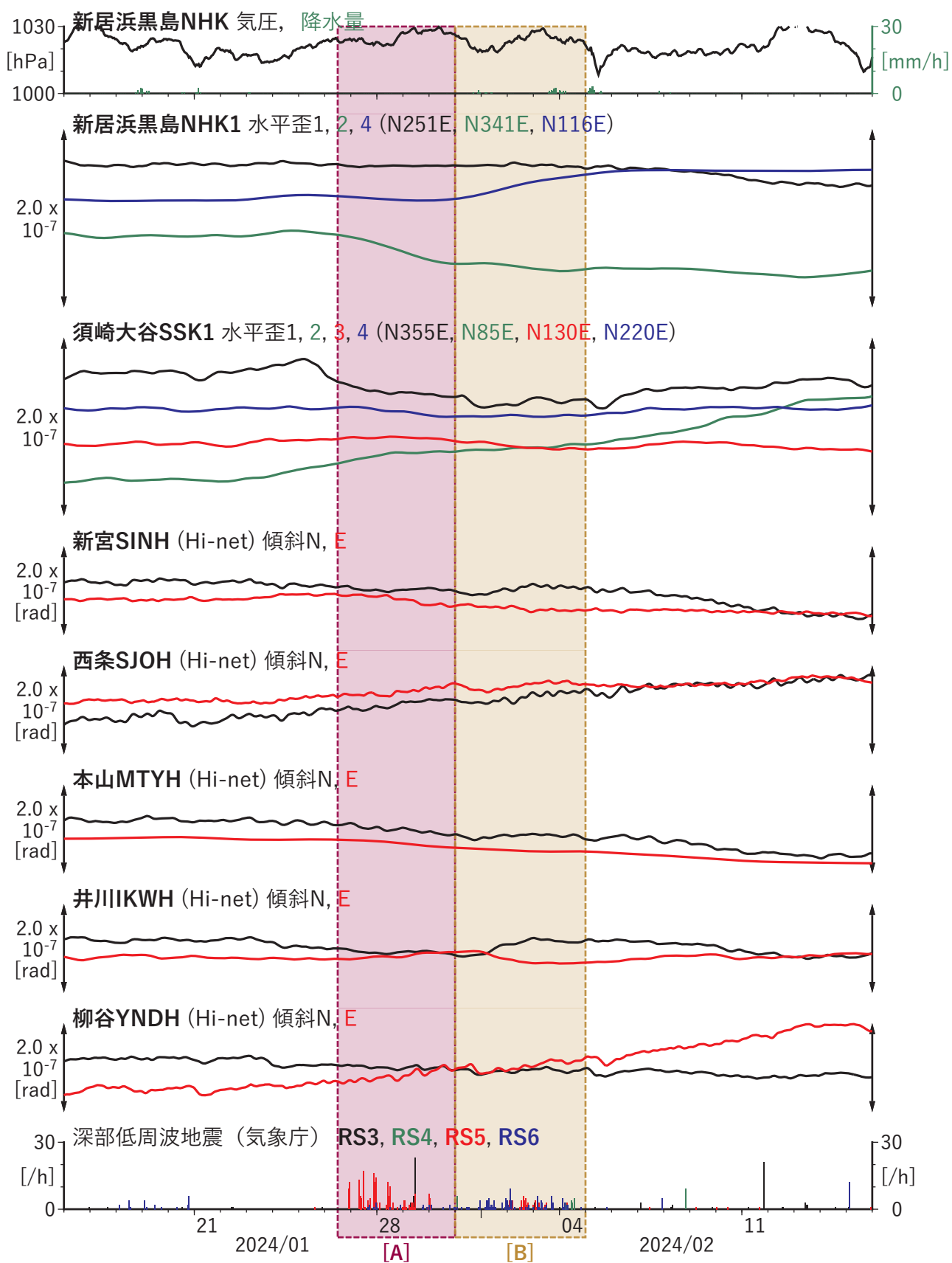
図2 四国地方における歪・傾斜の時間変化 (2024/01/16 00:00 - 2024/02/16 00:00 (JST))
