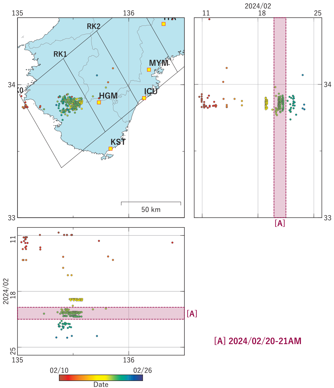
図5 紀伊半島における深部低周波地震の時空間分布図。 (2024/02/10 00:00 - 2024/02/26 00:00 (JST)) 気象庁カタログによる。
