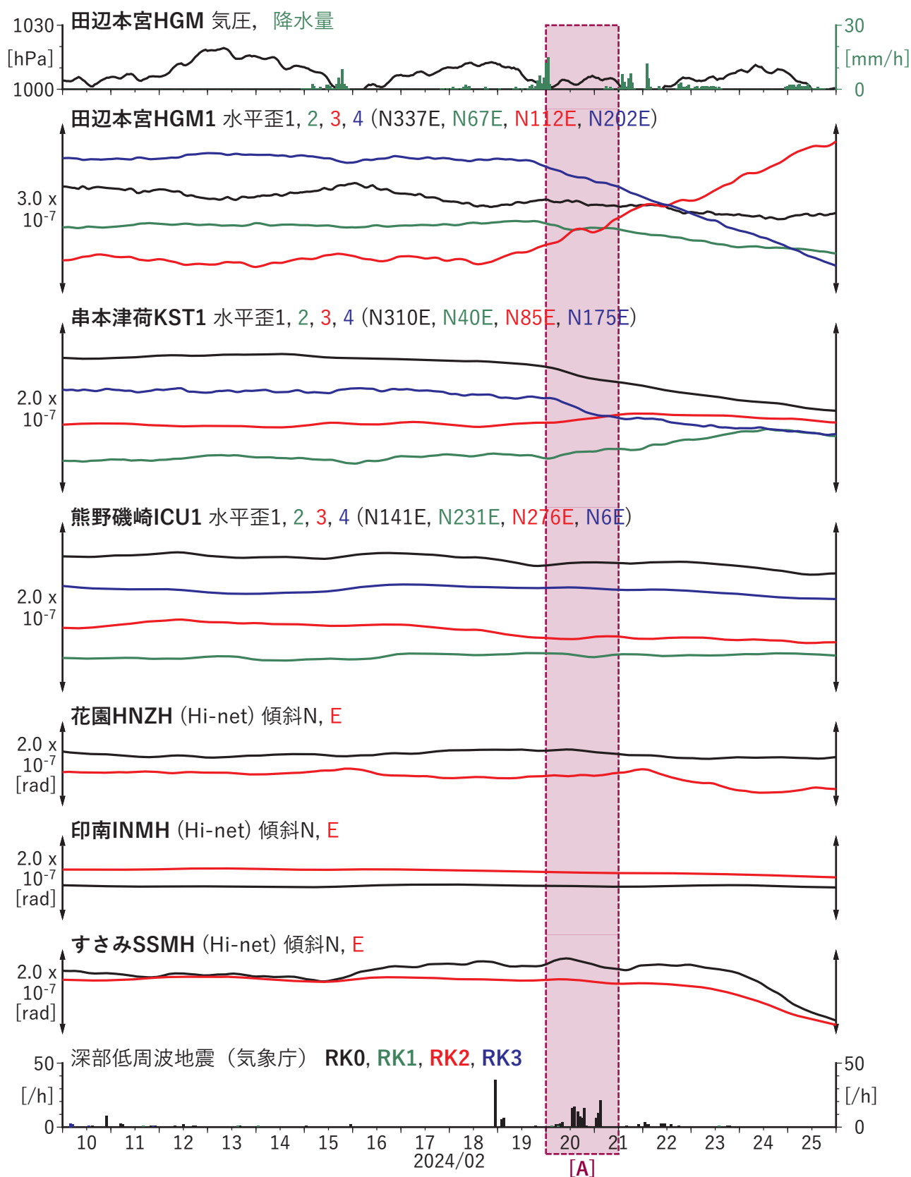
図6 紀伊半島における歪・傾斜の時間変化 (2024/02/10 00:00 - 2024/02/26 00:00 (JST))
