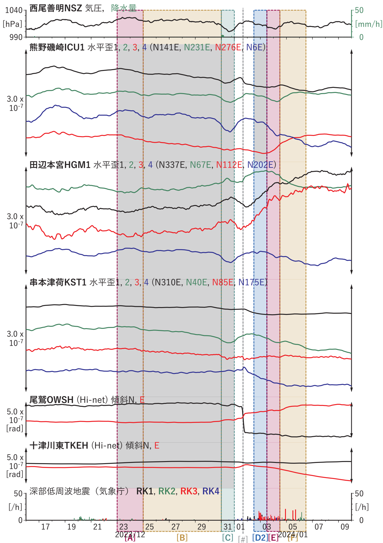
図2 歪・傾斜の時間変化(5) (2023/12/16 00:00-2024/01/10 00:00 (JST))
