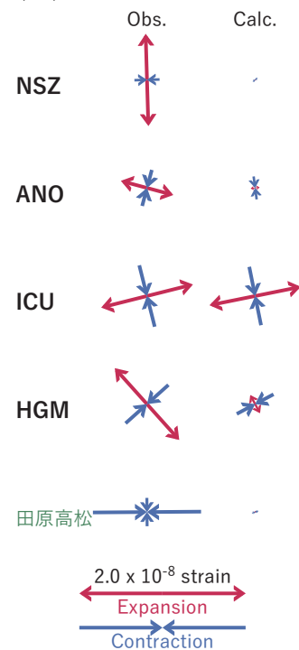
図9 2024/01/04PM-06AMの歪・傾斜変化（図2[F]）を説明する断層モデル。
