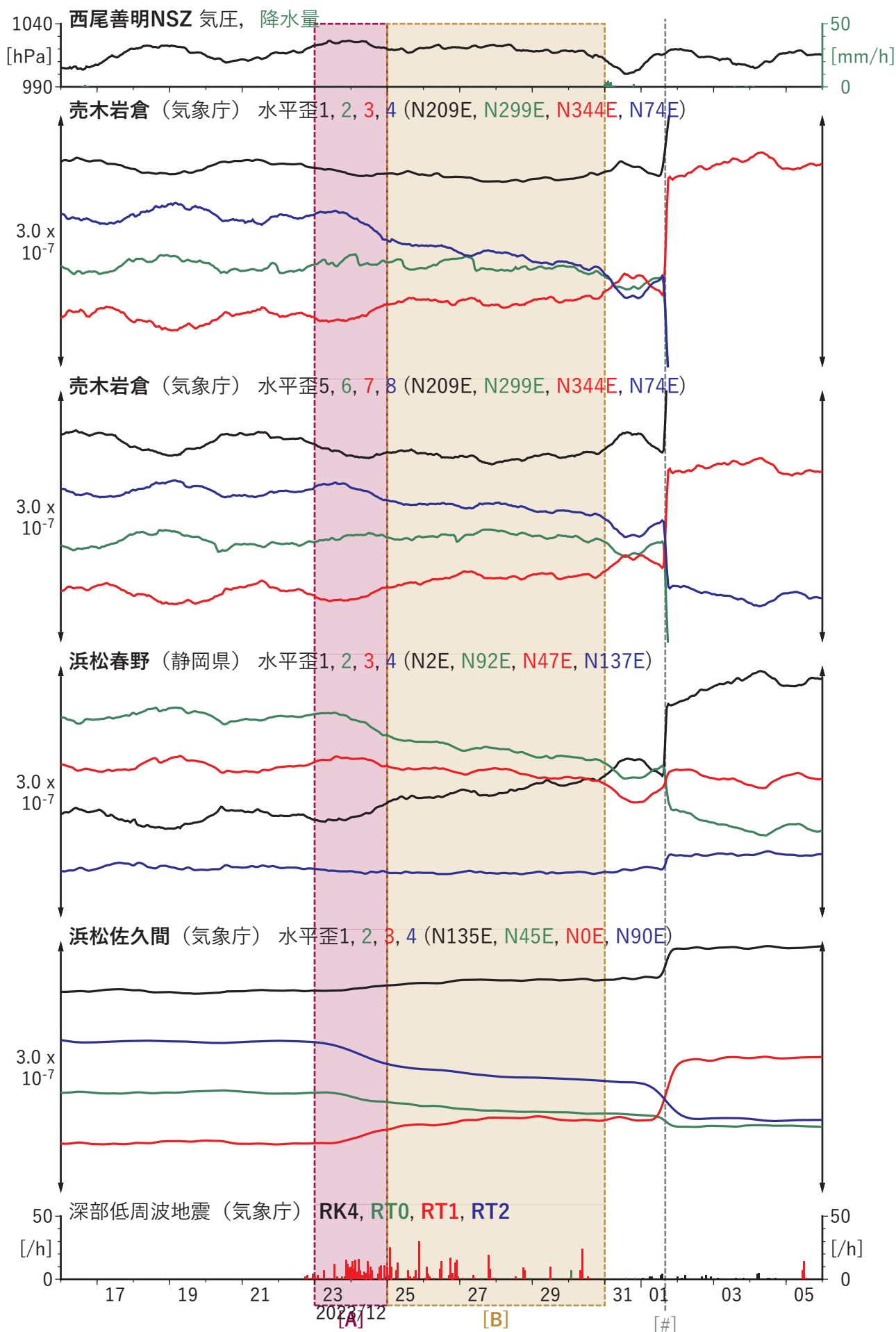
図2 歪・傾斜の時間変化(2) (2023/12/16 00:00-2024/01/06 00:00 (JST))
