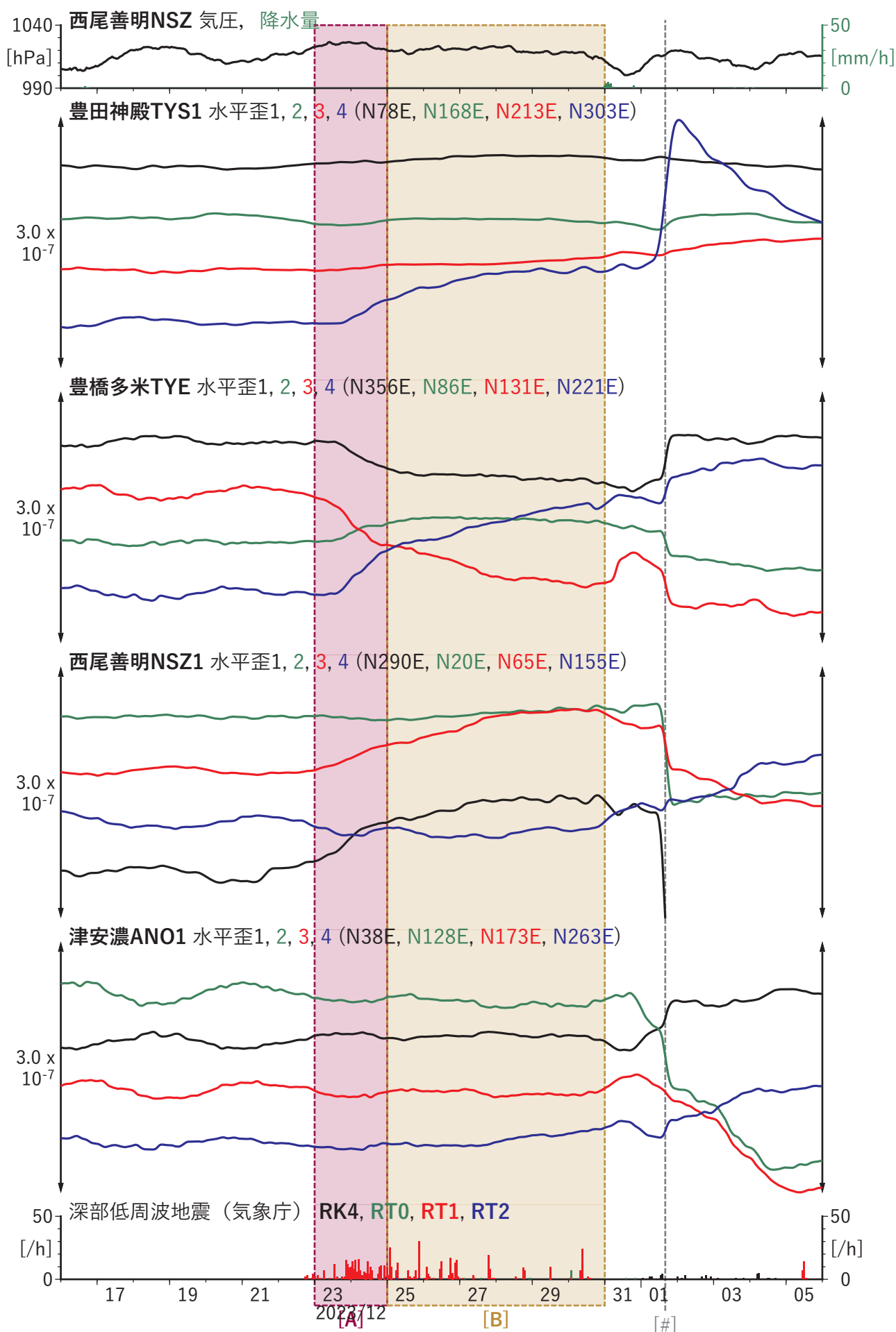
図2 歪・傾斜の時間変化(1) (2023/12/16 00:00-2024/01/06 00:00 (JST))
