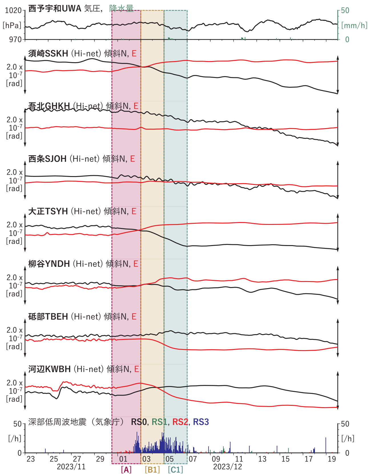
図6 歪・傾斜の時間変化(2) (2023/11/23 00:00-2023/12/20 00:00 (JST))
