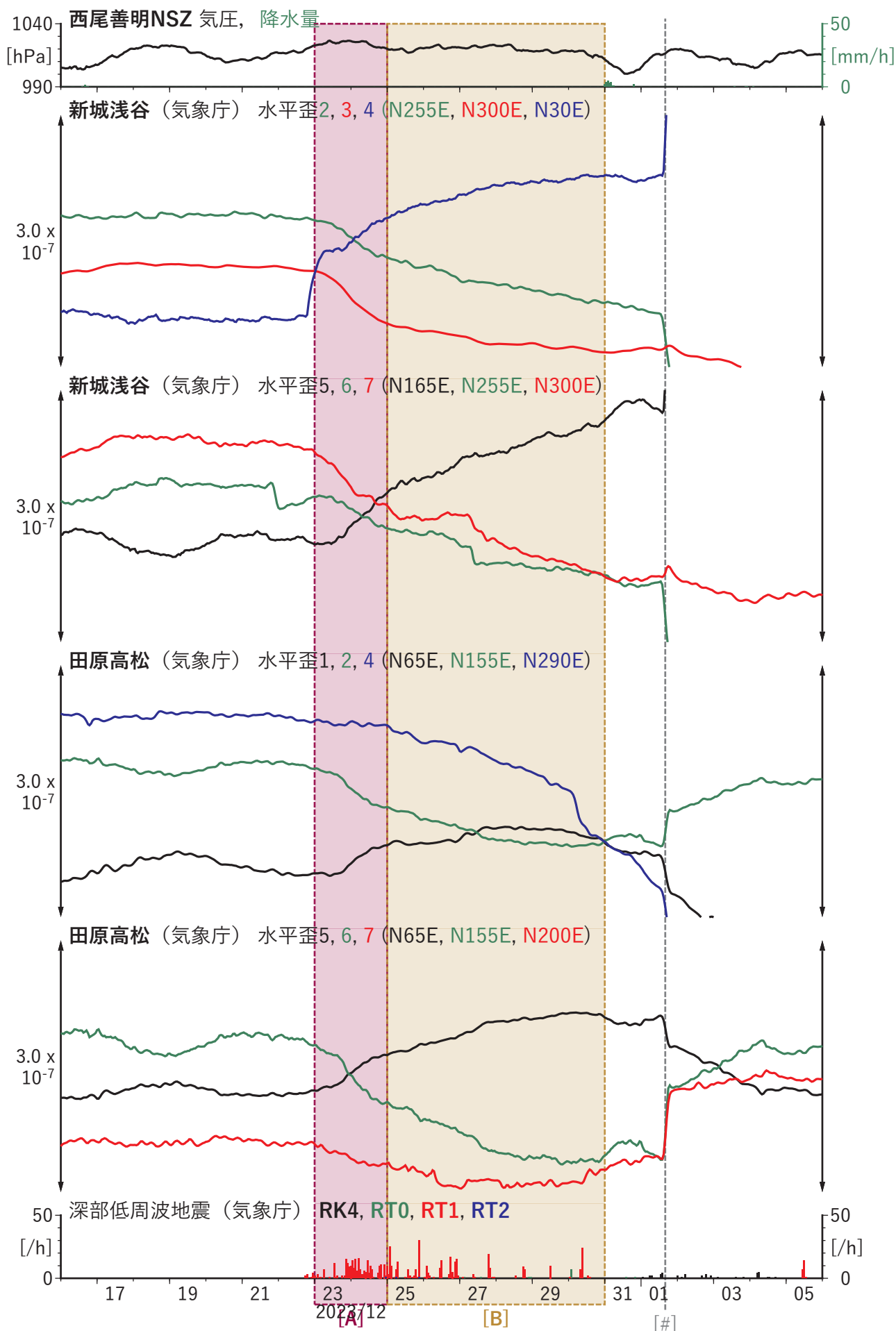
図2 歪・傾斜の時間変化(3) (2023/12/16 00:00-2024/01/06 00:00 (JST))
