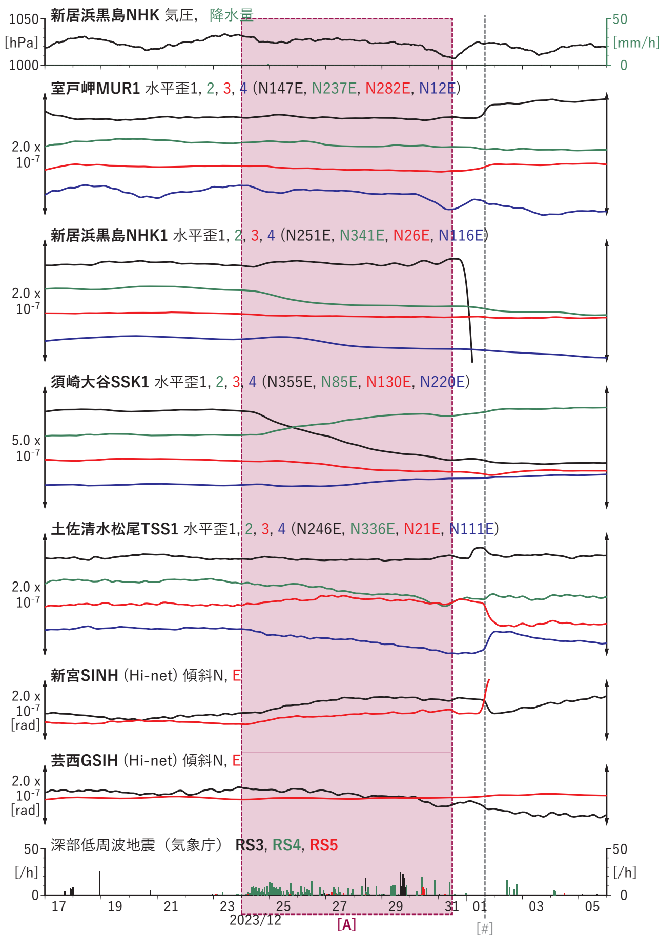
図13 歪・傾斜の時間変化(1) (2023/12/17 00:00-2024/01/06 00:00 (JST))
