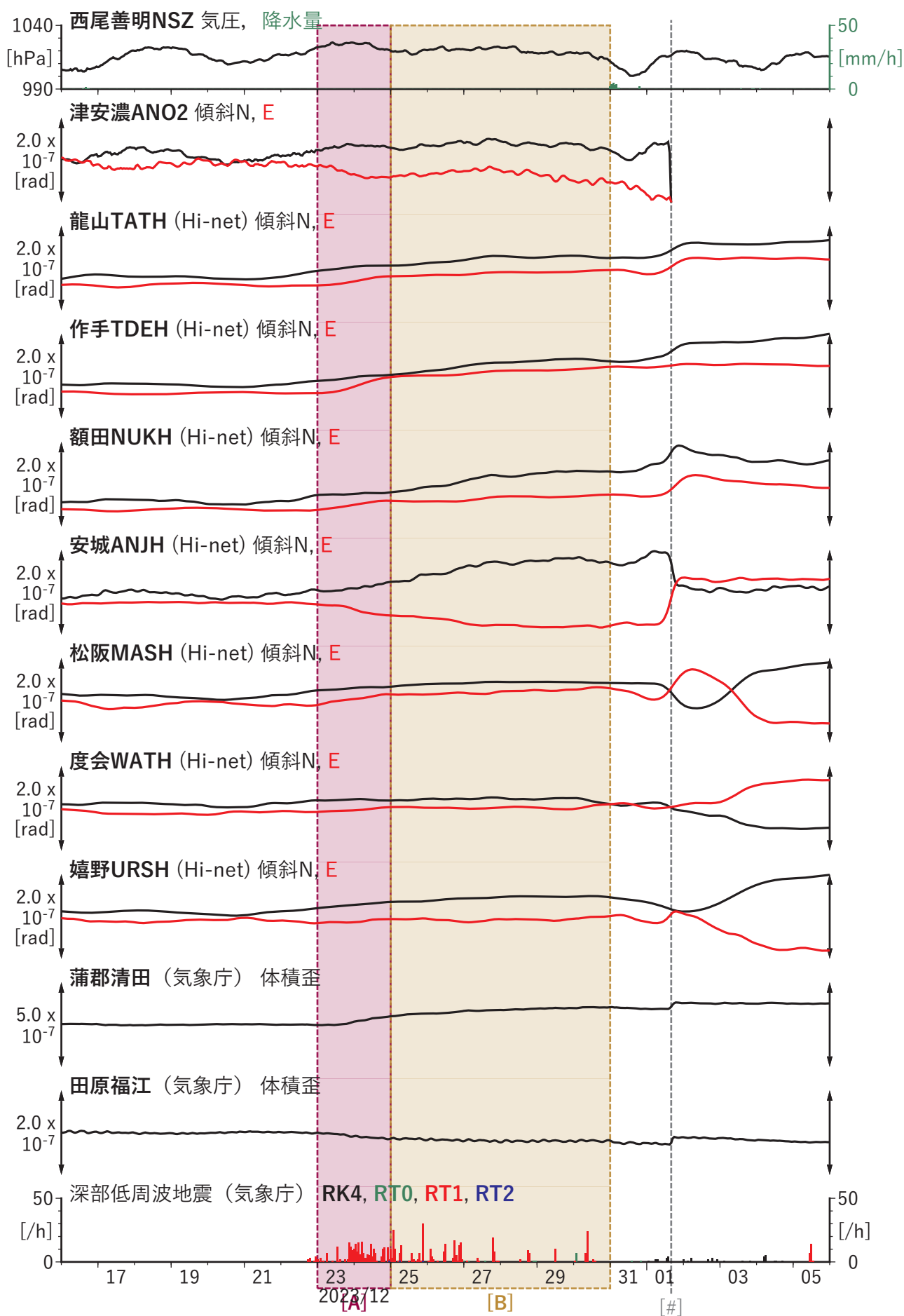
図2 歪・傾斜の時間変化(4) (2023/12/16 00:00-2024/01/06 00:00 (JST))
