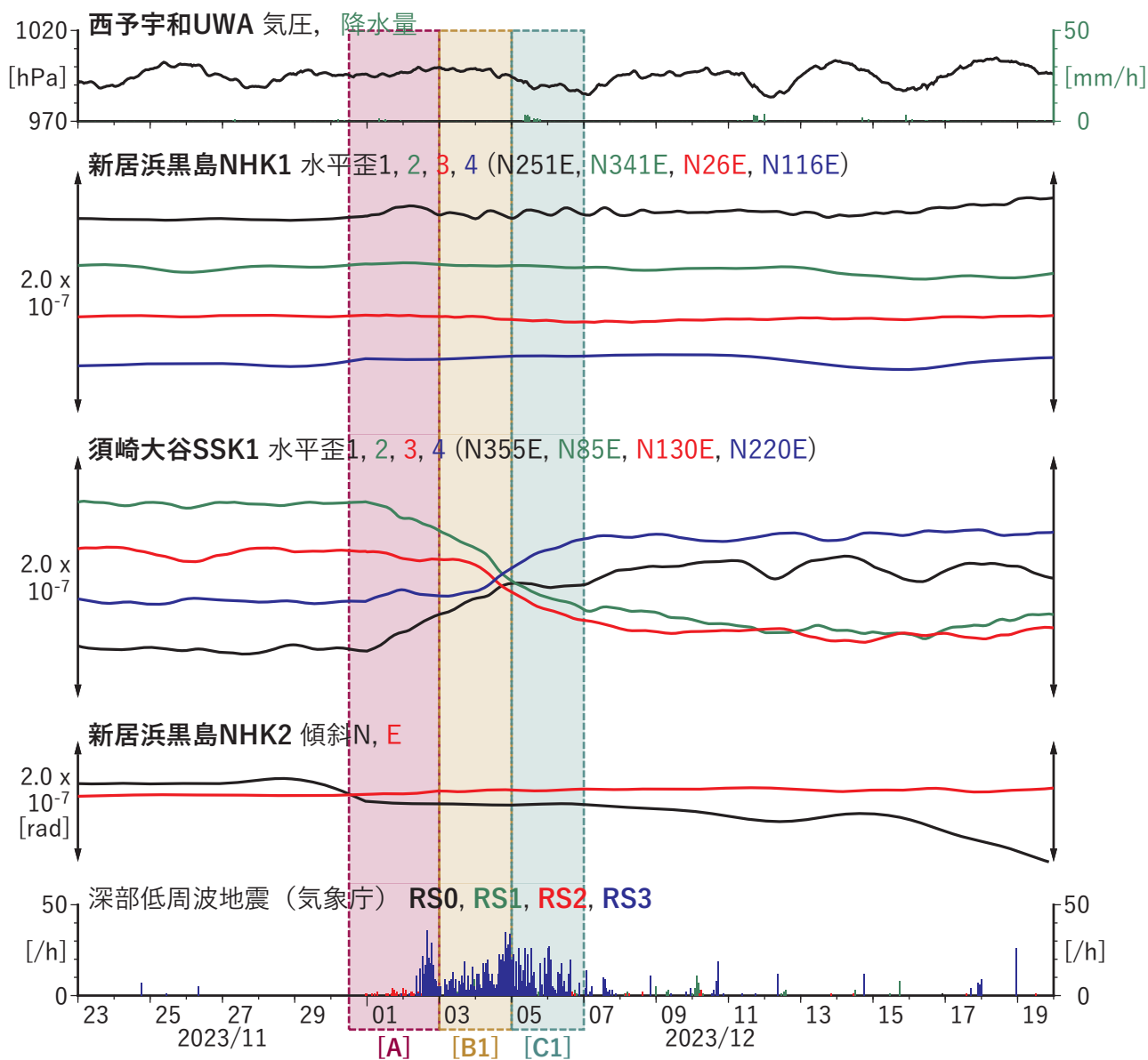
図6 歪・傾斜の時間変化(1) (2023/11/23 00:00-2023/12/20 00:00 (JST))
