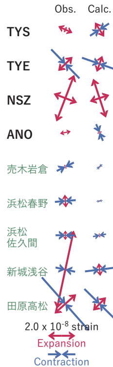
図4 2023/12/25-30の歪・傾斜変化(図2[B])を説明する断層モデル。
