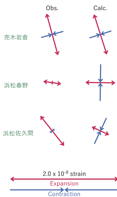
図3 2023/09/30PM - 10/02 の歪・傾斜変化（図2 [A]）を説明する断層モデル。
