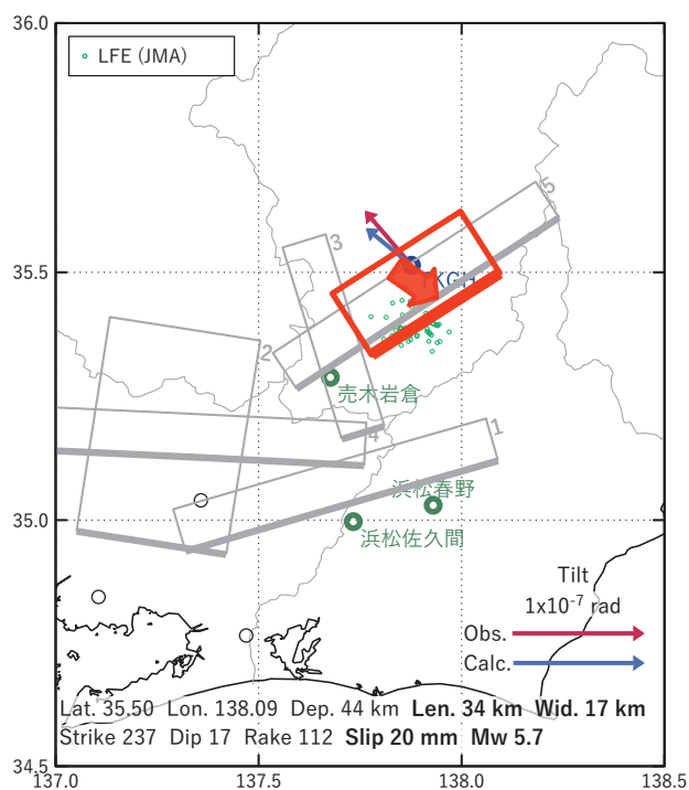
図3 2023/09/30PM - 10/02 の歪・傾斜変化（図2 [A]）を説明する断層モデル。
