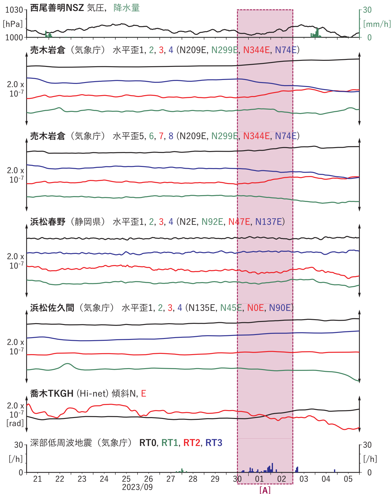
図2 東海地方における歪・傾斜の時間変化 (2023/09/21 00:00 - 2023/10/06 00:00 (JST))
