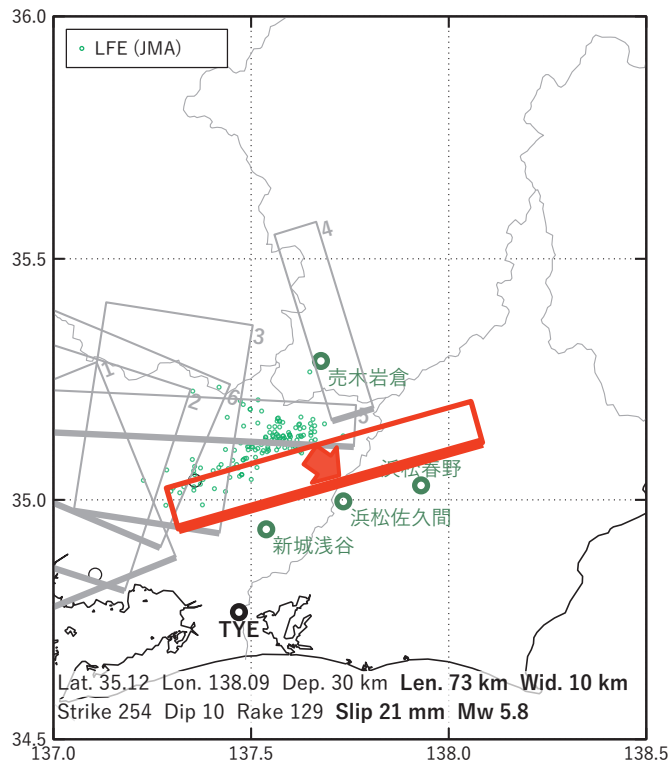
図7 2023/09/15 - 17 の歪・傾斜変化（図6 [A]）を説明する断層モデル。
