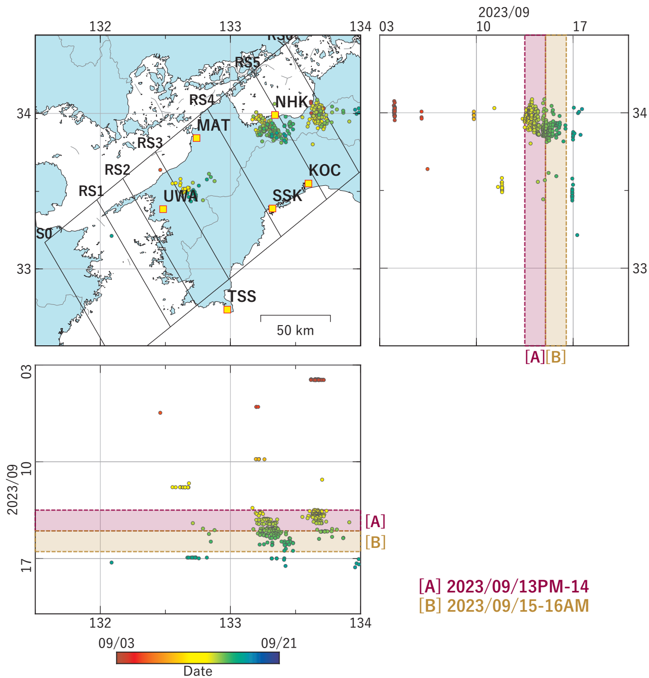
図1 四国地方における深部低周波地震の時空間分布図。 (2023/09/03 00:00 - 2023/09/21 00:00 (JST)) 気象庁カタログによる。
