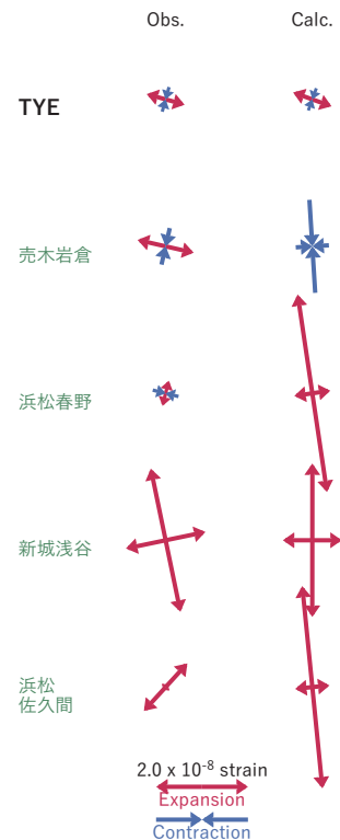
図7 2023/09/15 - 17 の歪・傾斜変化（図6 [A]）を説明する断層モデル。
