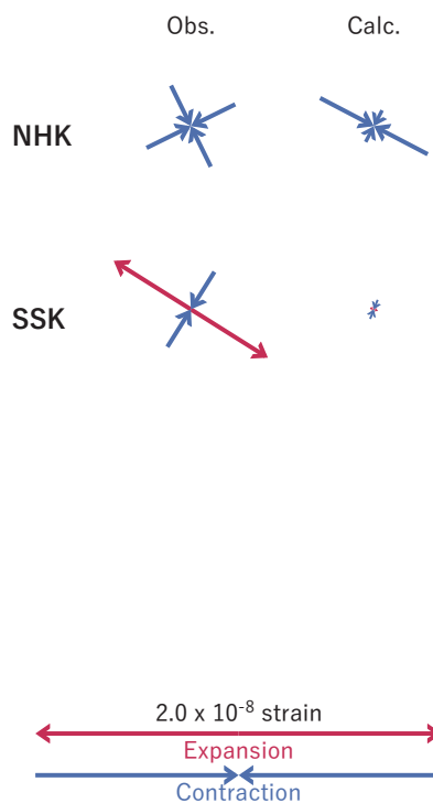
図4 2023/09/15 - 16AM の歪・傾斜変化 (図2 [B]) を説明する断層モデル。
