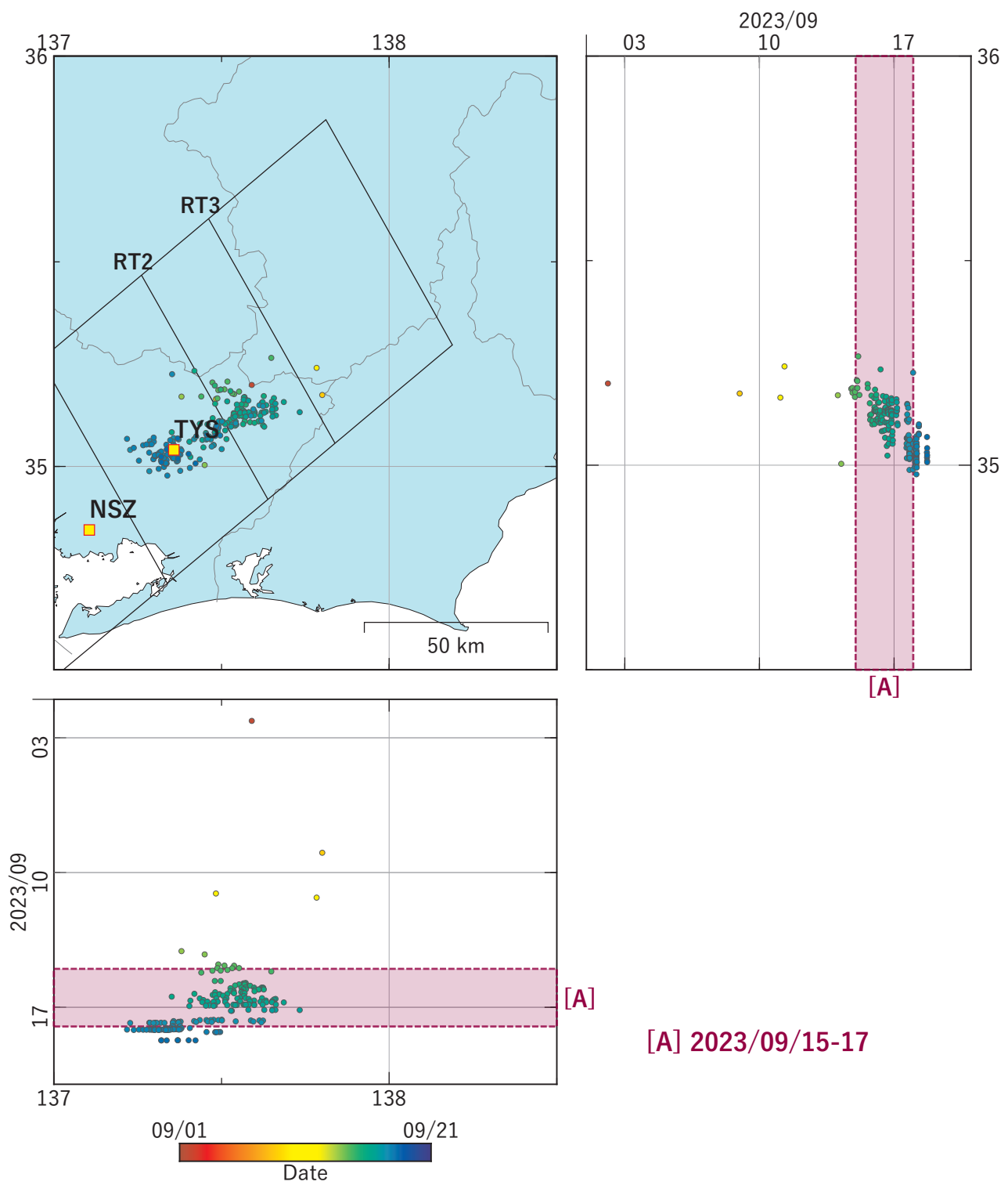
図5 東海地方における深部低周波地震の時空間分布図。 (2023/09/01 00:00 - 2023/09/21 00:00 (JST)) 気象庁カタログによる。
