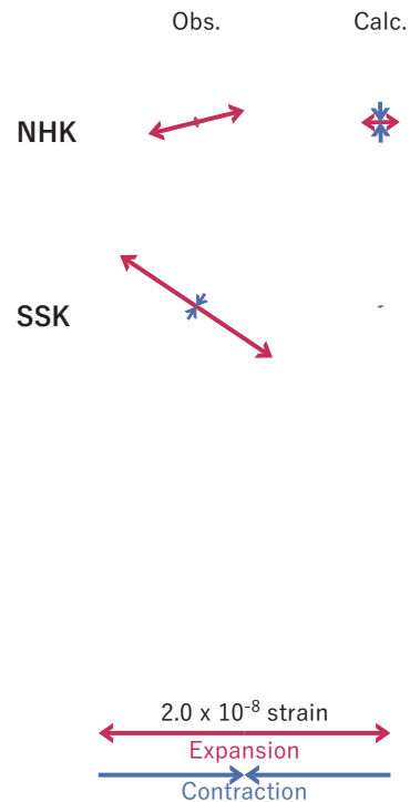
図3 2023/09/13PM - 14 の歪・傾斜変化 (図2 [A]) を説明する断層モデル。
