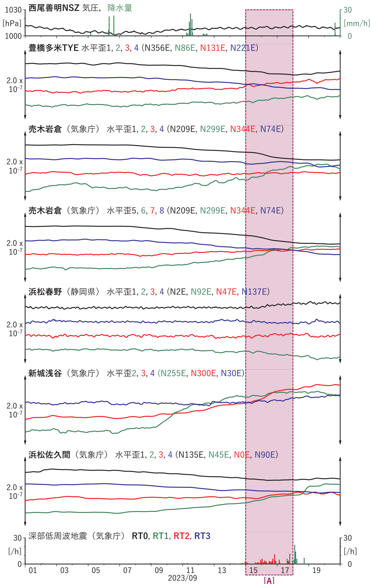
図6 東海地方における歪の時間変化 (2023/09/01 00:00 - 2023/09/21 00:00 (JST))
