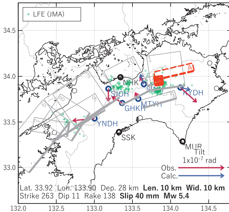
図4 2023/06/24PM-30AMの歪・傾斜変化（図2[B]）を説明する断層モデル。
