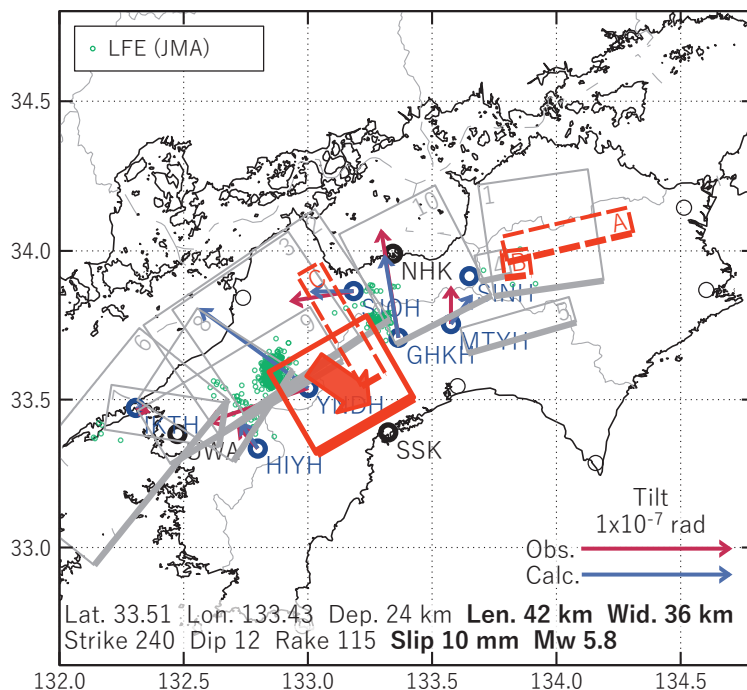
図6 2023/07/05PM-10AMの歪・傾斜変化（図2[D]）を説明する断層モデル。
