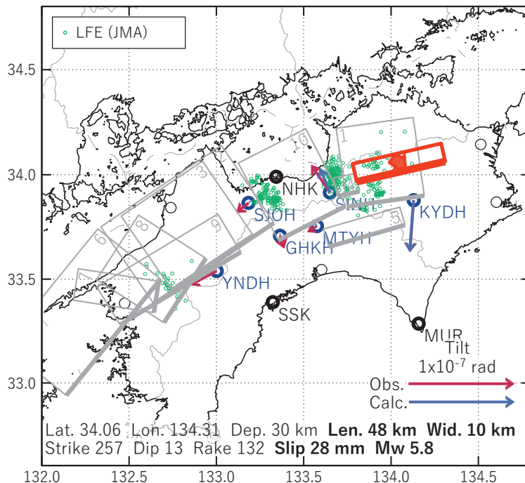
図3 2023/06/21PM-24AMの歪・傾斜変化（図2[A]）を説明する断層モデル。
