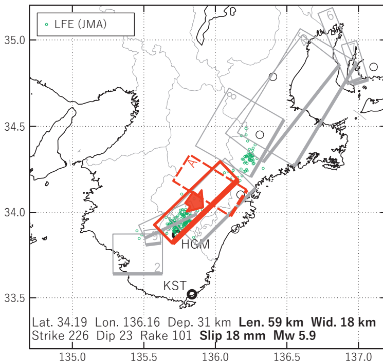
図10 2023/07/18PM-20AMの歪変化（図8[Bsw]）を説明する断層モデル。
