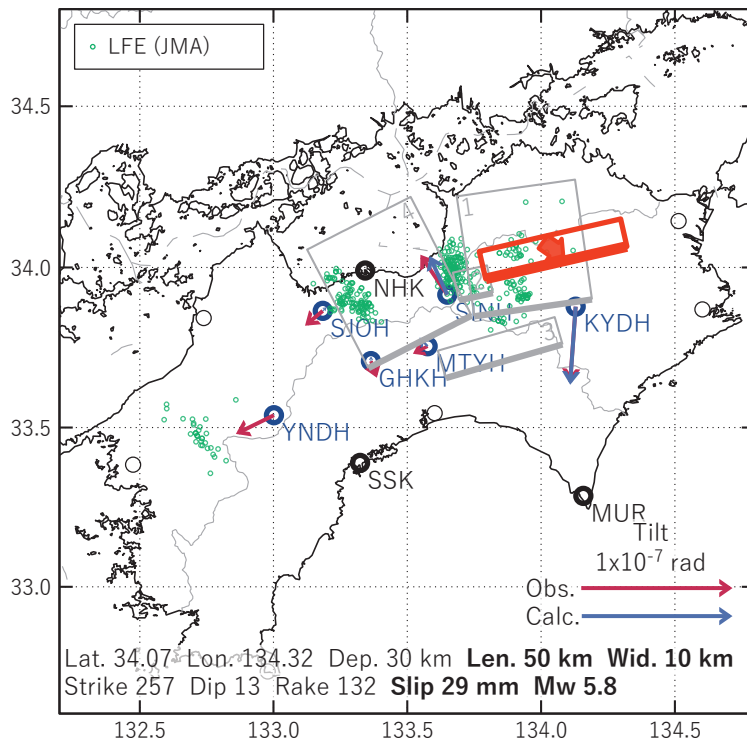
図6 2023/06/21PM-24AMの歪・傾斜変化（図5[A]）を説明する断層モデル。
