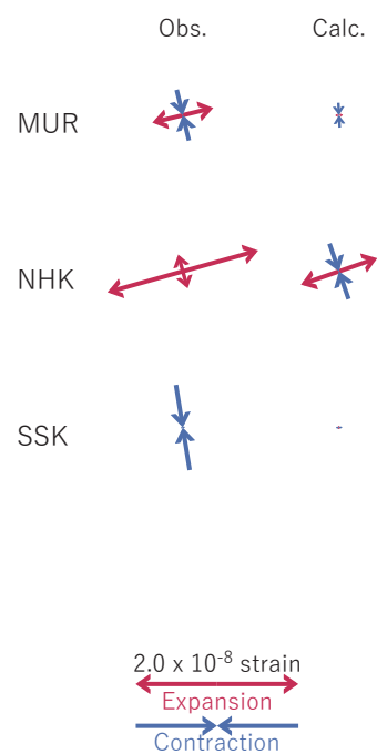
図6 2023/06/21PM-24AMの歪・傾斜変化（図5[A]）を説明する断層モデル。
