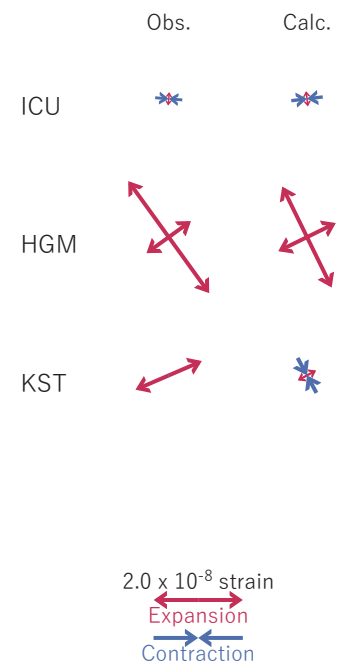
図3 2023/05/03-05の歪変化 (図2[A]) を説明する断層モデル。
