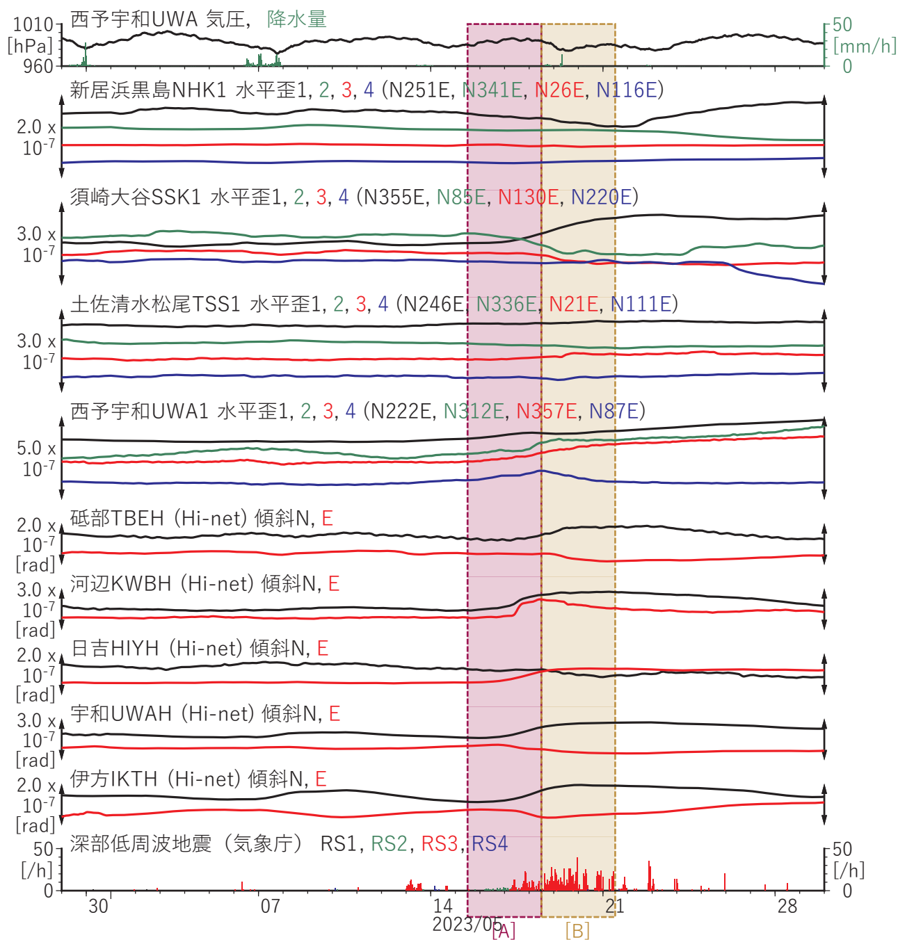
図5 四国地方における歪・傾斜観測結果 (2023/04/29 00:00 - 2023/05/30 00:00 (JST))
