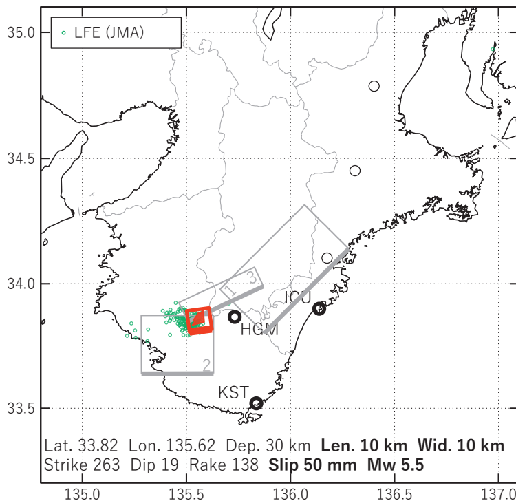
図3 2023/05/03-05の歪変化 (図2[A]) を説明する断層モデル。
