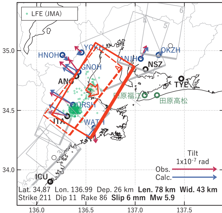
図4 2023/03/29-31の歪・傾斜・地下水位変化（図2[B]）を説明する断層モデル。
