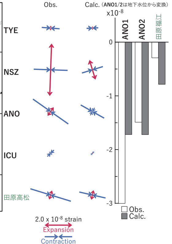
図4 2023/03/29-31の歪・傾斜・地下水位変化（図2[B]）を説明する断層モデル。
