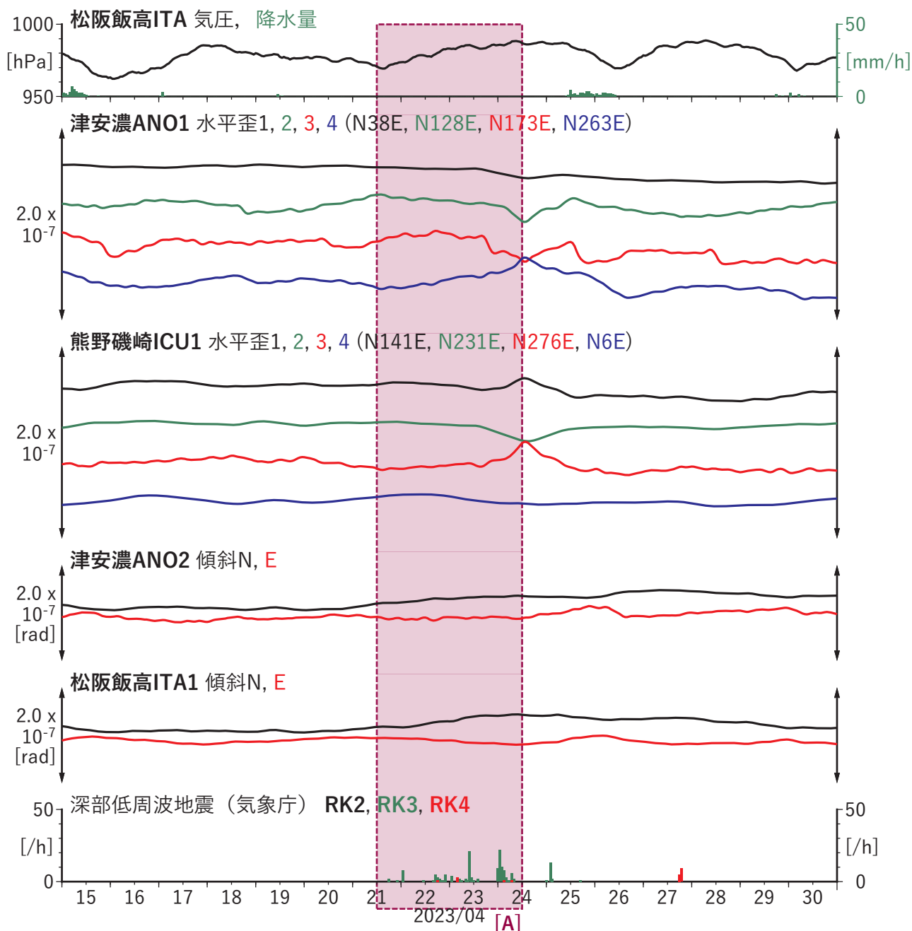
図8 歪・傾斜の時間変化(1) (2023/04/15 00:00-2023/05/01 00:00 (JST))
