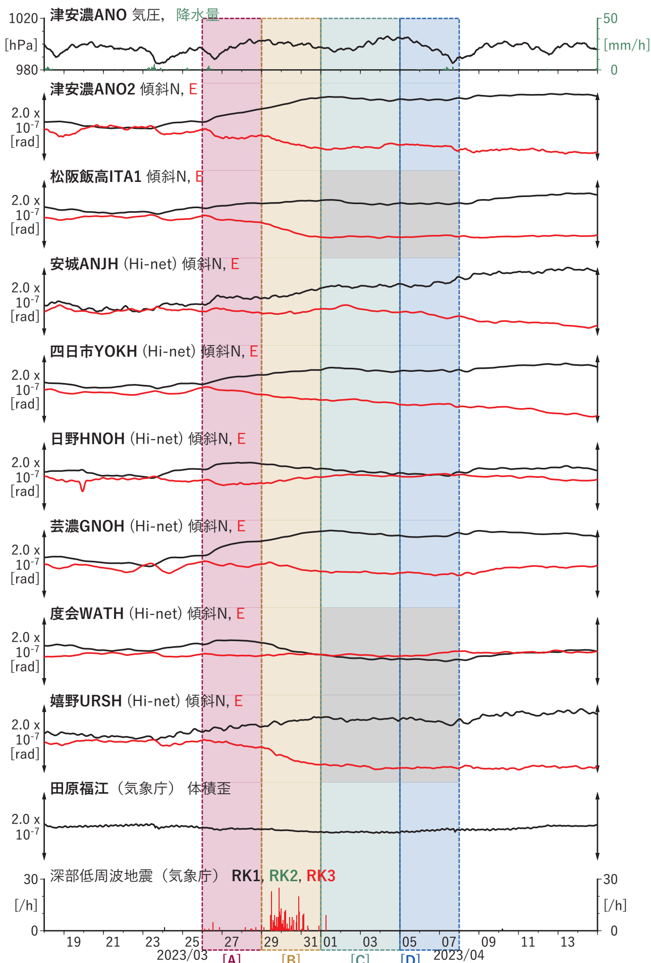
図2 歪・傾斜・地下水位の時間変化(3) (2023/03/18 00:00-2023/04/15 00:00 (JST))
