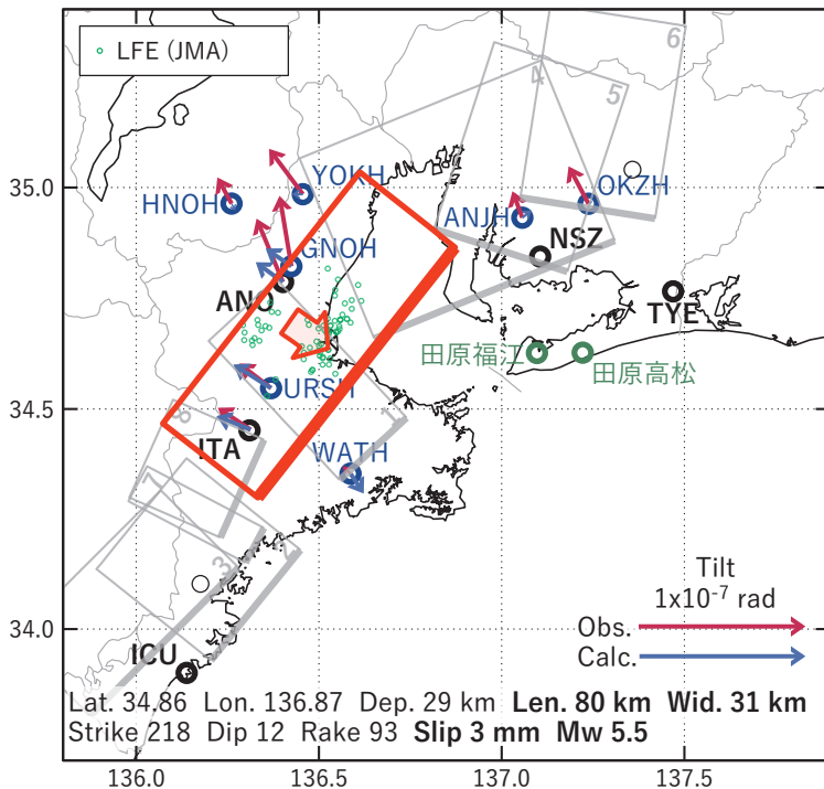
図3 2023/03/26-28の歪・傾斜・地下水位変化（図2[A]）を説明する断層モデル。
