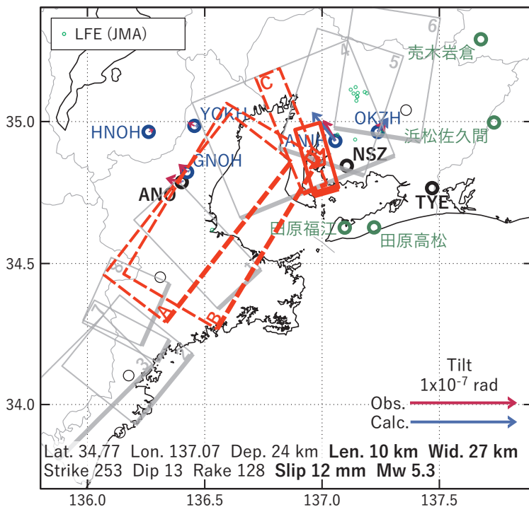
図6 2023/04/05-07の歪・傾斜変化 (図2[D]) を説明する断層モデル。
