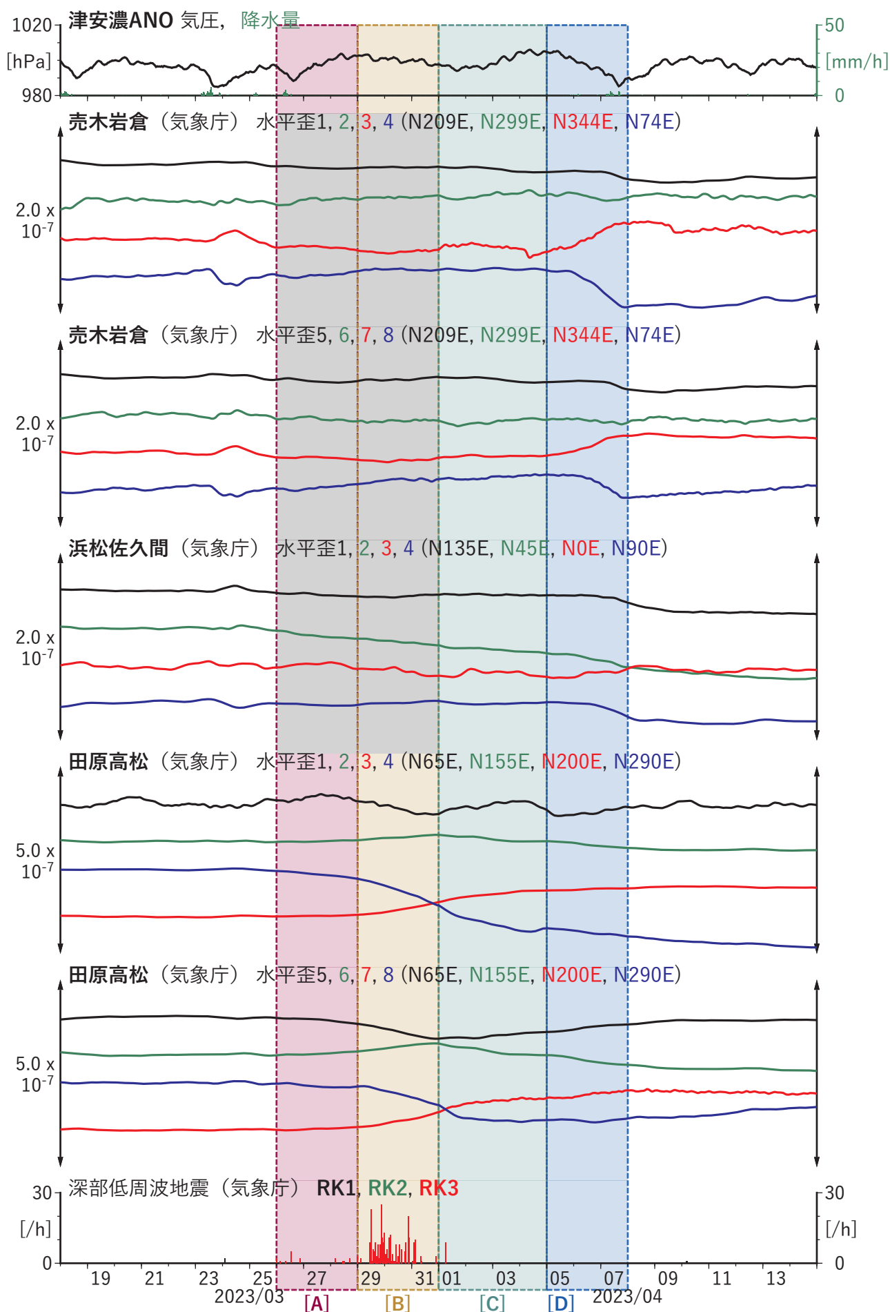
図2 歪・傾斜・地下水位の時間変化(2) (2023/03/18 00:00-2023/04/15 00:00 (JST))
