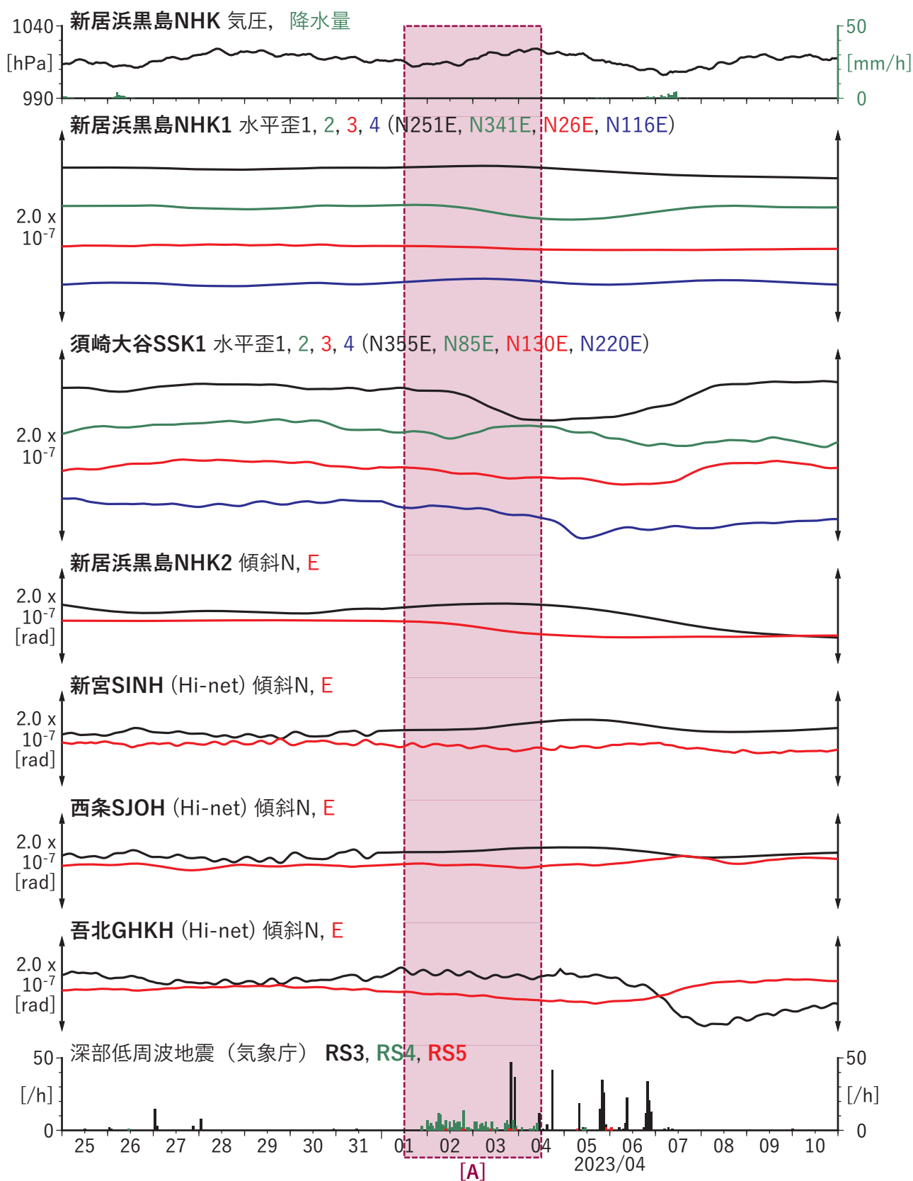
図11 歪・傾斜の時間変化 (2023/03/25 00:00-2023/04/11 00:00 (JST))
