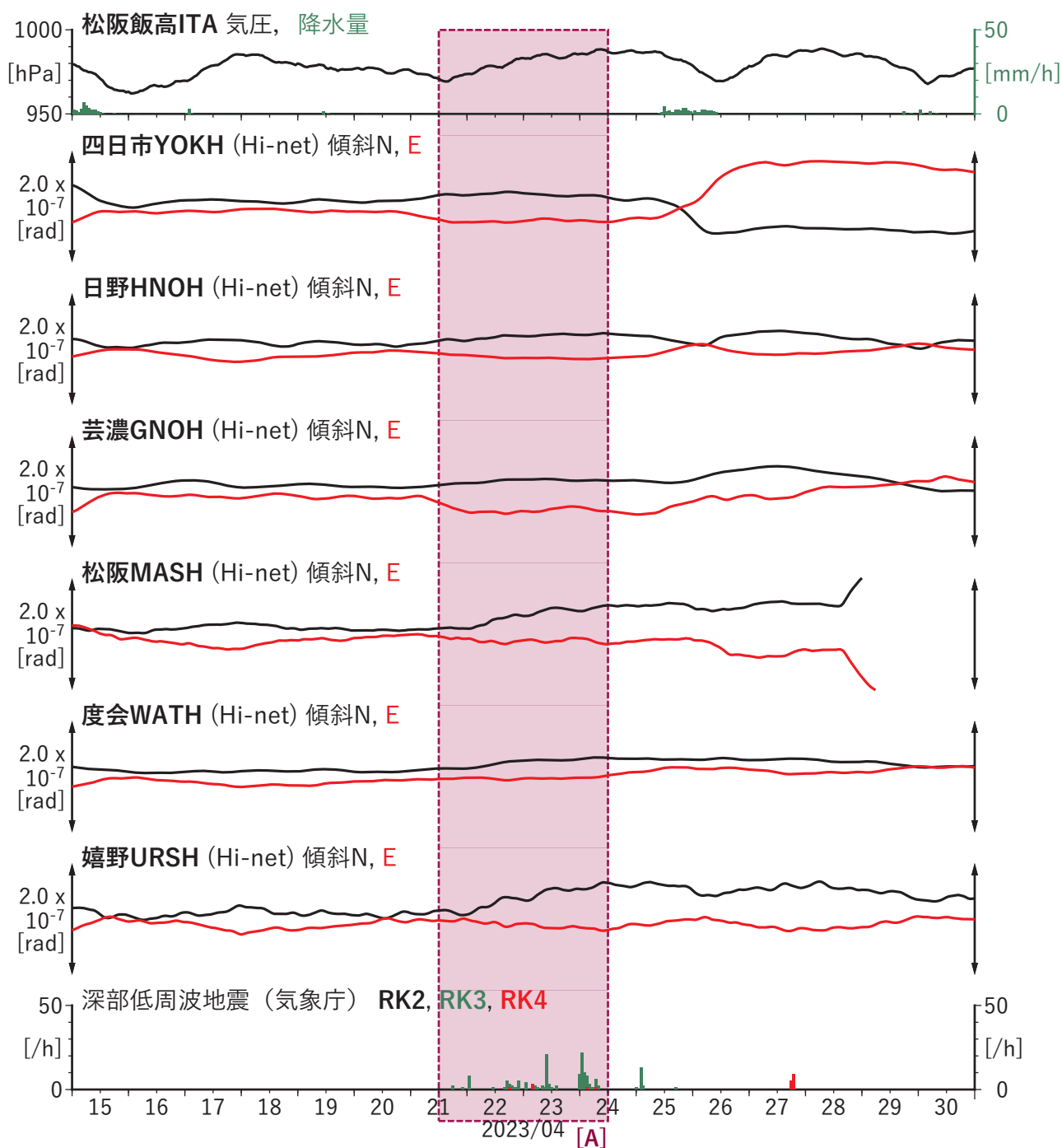
図8 歪・傾斜の時間変化(2) (2023/04/15 00:00-2023/05/01 00:00 (JST))
