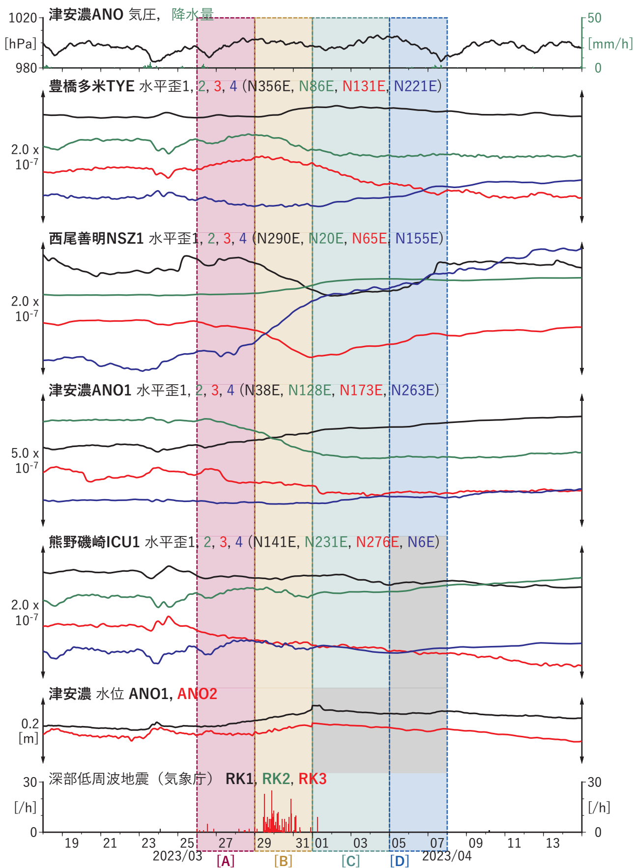
図2 歪・傾斜・地下水位の時間変化(1) (2023/03/18 00:00-2023/04/15 00:00 (JST))
