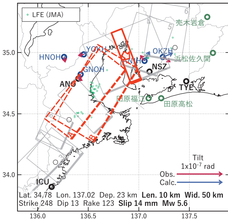
図5 2023/04/01-04の歪・傾斜変化 (図2[C]) を説明する断層モデル。
