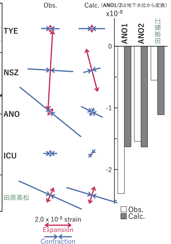
図6 2023/03/26-04/01の歪・傾斜・地下水位変化（図5[A]）を説明する断層モデル。
