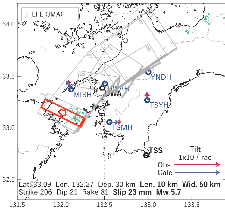
図3 2023/02/15-17AMの歪・傾斜変化（図2[A]）を説明する断層モデル。
