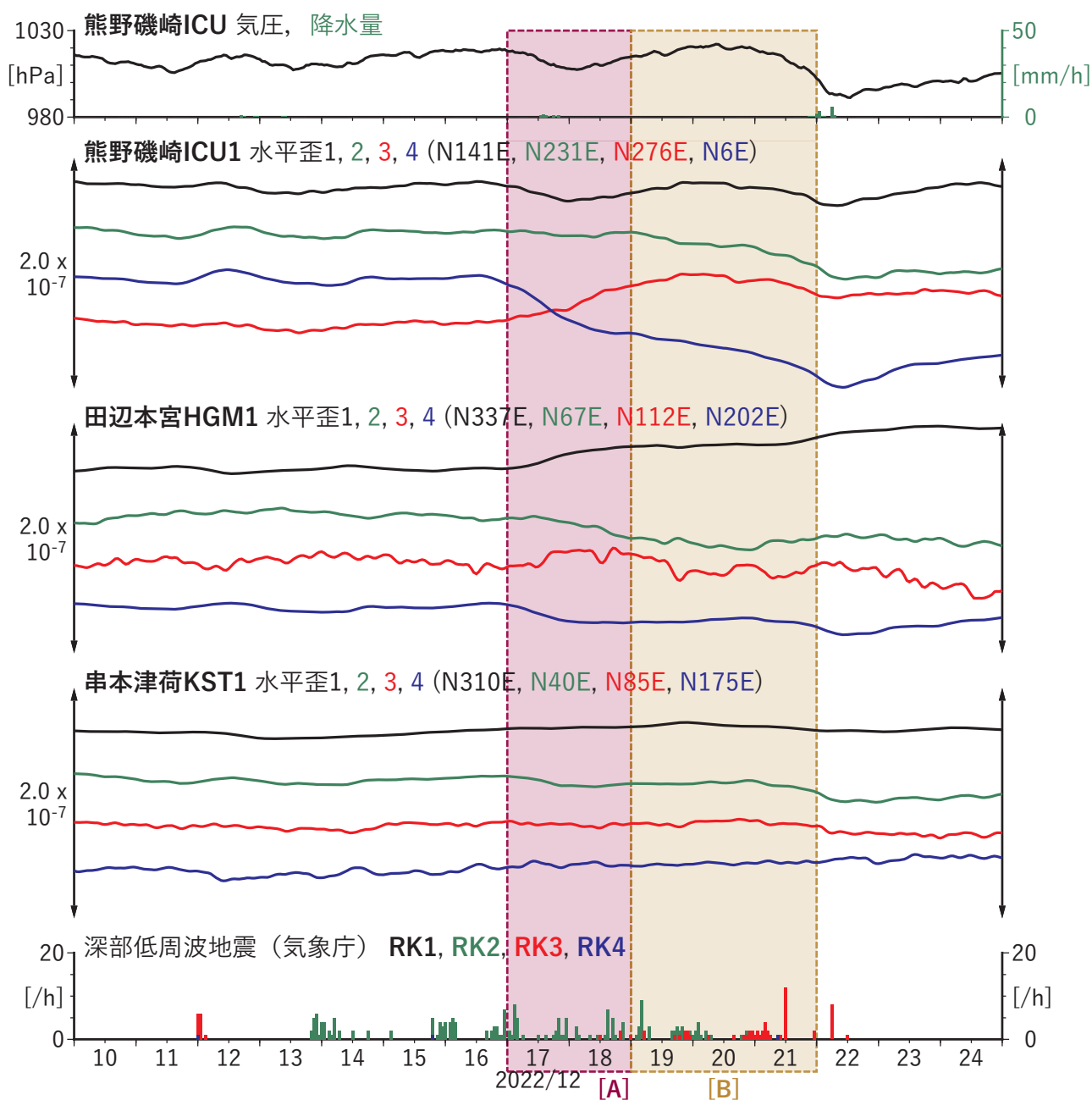
図2 歪・傾斜の時間変化(1) (2022/12/10 00:00-2022/12/25 00:00 (JST))
