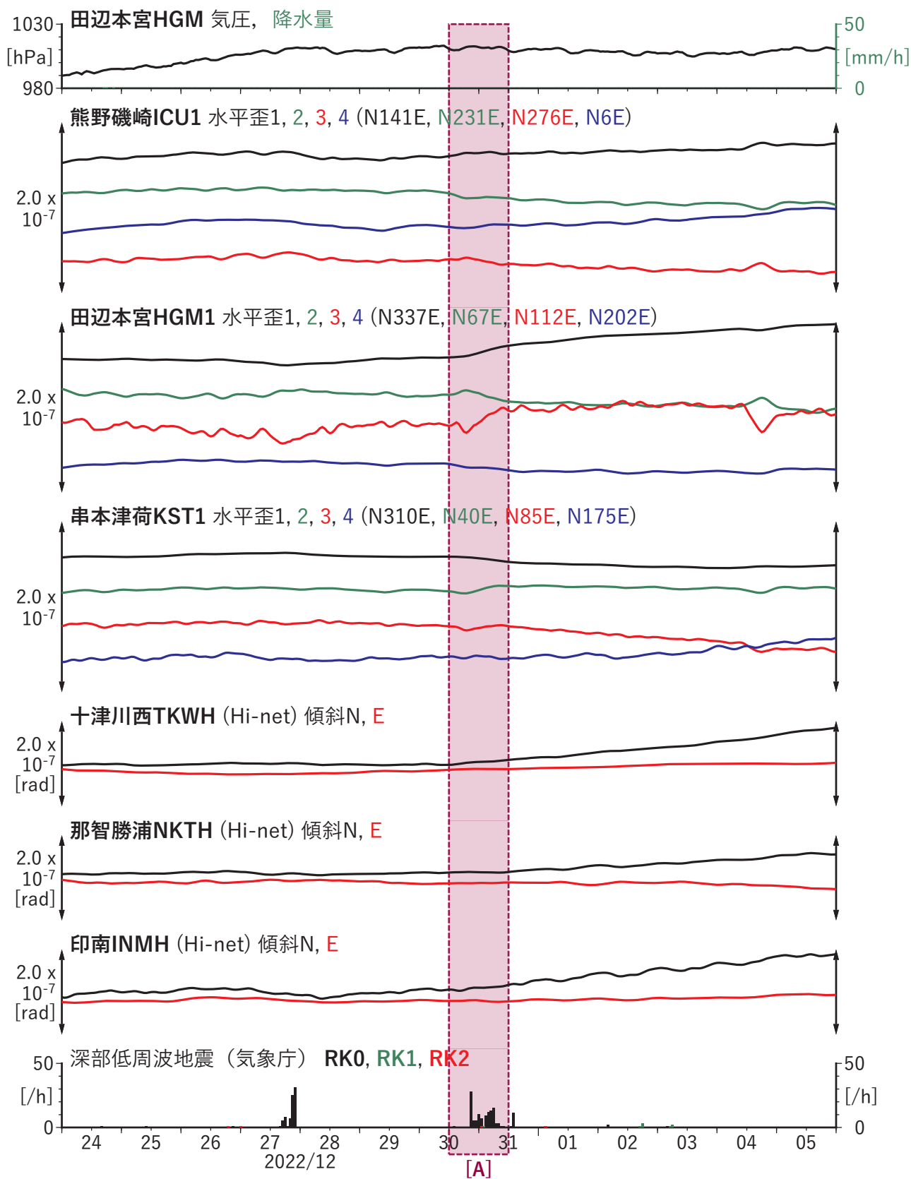
図6 歪・傾斜の時間変化 (2022/12/24 00:00-2023/01/06 00:00 (JST))
