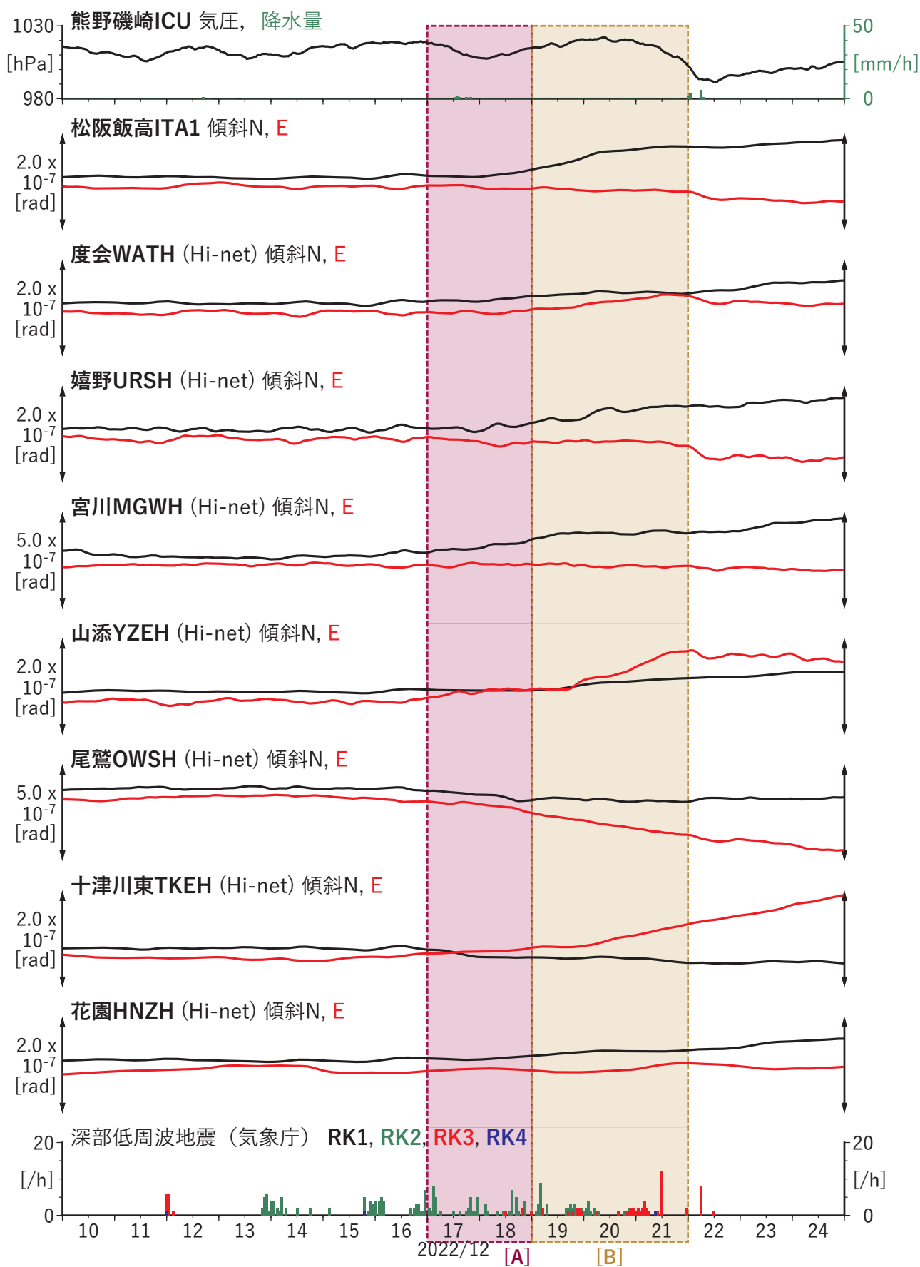
図2 歪・傾斜の時間変化(2) (2022/12/10 00:00-2022/12/25 00:00 (JST))
