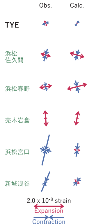
図3 2022/11/03-05の歪・傾斜変化（図2[A]）を説明する断層モデル。
