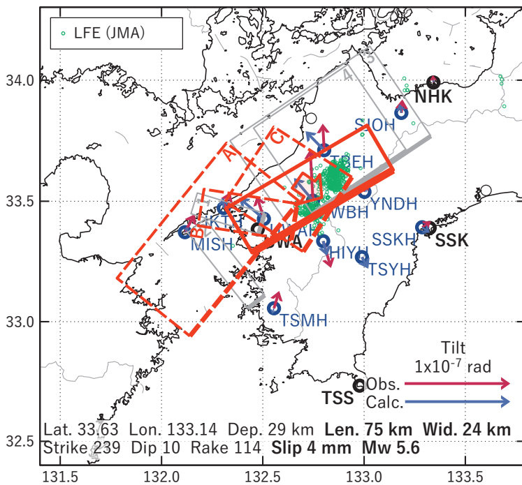
図12 2022/11/24PM-26の歪・傾斜変化（図8[D]）を説明する断層モデル。
