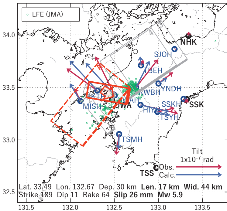
図10 2022/11/18PM-20の歪・傾斜変化（図8[B]）を説明する断層モデル。
