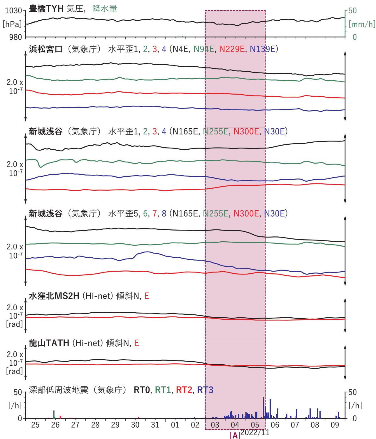
図2 歪・傾斜の時間変化(2) (2022/10/25 00:00-2022/11/10 00:00 (JST))
