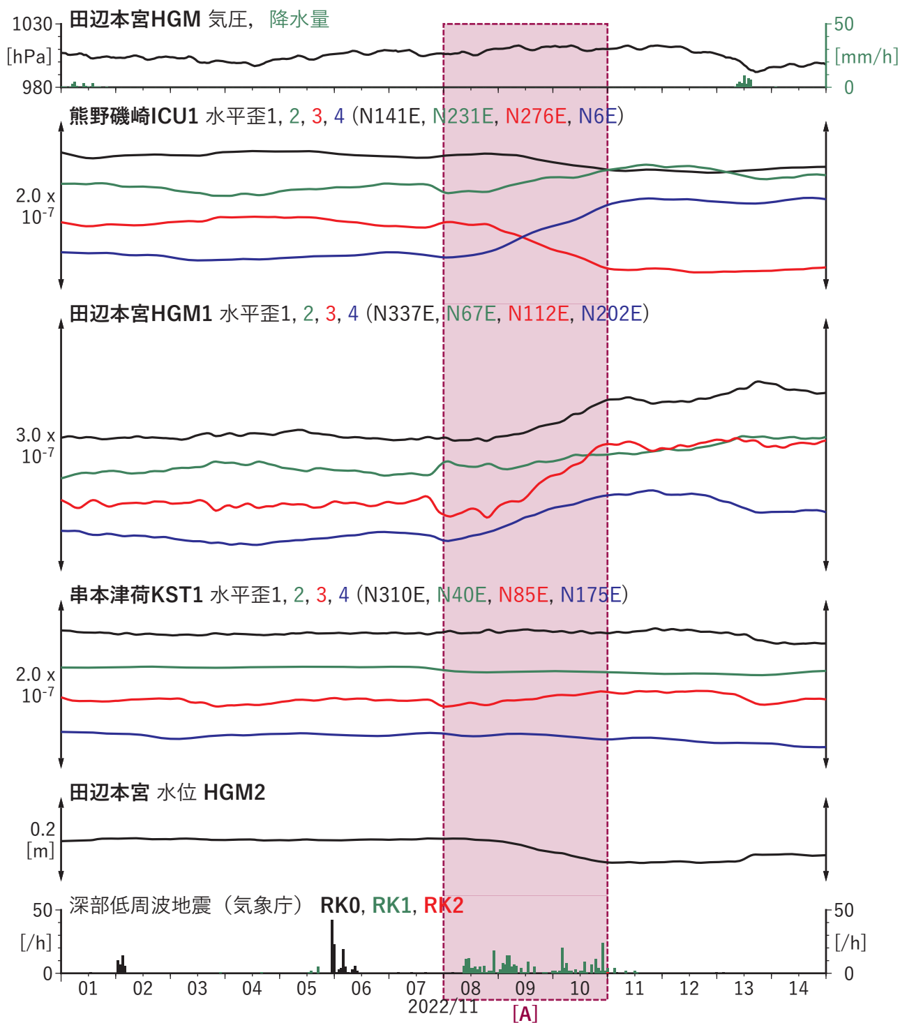
図5 歪・傾斜・地下水位の時間変化(1) (2022/11/01 00:00-2022/11/15 00:00 (JST))
