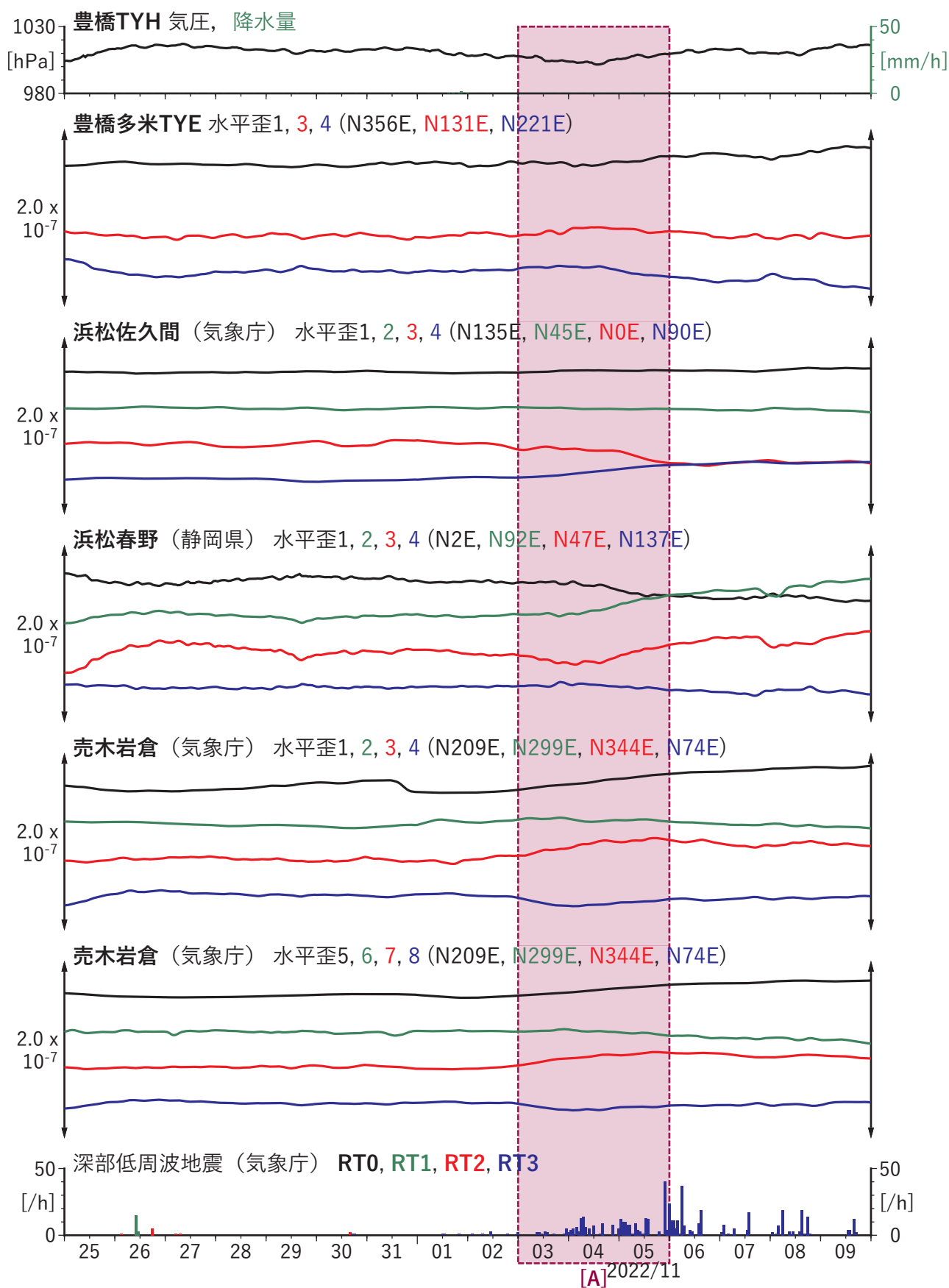
図2 歪・傾斜の時間変化(1) (2022/10/25 00:00-2022/11/10 00:00 (JST))
