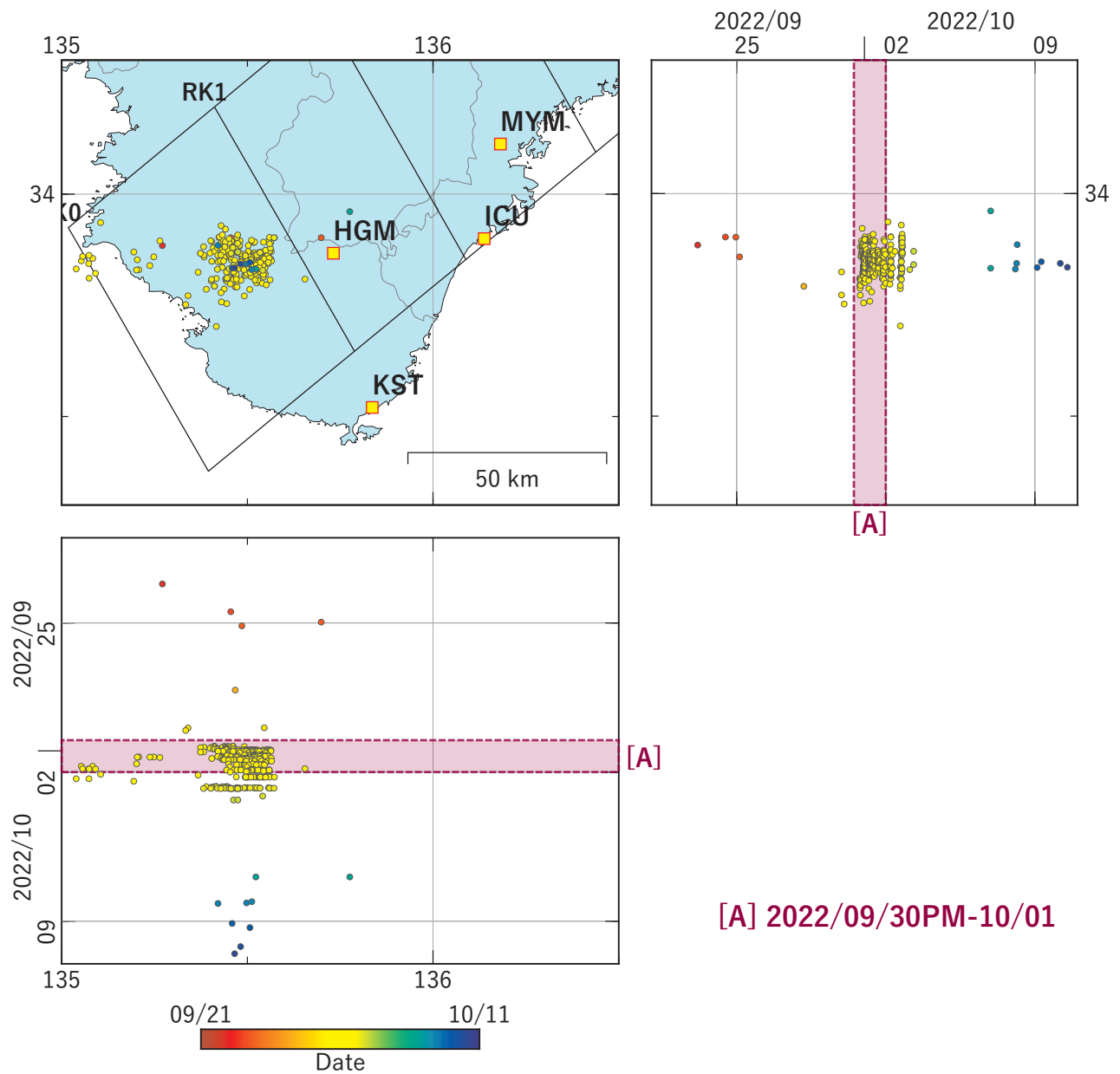
図1 紀伊半島における深部低周波地震の時空間分布図。 (2022/09/21 00:00 - 2022/10/11 00:00 (JST)) 気象庁カタログによる。
