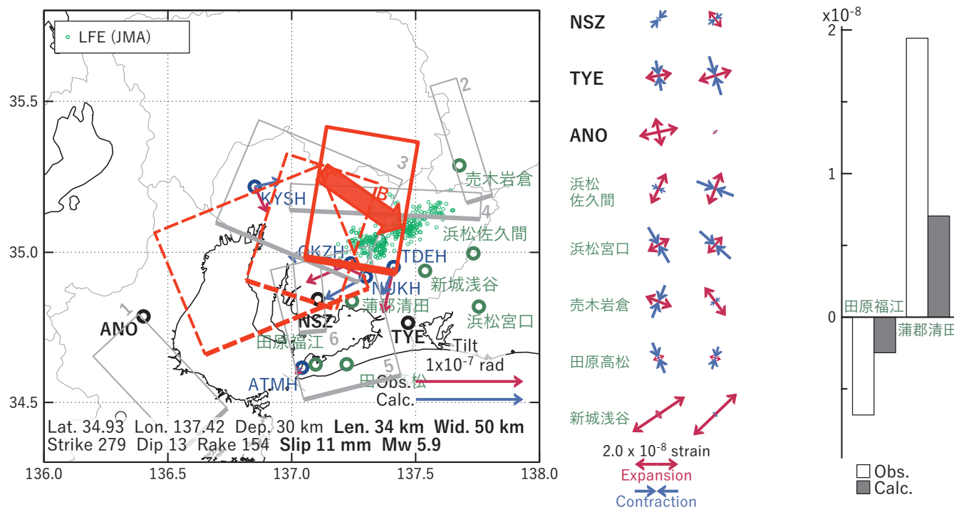
図15 2022/10/19-23AMの歪・傾斜変化（図10, 11, 12 [C]）を説明する断層モデル。
