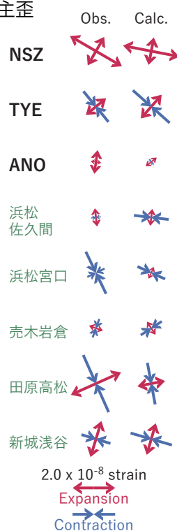
図14 2022/10/16-18の歪・傾斜変化 (図10, 11, 12 [B]) を説明する断層モデル。
