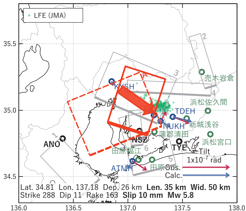
図14 2022/10/16-18の歪・傾斜変化 (図10, 11, 12 [B]) を説明する断層モデル。
