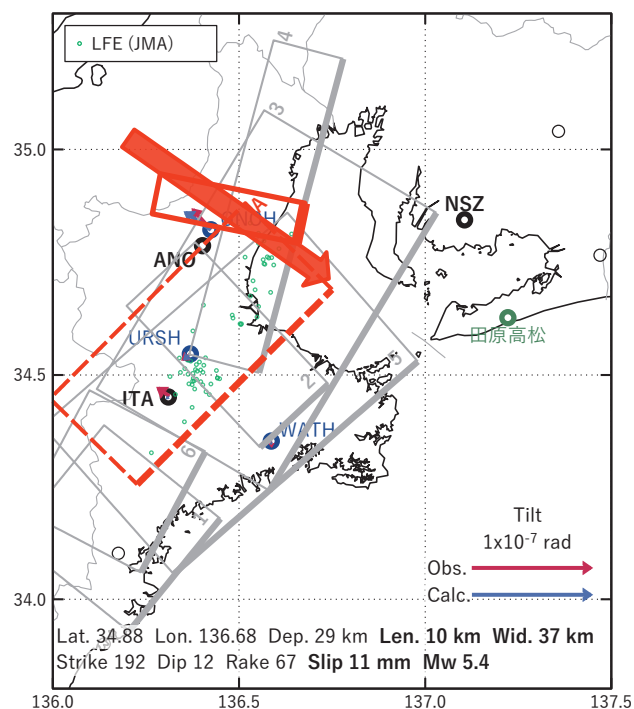
図8 2022/10/03PM-04 の歪・傾斜変化（図5, 6 [B]）を説明する断層モデル。
