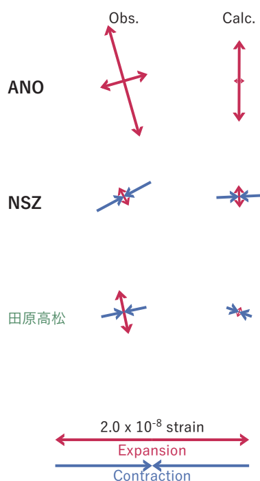
図8 2022/10/03PM-04 の歪・傾斜変化（図5, 6 [B]）を説明する断層モデル。
