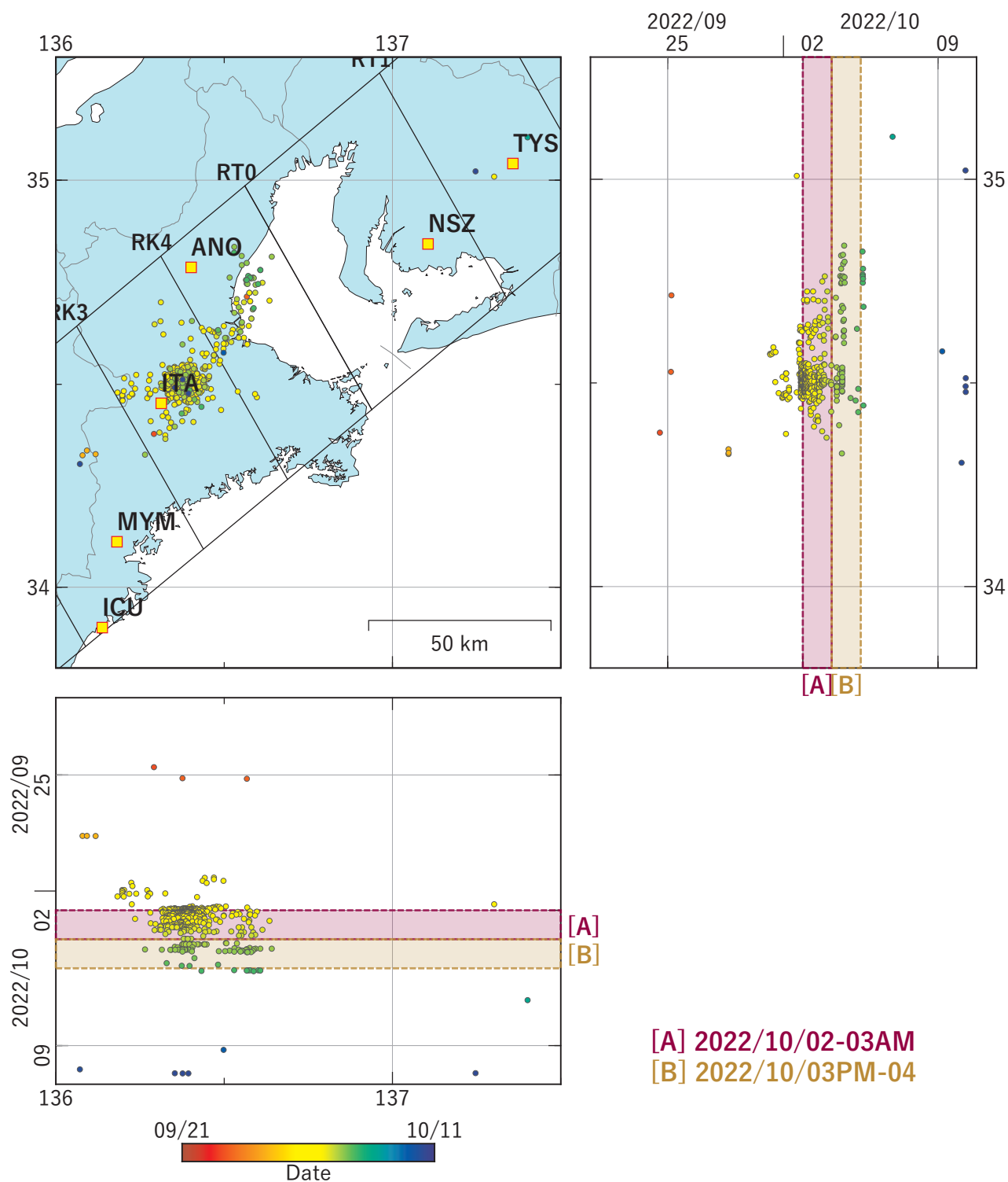
図4 紀伊半島から東海地方における深部低周波地震の時空間分布図。 (2022/09/21 00:00 - 2022/10/11 00:00 (JST)) 気象庁カタログによる。
