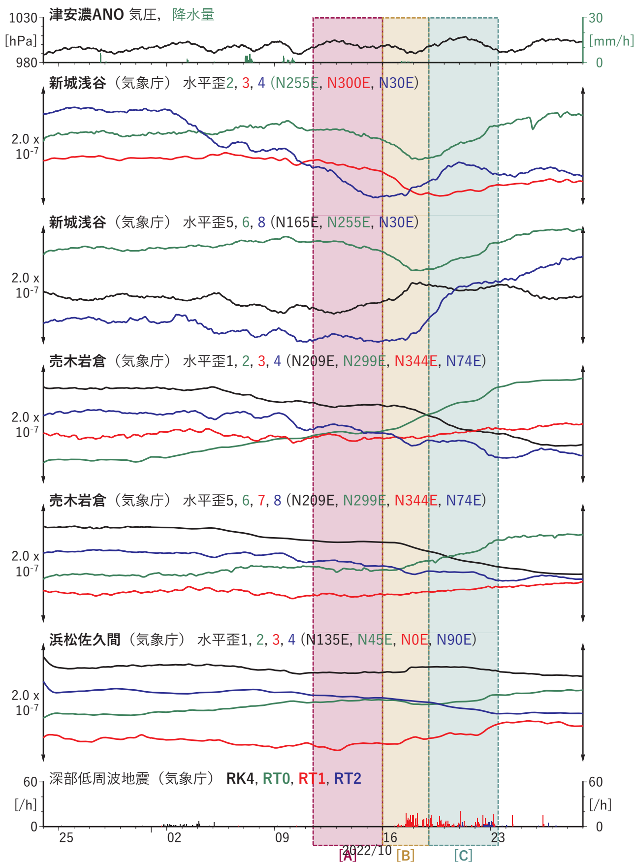
図11 紀伊半島から東海地方における歪・傾斜の時間変化 (2) (2022/09/24 00:00 - 2022/10/29 00:00 (JST))
