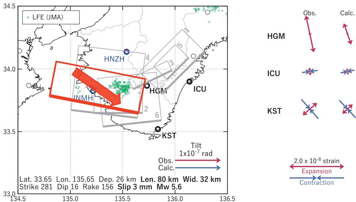
図3 2022/09/30PM - 10/01 の歪・傾斜変化（図2 [A]）を説明する断層モデル。
