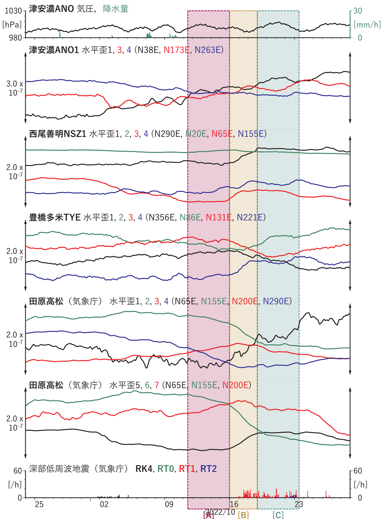
図10 紀伊半島から東海地方における歪・傾斜の時間変化 (1) (2022/09/24 00:00 - 2022/10/29 00:00 (JST))
