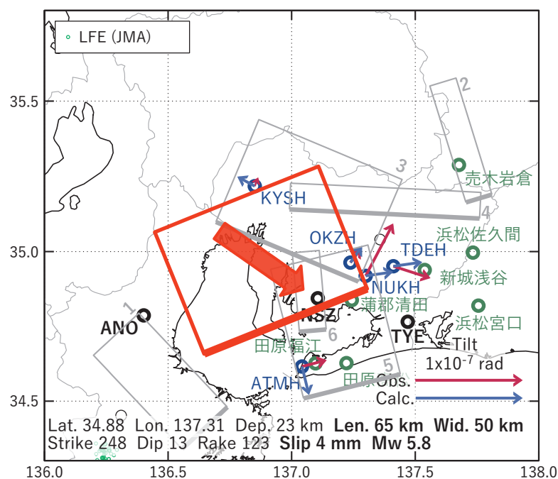
図13 2022/10/11PM-15 の歪・傾斜変化 (図10, 11, 12 [A]) を説明する断層モデル。
