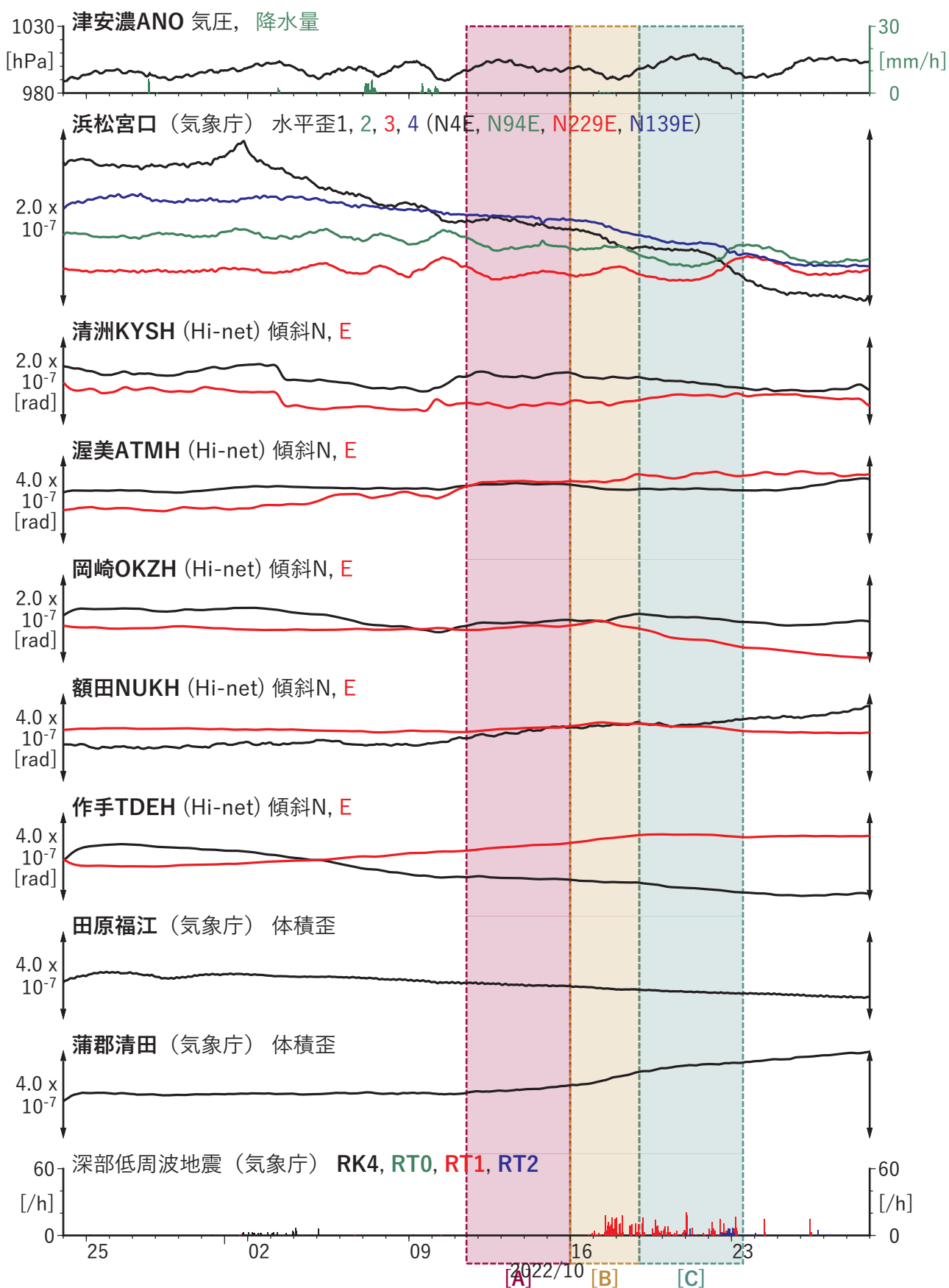
図12 紀伊半島から東海地方における歪・傾斜の時間変化 (3) (2022/09/24 00:00 - 2022/10/29 00:00 (JST))
