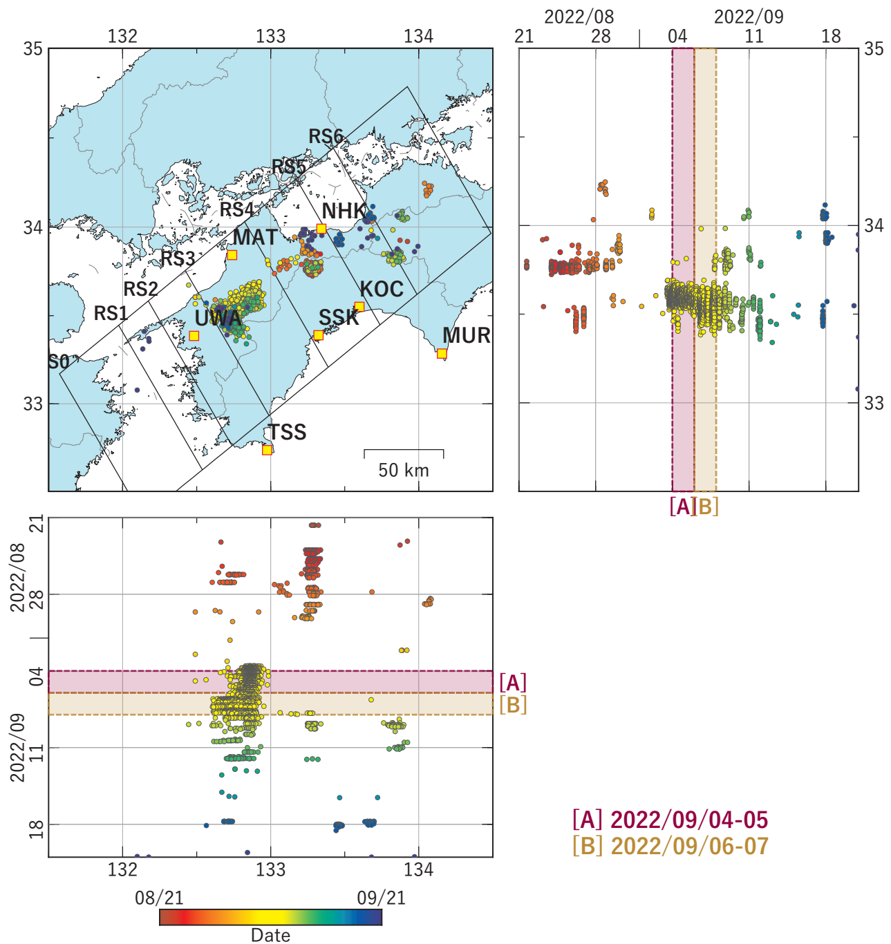
図1 四国地方における深部低周波地震の時空間分布図。 (2022/08/21 00:00 - 2022/09/21 00:00 (JST)) 気象庁カタログによる。
