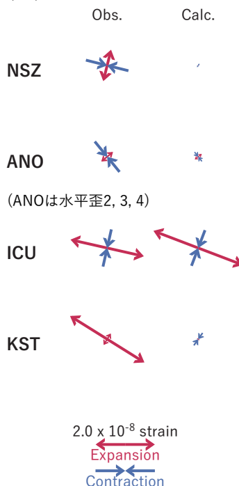
図4 2022/05/22PM-27の歪・傾斜変化（図2[B]）を説明する断層モデル。
