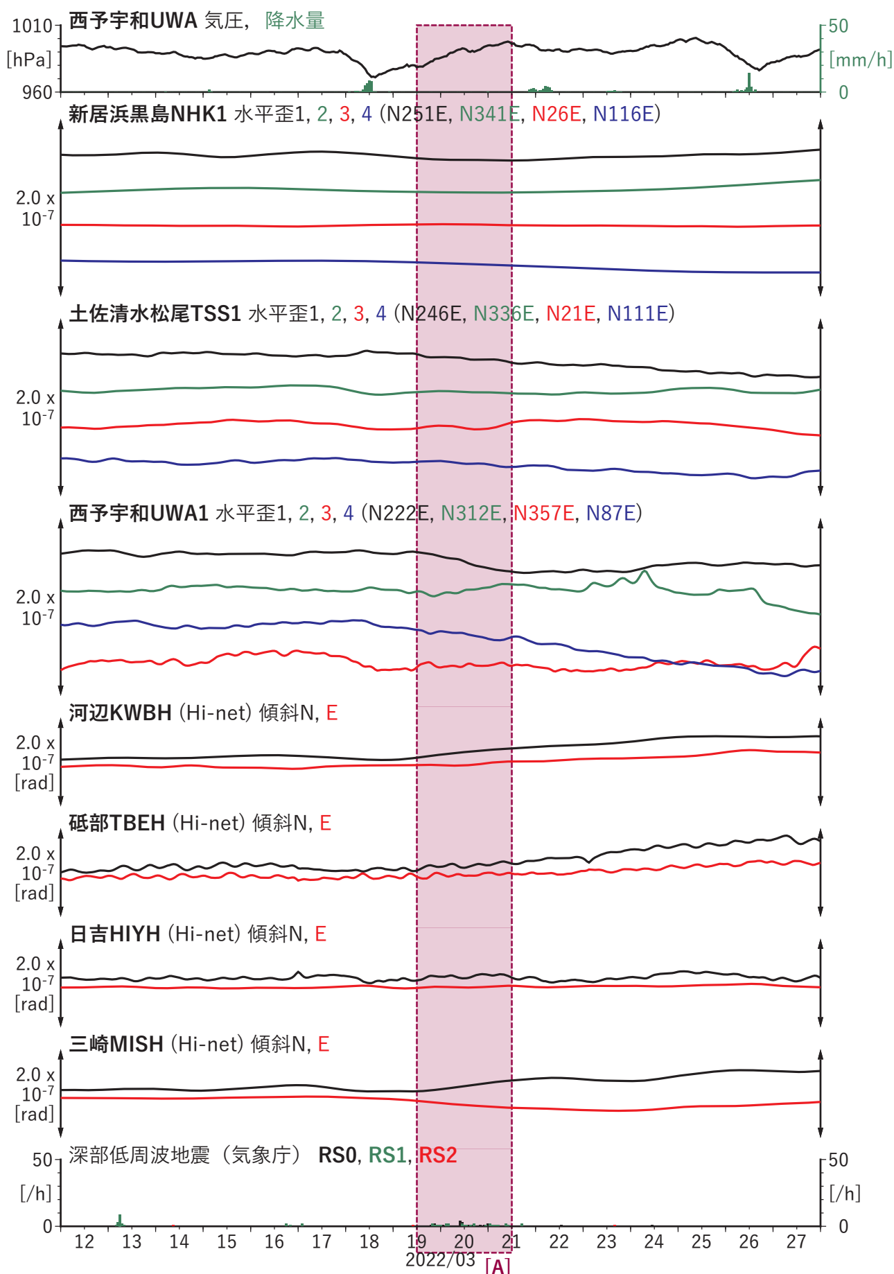
図8 歪・傾斜の時間変化 (2022/03/12 00:00-2022/03/28 00:00 (JST))
