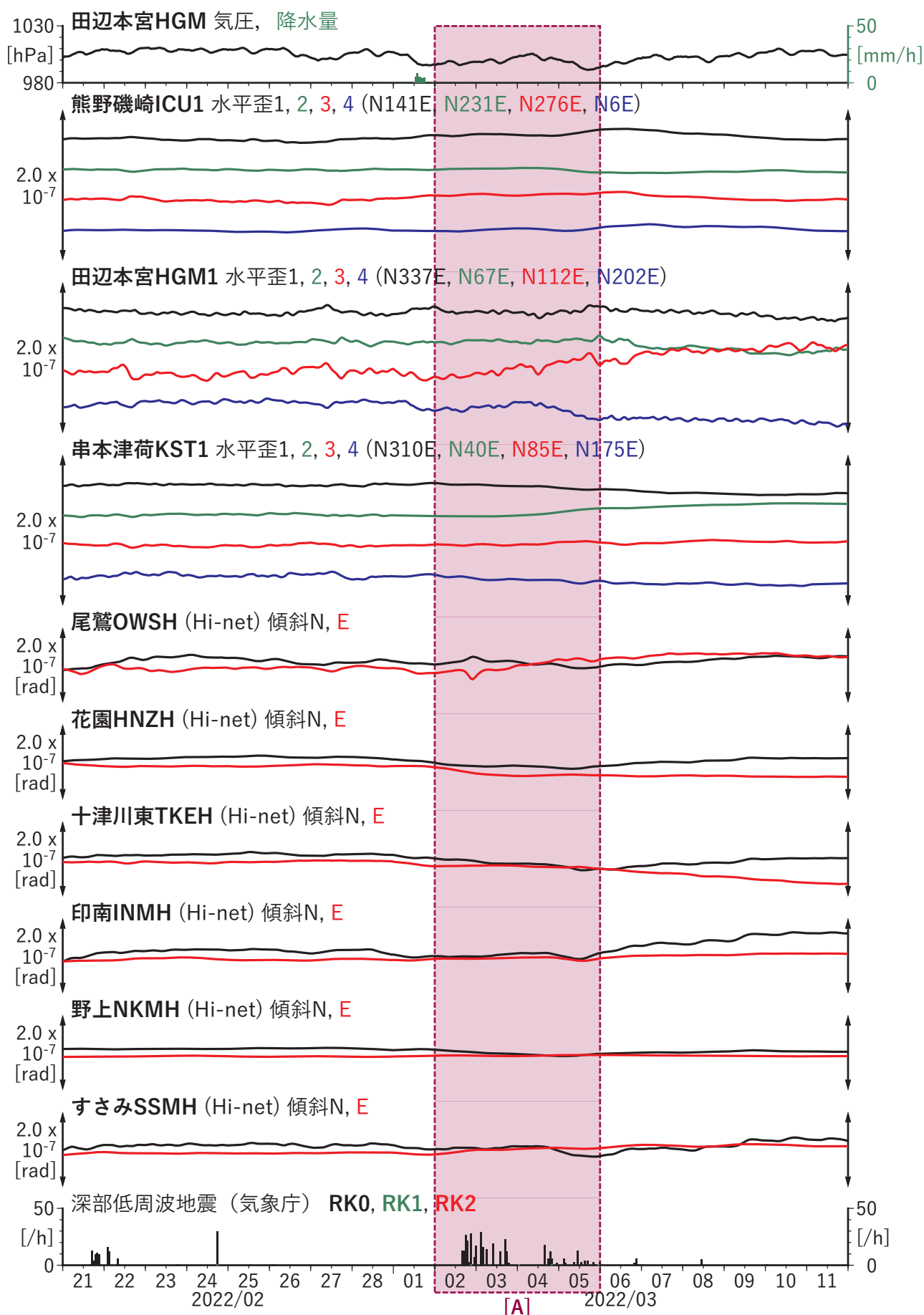
図2 歪・傾斜の時間変化 (2022/02/21 00:00-2022/03/12 00:00 (JST))
