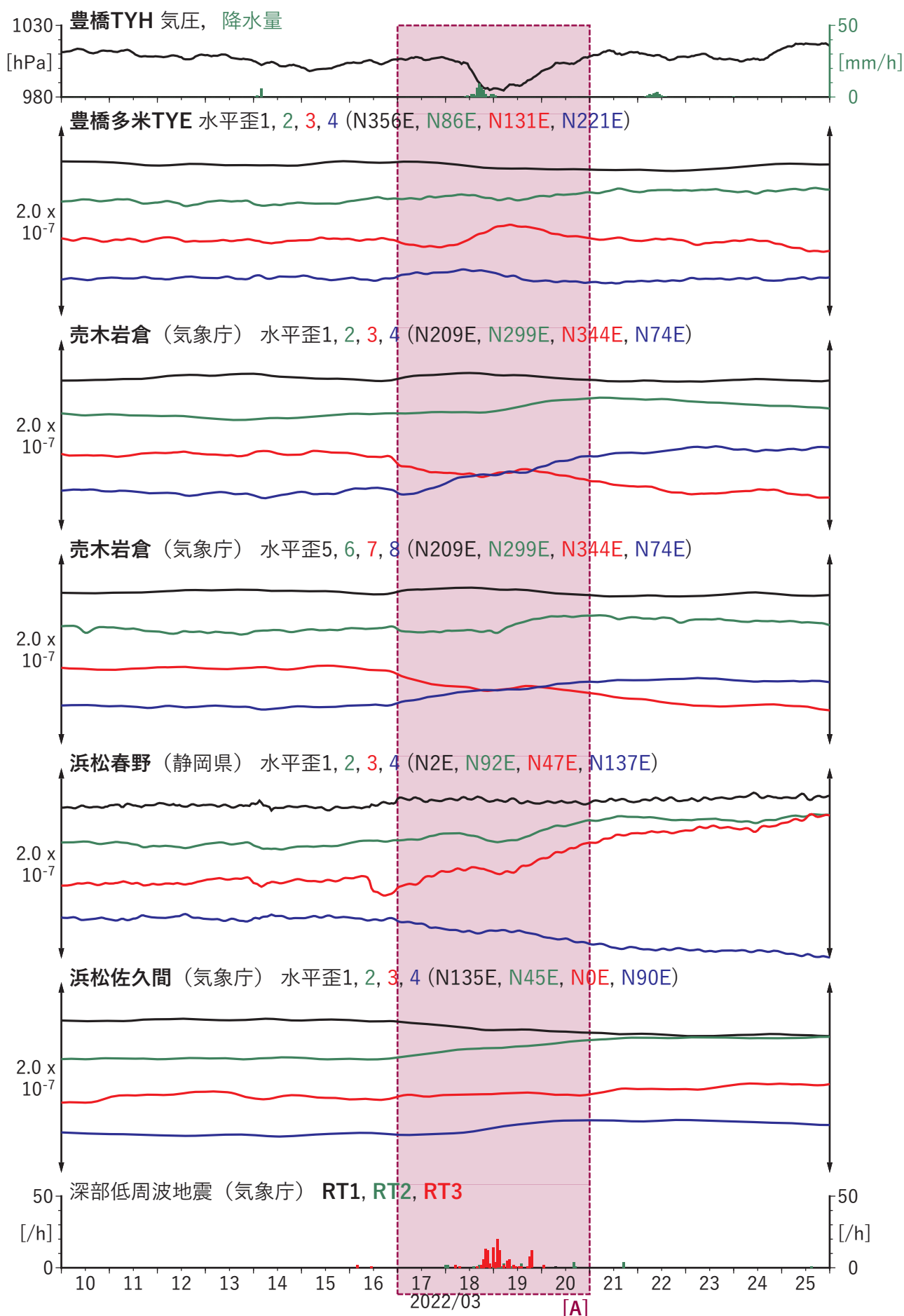
図5 歪・傾斜の時間変化(1) (2022/03/10 00:00-2022/03/26 00:00 (JST))
