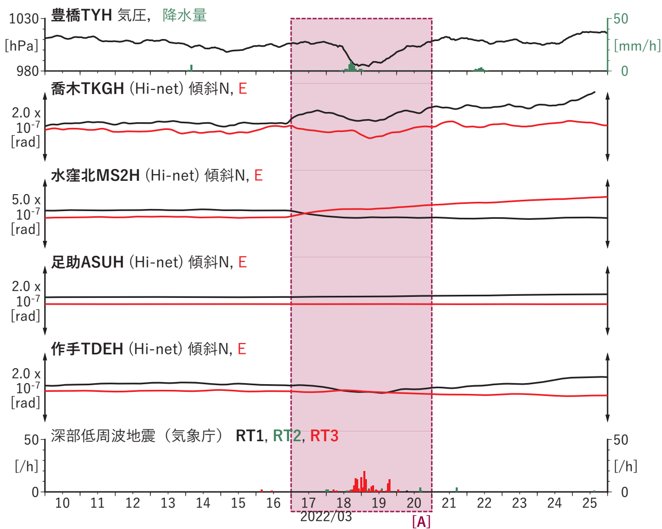
図5 歪・傾斜の時間変化(2) (2022/03/10 00:00-2022/03/26 00:00 (JST))
