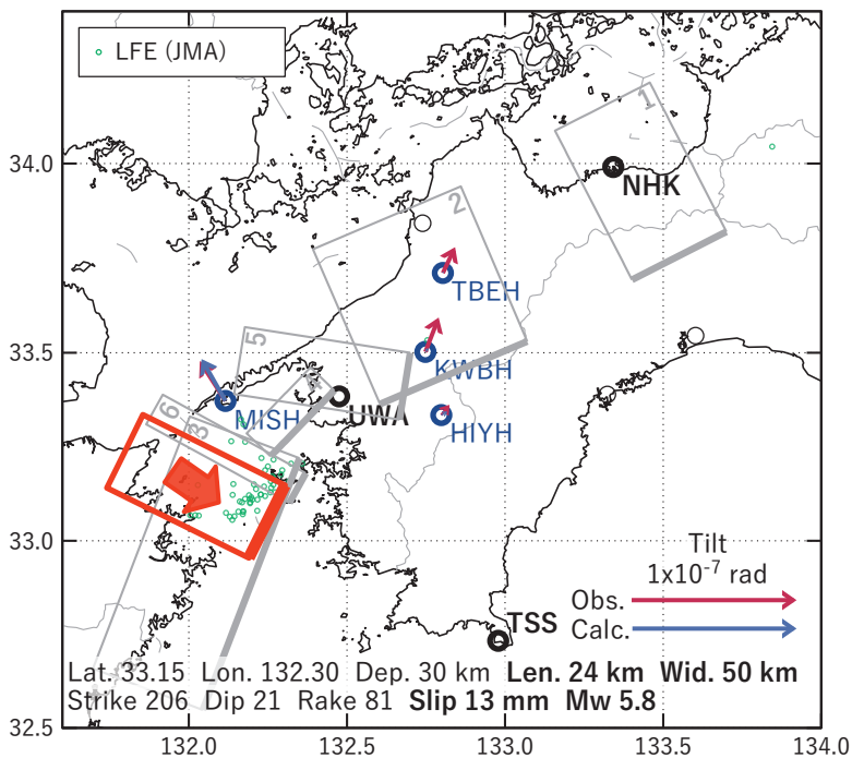
図9 2022/03/19PM-21AMの歪・傾斜変化（図8[A]）を説明する断層モデル。
