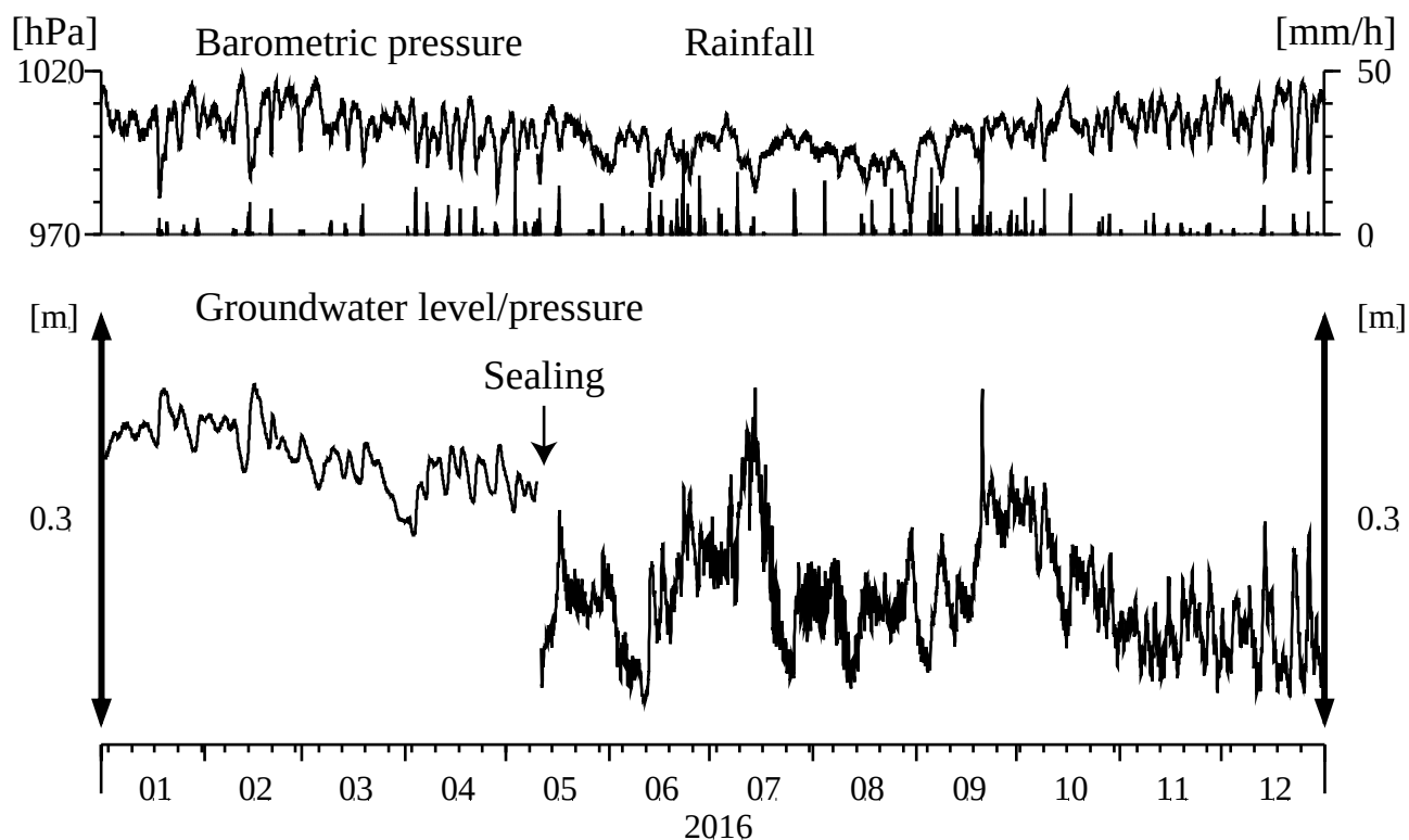
図3 2016年の北勢観測点の気圧・雨量・内管の地下水位（地下水压） 2016年5月11日にパッカーで内管を密閉した。密閉後は地下水压を測定しているが、地下水位に換算してグラフ化している。
