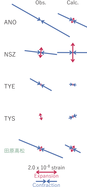
図5 2021/05/09PM-12の歪・傾斜・地下水変化（図2-4[A]）を説明する断層モデル。
