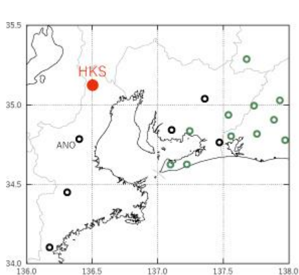
図1 北勢観測点 (HKS) の位置 ○ 産総研の観測点 ○ 気象庁・静岡県の観測点
