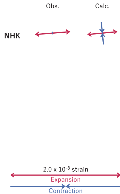
図6 2021/03/19-22 の歪・傾斜変化（図5[A]）を説明する断層モデル。
