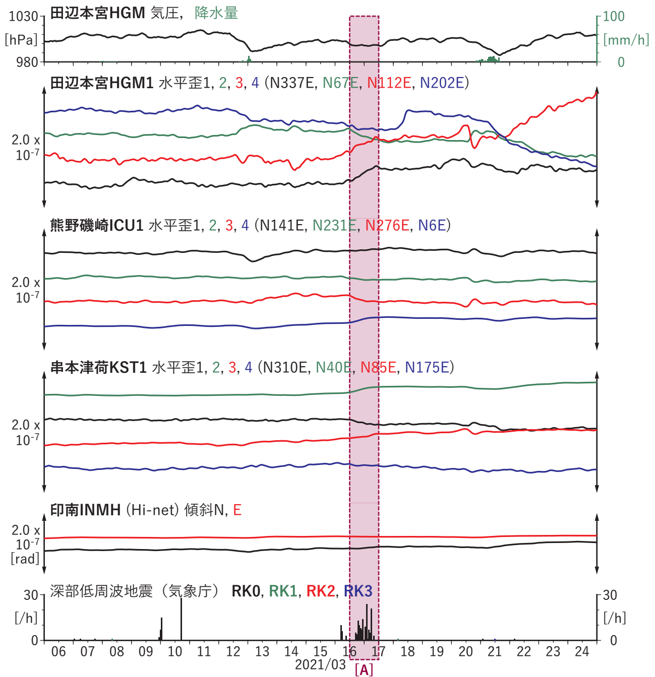
図2 歪・傾斜の時間変化 (2021/03/06 00:00 - 2021/03/25 00:00 (JST))
