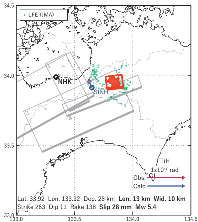
図6 2021/03/19-22 の歪・傾斜変化（図5[A]）を説明する断層モデル。
