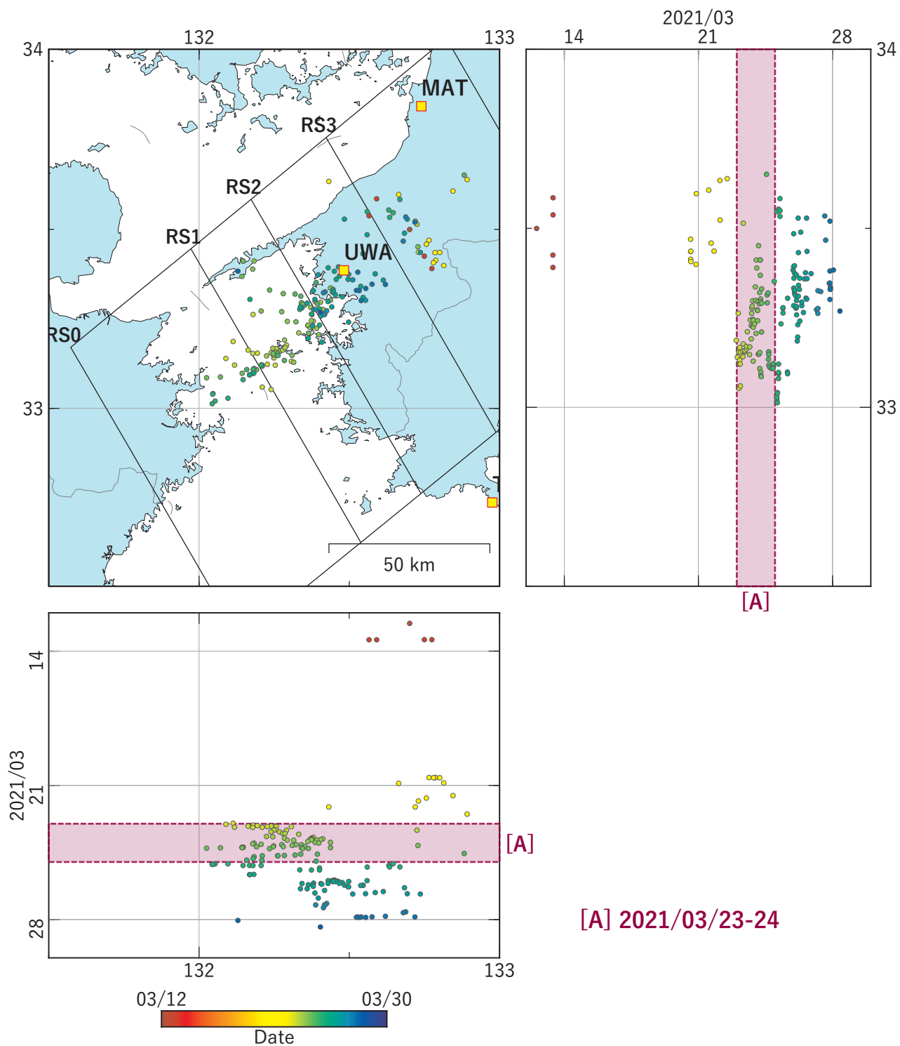
図7 四国における深部低周波地震の時空間分布図。 (2021/03/12 00:00 - 2021/03/30 00:00 (JST)) 気象庁カタログによる。
