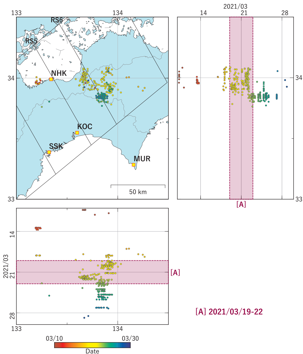
図4 四国における深部低周波地震の時空間分布図。 (2021/03/10 00:00 - 2021/03/30 00:00 (JST)) 気象庁カタログによる。
