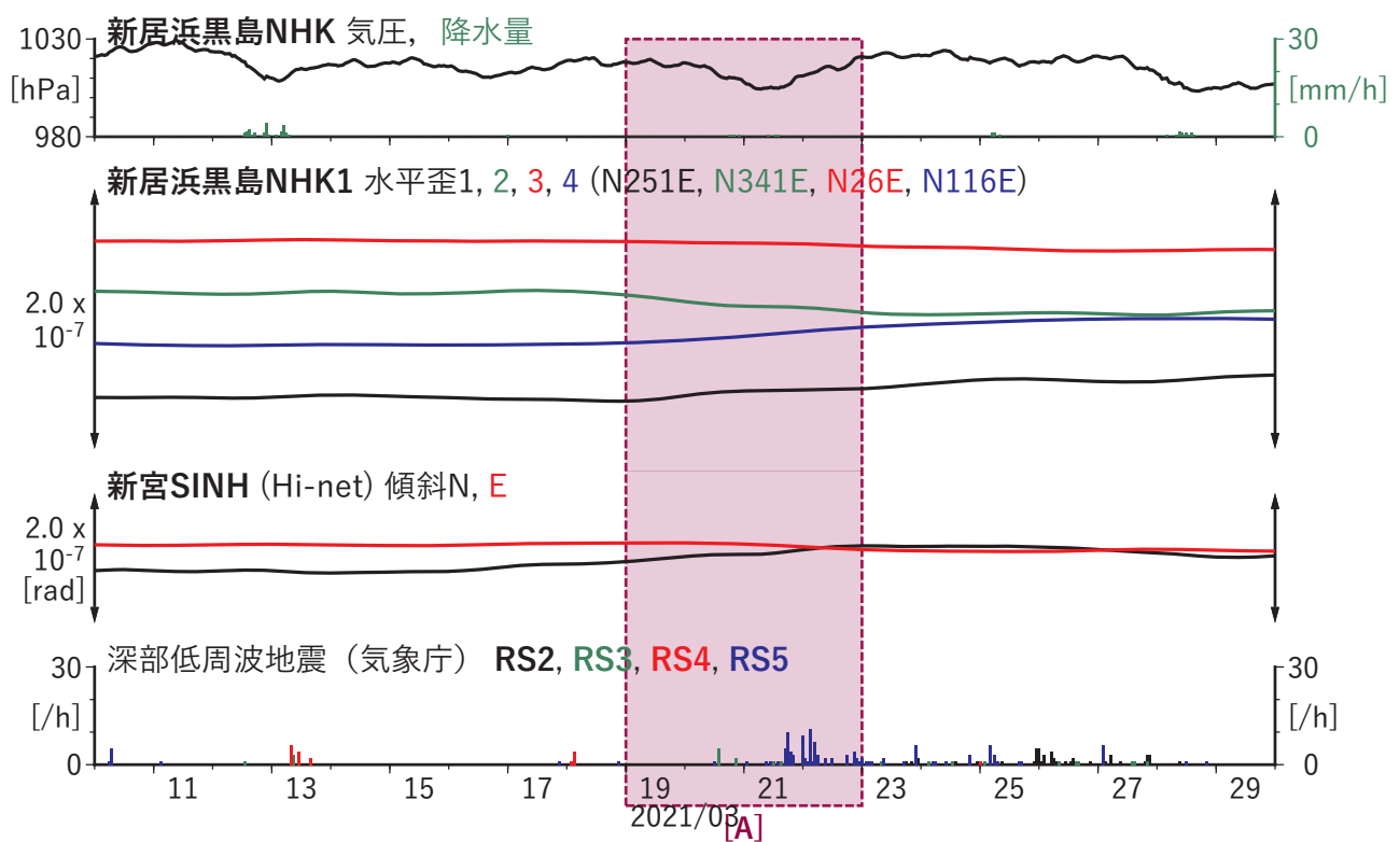
図5 歪・傾斜の時間変化 (2021/03/10 00:00 - 2021/03/30 00:00 (JST))
