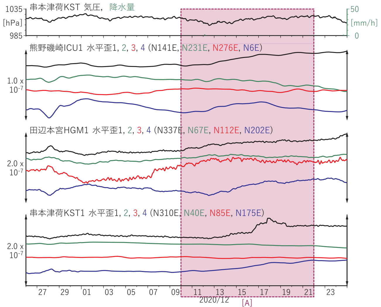
図10 紀伊半島における歪・傾斜観測結果 (2020/11/26 00:00 - 2020/12/25 00:00 (JST))
