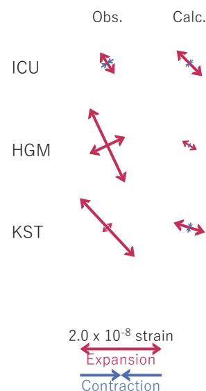
図7 2020/12/10-21の歪・傾斜変化（図5[A]）を説明する断層モデル。
