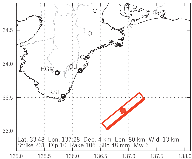
図7 2020/12/10-21の歪・傾斜変化（図5[A]）を説明する断層モデル。
