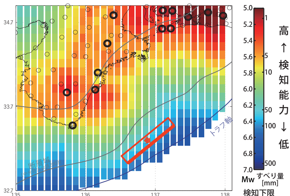
図8 プレート境界面におけるすべりの検知能力。プレート境界面上の20×20kmの断層面がゆっくりとすべった際に、陸上の3観測点3点以上でノイズレベル以上の変化が観測される下限のすべりを示している。陸上観測点は、産総研のボアホール多成分歪・傾斜、地下水（間隙水圧）観測点に加えて、気象庁のボアホール多成分歪・体積歪および防災科研Hi-net高感度化速度計（傾斜）観測点を使用。図7の断層面（赤色矩形）周辺の検知能力はMw6.2~6.4程度である。
