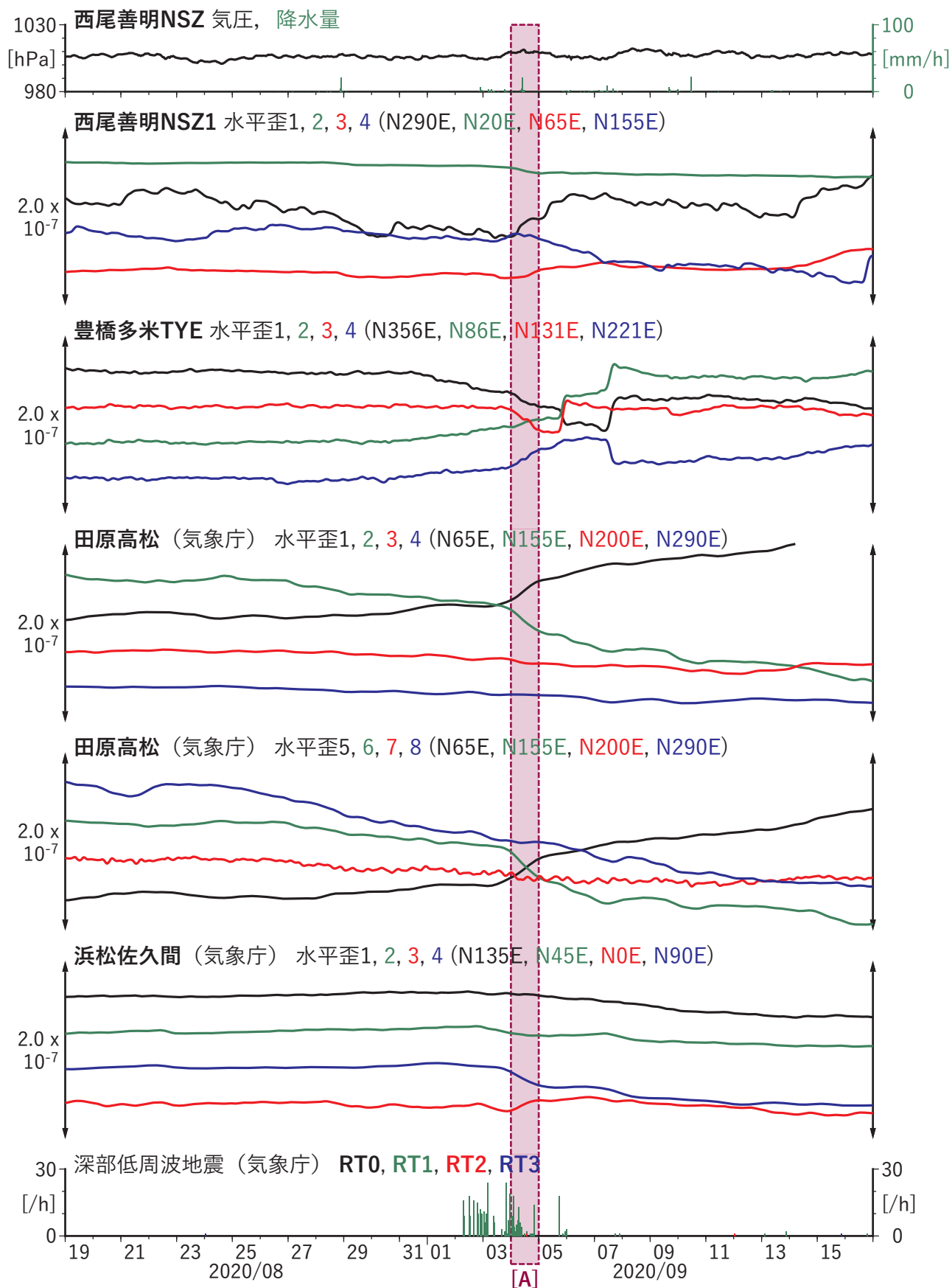
図02 歪の時間変化 (2020/08/19 00:00 - 2020/09/17 00:00 (JST))
