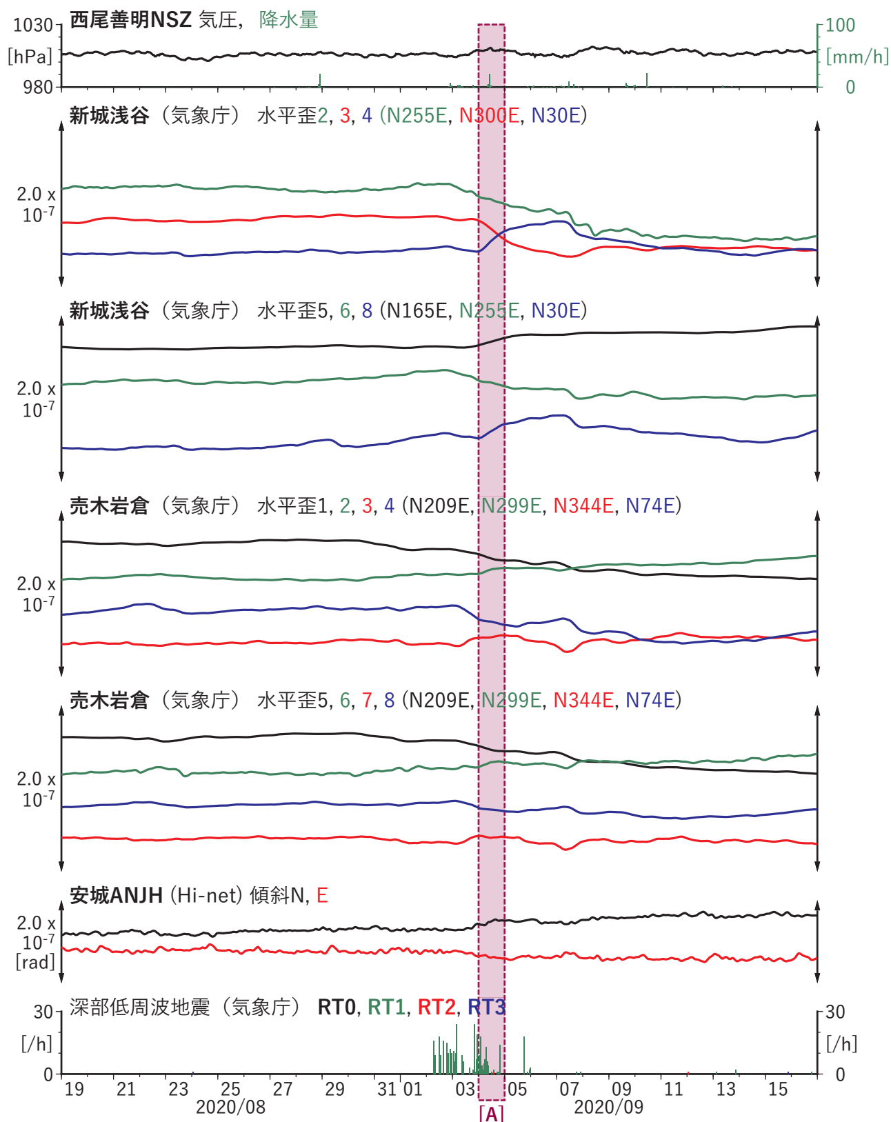
図03 歪・傾斜の時間変化 (2020/08/19 00:00 - 2020/09/17 00:00 (JST))
