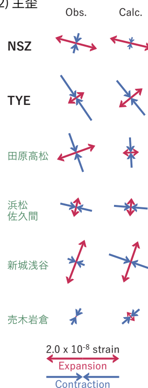
図04 2020/09/04 の歪・傾斜変化（図02-03[A]）を説明する断層モデル。
