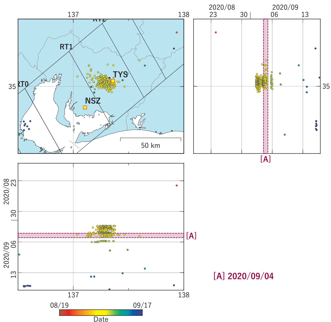
図01 東海地方における深部低周波地震の時空間分布図。 (2020/08/19 00:00 - 2020/09/17 00:00 (JST)) 気象庁カタログによる。
