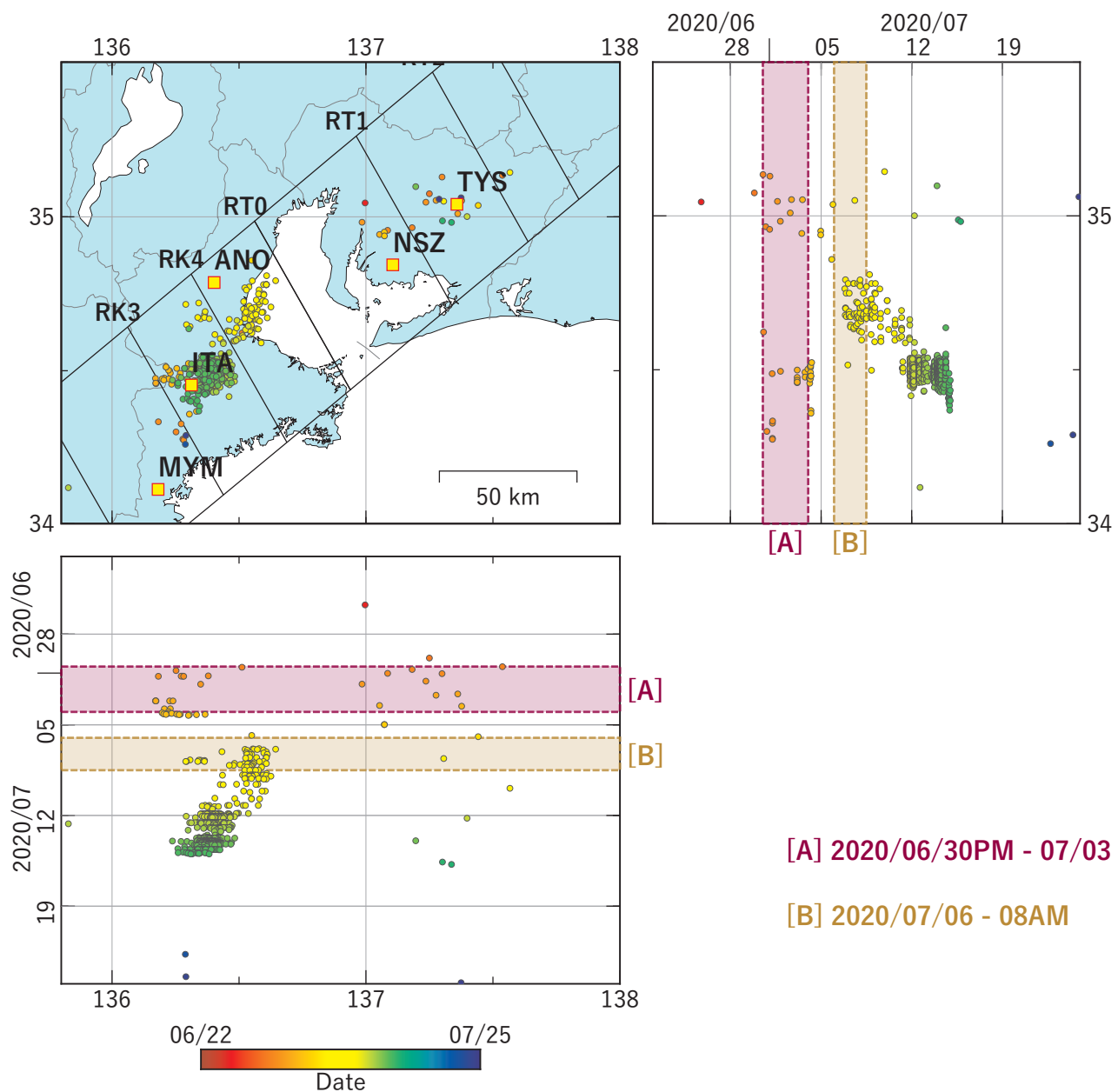
図1 紀伊半島から東海地方における深部低周波地震の時空間分布図。 (2020/06/22 00:00 - 2020/07/25 00:00 (JST)) 気象庁カタログによる。
