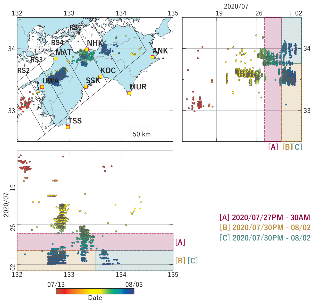
図5 四国地方における深部低周波地震の時空間分布図。 (2020/07/13 00:00 - 2020/08/03 00:00 (JST)) 気象庁カタログによる。
