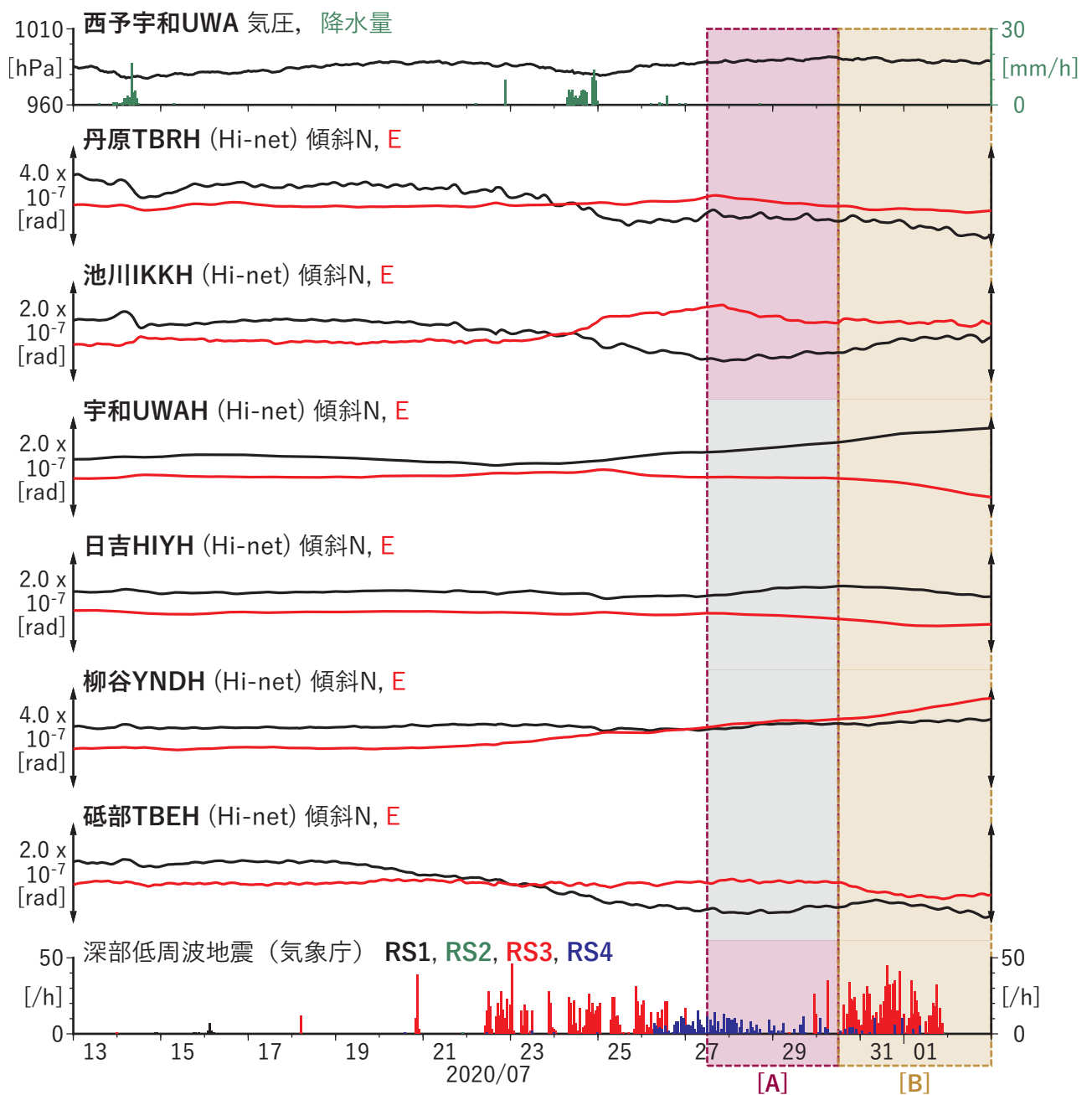
図7 傾斜の時間変化 (2020/07/13 00:00 - 2020/08/03 00:00 (JST))
