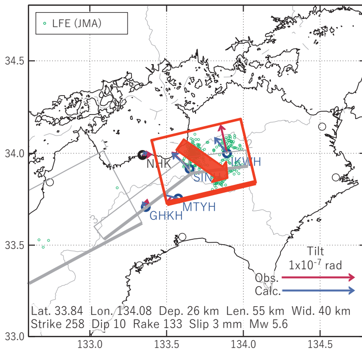
図3 2020/01/01-03の歪・傾斜変化（図2[A]）を説明する断層モデル。
