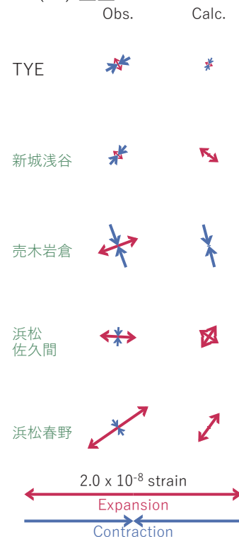
図7 2020/01/13-14AMの歪変化（図5[B]）を説明する断層モデル。
