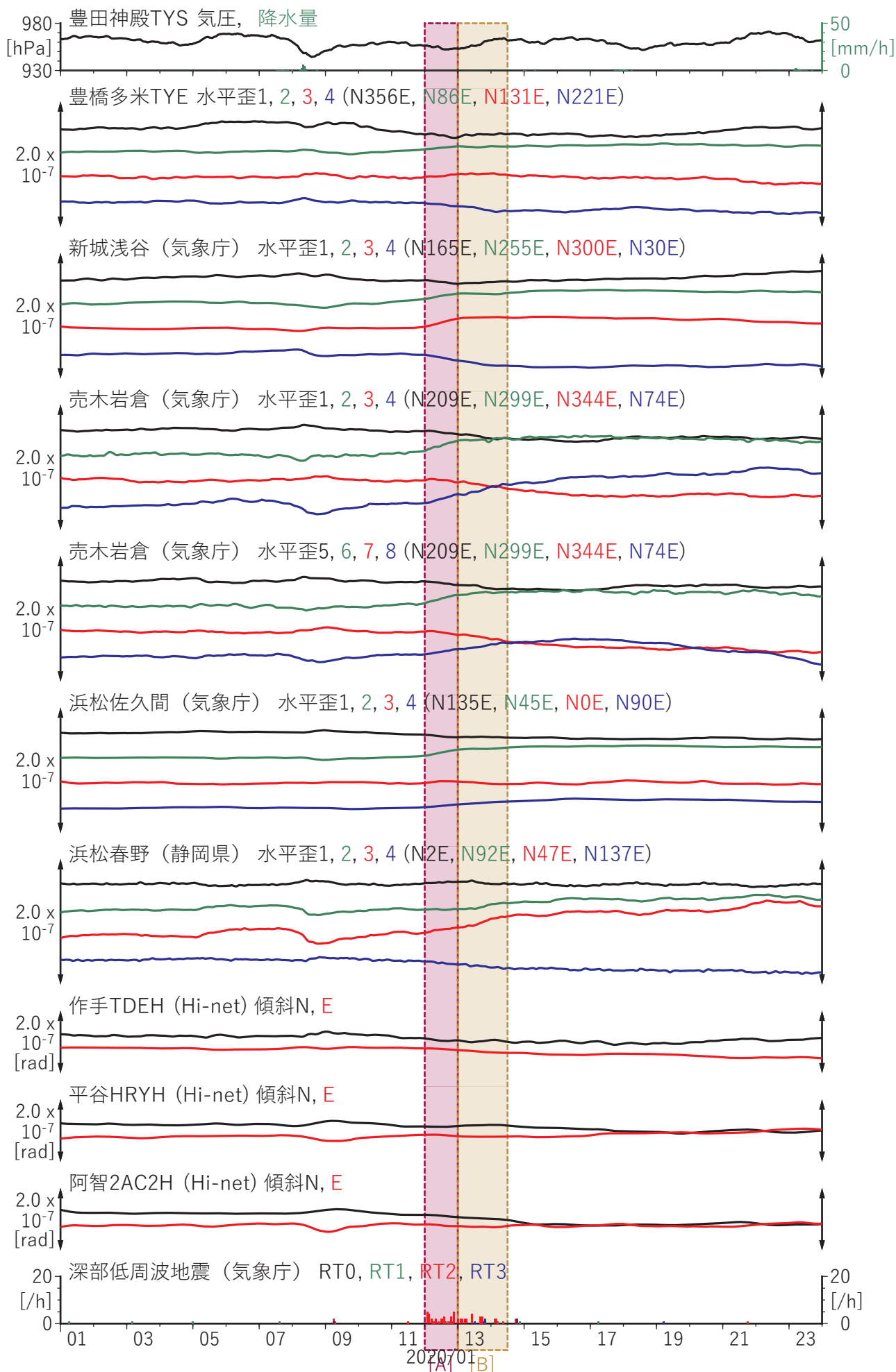
図5 東海地方における歪観測結果 (2020/01/01 00:00 - 2020/01/23 00:00 (JST))
