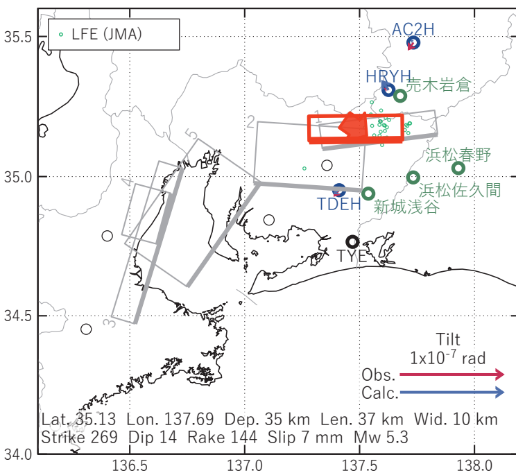
図6 2020/01/12の歪変化（図5[A]）を説明する断層モデル。
