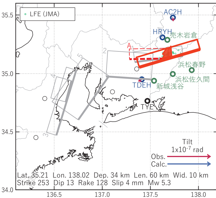
図7 2020/01/13-14AMの歪変化（図5[B]）を説明する断層モデル。
