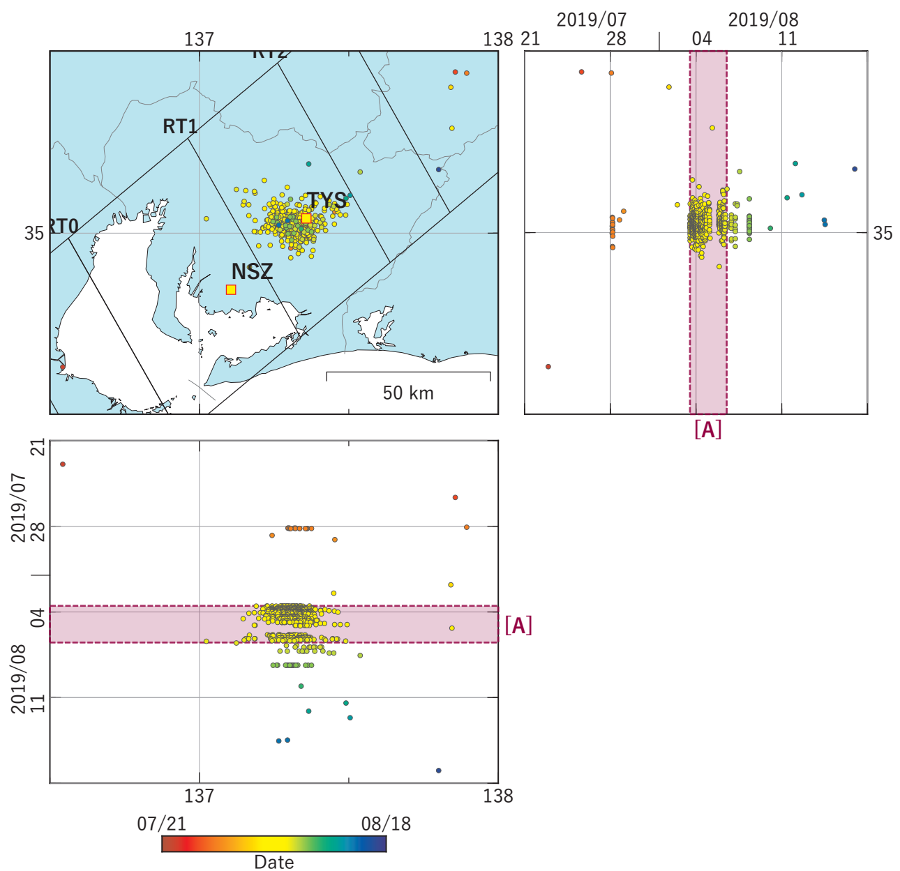
図1 東海地方における深部低周波地震（気象庁）の時空間分布図 (2019/07/21 00:00 - 2019/08/18 00:00 (JST)) (観測点) NSZ：西尾善明 TYS：豊田神殿
