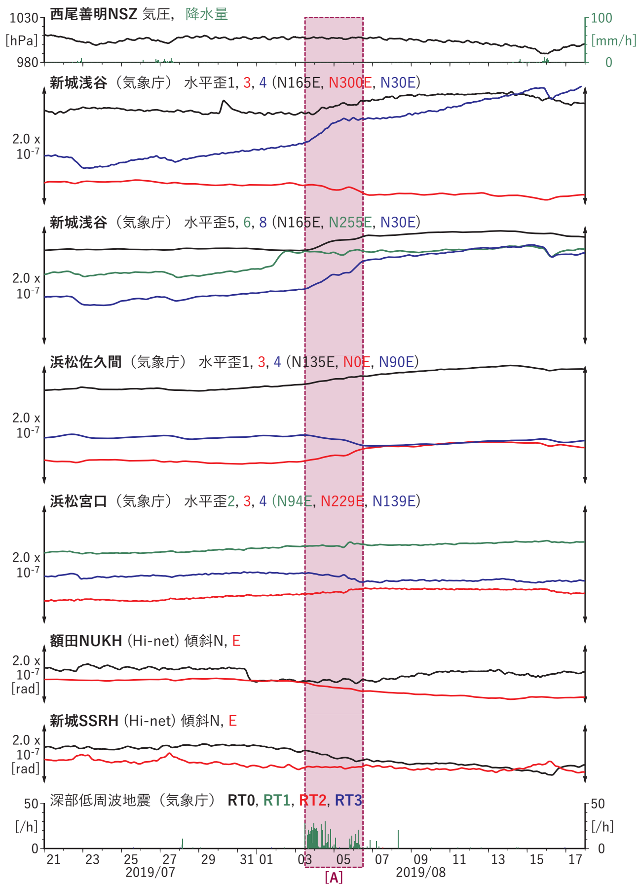
図2 (続) 東海地方における歪・傾斜観測結果 (2019/07/21 00:00 - 2019/08/18 00:00 (JST))
