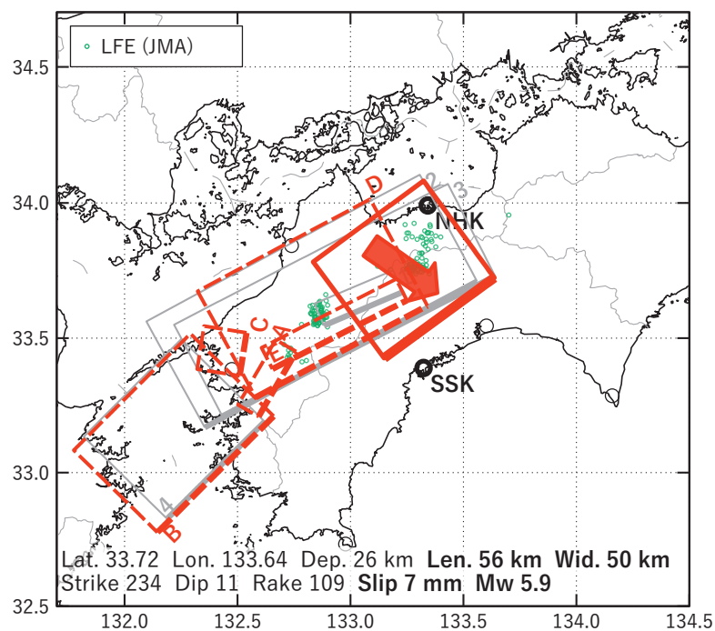
図12 2019/08/14-15の歪・傾斜変化（図6[F]）を説明する断層モデル。
