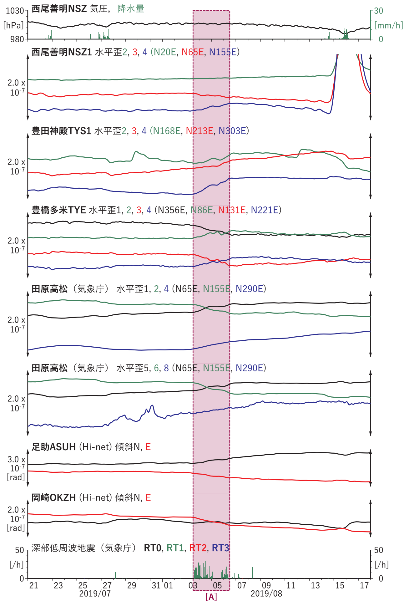
図2 東海地方における歪・傾斜観測結果 (2019/07/21 00:00 - 2019/08/18 00:00 (JST))
