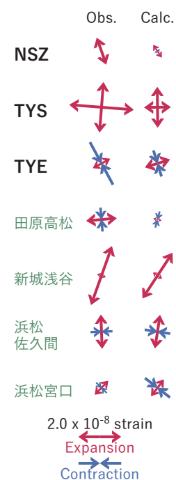
図3 2019/08/03PM-06AMの歪・傾斜変化（図2[A]）を説明する断層モデル。
