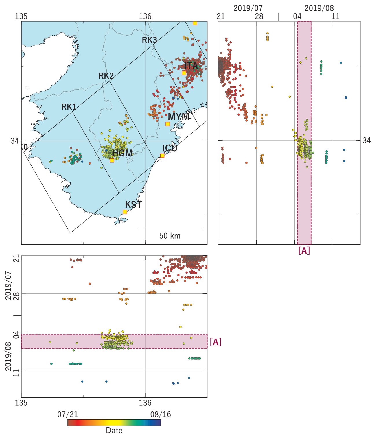
図13 紀伊半島における深部低周波地震（気象庁）の時空間分布図 (2019/07/21 00:00 - 2019/08/16 00:00 (JST)) (観測点) HGM: 田辺本宮, KST: 串本津荷, ICU: 熊野磯崎 MYM: 紀北海山
