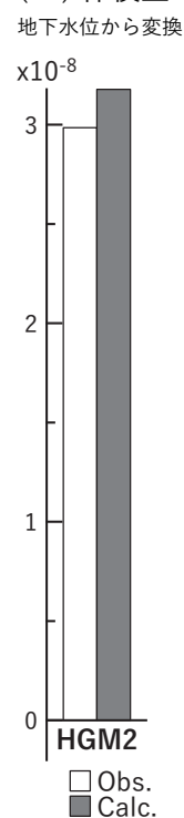
図6 2019/01/19PM-24AMの歪・傾斜・地下水位変化（図5[A]）を説明する断層モデル。
