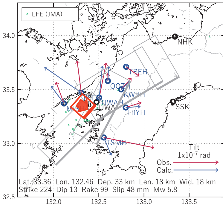
図9 2018/09/29PM-10/01AMの歪・傾斜変化（図8[A]）を説明する断層モデル。
