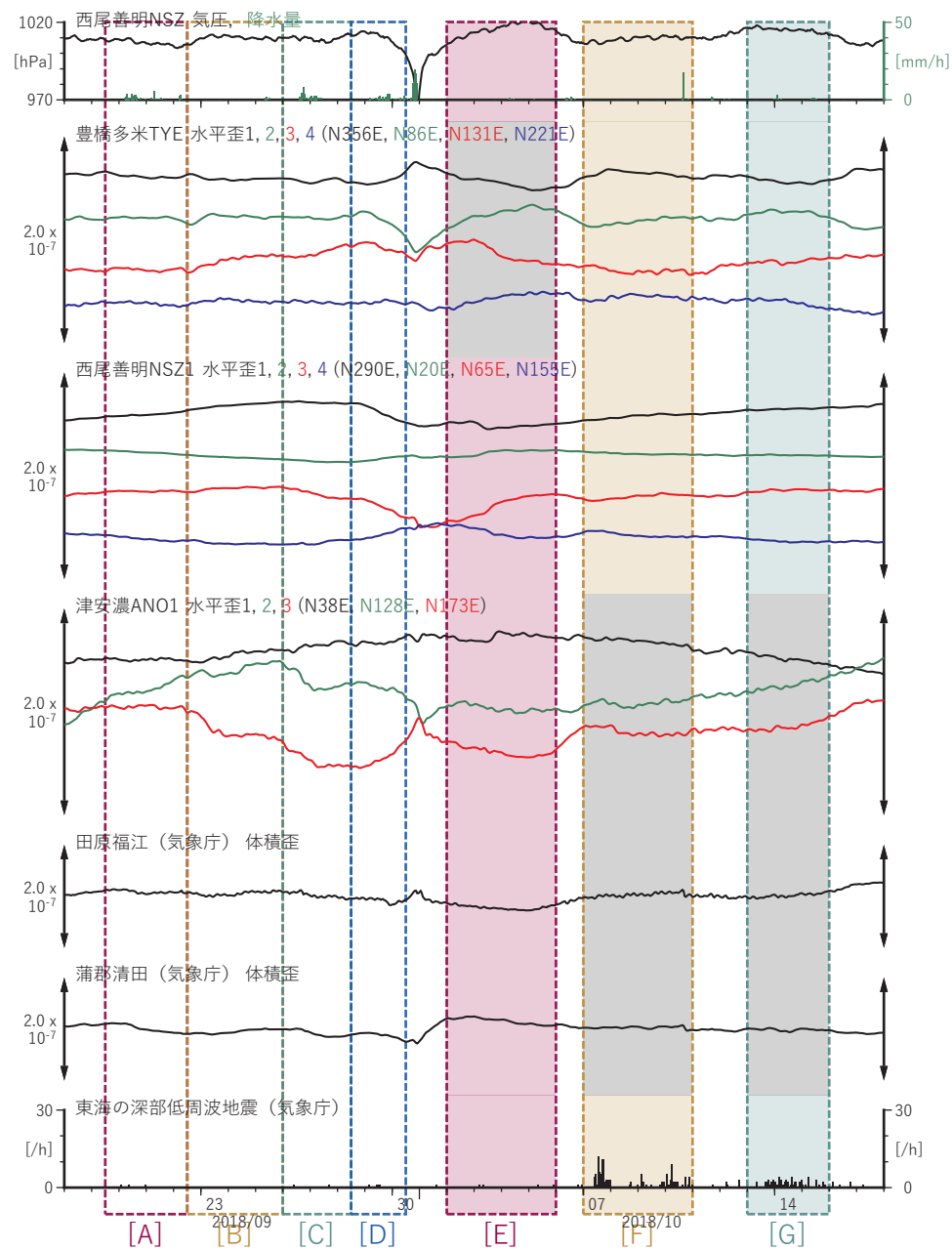
図2 歪・傾斜の時間変化(1) (2018/09/18 00:00 - 2018/10/18 00:00 (JST))
