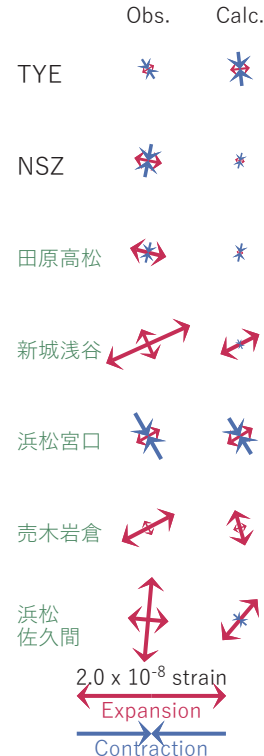
図5 2018/10/07-10の歪・傾斜変化 (図2.3[F]) を説明する断層モデル。
